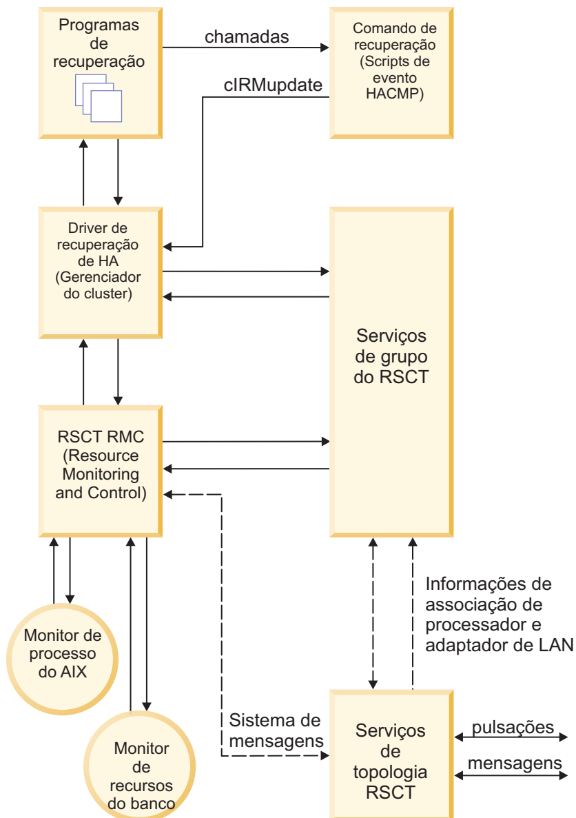
Figura 10. Componentes da arquitetura do PowerHA SystemMirror
