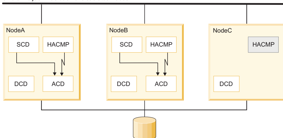
Sincronização 3: Reconfiguração dinâmica completa; serviços de cluster iniciados no NodeC
