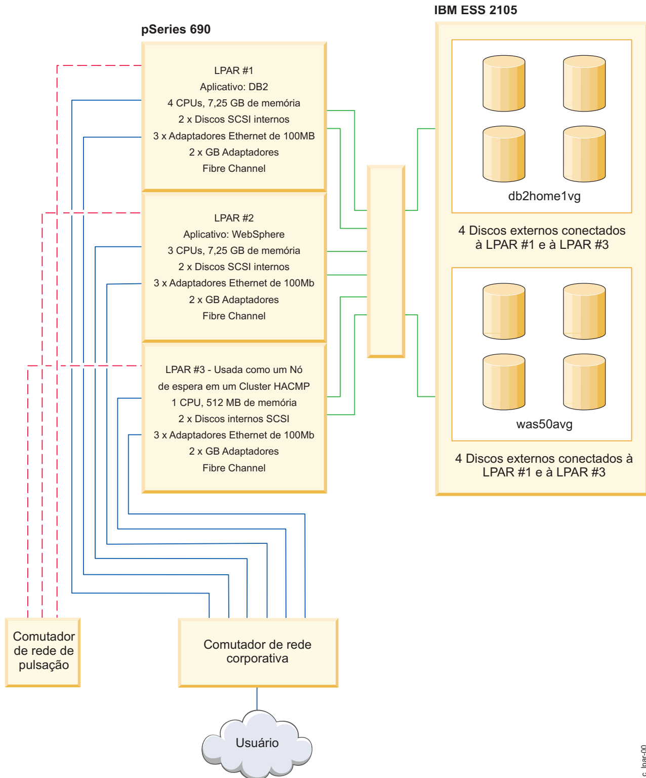
Figura 31. Cluster com três LPARs
