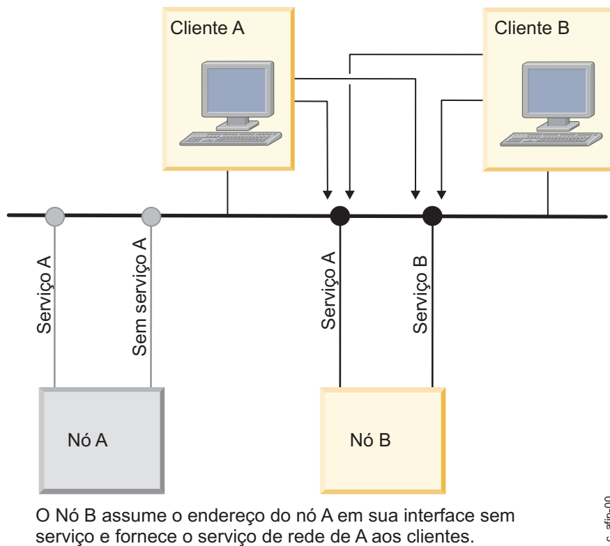
Figura 14. Configuração após controle de endereço IP por meio de substituição de IP
