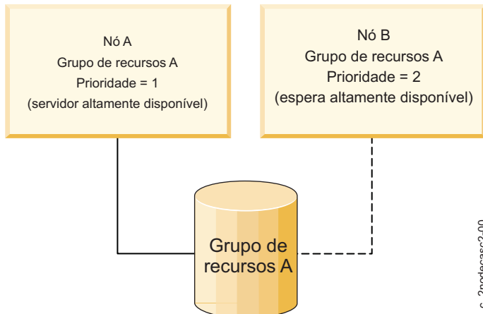
Figura 24. Configuração de controle unilateral com grupos de recursos nos quais o rótulo de IP retorna ao nó inicial
