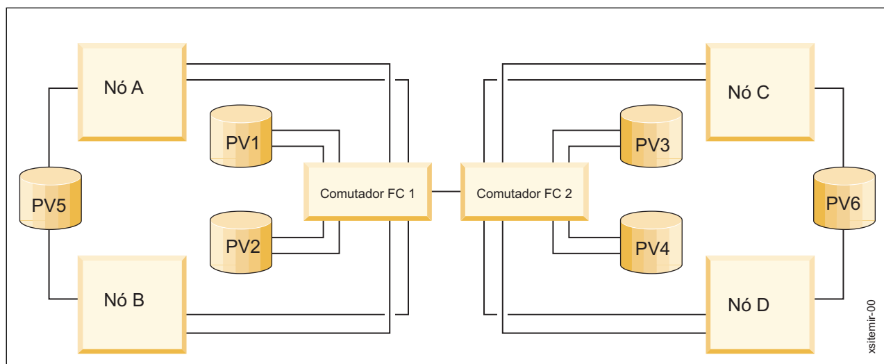
Figura 30. Configuração de espelhamento do LVM entre sites com uma SAN
