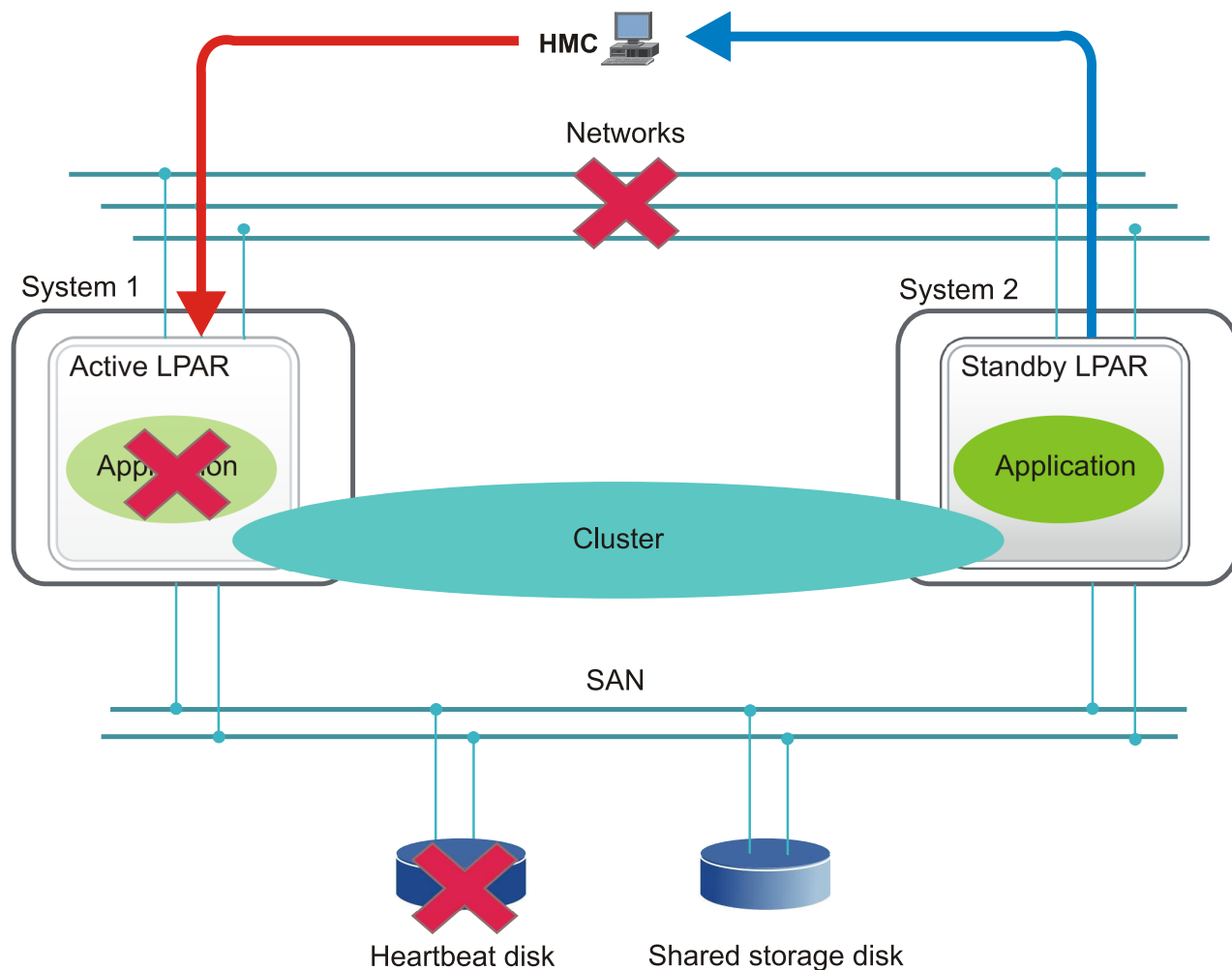
Figura 3. Política de interrupção do nó ativo
