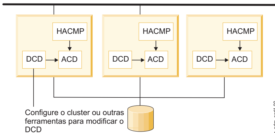
Figura 19. Relacionamento do PowerHA SystemMirror com o ACD quando um cluster é iniciado.
