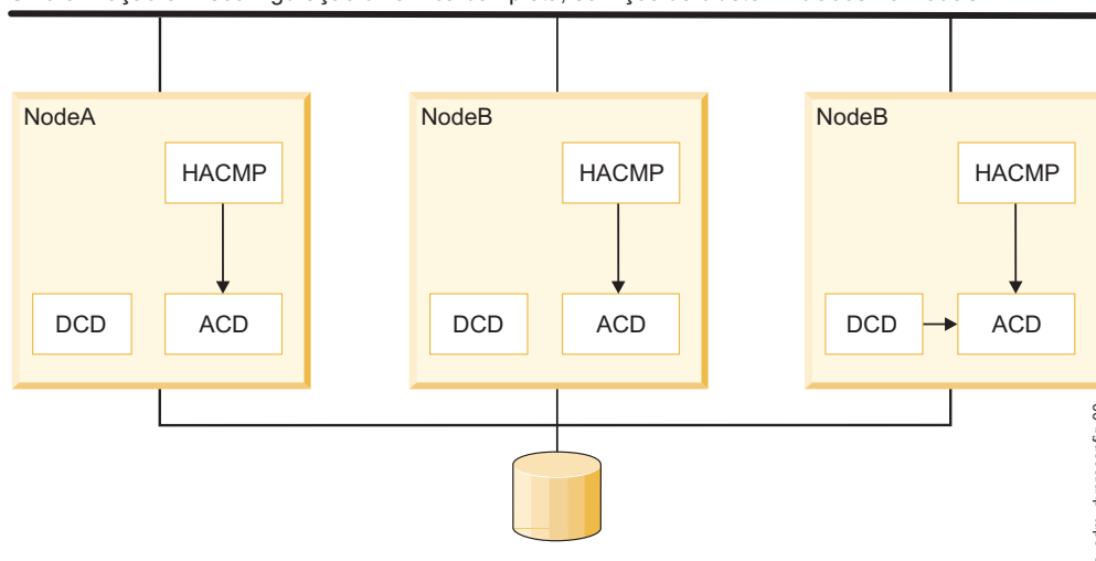
Figura 20. Processamento de reconfiguração dinâmica
