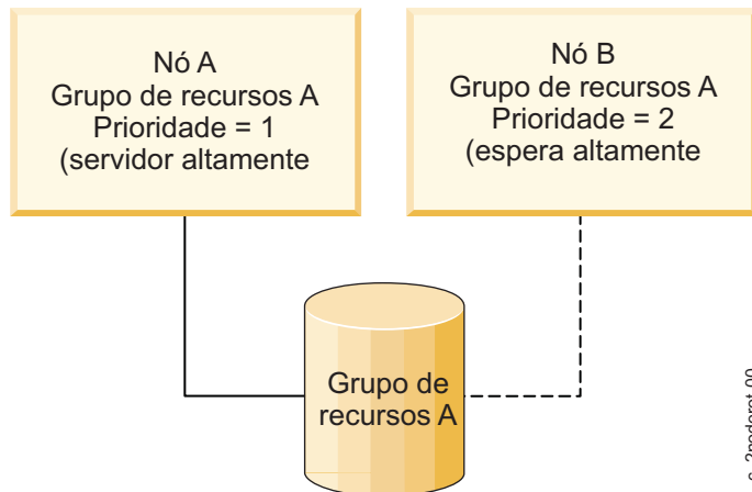
Figura 23. Configuração de espera de um para um com grupos de recursos em que o rótulo de IP gira
