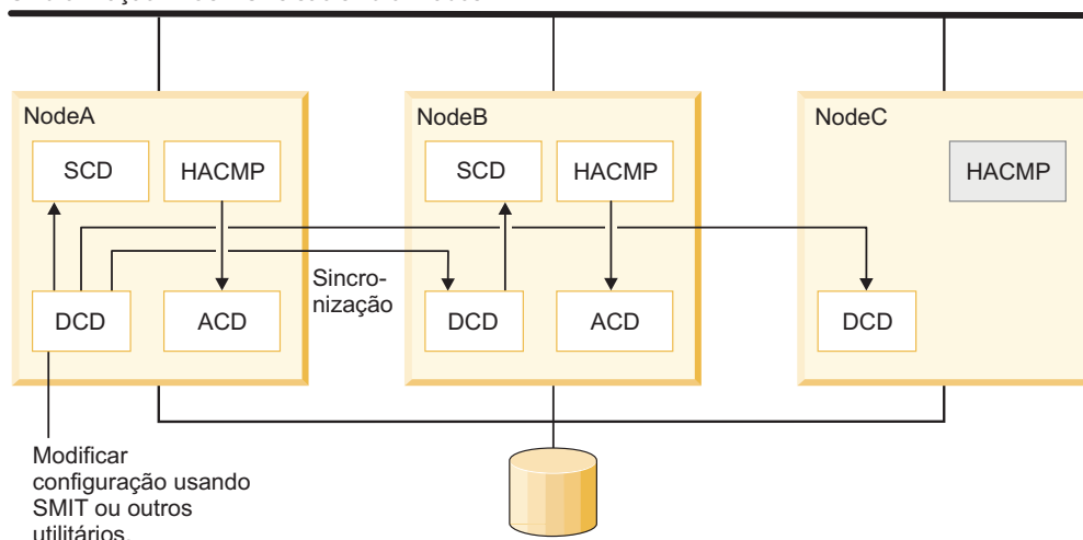
Sincronização 2: Os daemons são atualizados
