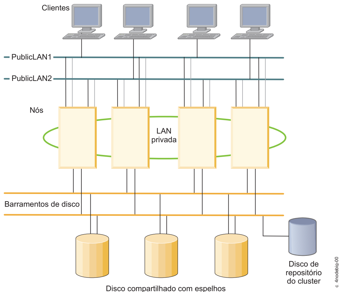
Figura 2. Exemplo de um cluster do PowerHA SystemMirror
