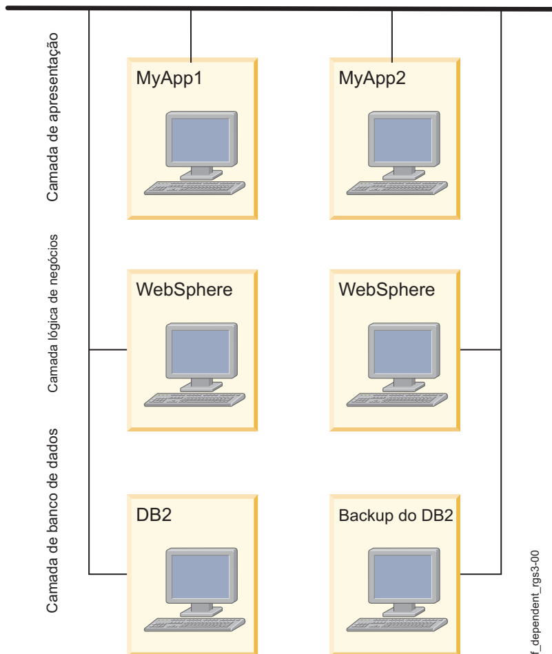
Figura 28. Ambiente em cluster com multicamadas típico com dependências entre aplicativos
