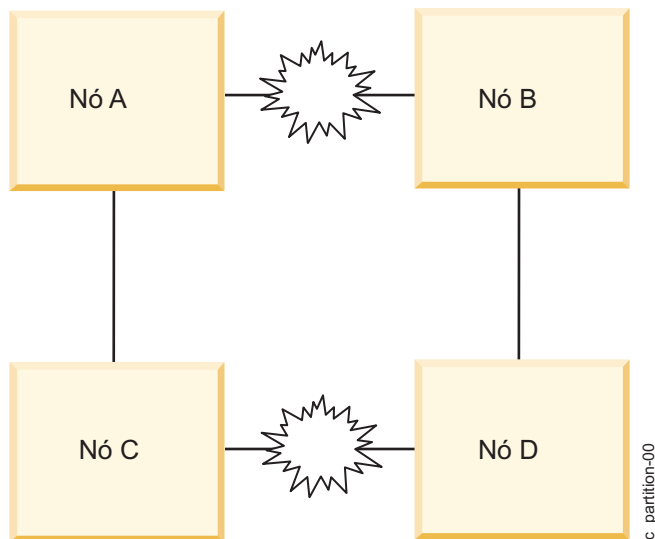
Figura 18. Cluster particionado
