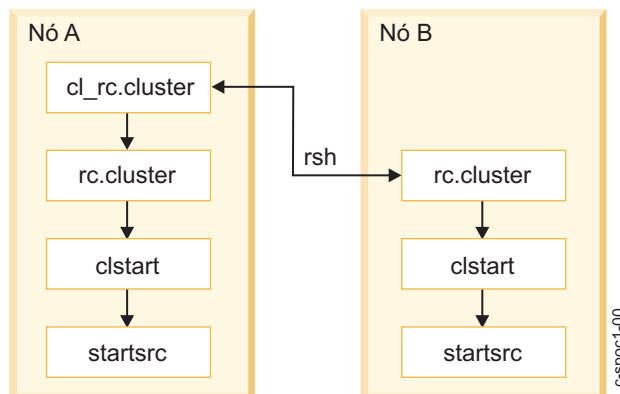
Figura 32. Fluxo de comandos usados na inicialização do cluster pelo utilitário C-SPOC
