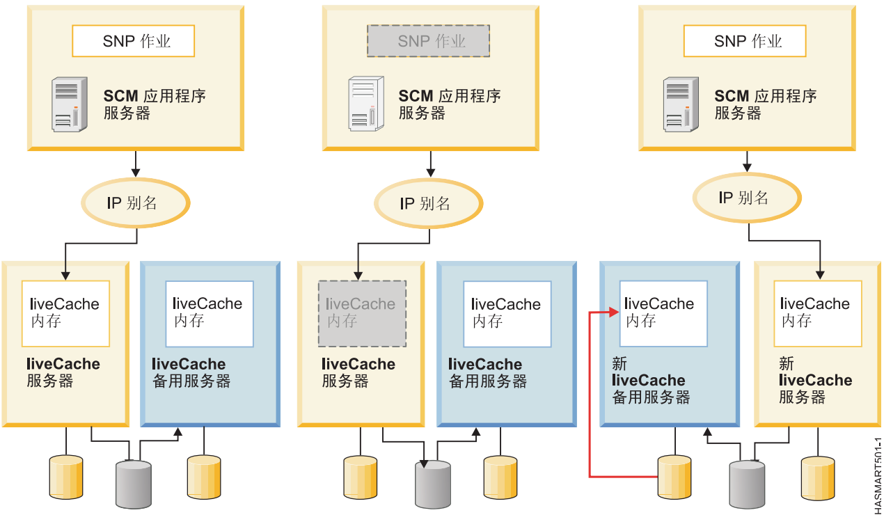
图 13. 运行 SAP liveCache 热备用的双节点集群
