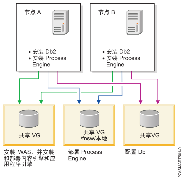
图 8. 双节点安装和配置的示例
