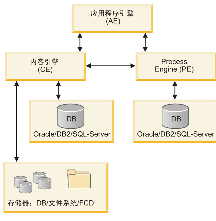
图 7. FileNet P8 体系结构
