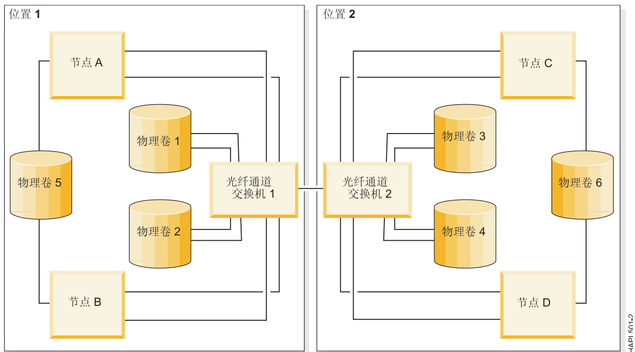
图 8. 使用 SAN 的 LVM 分割站点镜像配置
