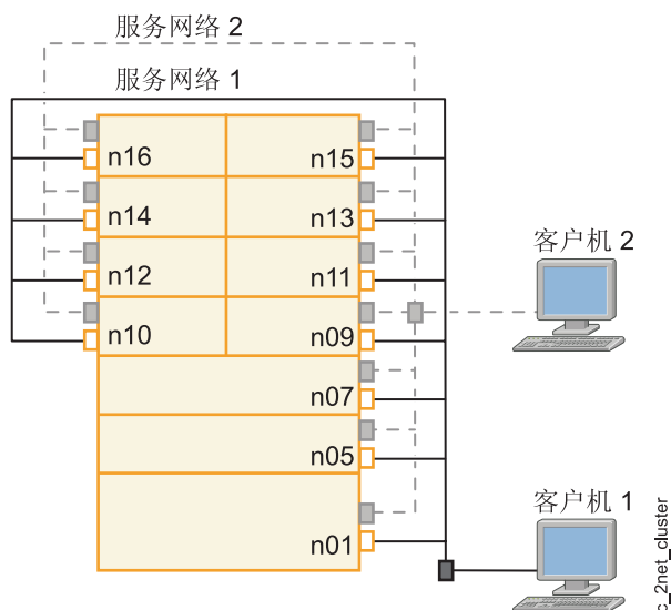
图 2. 双网络设置
