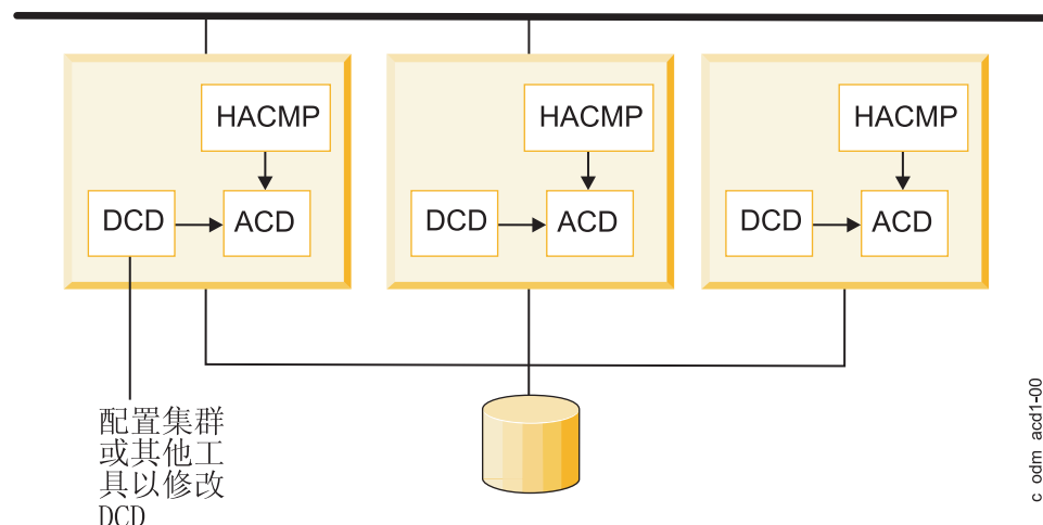
图 19. 当集群启动时，PowerHA SystemMirror 与 ACD 的关系。
