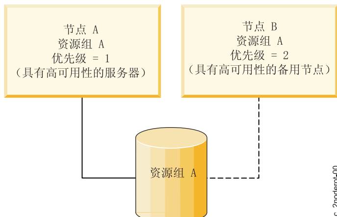
图 23. 具有 IP 标签可切换的资源组的一对一备用配置
