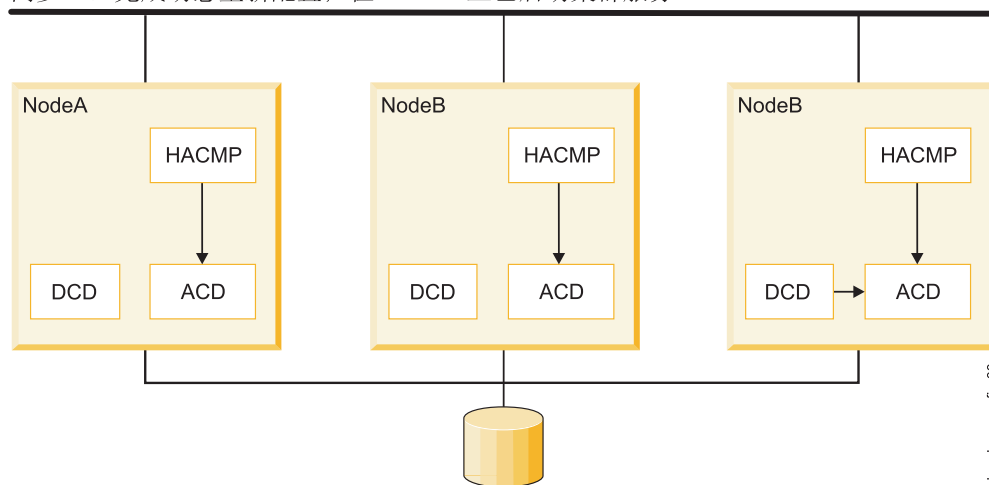
图 20. 动态重新配置处理
