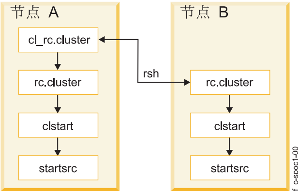
图 32. 集群启动时 C-SPOC 实用程序使用的命令流
