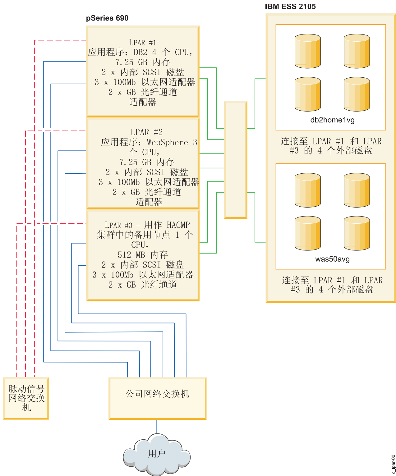
图 31. 具有三个 LPAR 的集群
