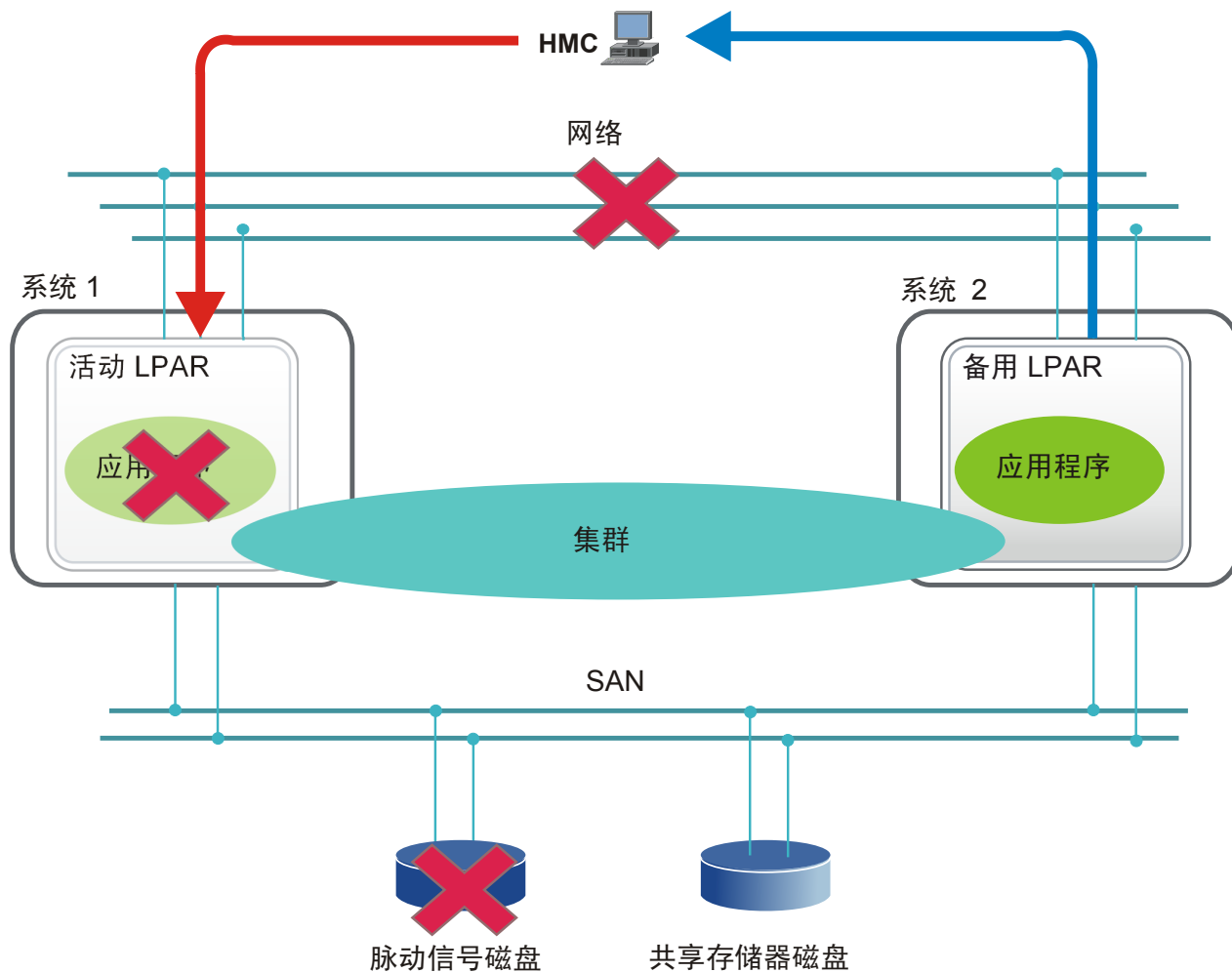
| 图 3. 活动节点暂停策略
