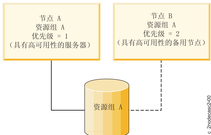
图 24. 资源组中的 IP 标签返回至主节点的单边接管配置
