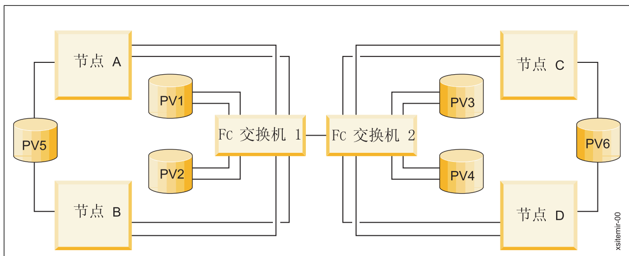
图 30. 使用 SAN 的跨站点 LVM 镜像配置
