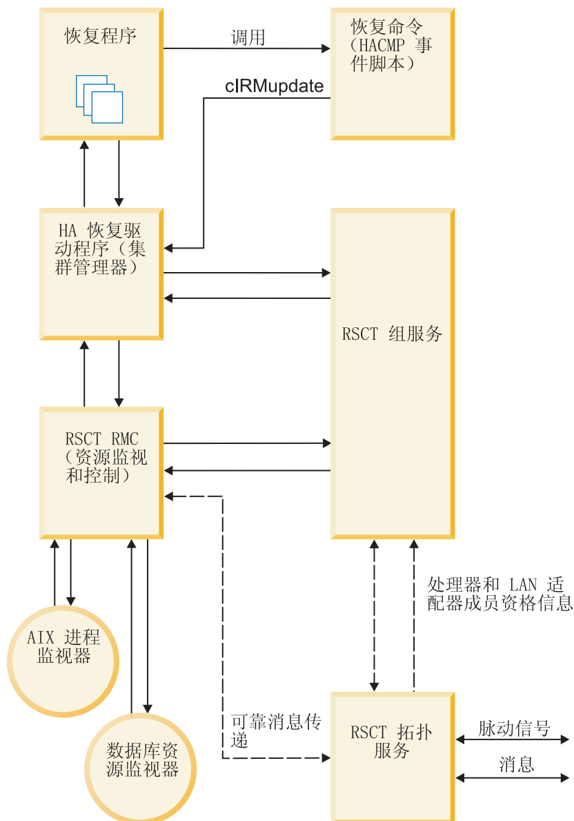
图 10. PowerHA SystemMirror 体系结构的组件
