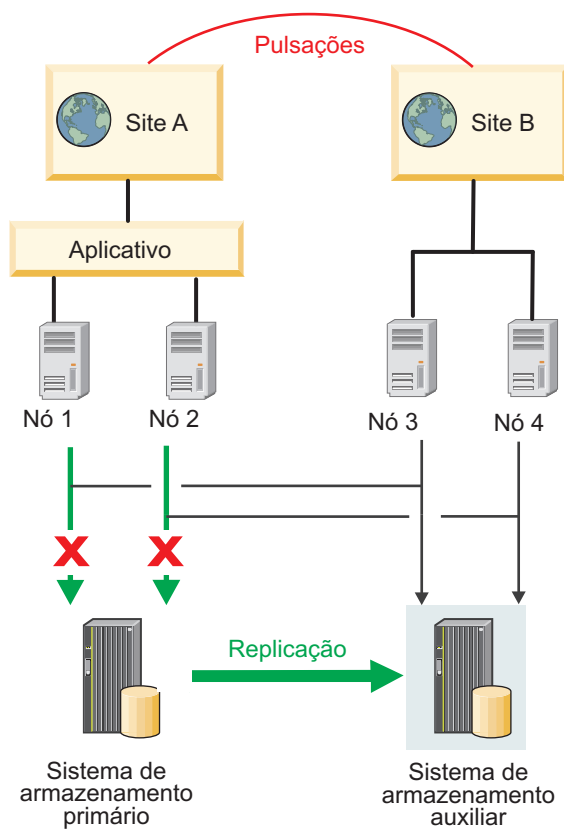
Figura 3. Configuração de HyperSwap não planejado para falha de acesso ao nó
