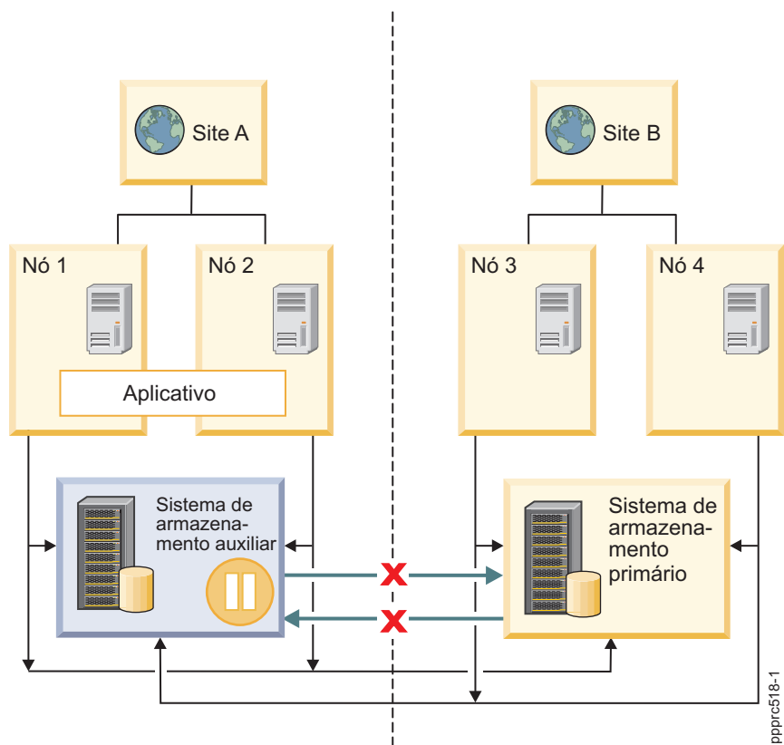
Figura 11. Os caminhos de replicação estão divididos
