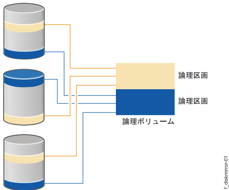
図 7. 3 つのミラー・コピーを備えた 2 つの論理区画の論理ボリューム
