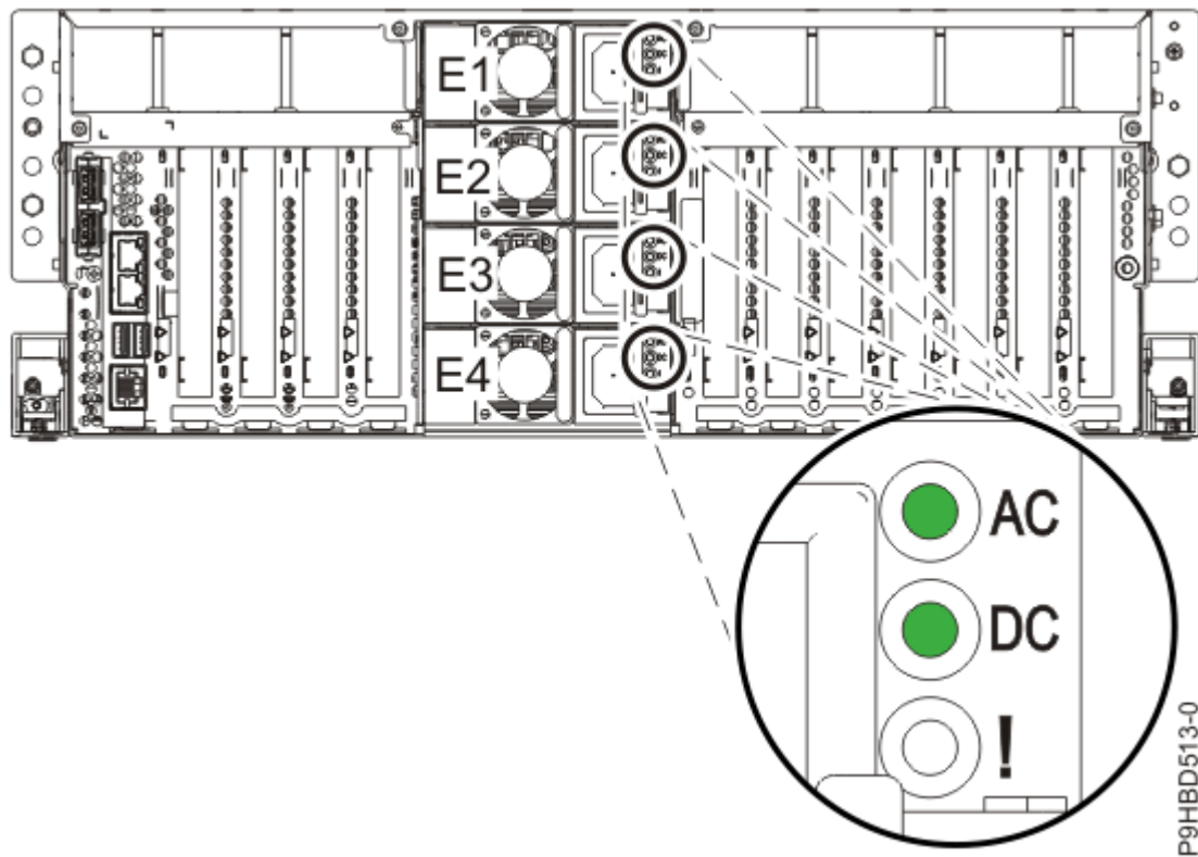
รูปที่ 10. LED สำหรับตัวจ่ายไฟที่ใช้งานอยู่ ระบบที่ประกอบเข้ากับชั้นวาง
