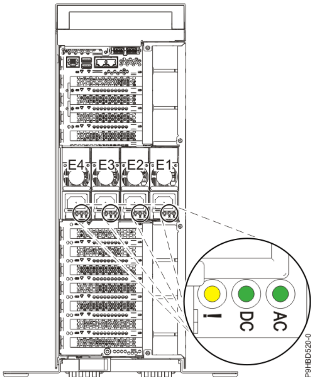
รูปที่ 2. ตำแหน่งของแหล่งจ่ายไฟและ LED ในระบบแบบสแตนด์เอโลน
