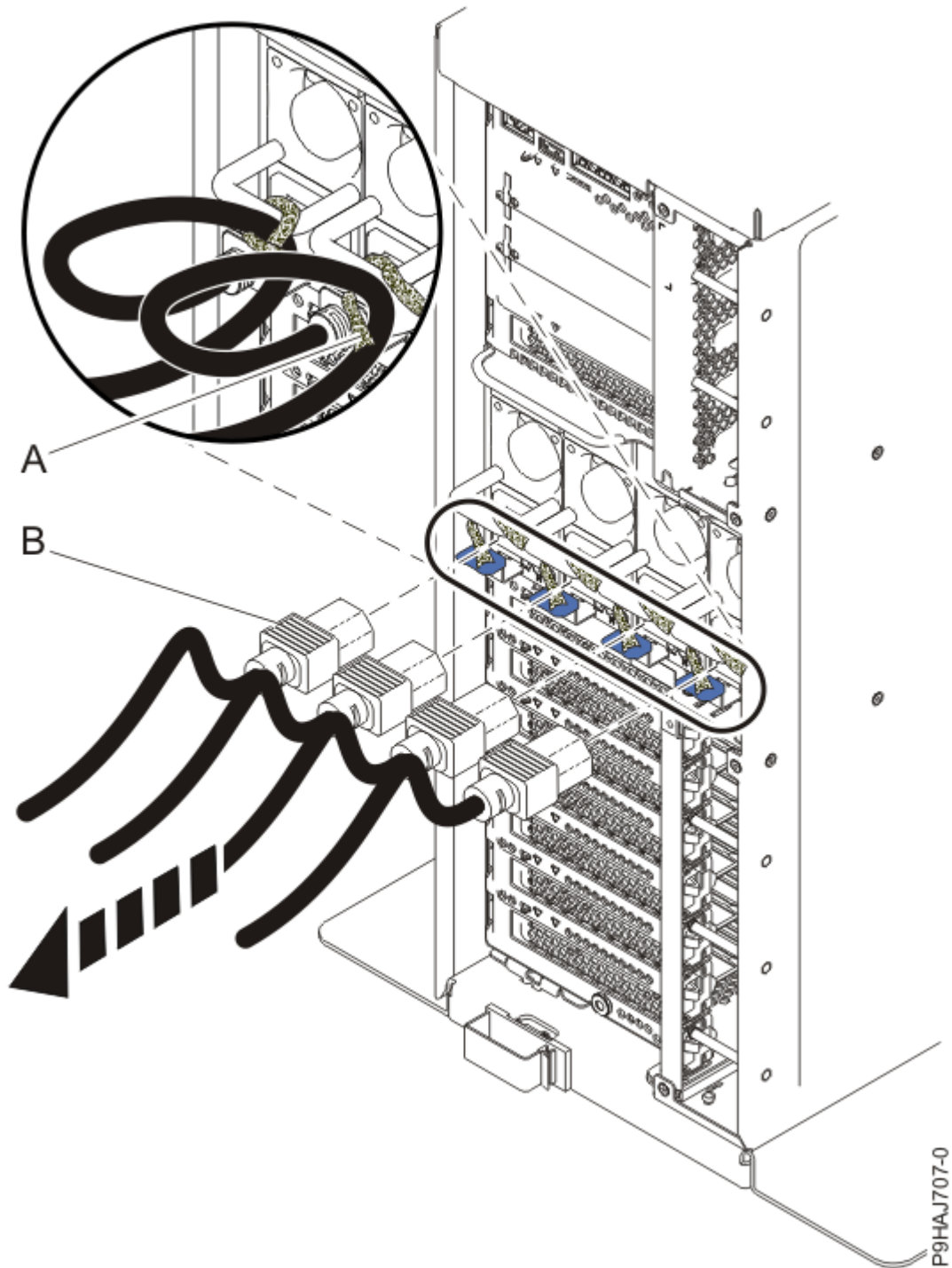
รูปที่ 6. การถอดสายไฟออกจากเซิร์ฟเวอร์แบบสแตนด์อะโลน
