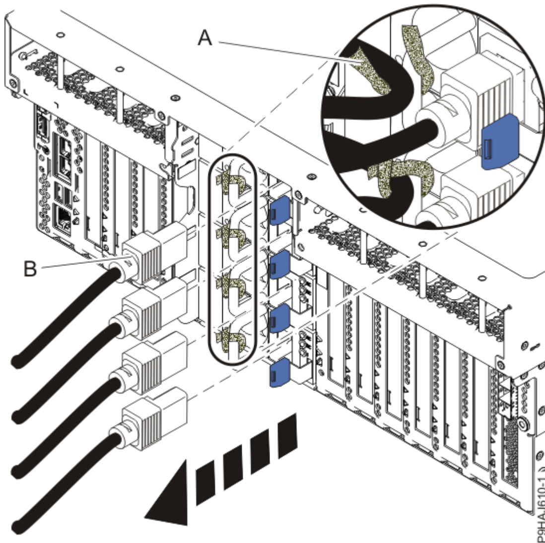
รูปที่ 5. การถอดสายไฟออกจากเซิร์ฟเวอร์ที่ประกอบเข้ากับชั้นวาง
