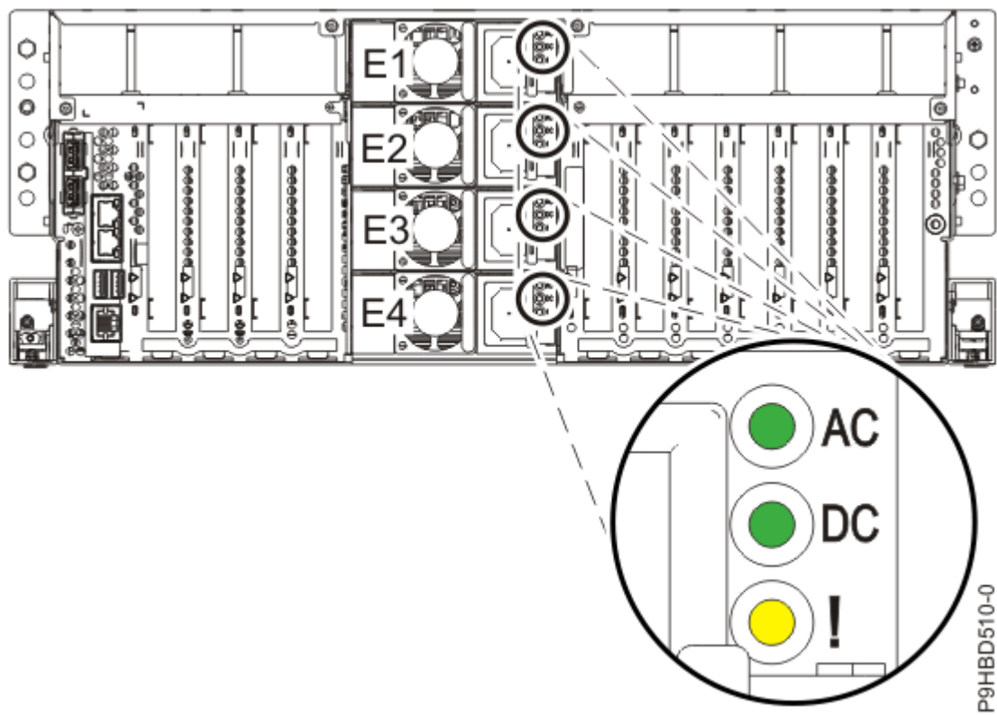
รูปที่ 1. ตำแหน่งของแหล่งจ่ายไฟและ LED ในระบบที่ประกอบเข้ากับชั้นวาง
