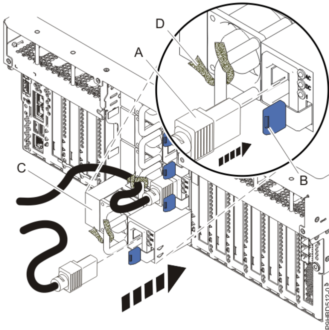
รูปที่ 9. การถอดตัวจ่ายไฟ
