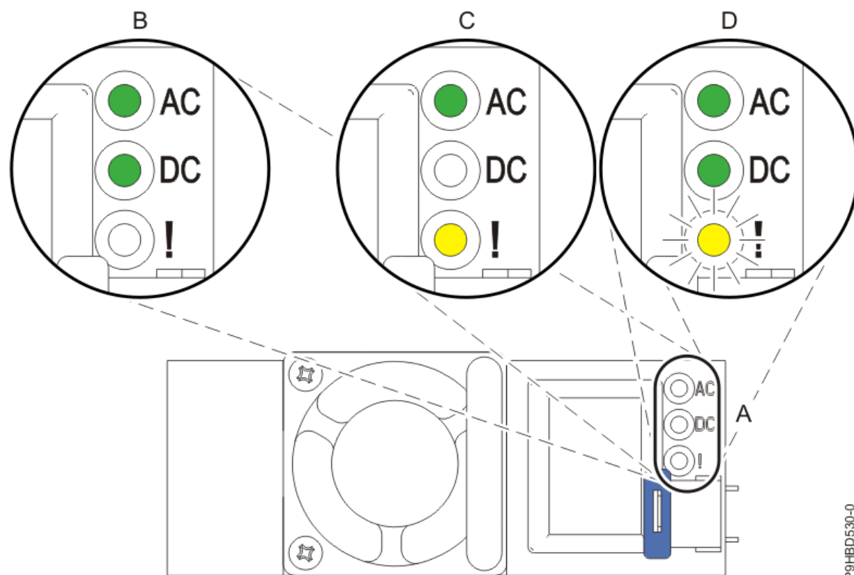
รูปที่ 3. LED สำหรับแหล่งจ่ายไฟ (B) ที่ทำงานและ (C, D) ที่ล้มเหลวในระบบที่ประกอบเข้ากับชั้นวาง
