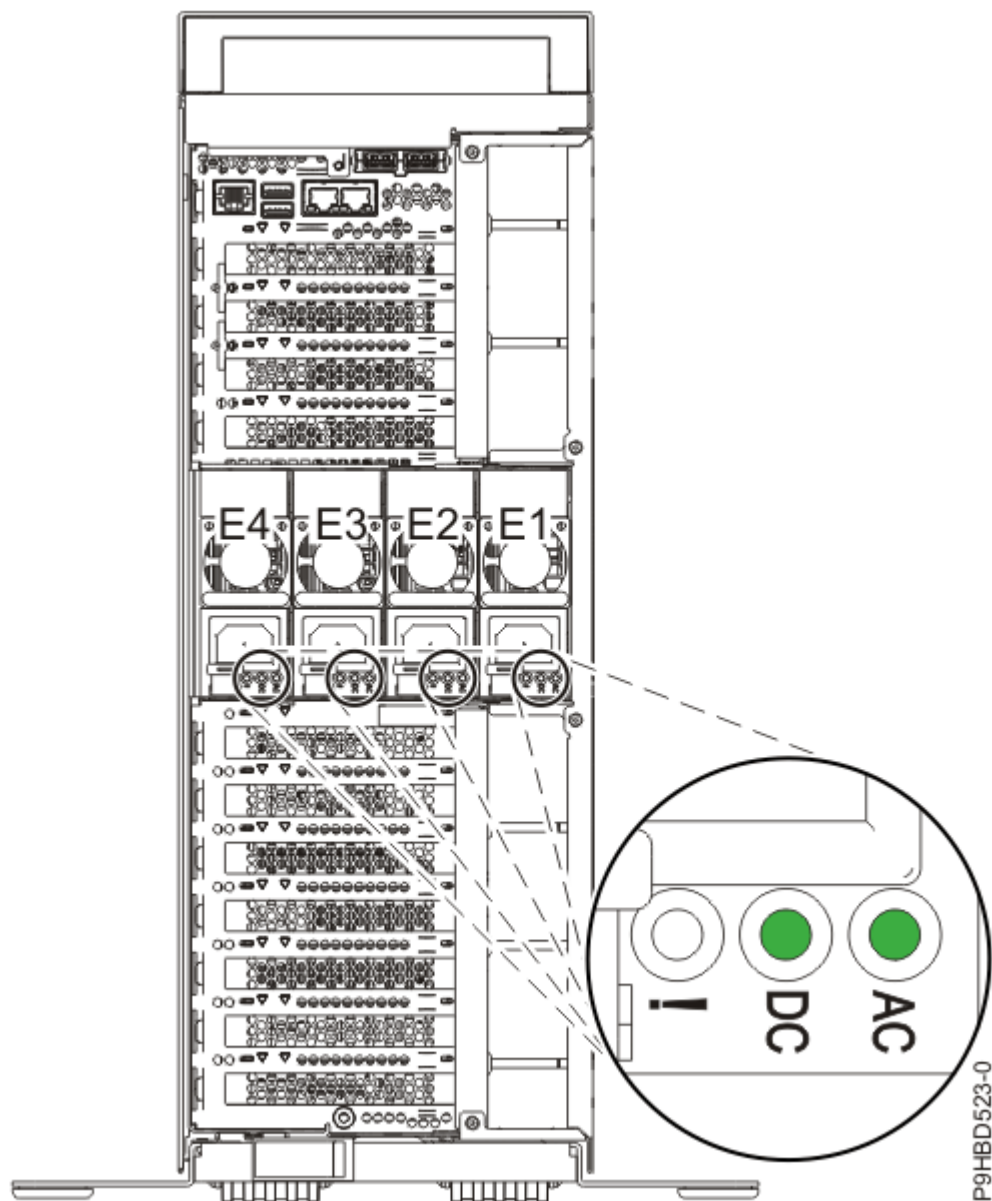
รูปที่ 11. LED สำหรับตัวจ่ายไฟที่ใช้ทำงานอยู่บนระบบสแตนด์อะโลน
