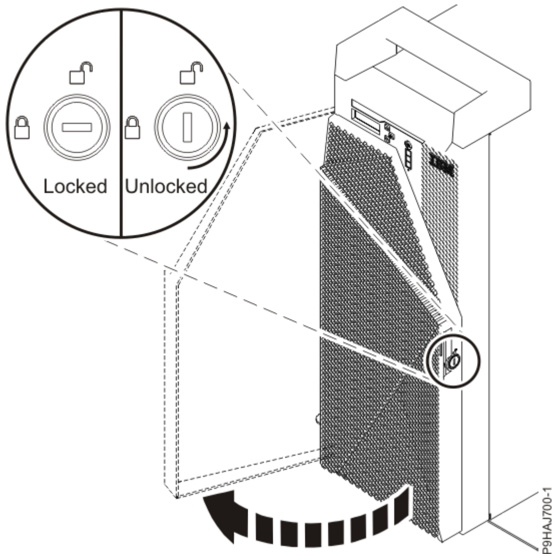
รูปที่ 6. การปลดล็อกประตูด้านหน้า
