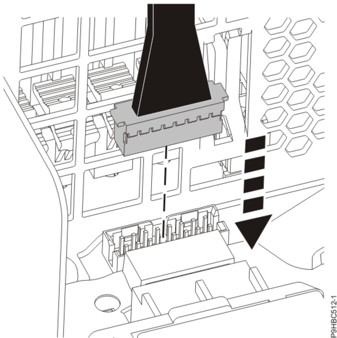
รูปที่ 82. การเชื่อมต่อสายเคเบิลแผงควบคุมกับแบ็คเพลนของระบบสำหรับระบบที่ประกอบเข้ากับชั้นวาง
