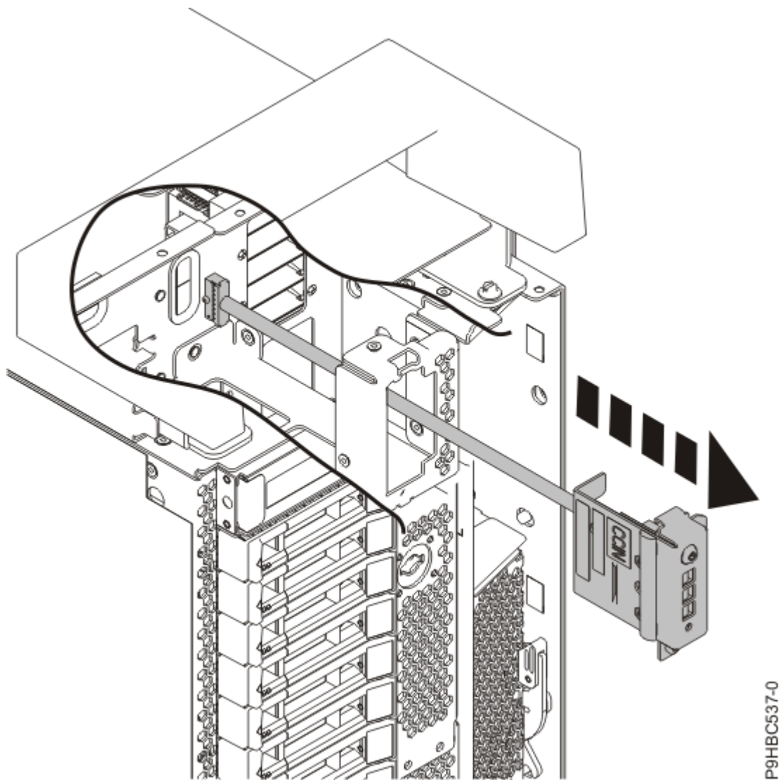
รูปที่ 69. การถอดแผงควบคุมและสายเคเบิลออกจากระบบแบบสแตนด์อะโลน
