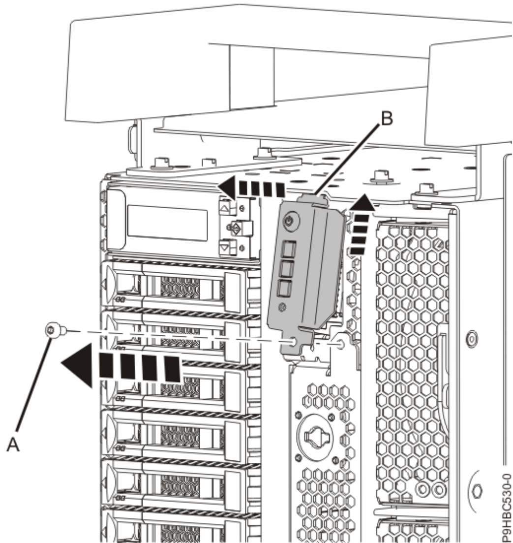
รูปที่ 66. การถอดสกรูแผงแผงควบคุมออกจากระบบแบบสแตนด์อะโลน b) ถอดแผงควบคุมออกจากระบบโดยหมุนแผงควบคุมไปทางด้านซ้ายตามที่แสดงใน รูปที่ 67 ในหน้า 72
