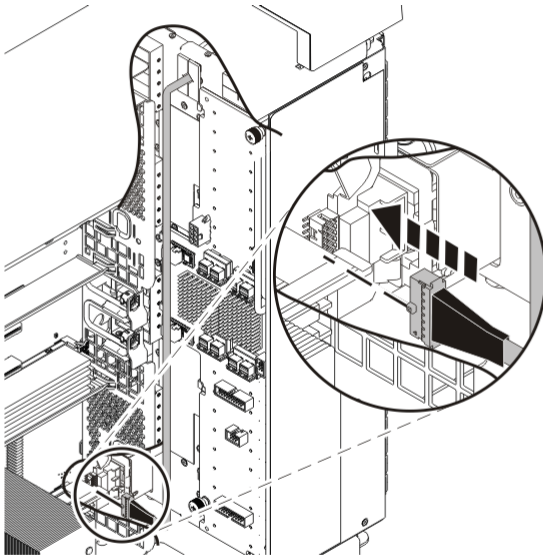
รูปที่ 83. การเชื่อมต่อสายเคเบิลแผงควบคุมกับแบ็คเพลนของระบบสำหรับระบบแบบสแตนด์อะโลน
