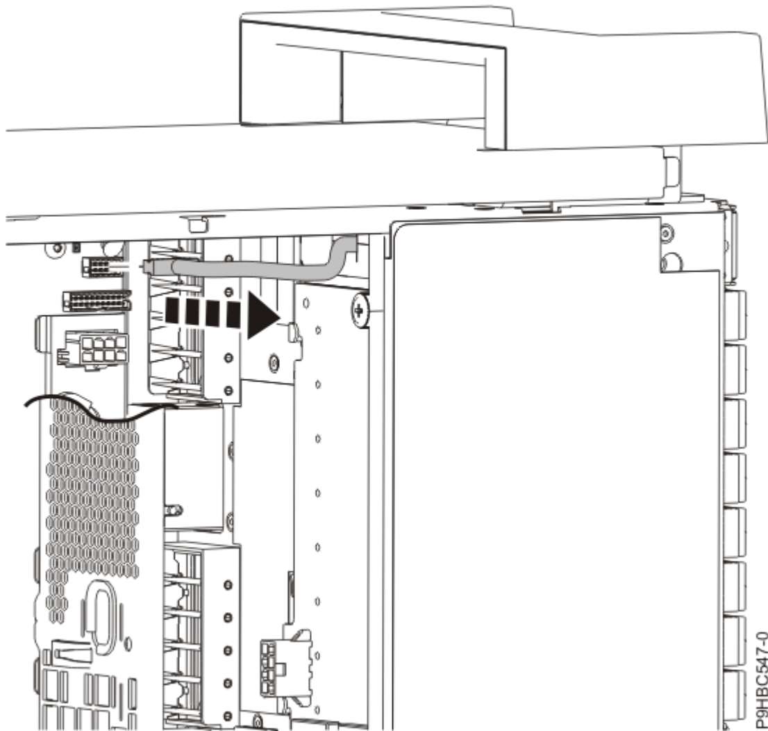
รูปที่ 110. การยกเลิกการเชื่อมต่อสายเคเบิลหน้าจอลงแผงควบคุมจากเบ็คเพลของระบบสำหรับระบบ แบบสแตนด์อะโลน
