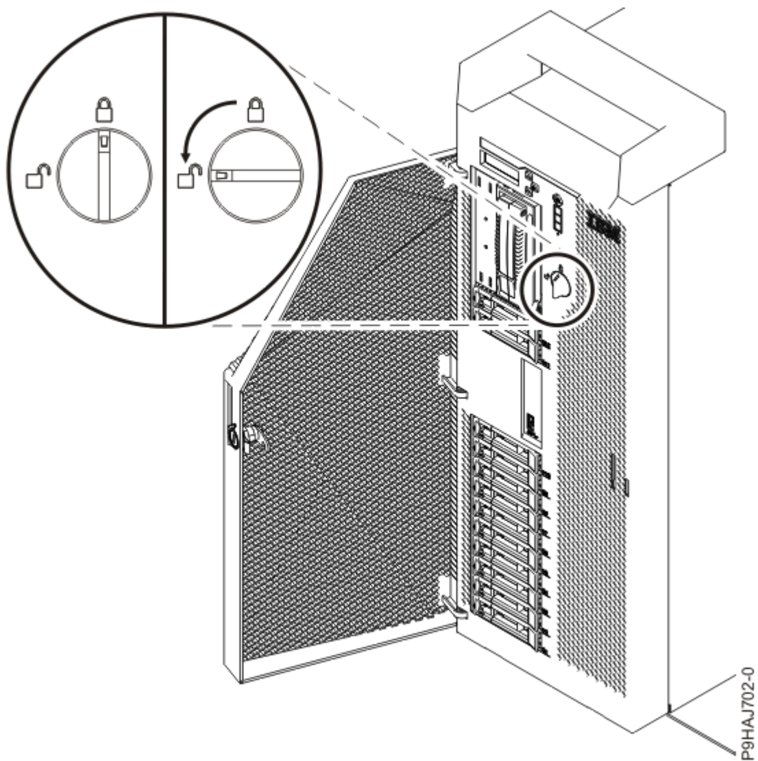
รูปที่ 54. การเปิดแลตซ์ฝาครอบด้านหน้า
