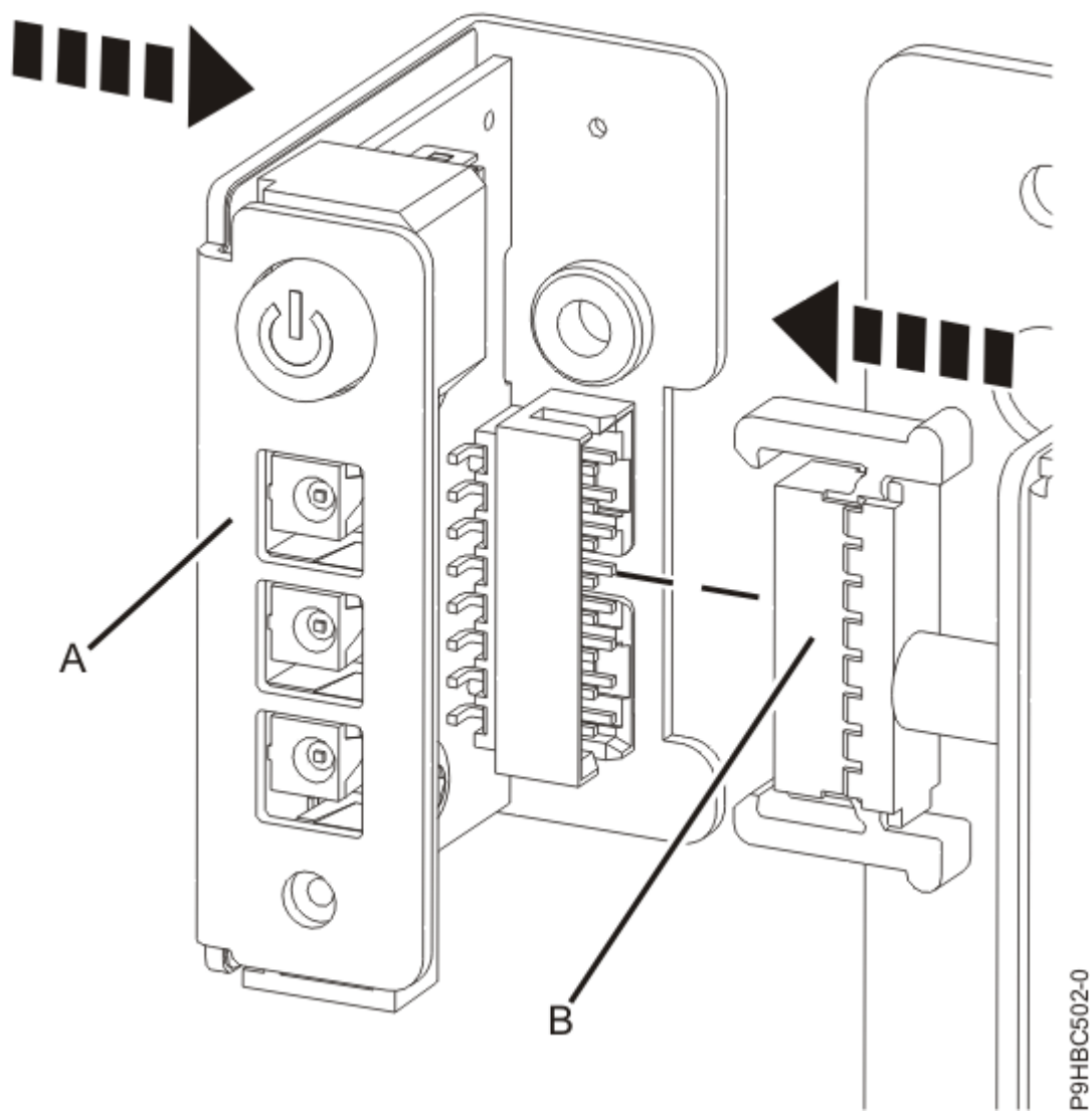
รูปที่ 72. การเชื่อมต่อแผงควบคุมและสายเคเบิลสำหรับระบบที่ประกอบเข้ากับชั้นวาง
