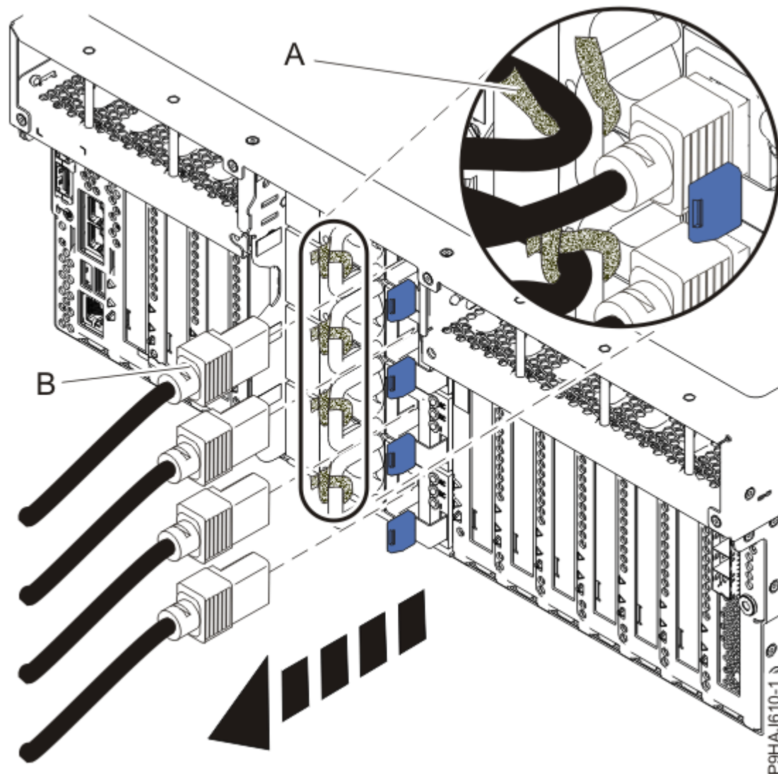
รูปที่ 96. การถอดสายไฟออกจากเซิร์ฟเวอร์ที่ประกอบเข้ากับชั้นวาง
