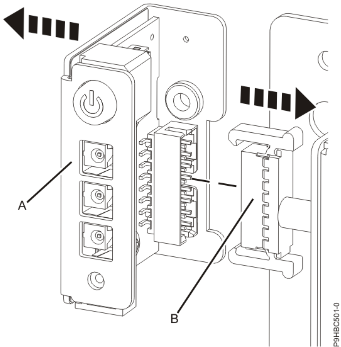
รูปที่ 20. การปิดการเชื่อมต่อแผงควบคุมจากสายเคเบิลสำหรับระบบที่ประกอบเข้ากับชั้นวาง
