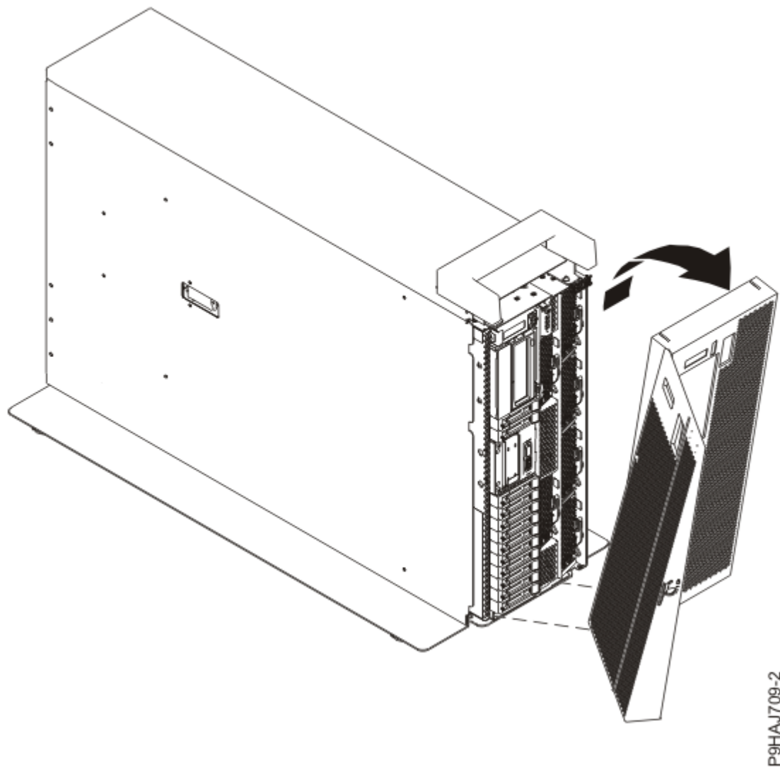
รูปที่ 8. การถอดฝาครอบด้านหน้า
