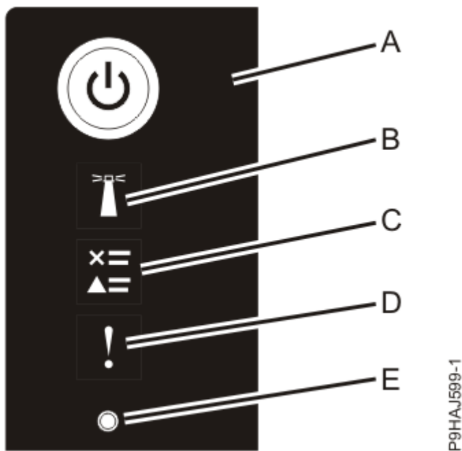
รูปที่ 36. คอนโทรลพาเนล LED
