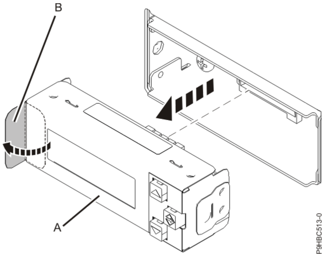
รูปที่ 111. การถอดหน้าจอสวิตช์ควบคุม
