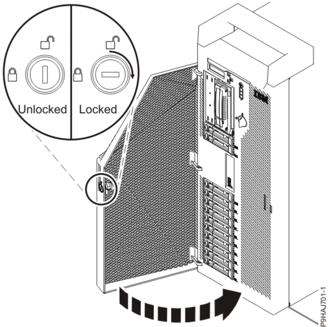
รูปที่ 137. การล็อกประตูด้านหน้า
