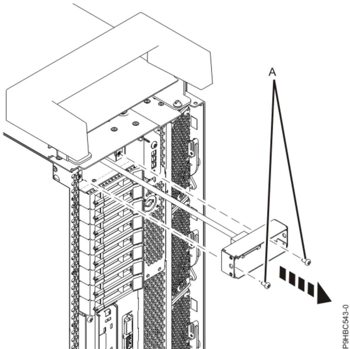
รูปที่ 113. การถอดด้ามจับหน้าจอลำดับความออกจากฉากรัดสำหรับระบบที่ประกอบเข้ากับชั้นวาง 8. สำหรับระบบที่ประกอบเข้ากับชั้นวาง ให้เปิดด้ามจับหน้าจอลำดับความตามที่แสดงใน รูปที่ 114 ในหน้า 120
