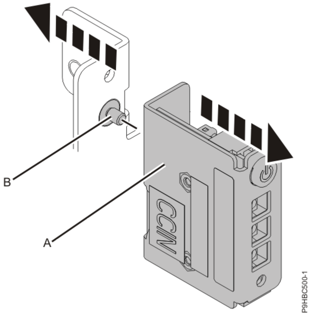
รูปที่ 17. การถอดแผงควบคุมจากฉากยึดสำหรับระบบที่ประกอบเข้ากับชั้นวาง
