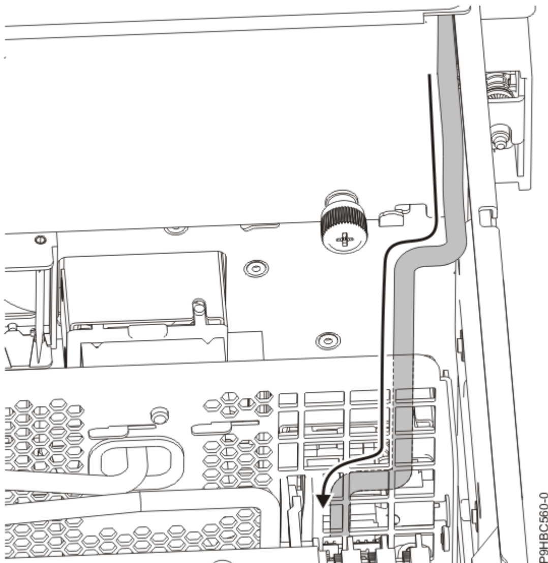
รูปที่ 75. เส้นทางสายเคเบิลแผงควบคุมสำหรับระบบที่ประกอบเข้ากับชั้นวาง
