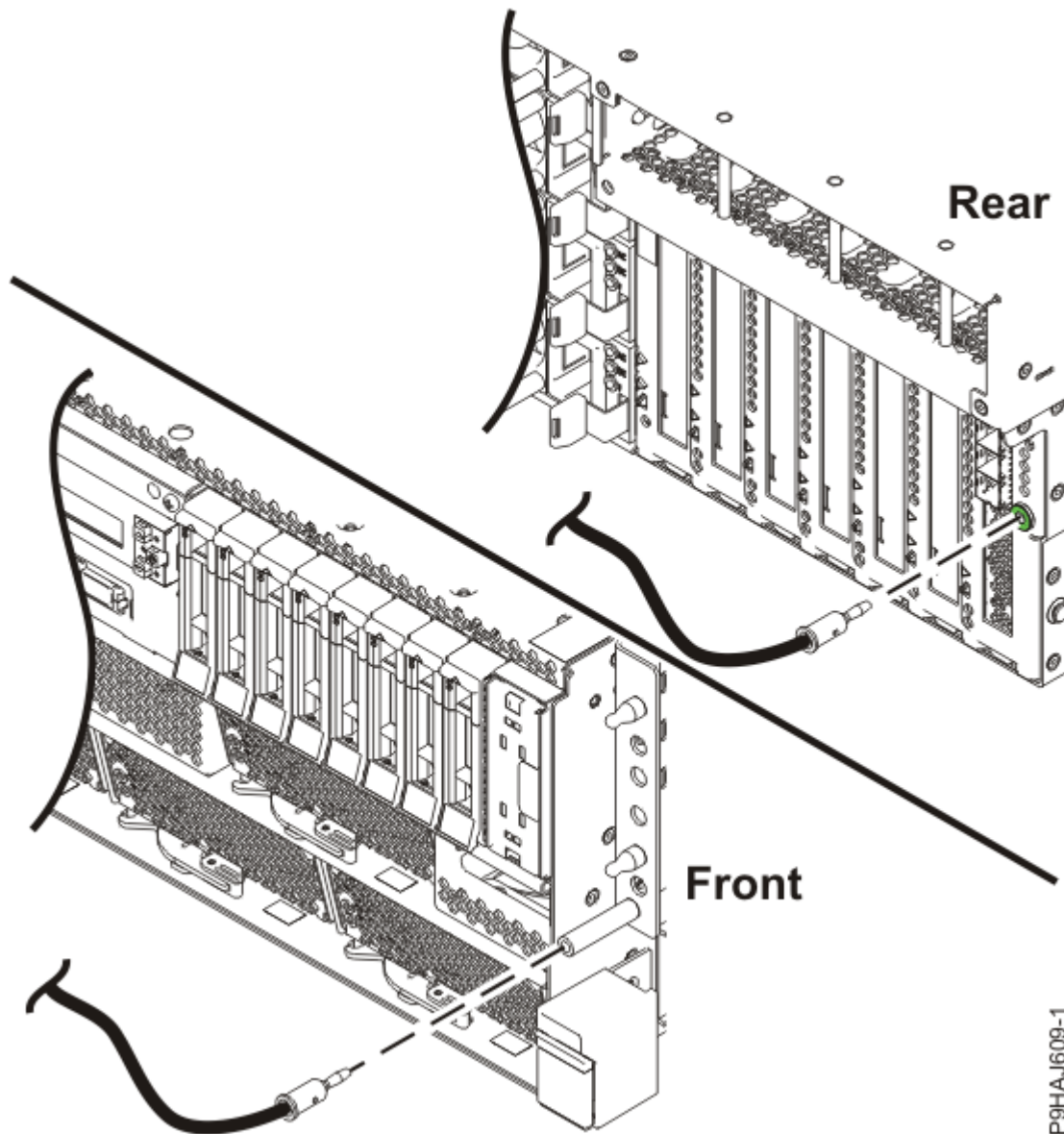
รูปที่ 10. ตำแหน่งของปลั๊ก ESD
