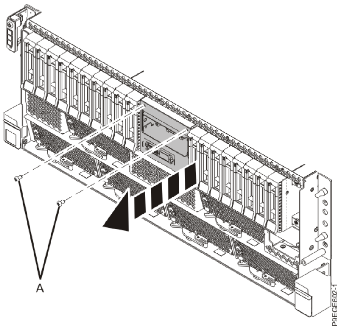
รูปที่ 112. การถอดด้ามจับหน้าจอแผงควบคุมออกจากฉากยึดสำหรับระบบที่ประกอบเข้ากับชั้นวาง
