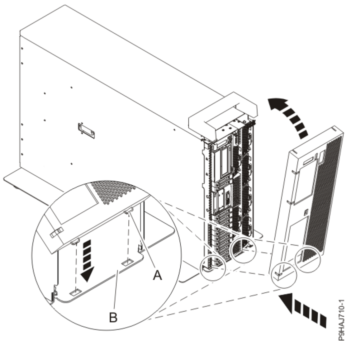
รูปที่ 47. การติดตั้งฝาครอบและประตูด้านหน้า
