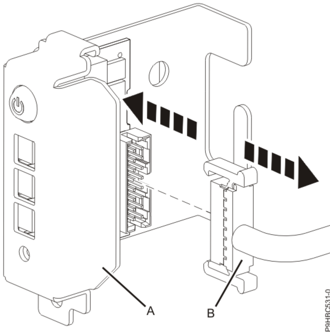
รูปที่ 21. การปิดการเชื่อมต่อแผงควบคุมจากสายเคเบิลสำหรับระบบแบบสแตนด์เอโลน
