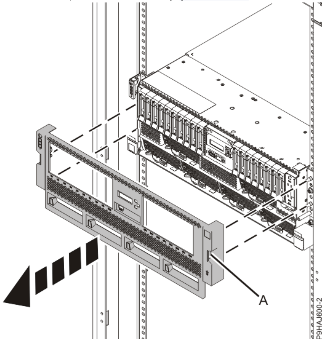
รูปที่ 98. การถอดฝาครอบด้านหน้า
