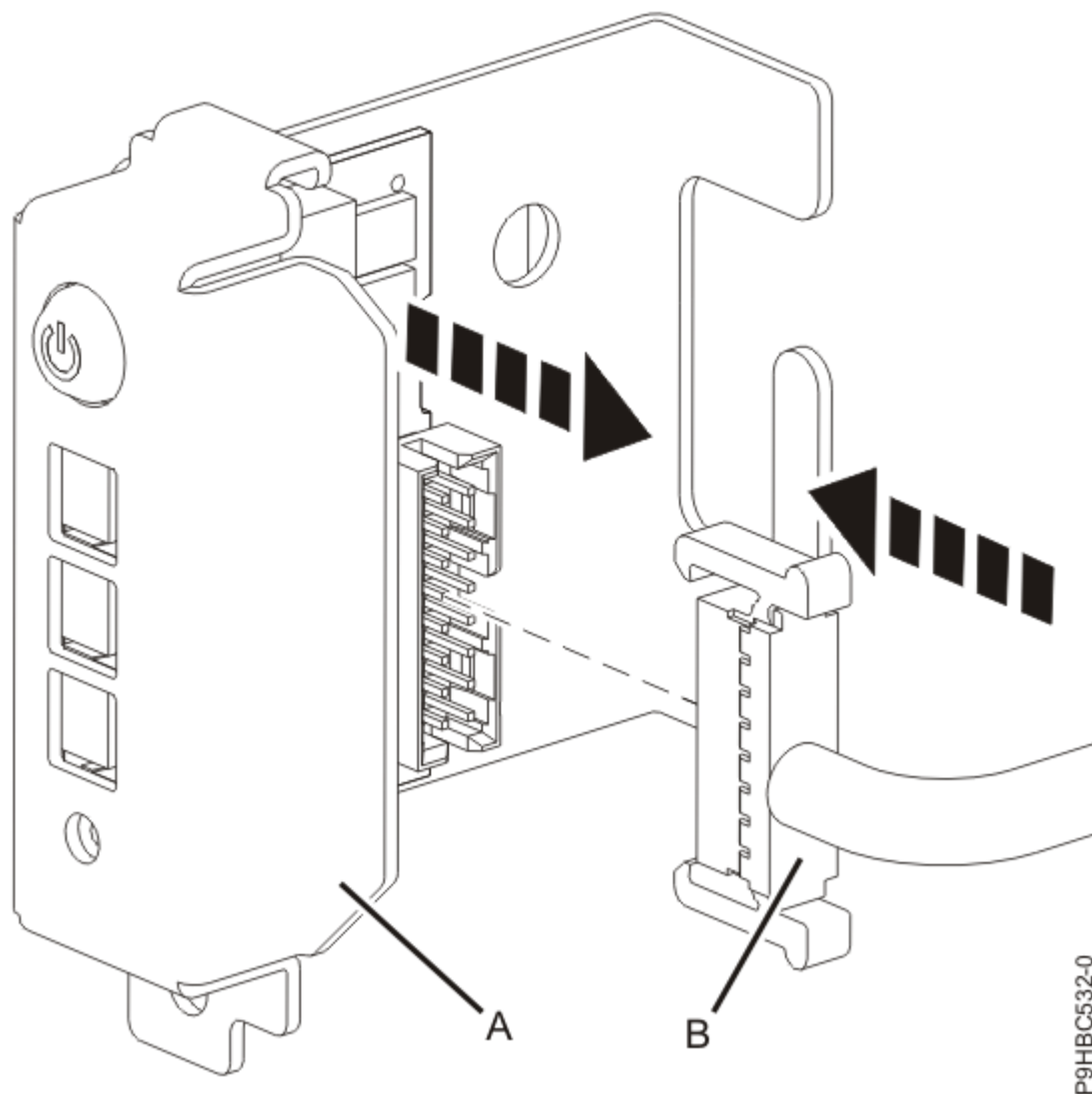
รูปที่ 73. การเชื่อมต่อแผงควบคุมและสายเคเบิลสำหรับระบบแบบสแตนด์เอโลน
