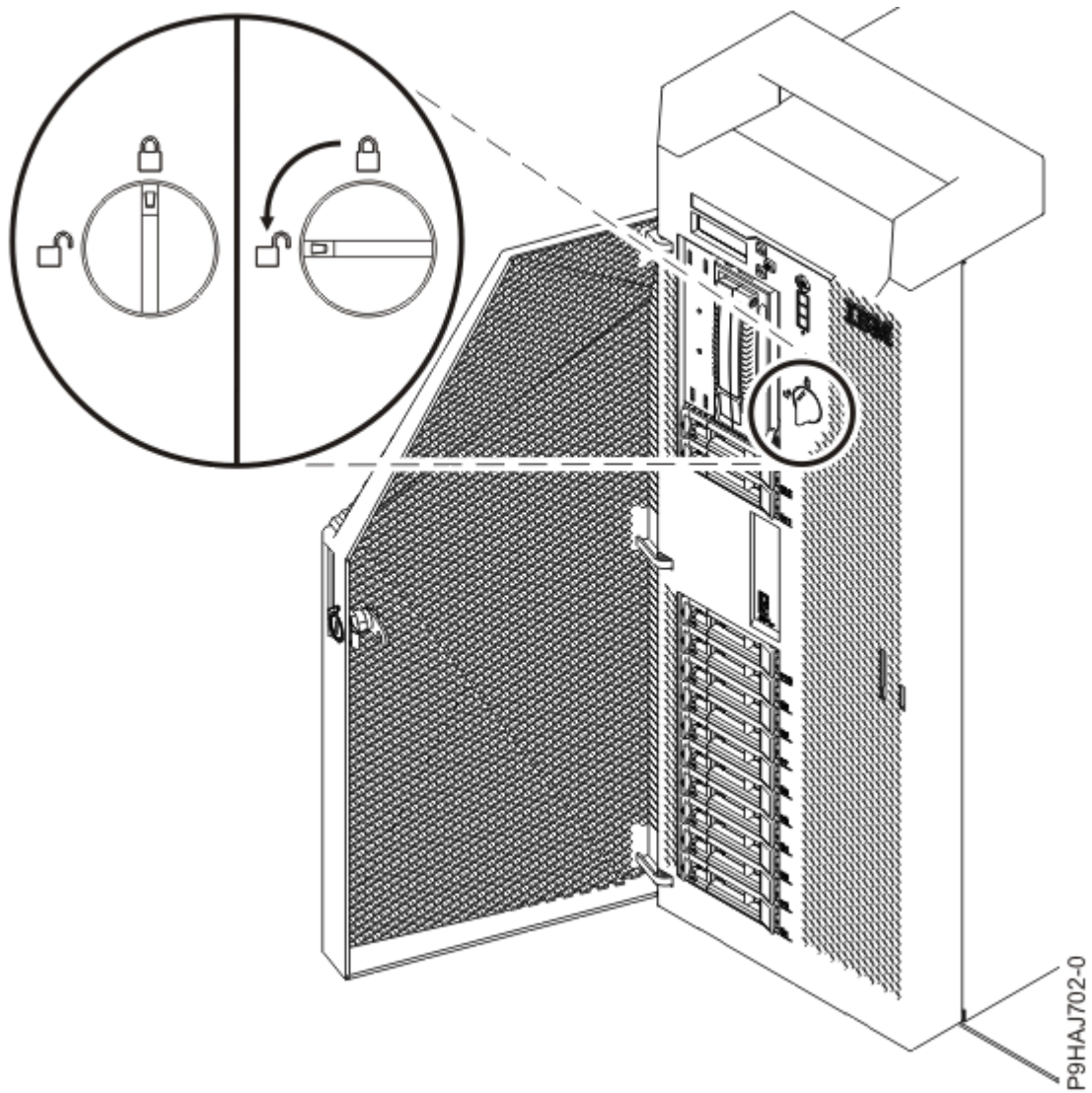
รูปที่ 7. การเปิดแลตซ์ฝาครอบด้านหน้า
