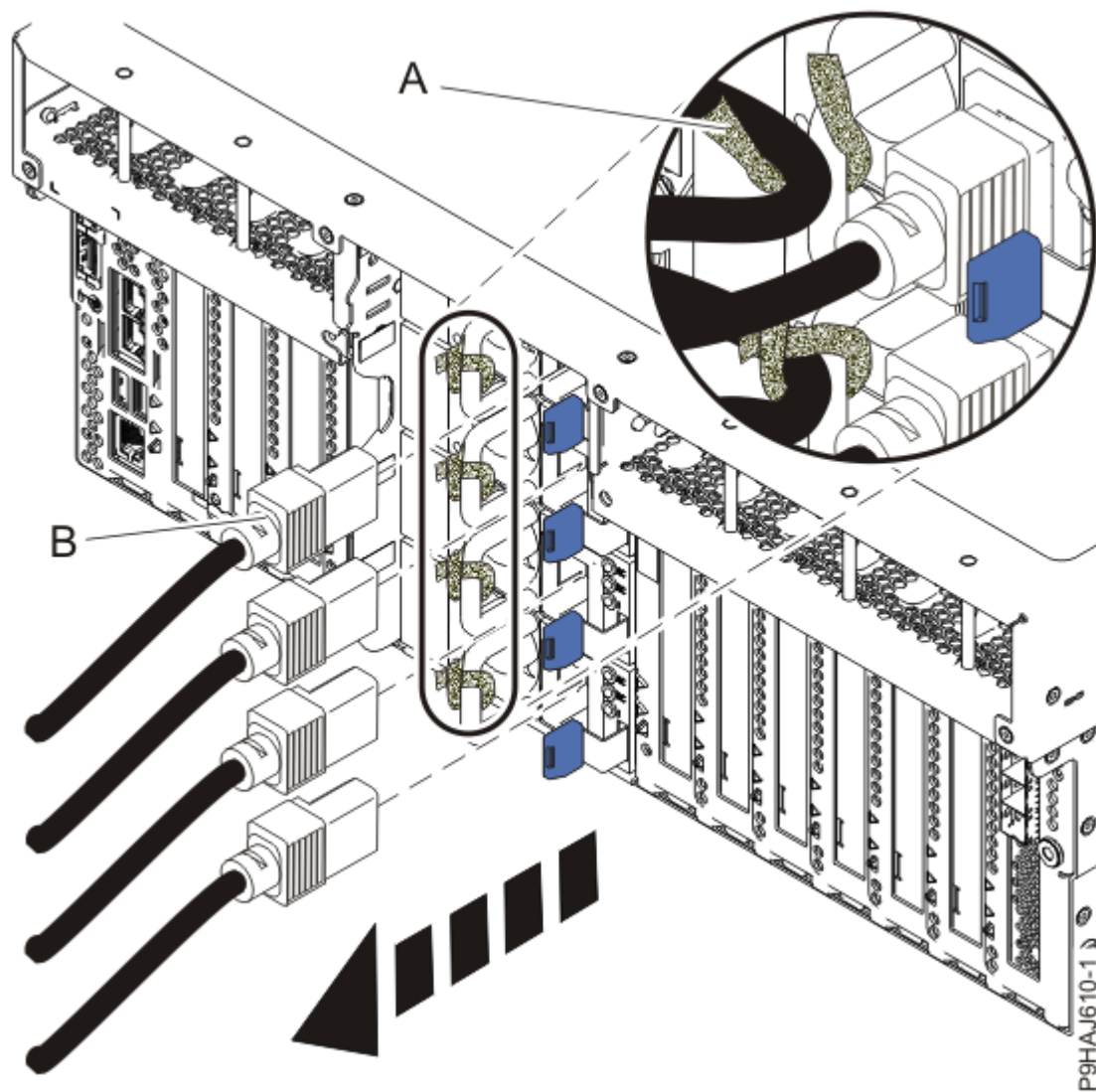
รูปที่ 3. การถอดสายไฟออกจากเซิร์ฟเวอร์ที่ประกอบเข้ากับชั้นวาง
