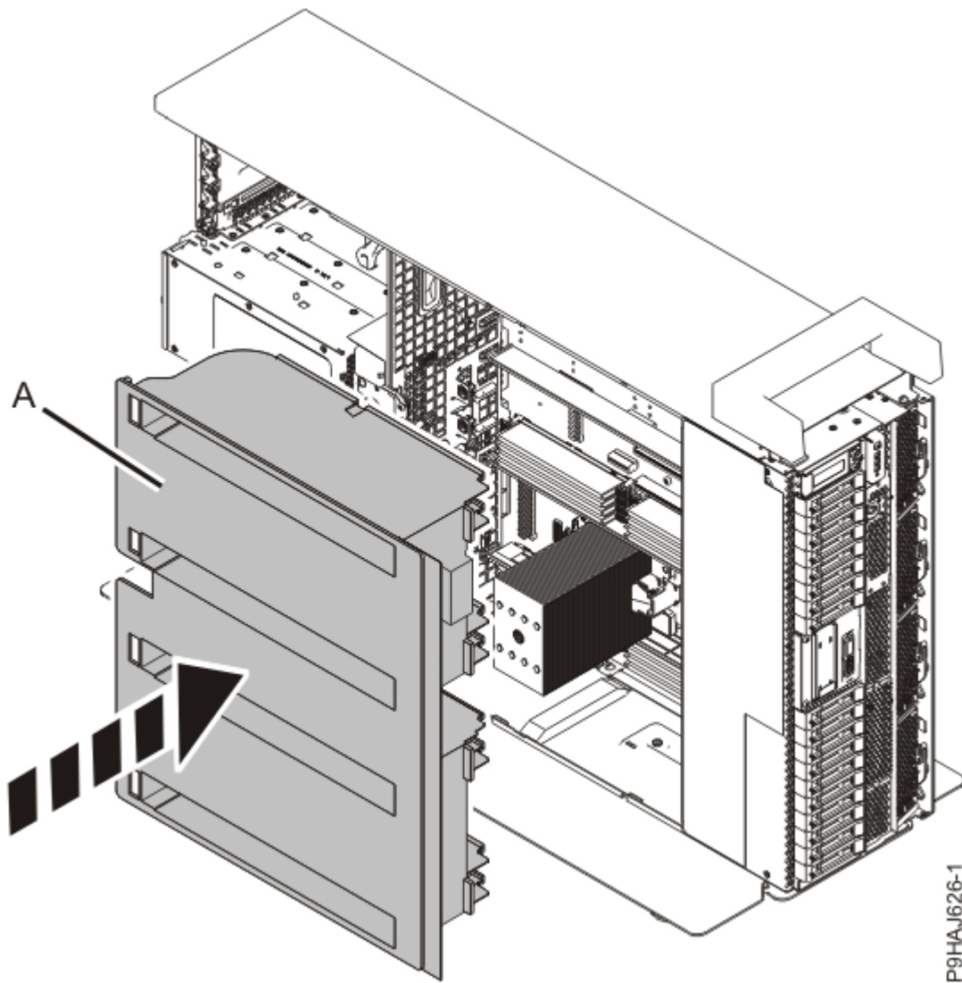
รูปที่ 85. การเปลี่ยนตัวไหลเวียนอากาศในระบบแบบสแตนด์อะโลน
