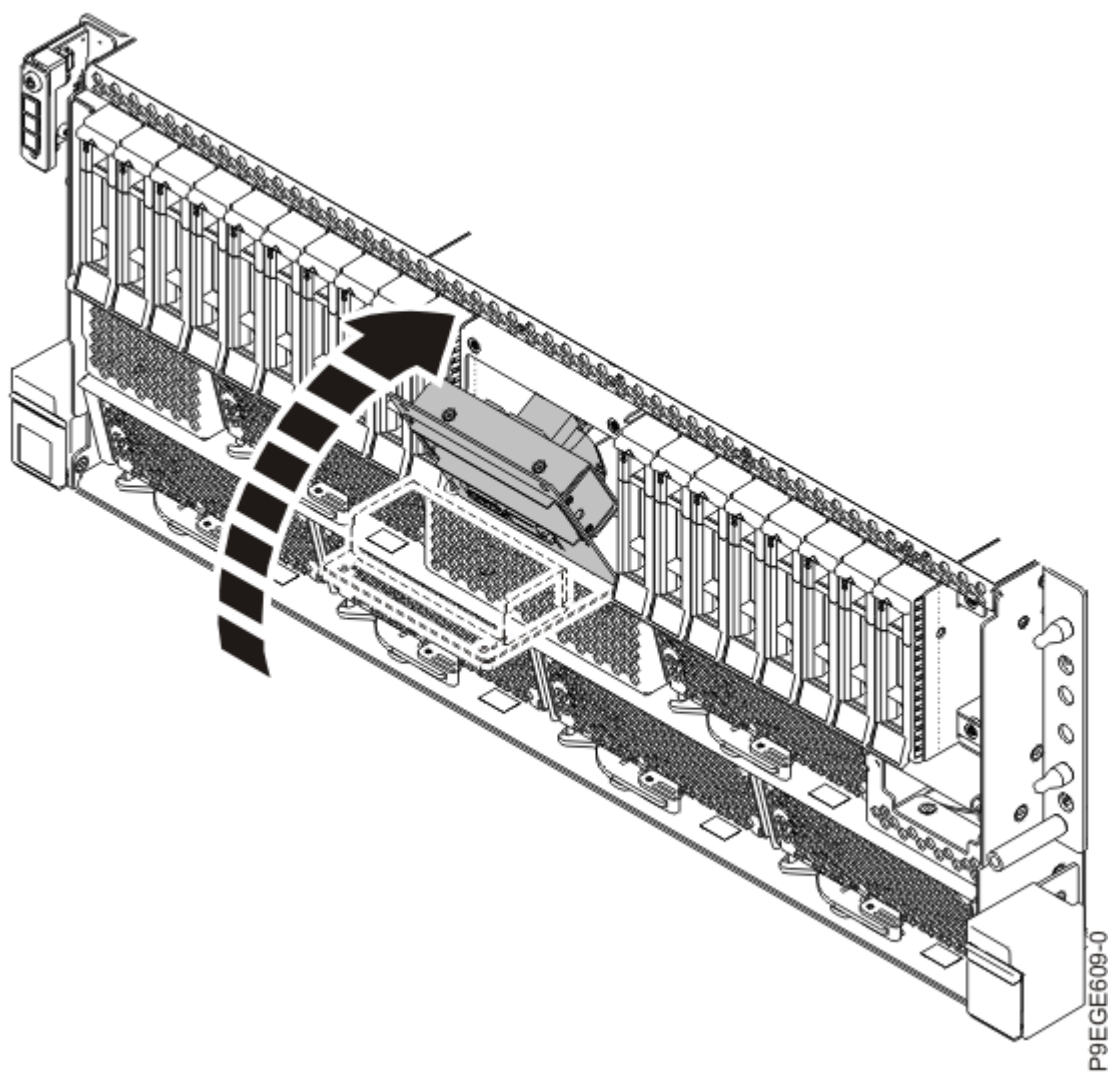
รูปที่ 120. การบิดด้ามจับหน้าจอแผงควบคุมสำหรับระบบที่ประกอบเข้ากับชั้นวาง
