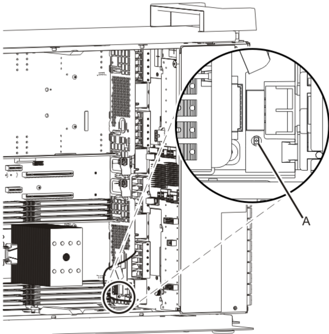
รูปที่ 16. ตำแหน่งของ LED แผงควบคุมในระบบแบบสแตนด์เอโลน
