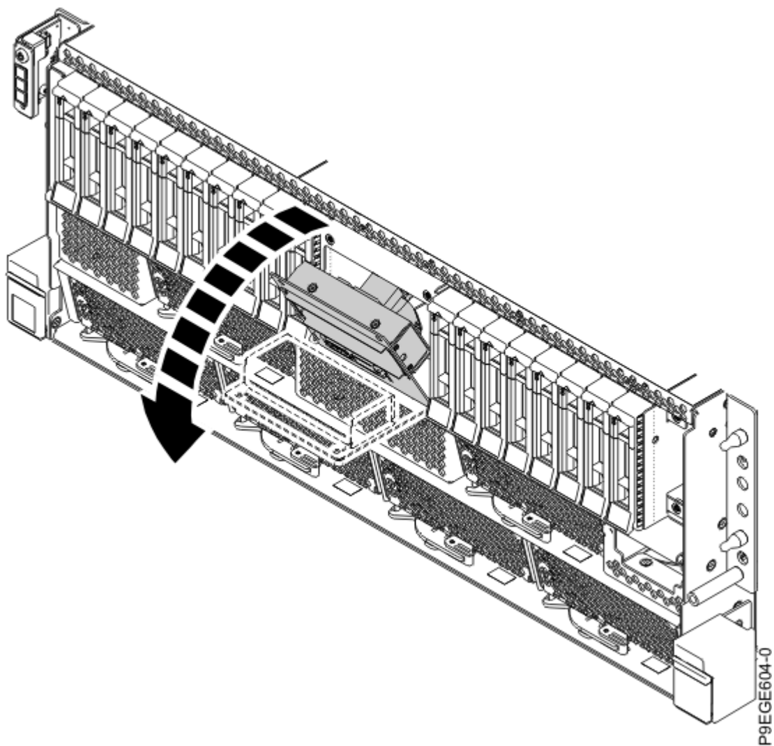
รูปที่ 114. การเปิดด้ามจับหน้าจอแผงควบคุมสำหรับระบบที่ประกอบเข้ากับชั้นวาง
