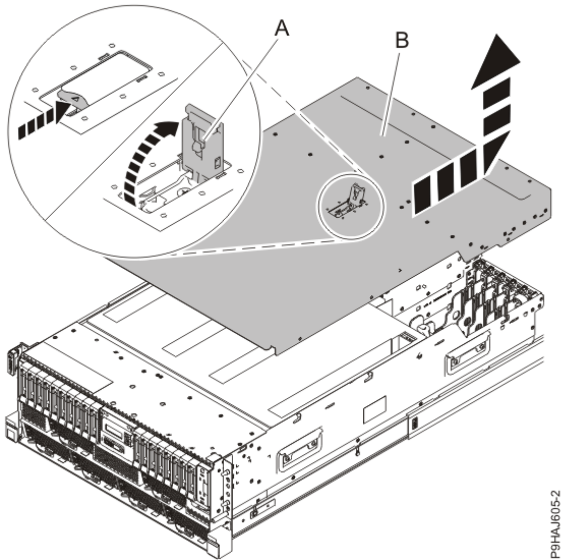
รูปที่ 11. การถอดฝาครอบการเข้าถึงเซิร์ฟเวอร์ออกจากระบบที่ติดตั้งในชั้นวาง
