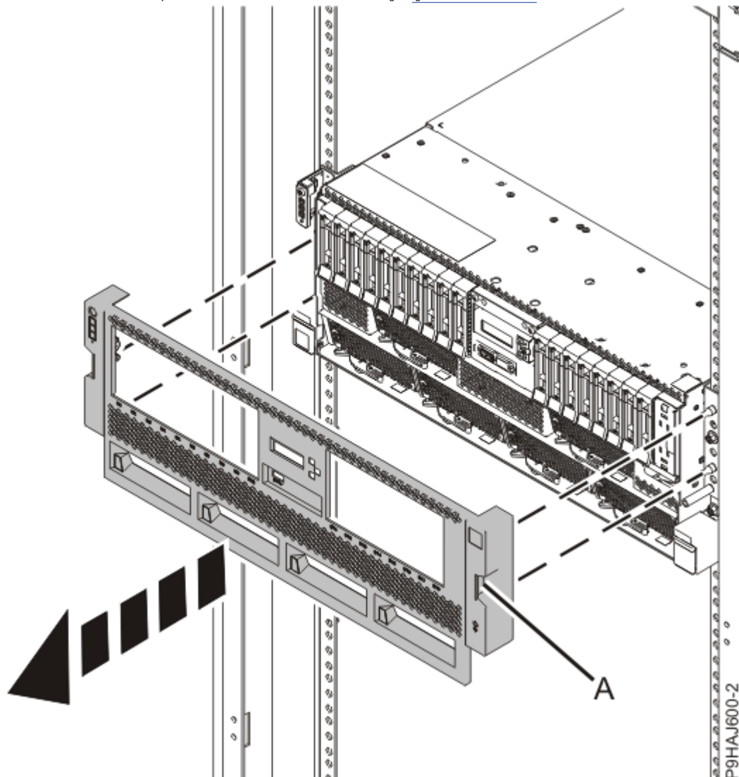
รูปที่ 5. การถอดฝาครอบด้านหน้า
