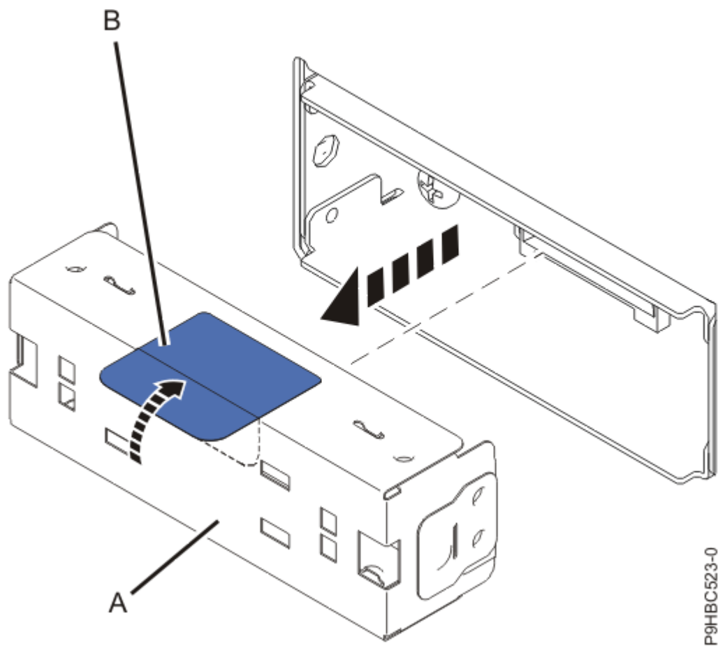
รูปที่ 44. การถอดฟิลเลอร์หน้าจอ
