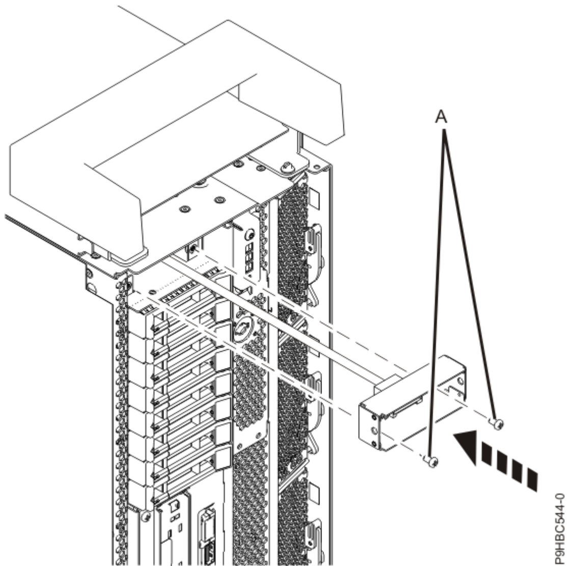
รูปที่ 122. การใส่สายเคเบิลหน้าจอแผงควบคุมสำหรับระบบแบบสแตนด์อะโลน
