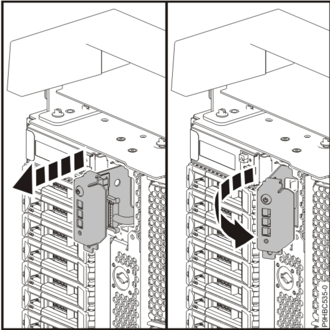
รูปที่ 19. การถอดแผงควบคุมออกจากระบบแบบสแตนด์เอโลน
