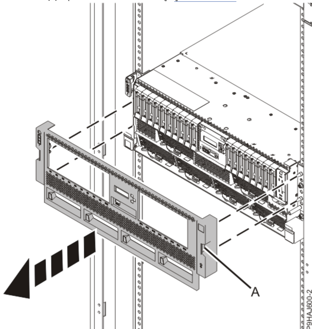
รูปที่ 52. การถอดฝาครอบด้านหน้า
