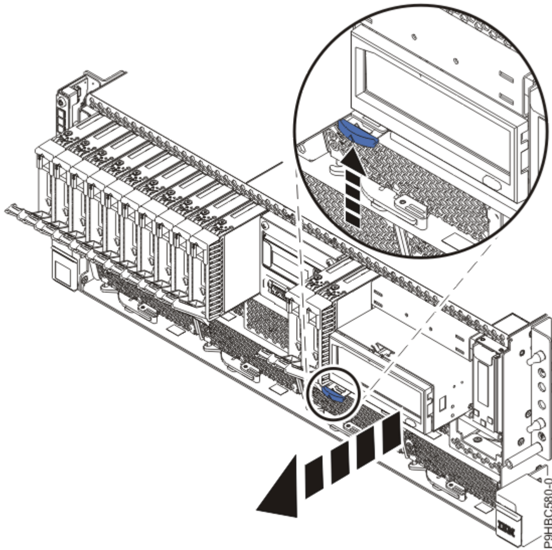
รูปที่ 108. การถอดแทนวาง RDX ออกบางส่วน
