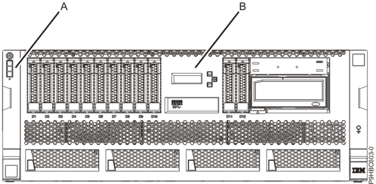
รูปที่ 1. แผงควบคุมในระบบที่ประกอบเข้ากับชั้นวาง
