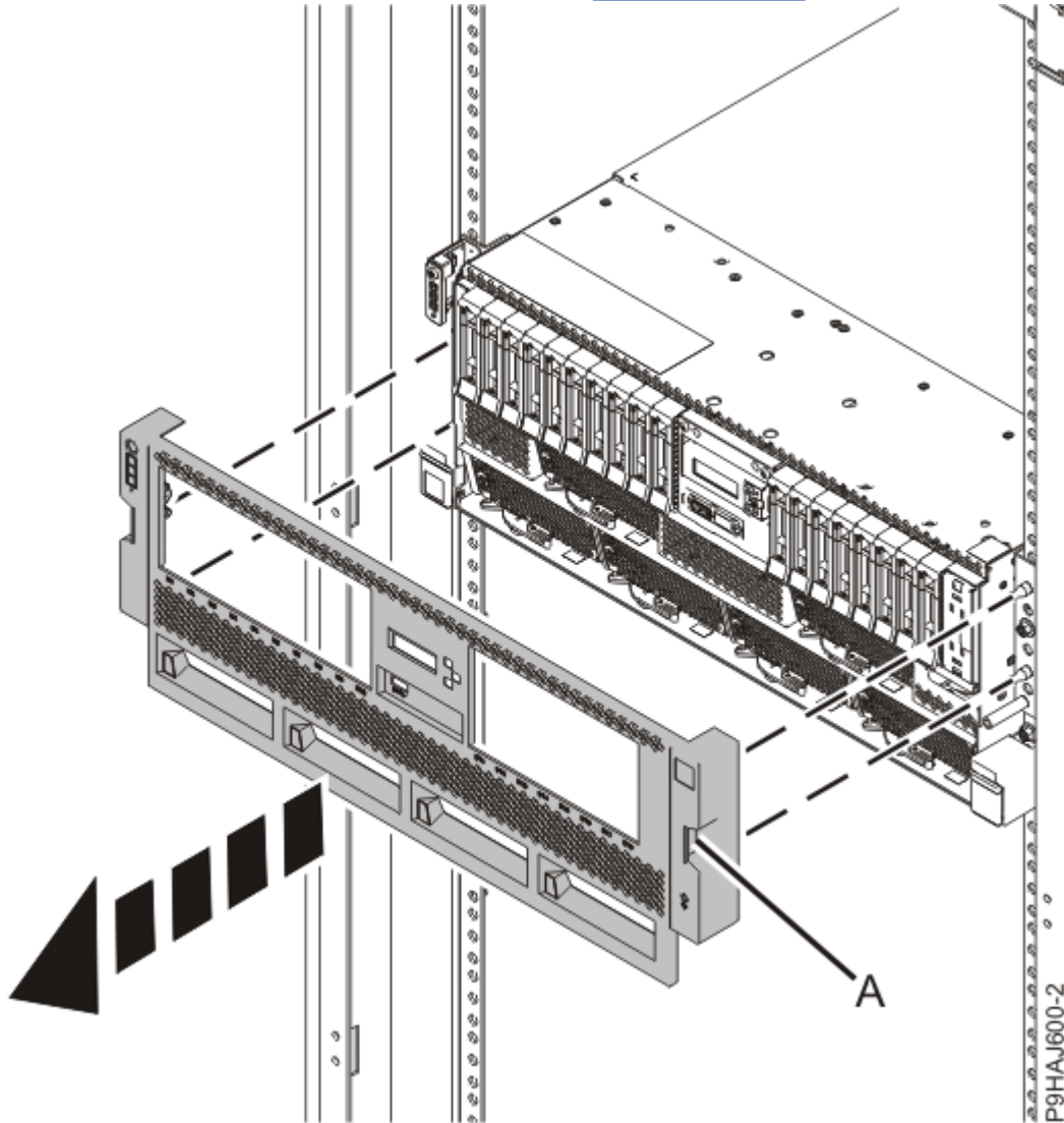
รูปที่ 37. การถอดฝาครอบด้านหน้า
