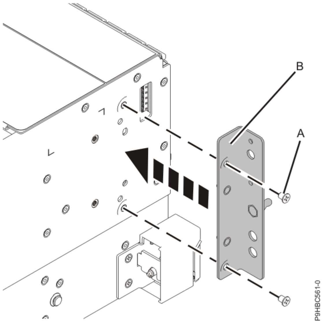
รูปที่ 78. การเปลี่ยนโครงแผงควบคุม
