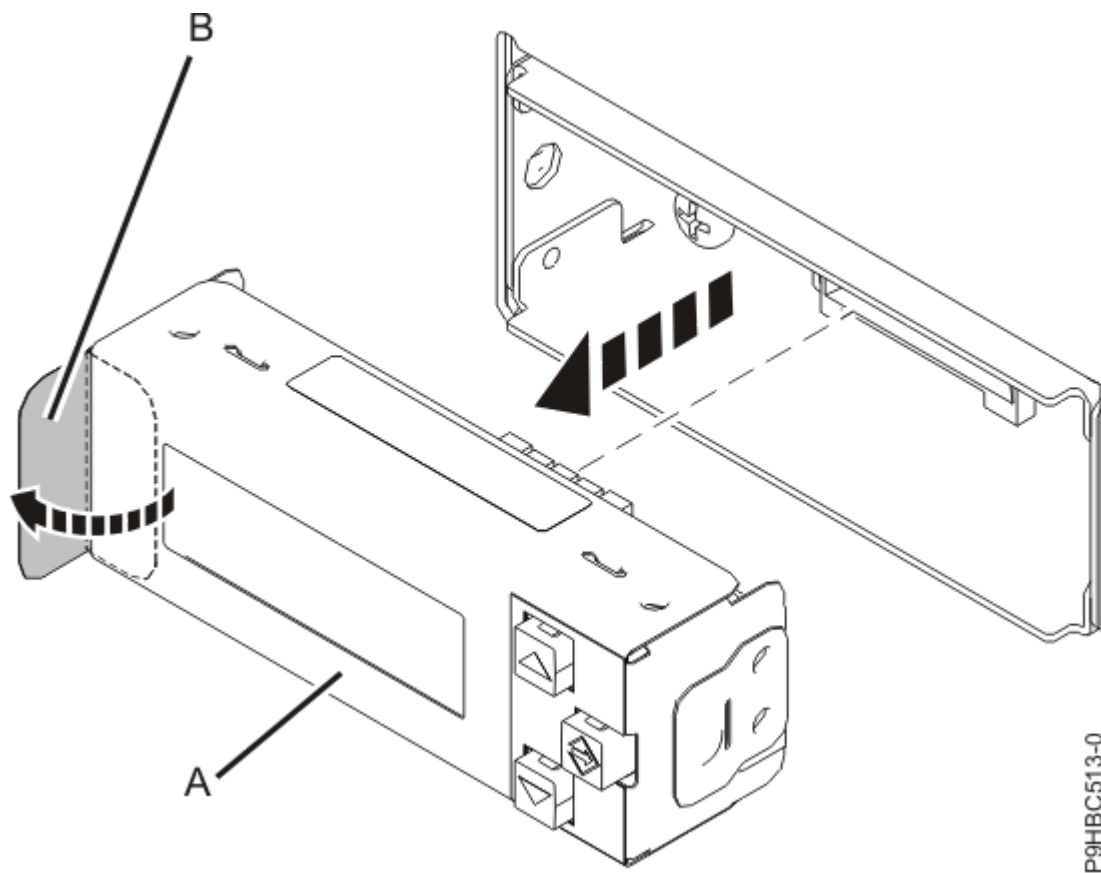
รูปที่ 42. การถอดหน้าจ่อแผงควบคุม
