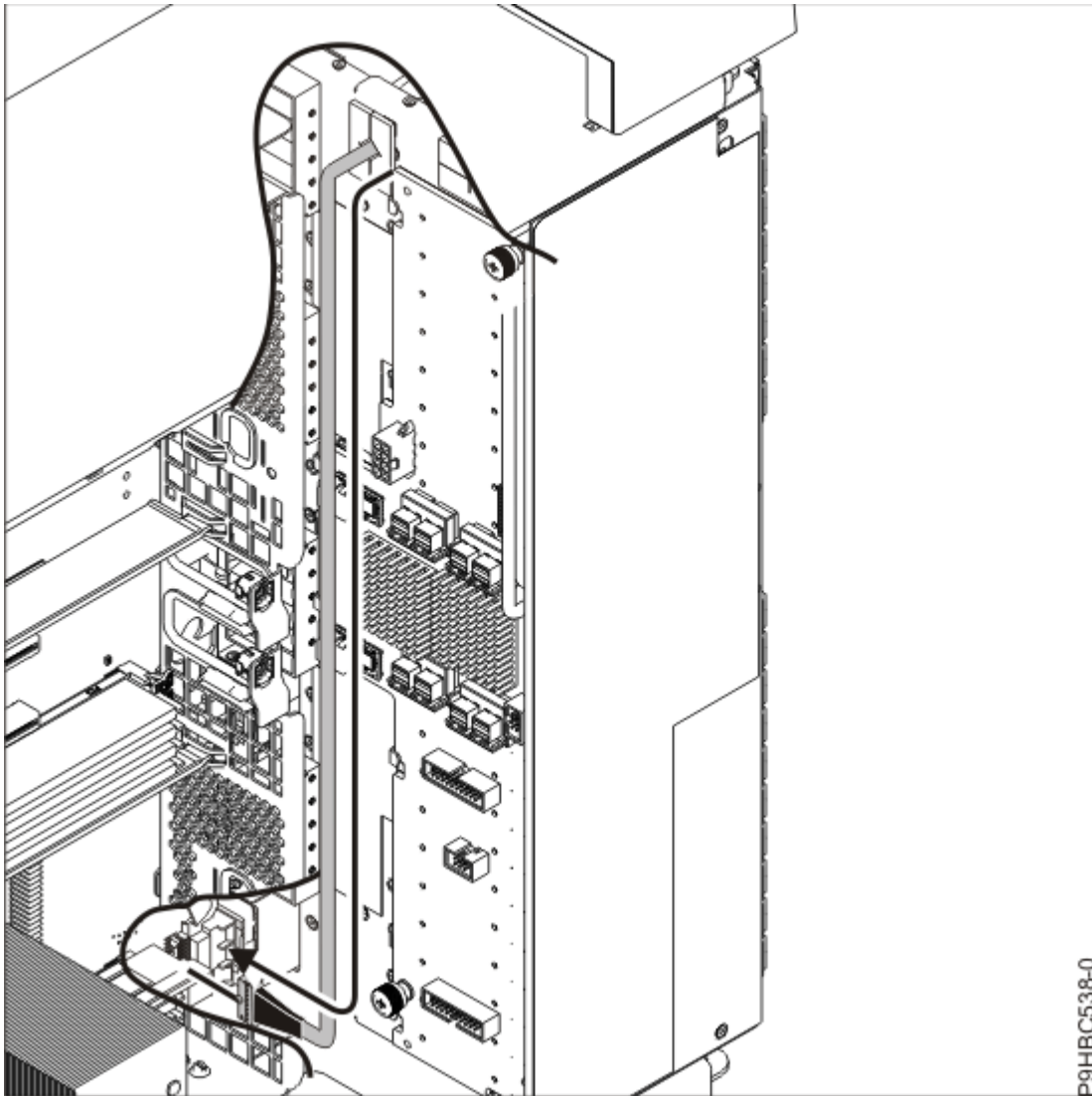
รูปที่ 77. เส้นทางสายเคเบิลแผงควบคุมสำหรับระบบแบบสแตนด์อะโลน
