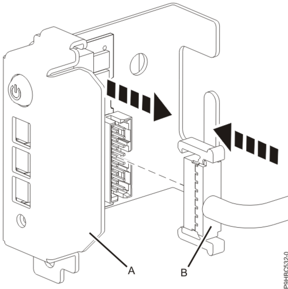
รูปที่ 23. การเชื่อมต่อแผงควบคุมและสายเคเบิลสำหรับระบบแบบสแตนด์เอโลน
