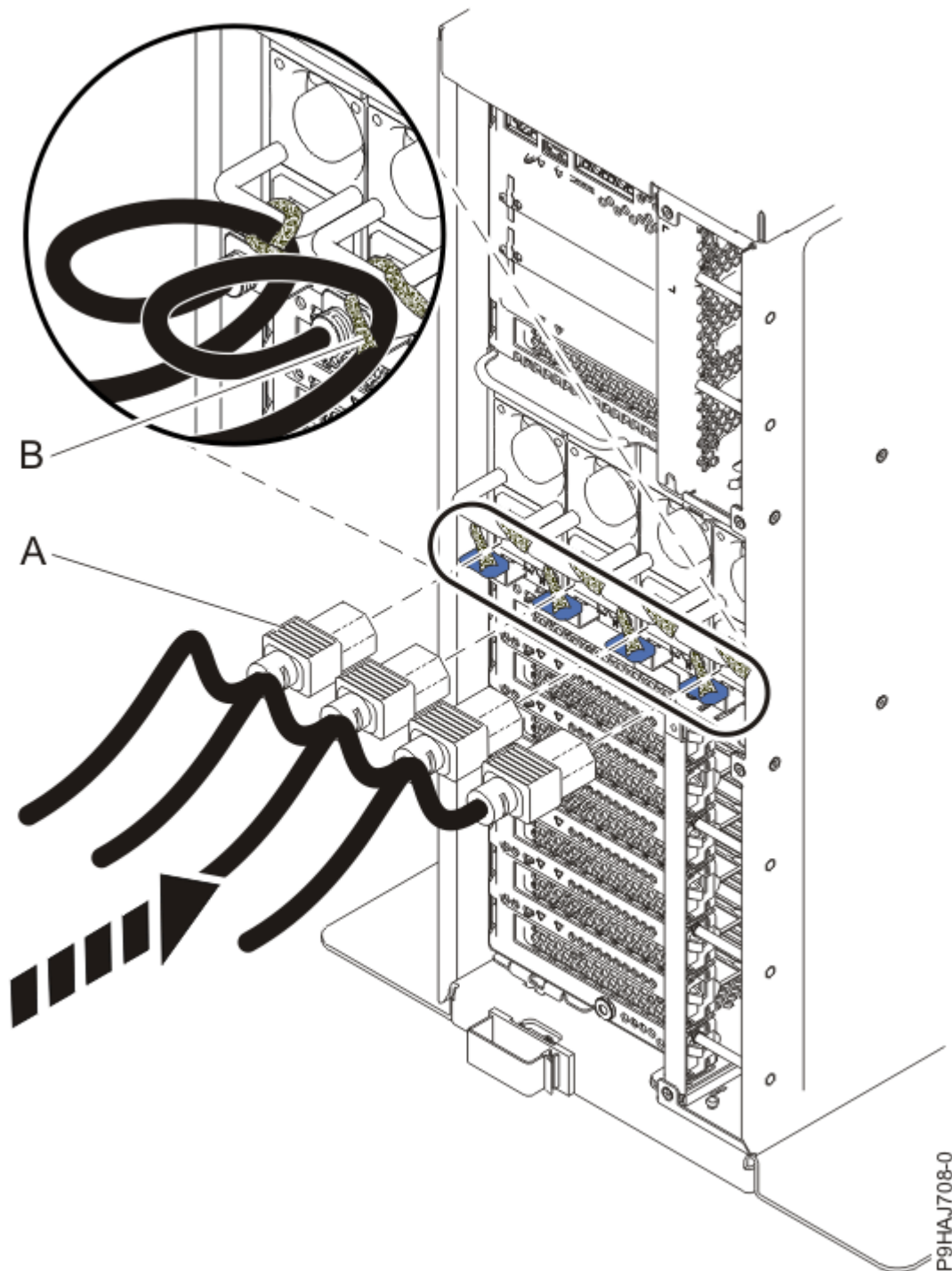
รูปที่ 139. การเชื่อมต่อสายไฟเข้ากับระบบแบบสแตนด์เอโลน
