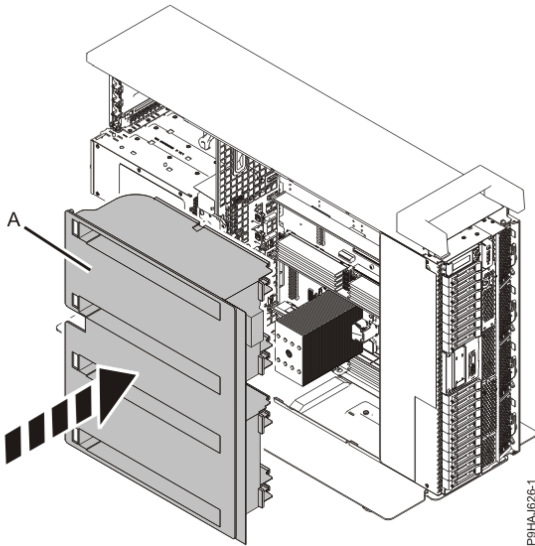
รูปที่ 130. การเปลี่ยนตัวไหลเวียนอากาศในระบบแบบสแตนด์อะโลน
