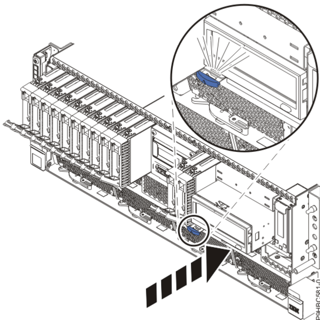
รูปที่ 127. การเปลี่ยนตำแหน่ง RDX
