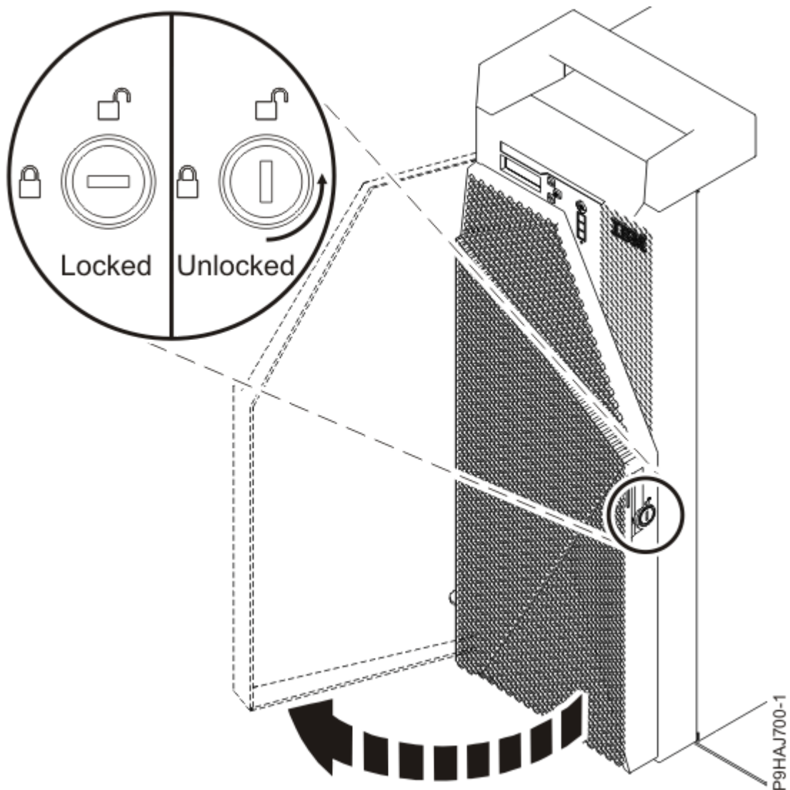
รูปที่ 53. การปลดล็อกประตูด้านหน้า
