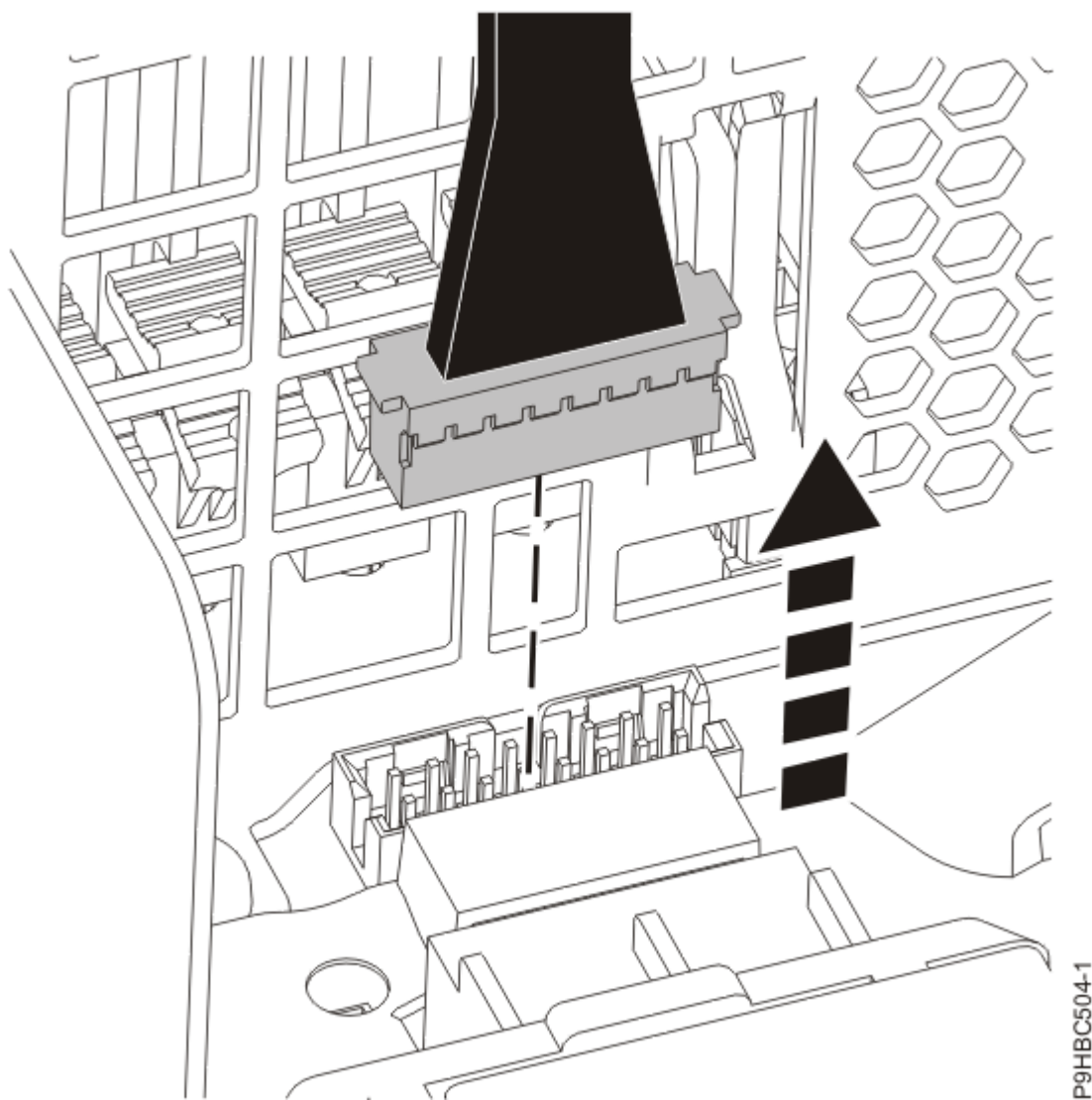
รูปที่ 62. การยกเลิกการเชื่อมต่อสายเคเบิลแผงควบคุมจากเบ็คเพลนของระบบสำหรับระบบที่ประกอบเข้ากับ ชั้นวาง
