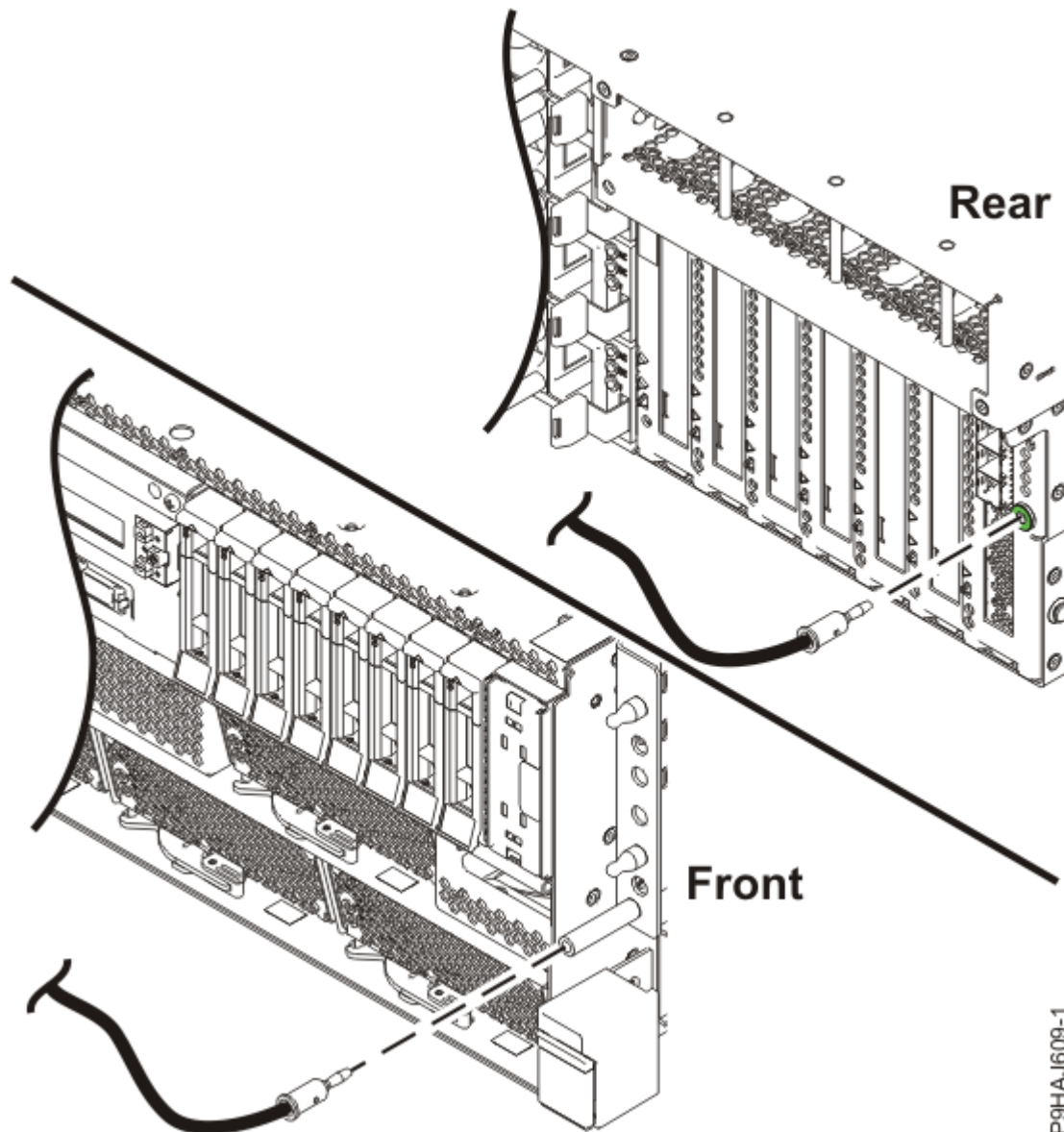
รูปที่ 41. ตำแหน่งของปลั๊ก ESD
