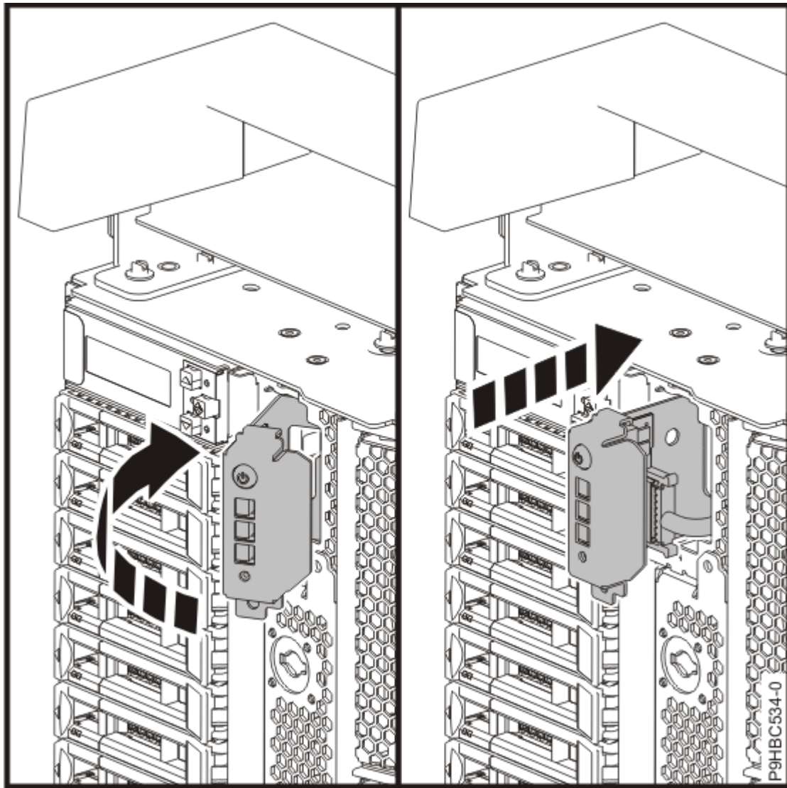
รูปที่ 25. การเปลี่ยนแผงควบคุมในระบบแบบสแตนด์อะโลน
