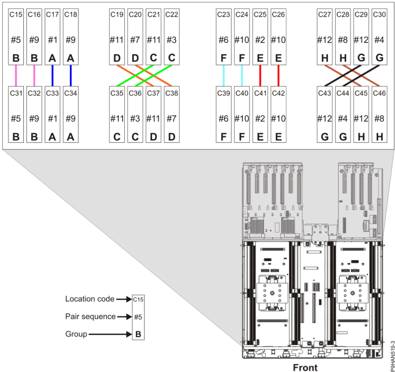
รูปที่ 29. ลำดับการเชื่อมต่อ สองตัวประมวลผลระบบ
