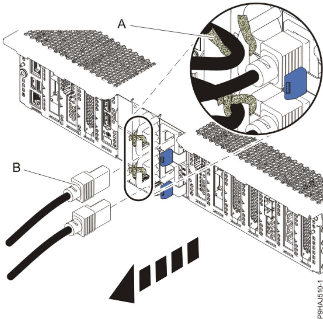
รูปที่ 4. การถอดสายไฟ
