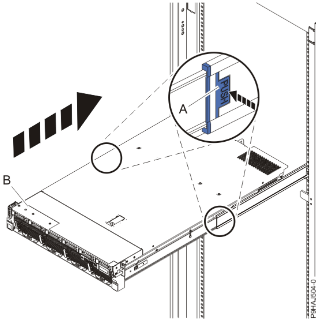
รูปที่ 25. การจัดตำแหน่งระบบในตำแหน่งการทำงาน
