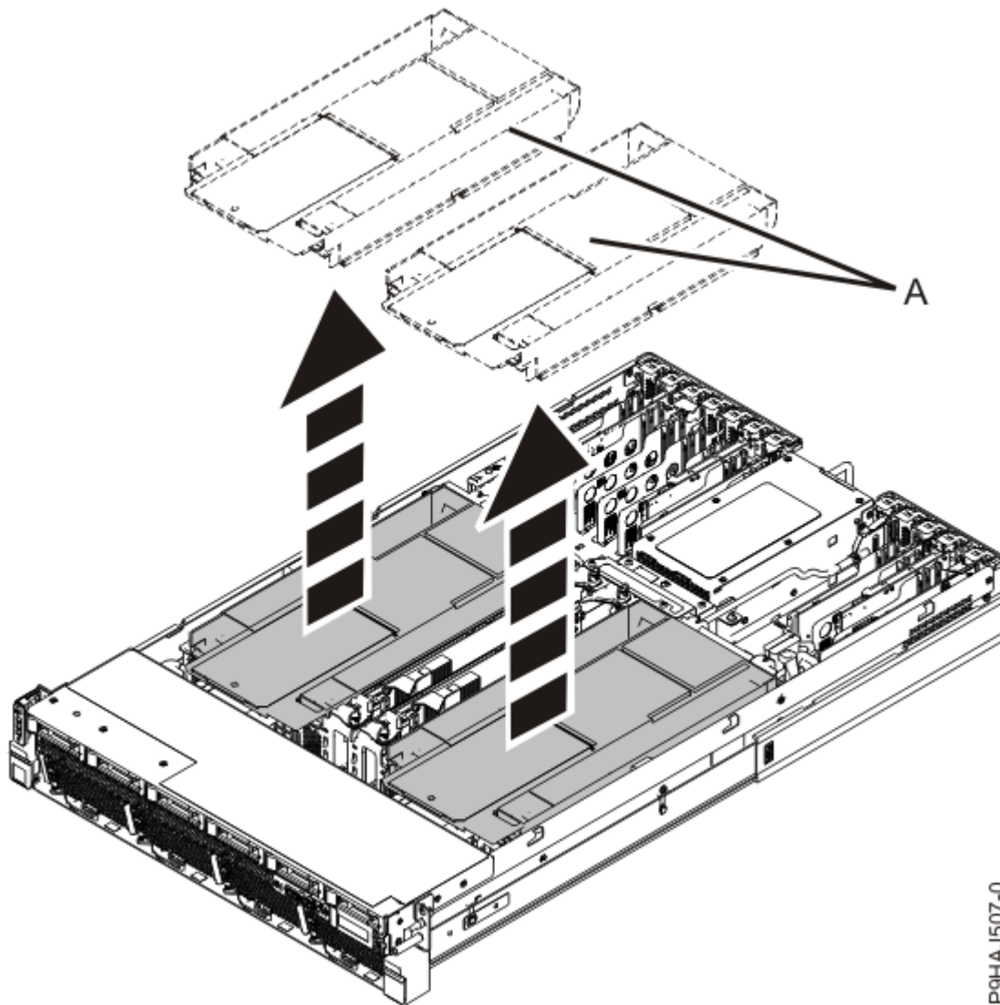
รูปที่ 8. การถอดตัวโหลเวียนอากาศ
