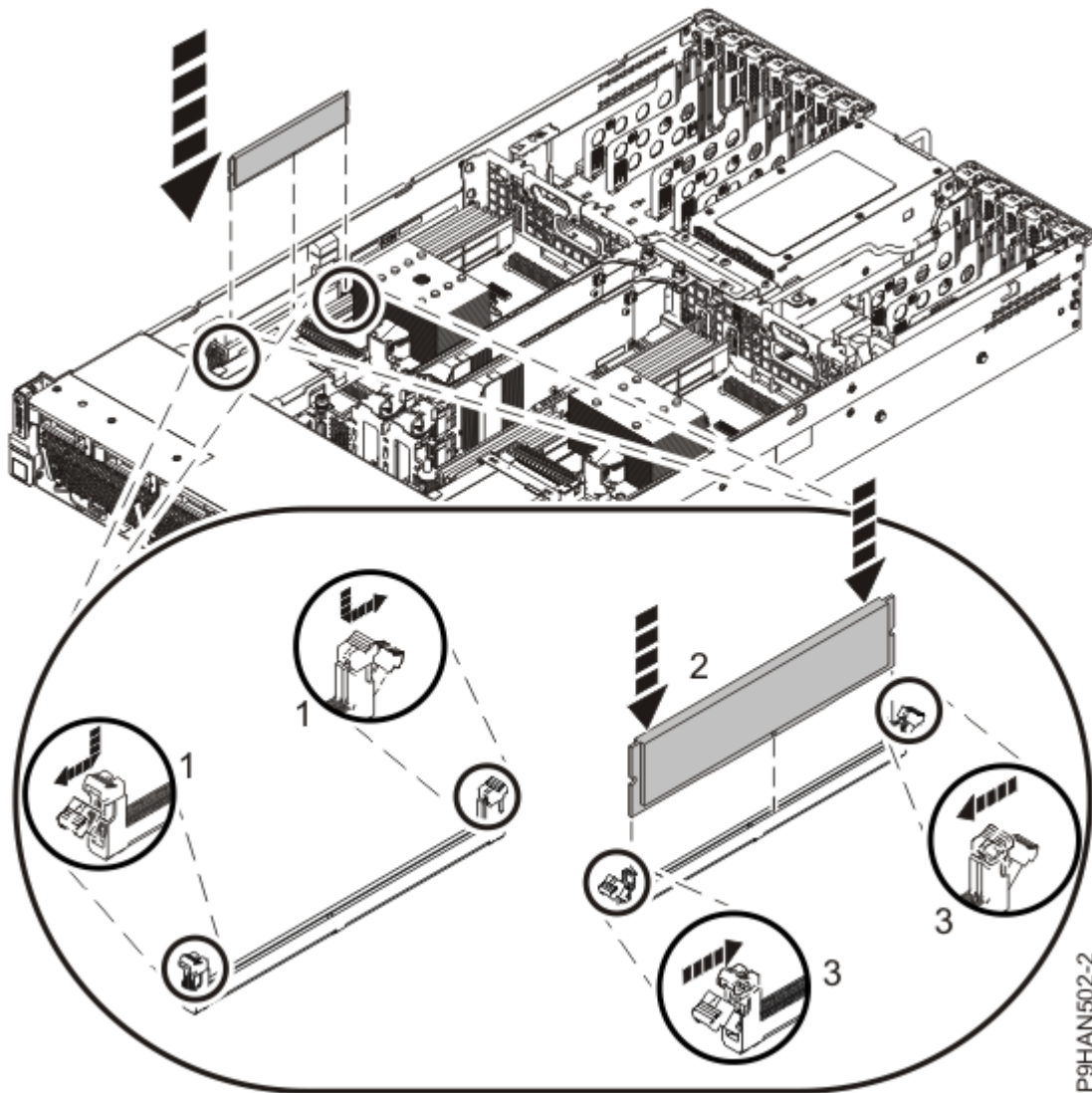
รูปที่ 9. การติดตั้ง โมดูลหน่วยความจำ
