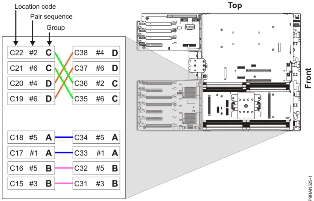
รูปที่ 28. ลำดับของการเชื่อมต่อ ตัวประมวลผลระบบหนึ่งตัว ระบบสแตนด์อะโลน
