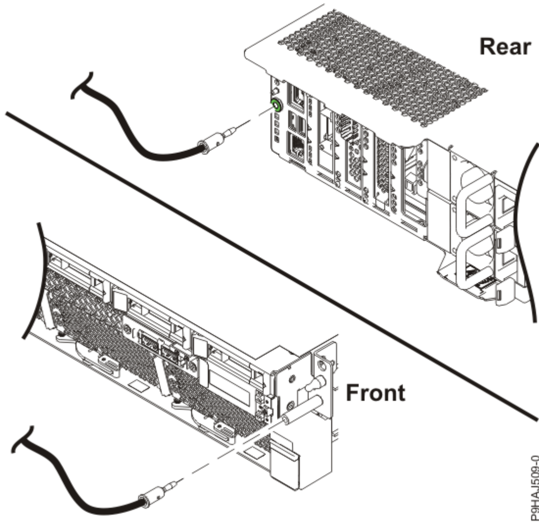
รูปที่ 32. ตำแหน่งของปลั๊ก ESD
