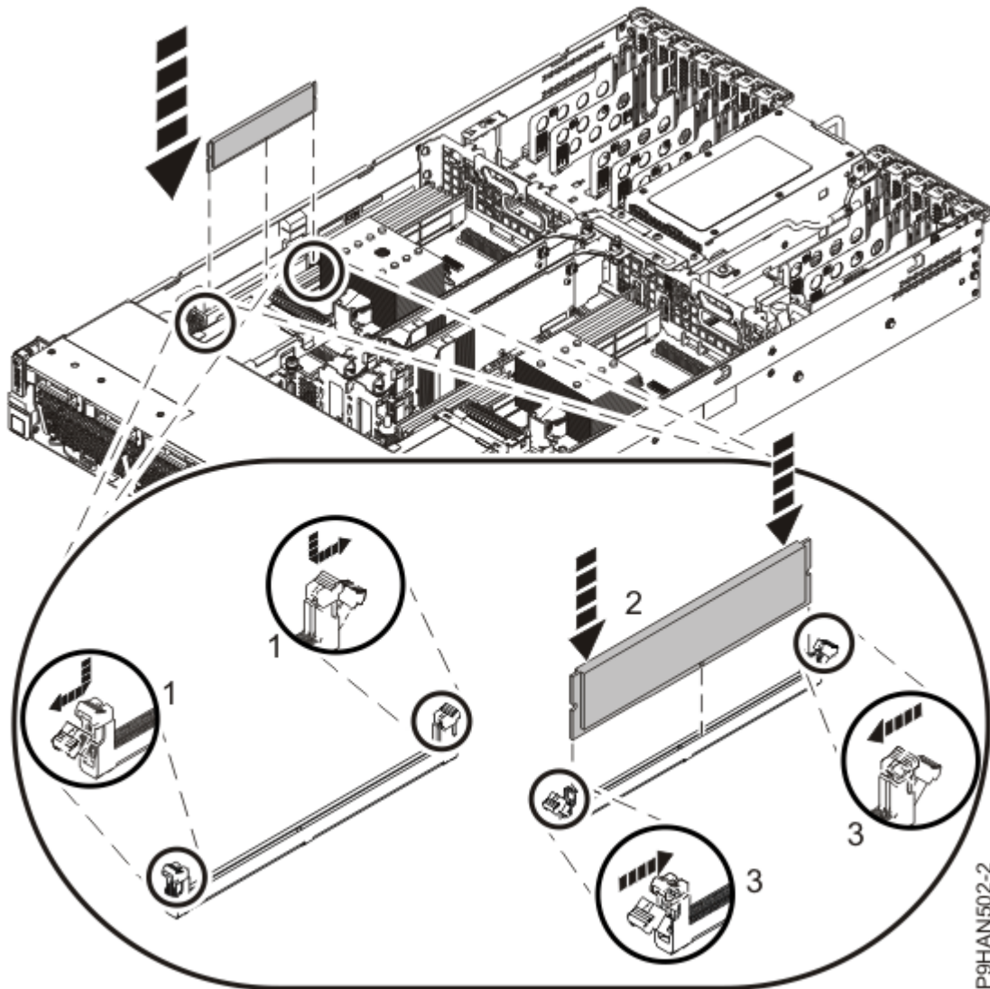
รูปที่ 22. การเปลี่ยน โมดูลหน่วยความจำ
