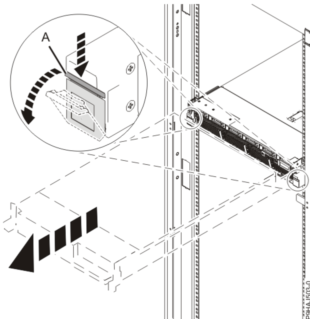
รูปที่ 15. การปลดแลตซ์ด้านข้าง
