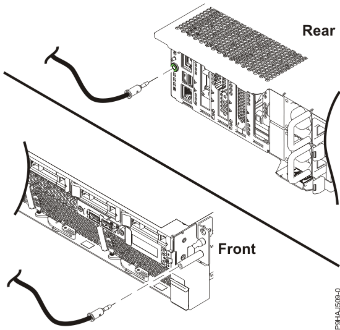
รูปที่ 6. ตำแหน่งของปลั๊ก ESD
