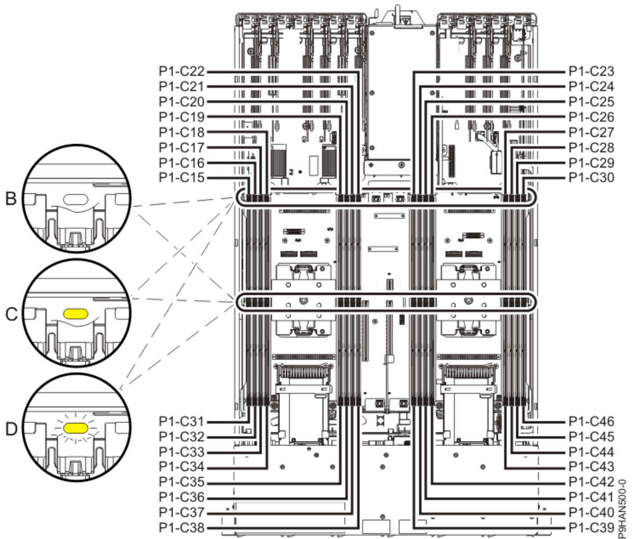
รูปที่ 19. LEDs สำหรับการทำงานและ โมดูลหน่วยความจำ ที่ล้มเหลว
