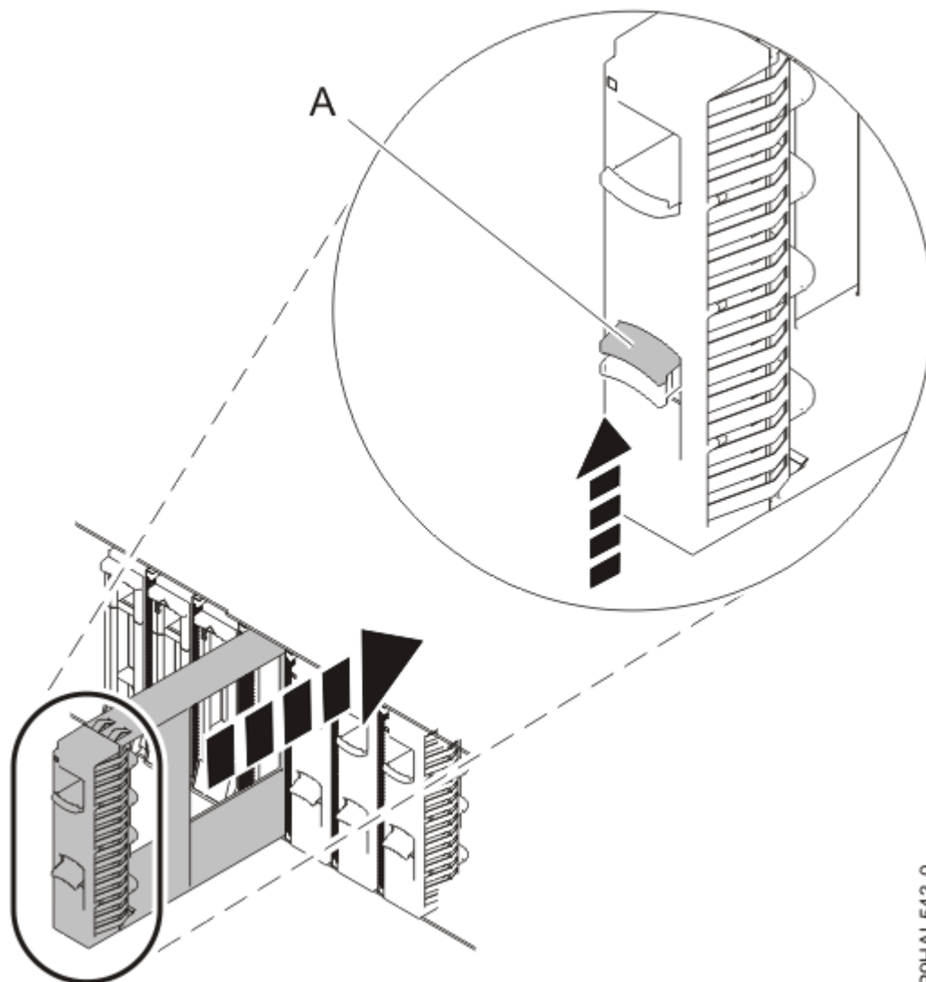
รูปที่ 31. การติดตั้งไดรฟ์ฟลเลอร์ในระบบ
