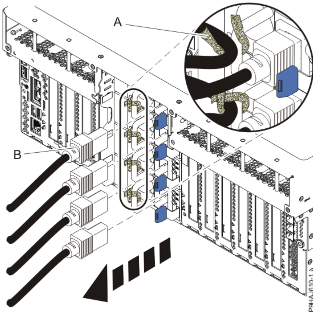
รูปที่ 28. การถอดสายไฟจากเซิร์ฟเวอร์ที่ประกอบเข้ากับชั้นวาง
