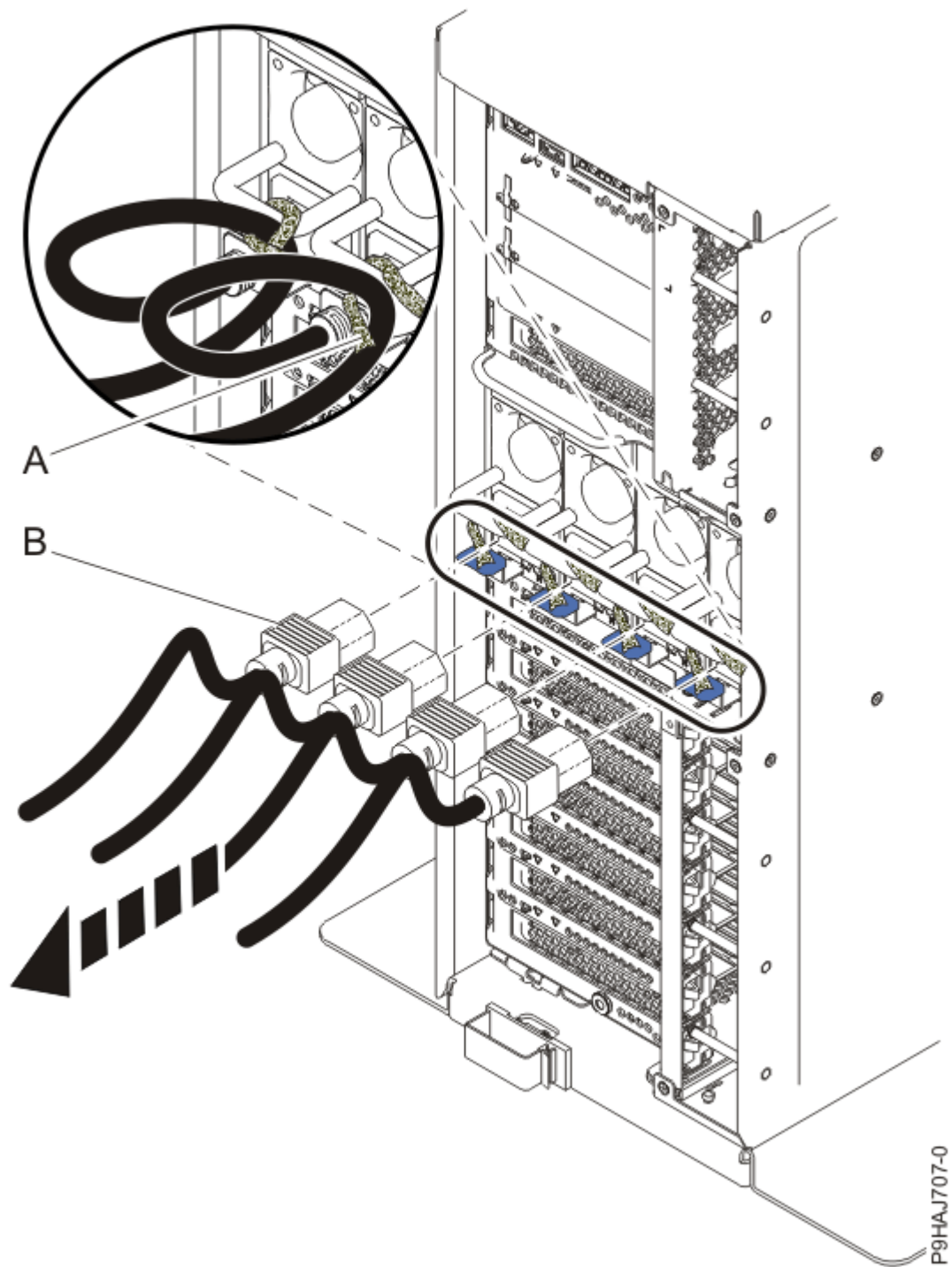
รูปที่ 4. การถอดสายไฟจากเซิร์ฟเวอร์แบบสแตนด์อะโลน
