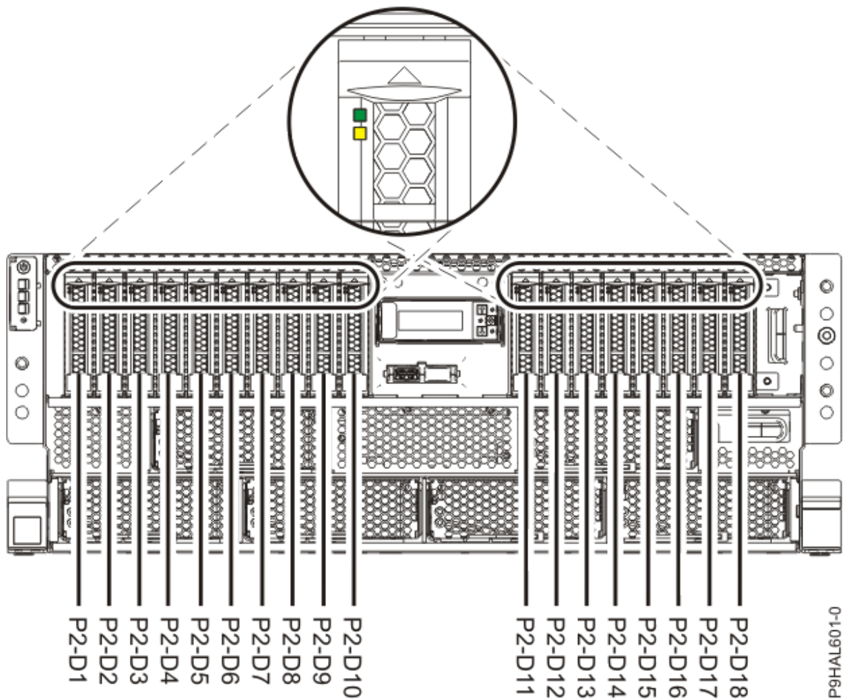
รูปที่ 11. ตำแหน่งดิสก์ไดรฟ์หรือโซลิดสเตตไดรฟ์และตัวบ่งชี้เซอวิสในระบบ 9009-41A, 9009-42A หรือ 9223-42H ที่ประกอบเข้ากับชั้นวาง
