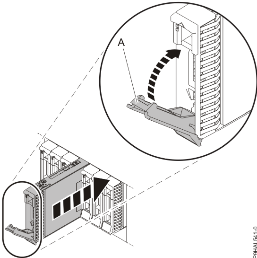
รูปที่ 21. การติดตั้งไดรฟ์ในระบบ
