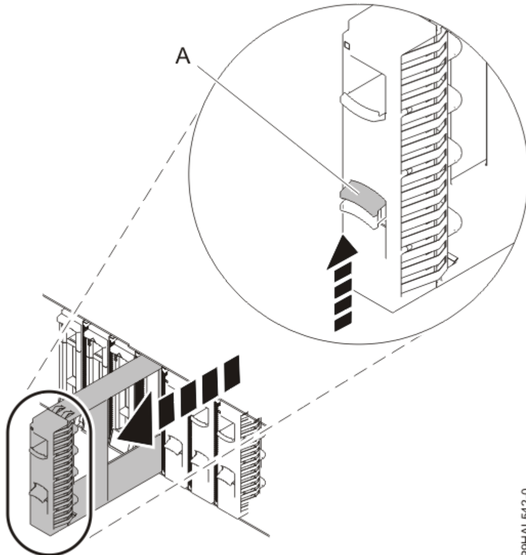
รูปที่ 5. การถอดฟิลเลอร์ของไดรฟ์
