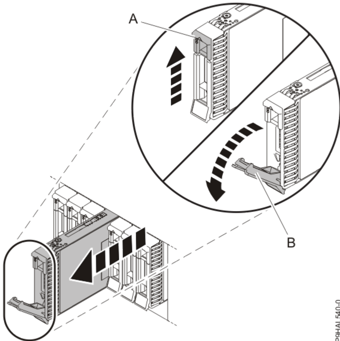
รูปที่ 15. การปลดล็อกและการถอดไดรฟ์
