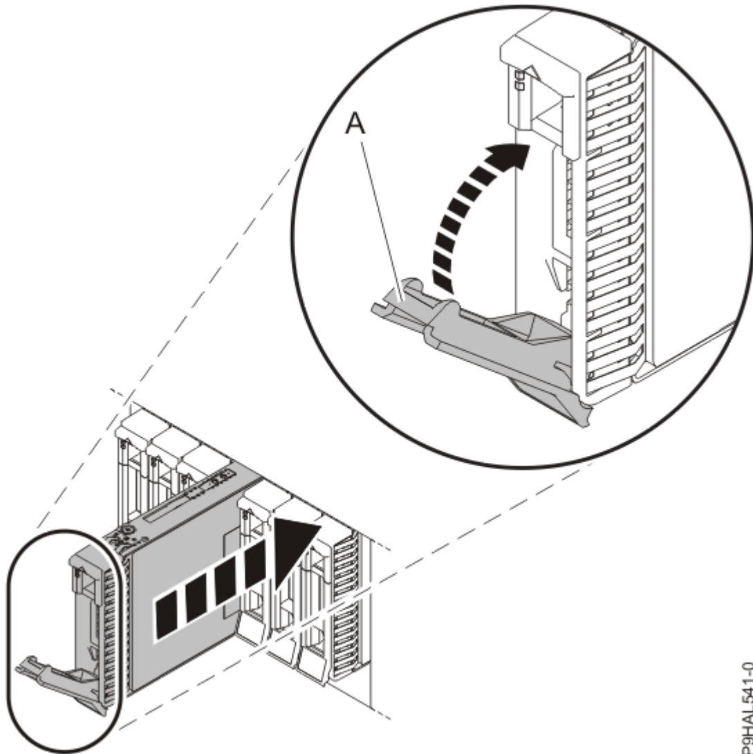
รูปที่ 19. การติดตั้งไดรฟ์ในระบบ
