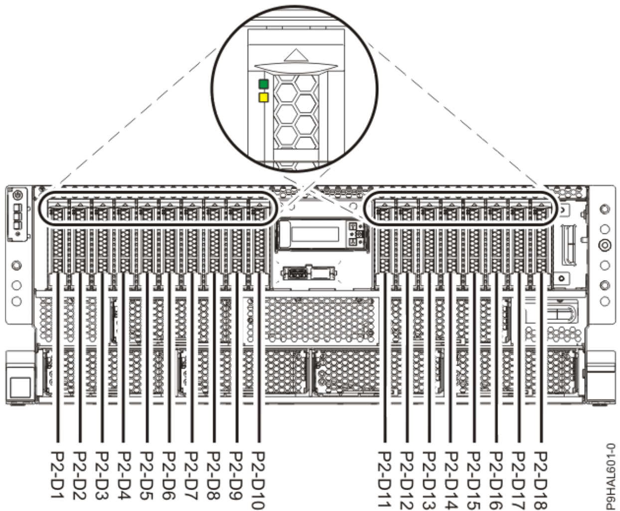
รูปที่ 26. ตำแหน่งดิสก์ไดรฟ์หรือโซลิดสเตทไดรฟ์และตัวบ่งชี้เซอร์วิสในระบบ 9009-41A, 9009-42A หรือ 9223-42H ที่ประกอบเข้ากับชั้นวาง
