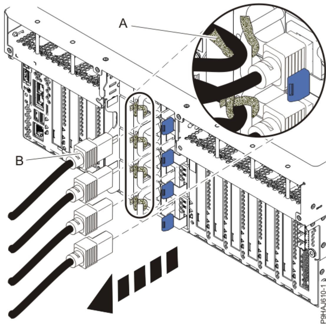
รูปที่ 13. การถอดสายไฟจากเซิร์ฟเวอร์ที่ประกอบเข้ากับชั้นวาง
