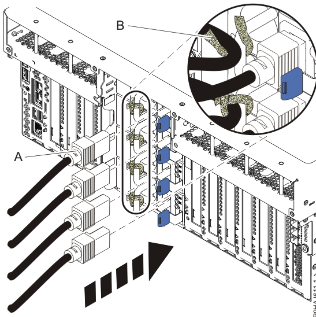
รูปที่ 9. การเชื่อมต่อสายไฟเข้ากับระบบที่ประกอบเข้ากับชั้นวาง
