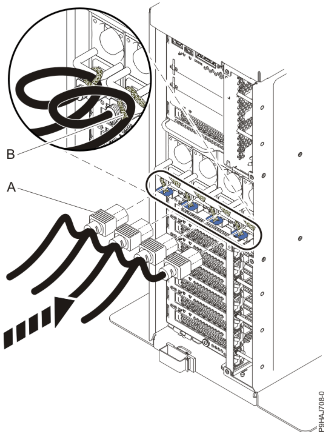
รูปที่ 10. การเชื่อมต่อสายไฟเข้ากับระบบแบบสแตนด์เอโลน
