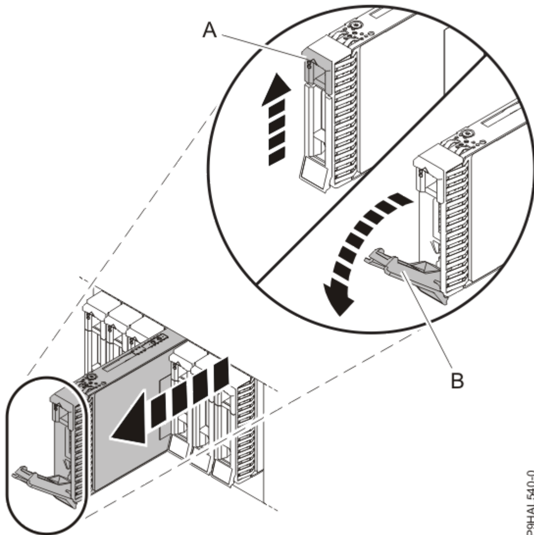
รูปที่ 17. การปลดล็อกและการถอดไดรฟ์
