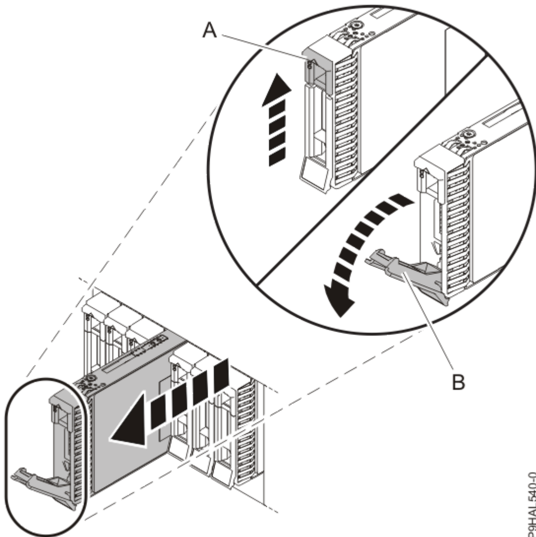
รูปที่ 30. การปลดล็อกและการถอดไดรฟ์
