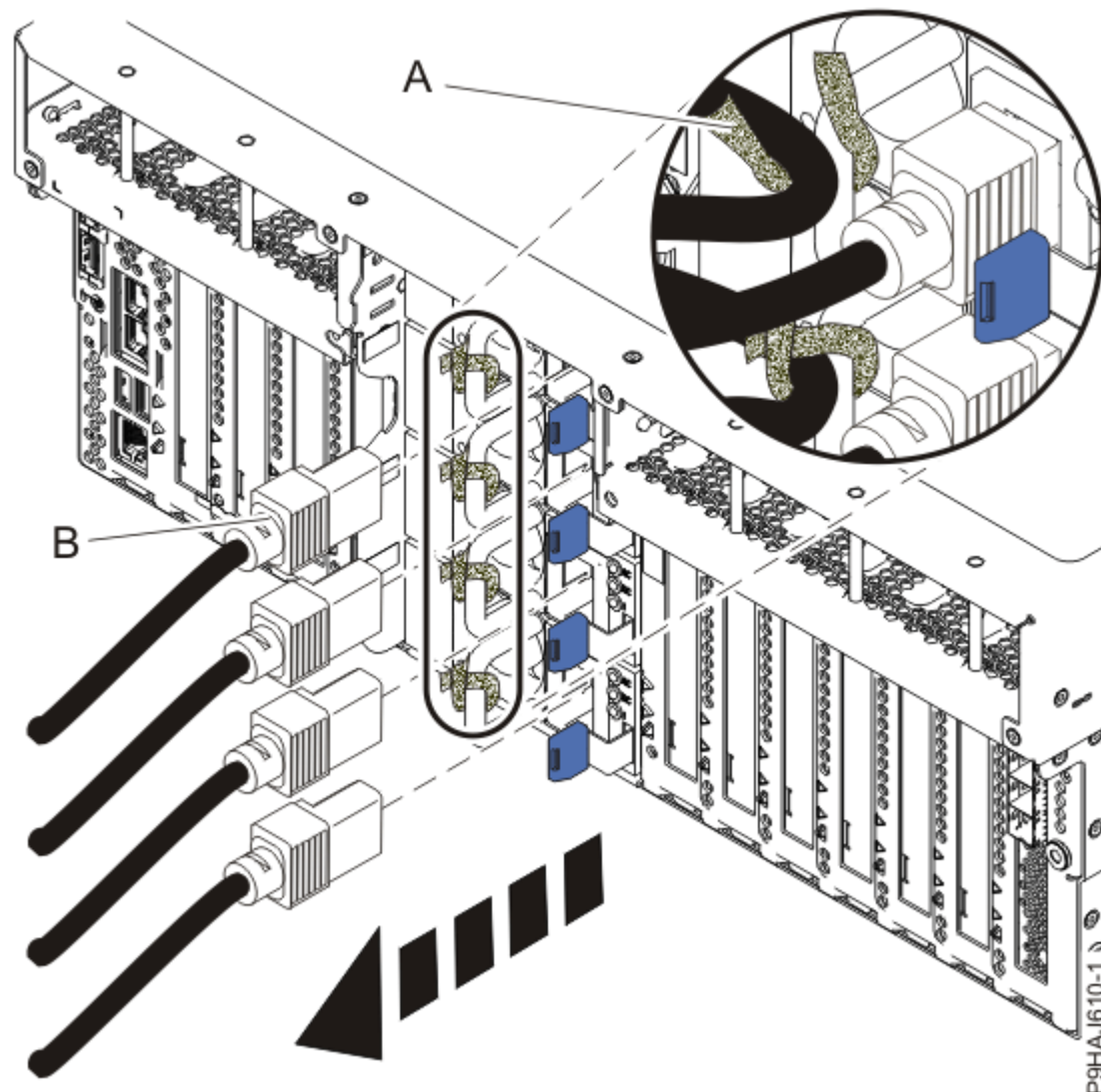
รูปที่ 3. การถอดสายไฟจากเซิร์ฟเวอร์ที่ประกอบเข้ากับชั้นวาง
