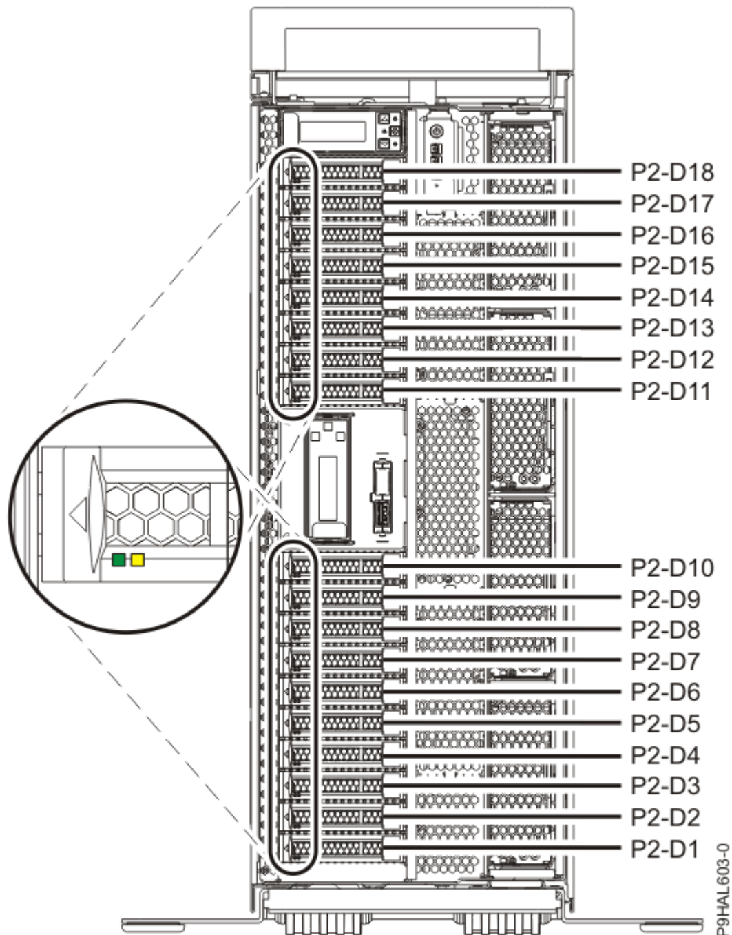
รูปที่ 2. ตำแหน่งดิสก์ไดรฟ์หรือโซลิดสเตตไดรฟ์และตัวบ่งชี้เซอวิวิสในระบบ 9009-41A, 9009-42A หรือ 9223-42H แบบสแตนด์อะโลน
