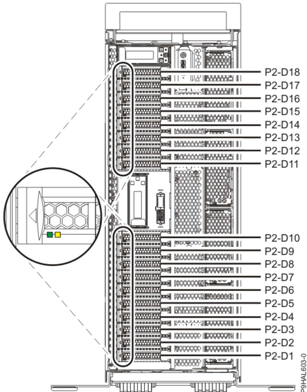
รูปที่ 27. ตำแหน่งดิสก์ไดรฟ์หรือโซลิดสเตตไดรฟ์และตัวบ่งชี้เซอร์วิสในระบบ 9009-41A, 9009-42A หรือ 9223-42H แบบสแตนด์อะโลน
