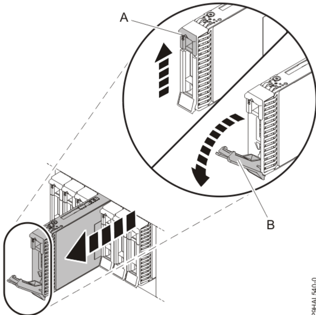
รูปที่ 16. การปลดล็อกและการถอดไดรฟ์
