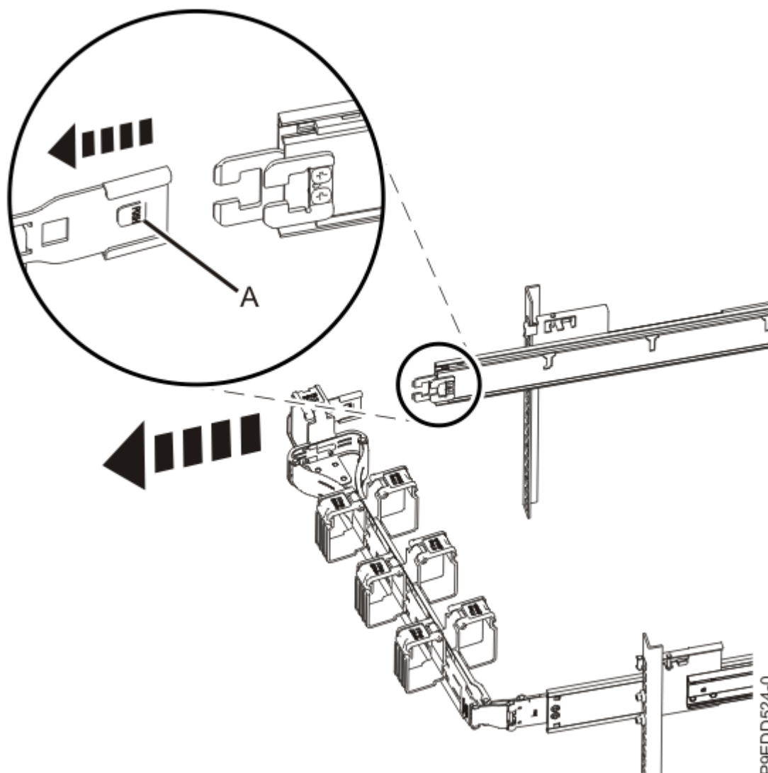
รูปที่ 22. การปลดแขนยึดการจัดการสายเคเบิล
