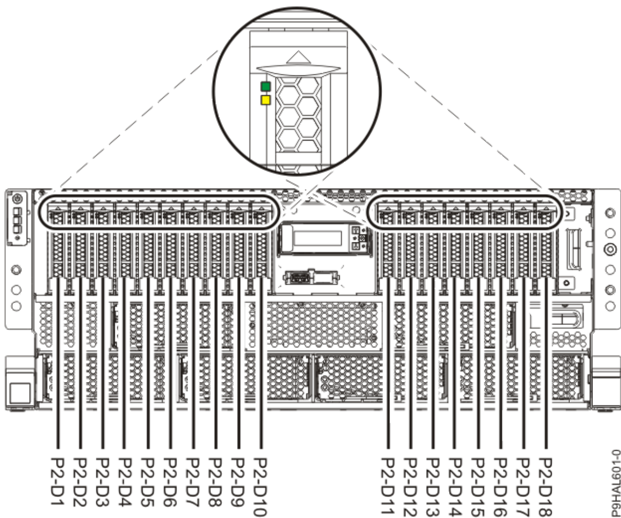
รูปที่ 1. ตำแหน่งดิสก์ไดรฟ์หรือโซลิดสเตตไดรฟ์และตัวบ่งชี้เซอร์วิสในระบบ 9009-41A, 9009-42A หรือ 9223-42H ที่ประกอบเข้ากับชั้นวาง
