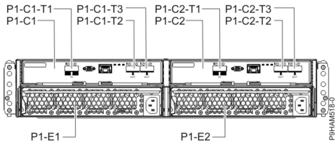
รูปที่ 8. มุมมองด้านหลังของ 5887 กล่องหุ้ม ดิสก์ไดรฟ์
