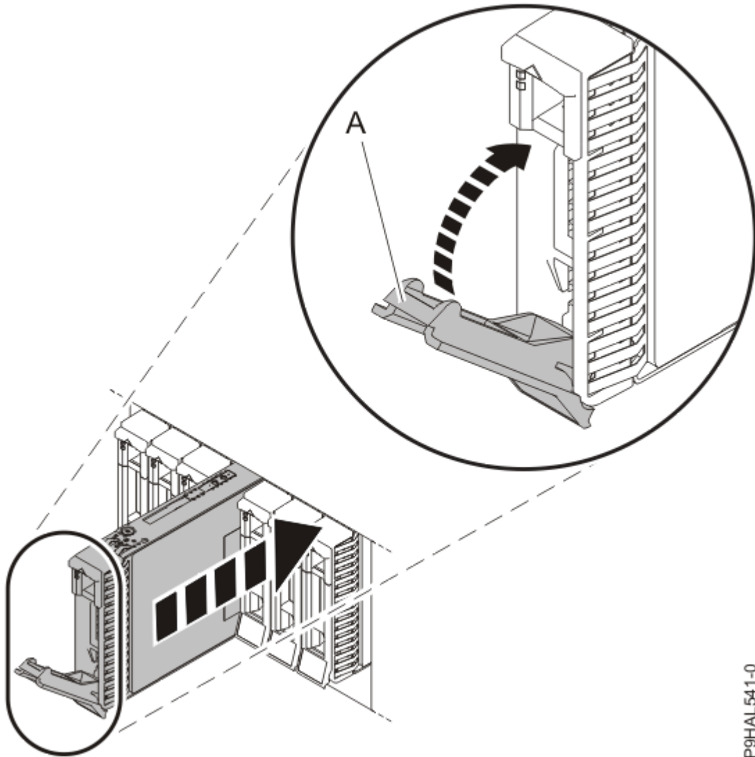
รูปที่ 14. การเปลี่ยนไดรฟ์ในกล่องหุ้ม
