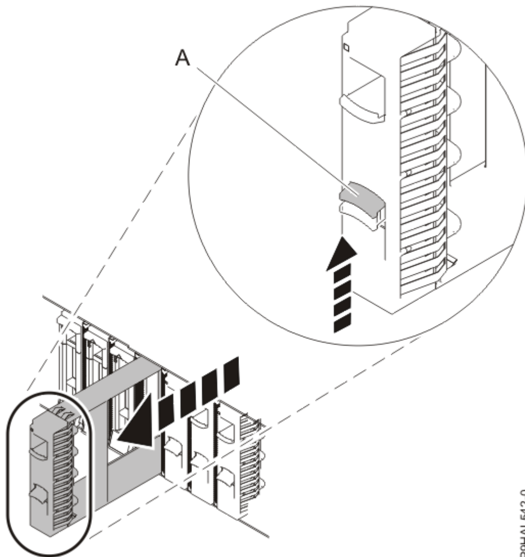
รูปที่ 4. การถอดฟิลเลอร์ของไดรฟ์
