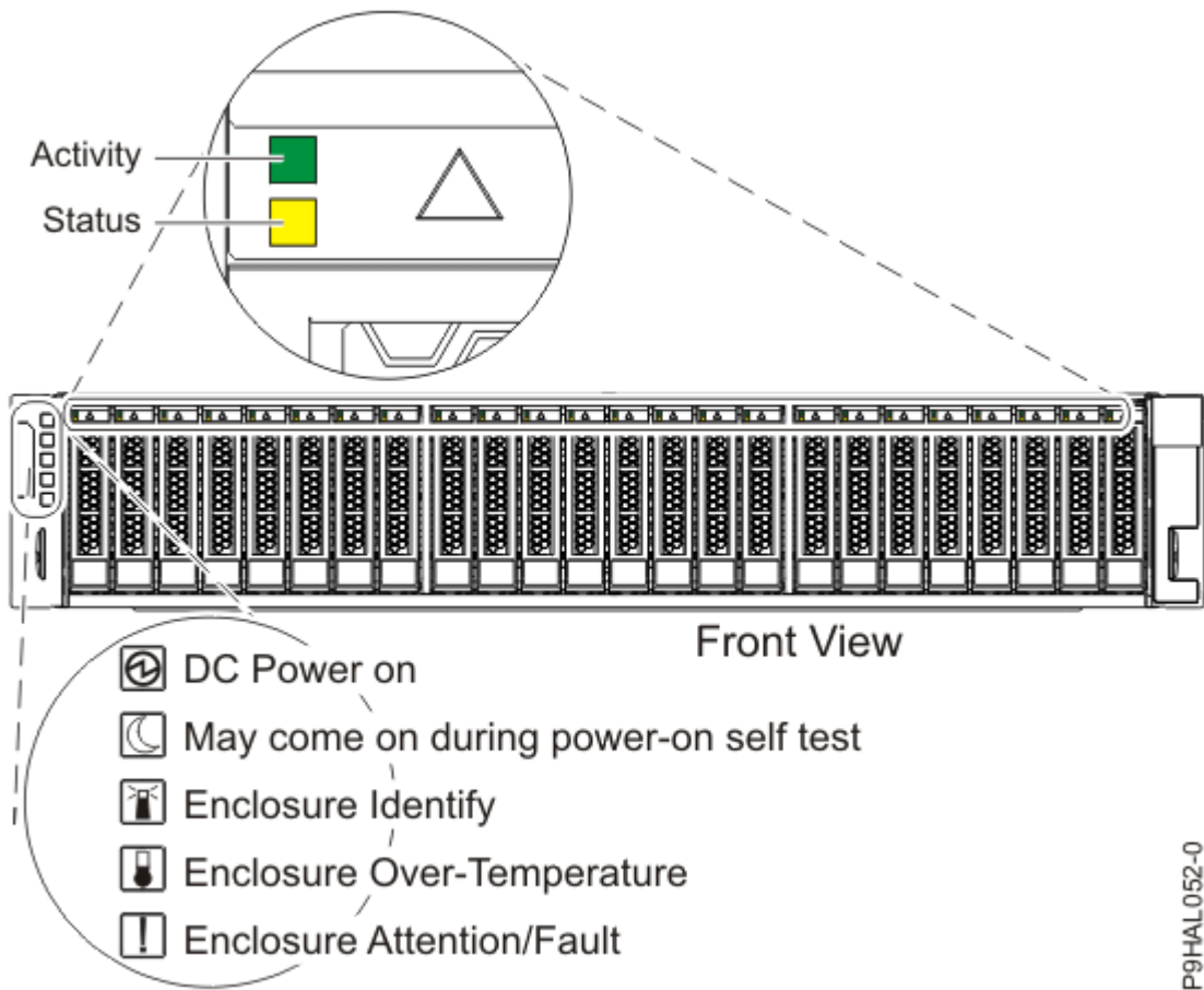
รูปที่ 3. มุมมองด้านหน้าของ 5887 กล่องหุ้ม ดิสก์ไดรฟ์ ที่แสดง ไฟแสดงสถานะเซอร์วิส
