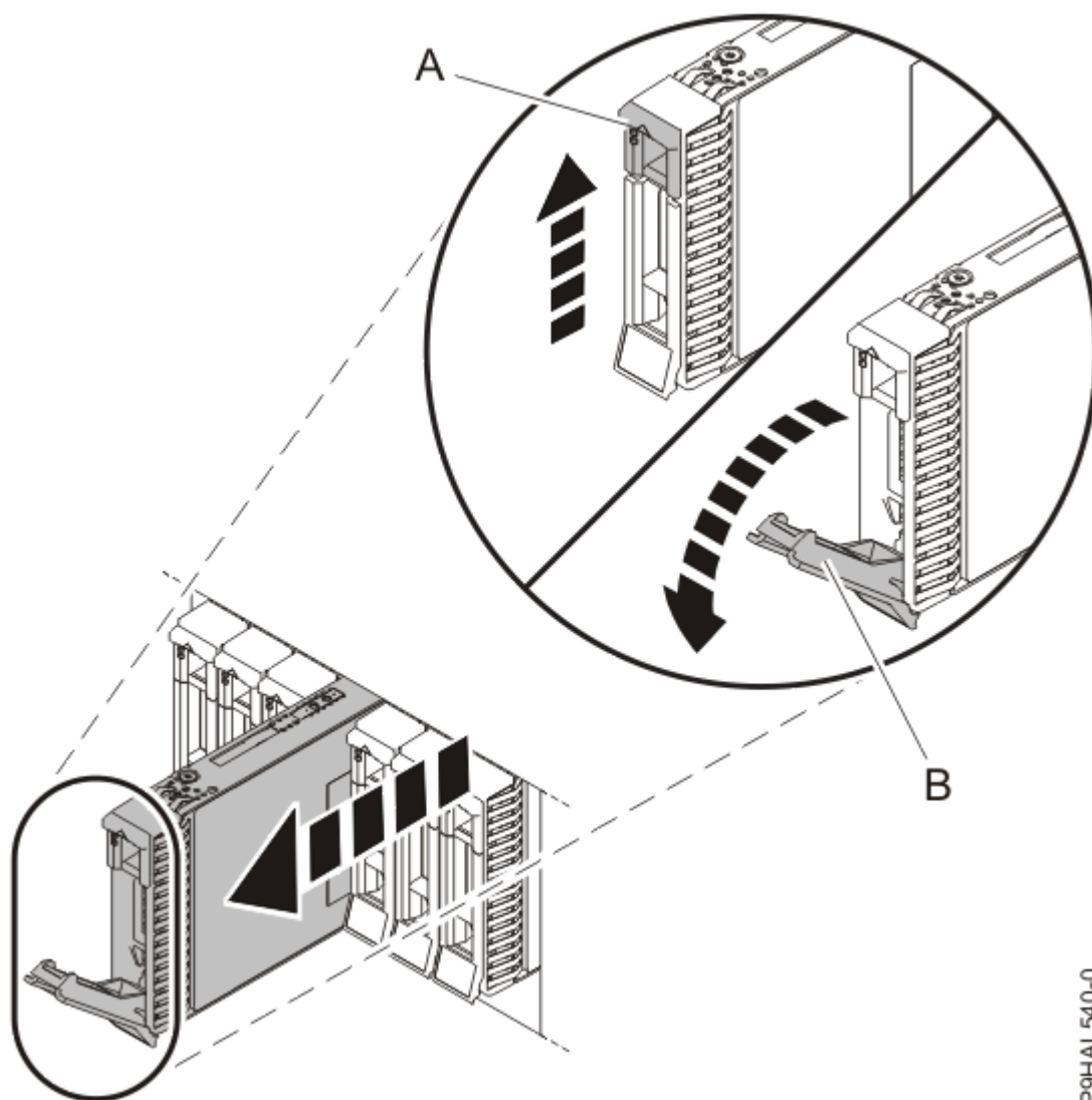
รูปที่ 10. การปลดล็อกและการถอดไดรฟ์
