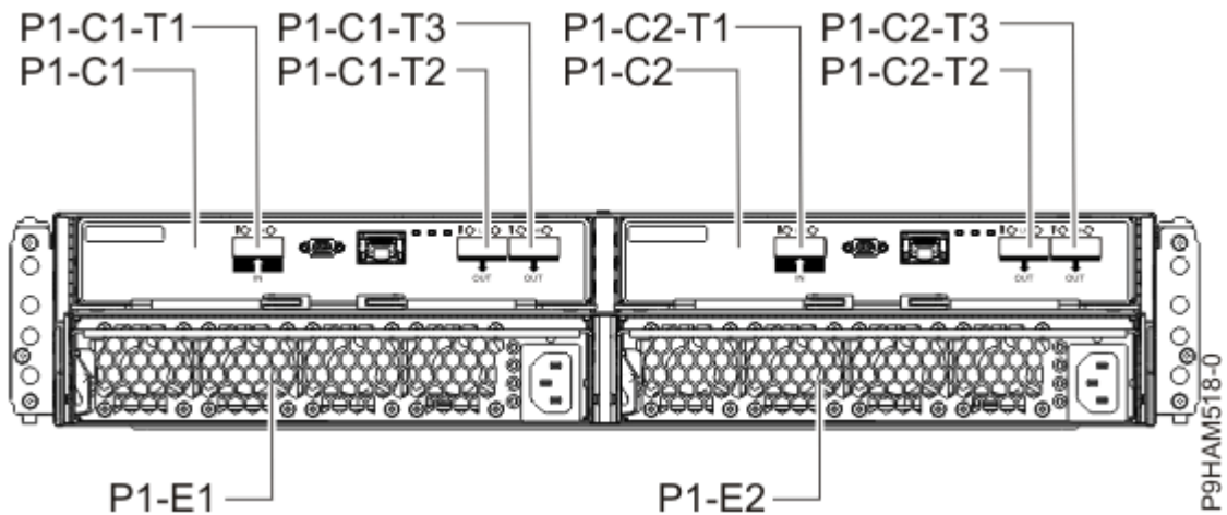
รูปที่ 2. มุมมองด้านหลังของ 5887 กล่องหุ้ม ดิสก์ไดรฟ์
