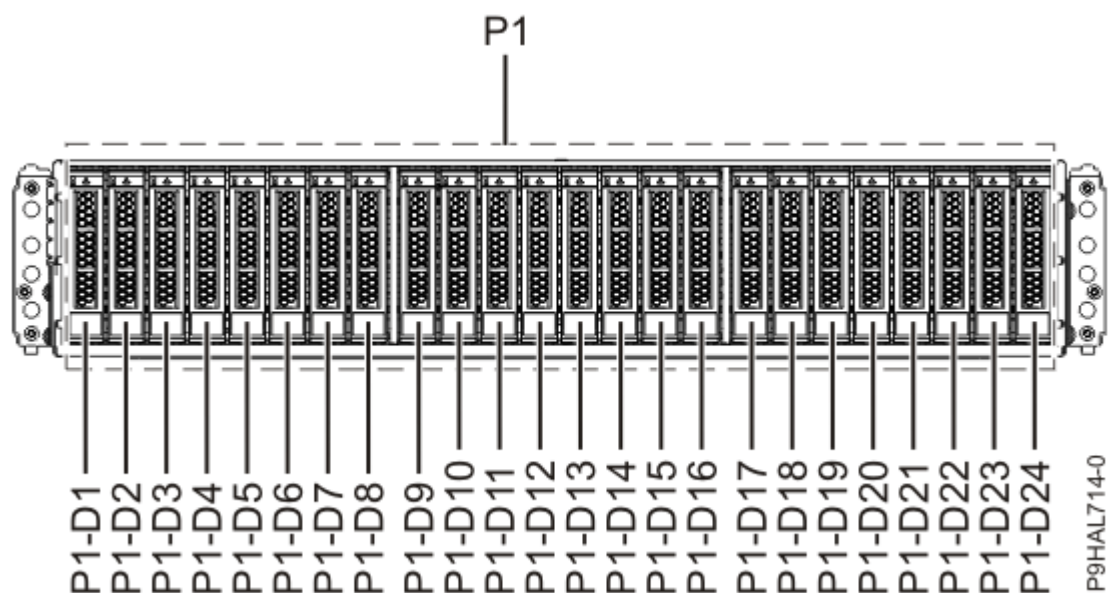
รูปที่ 7. มุมมองด้านหน้าของ 5887 กล่องหุ้ม ดิสก์ไดรฟ์ ที่แสดง ตำแหน่งของดิสก์ไดรฟ์
