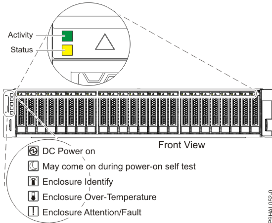
รูปที่ 9. มุมมองด้านหน้าของ 5887 กล่องหุ้ม ดิสก์ไดรฟ์ ที่แสดง ไฟแสดงสถานะเซอร์วิส
