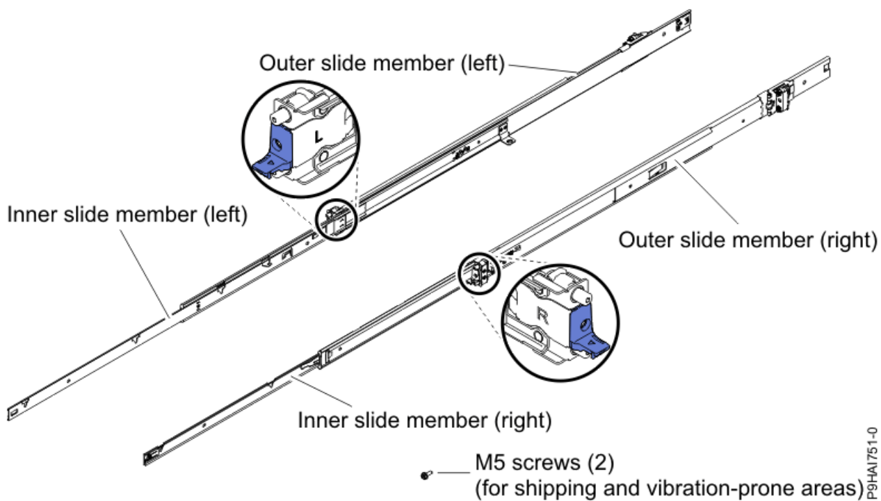
รูปที่ 10. ส่วนประกอบของกล่องราง
