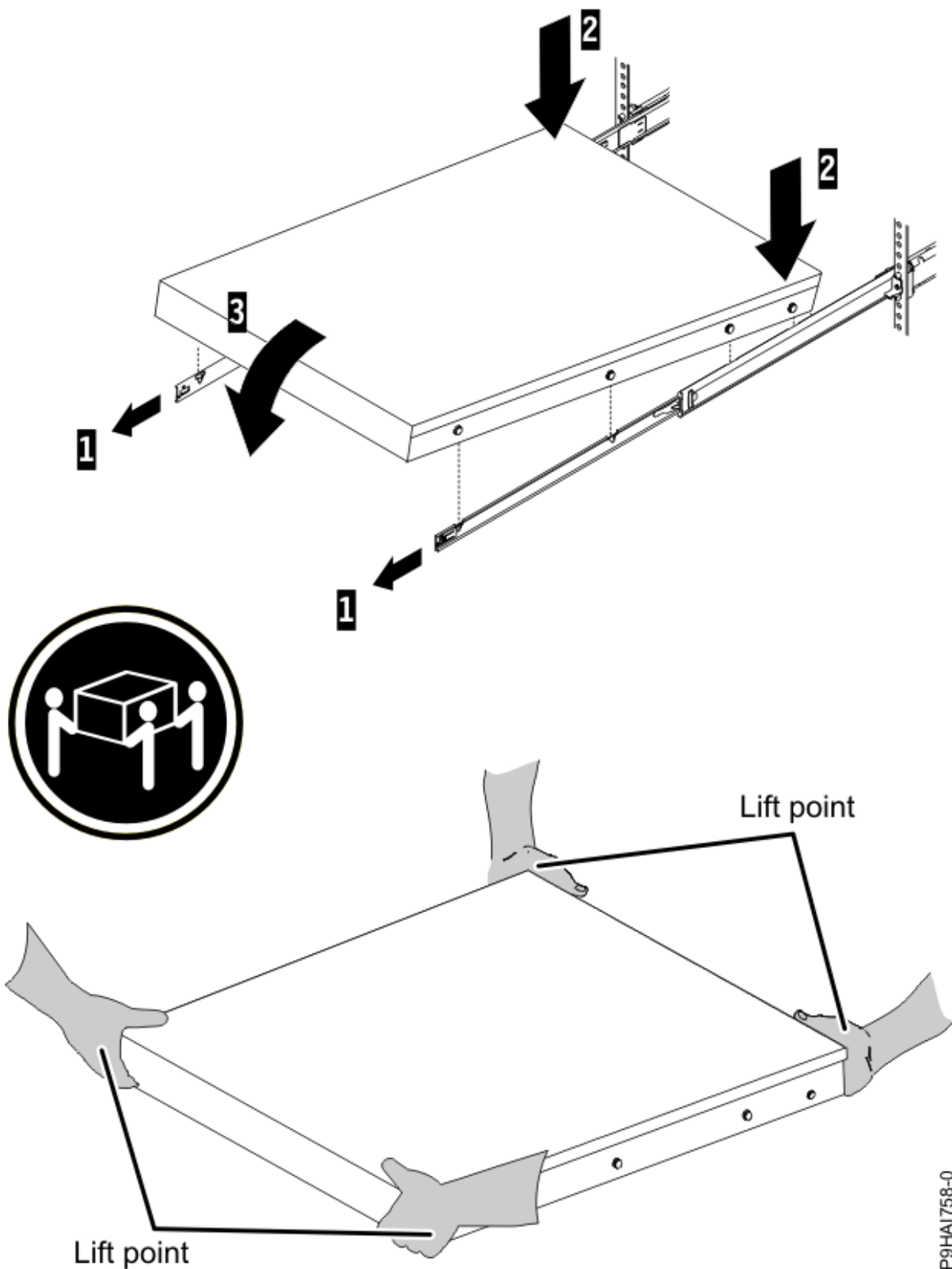
รูปที่ 16. รางสไลด์ ที่ขยายเพิ่ม หัวตะปูของเชิร์ฟเวอร์ที่จัดตำแหน่งให้ตรงกับช่องในราง และจุดยก
