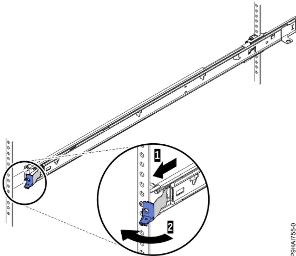
รูปที่ 14. แลตซ์รางสไลด์ ด้านหน้า
