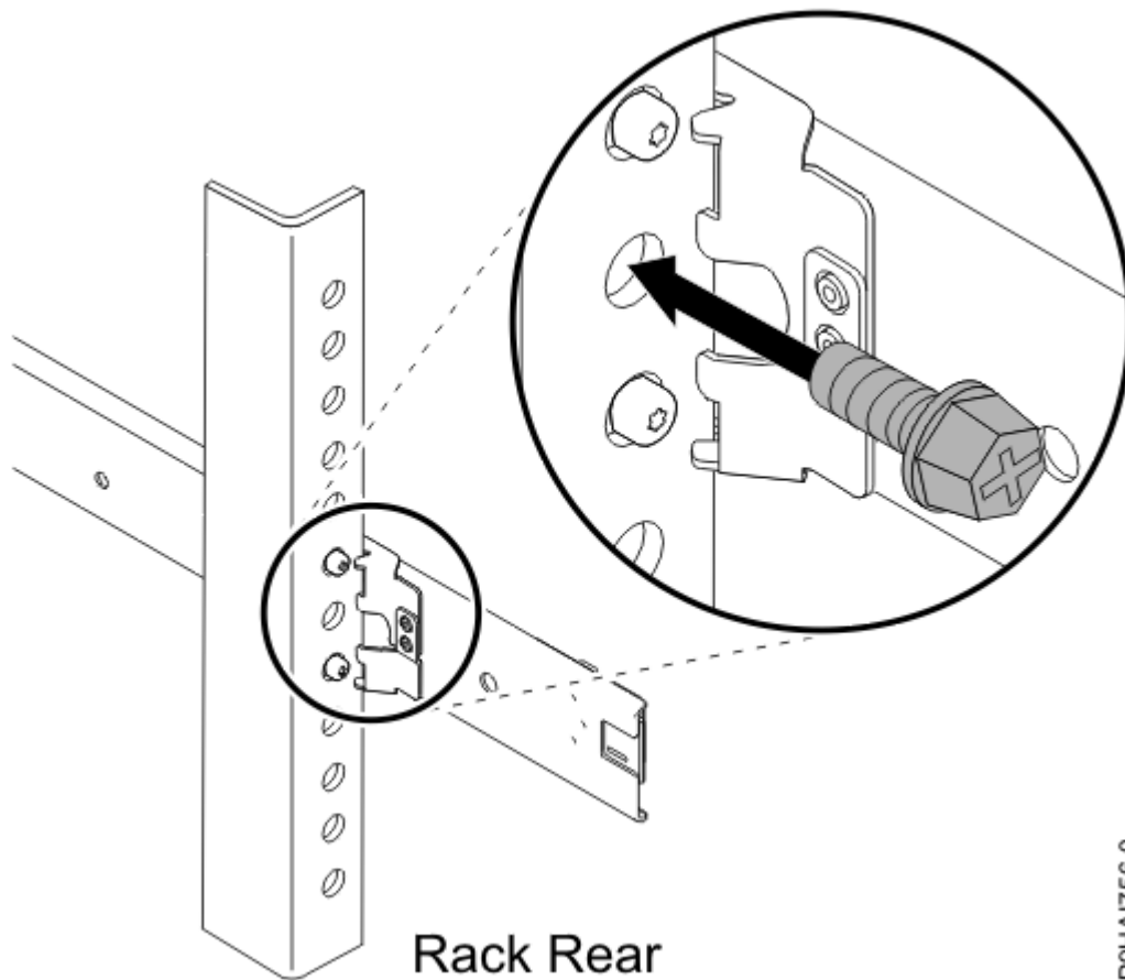
รูปที่ 24. การรักษาความปลอดภัยของ เซิร์ฟเวอร์สำหรับการจัดส่ง
