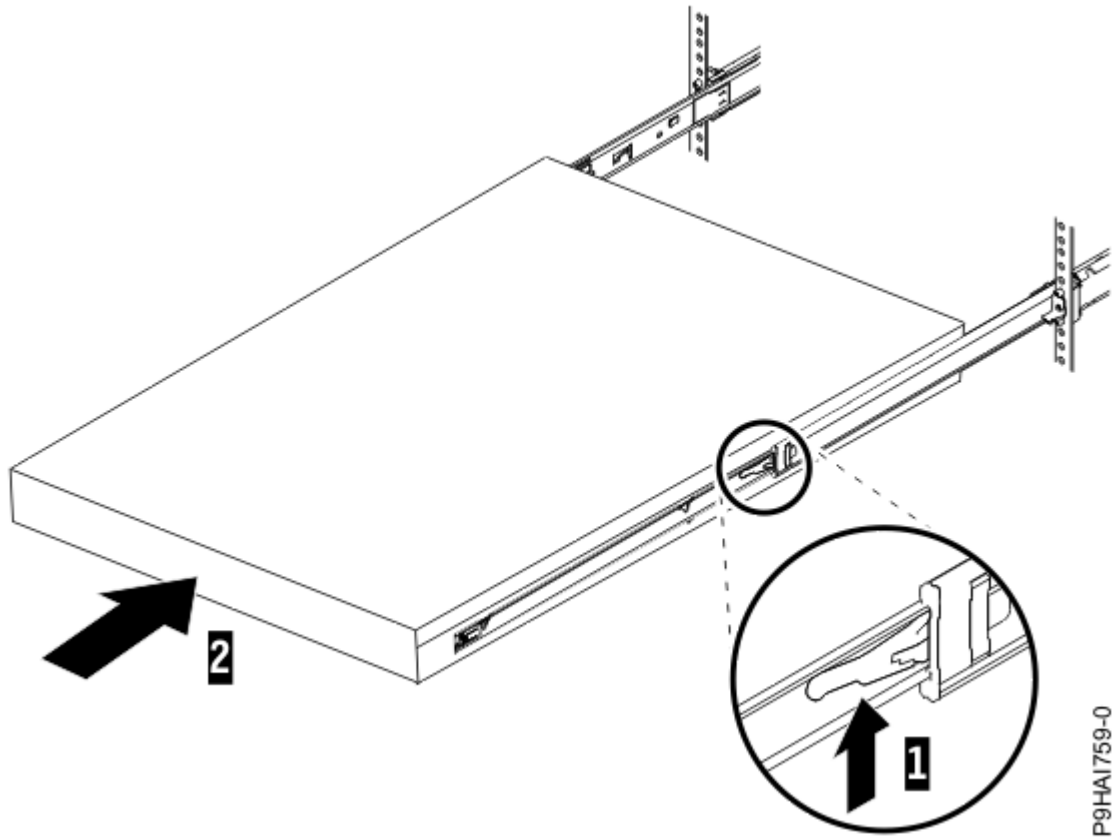
รูปที่ 17. ปลดแลตซ์และเซิร์ฟเวอร์
