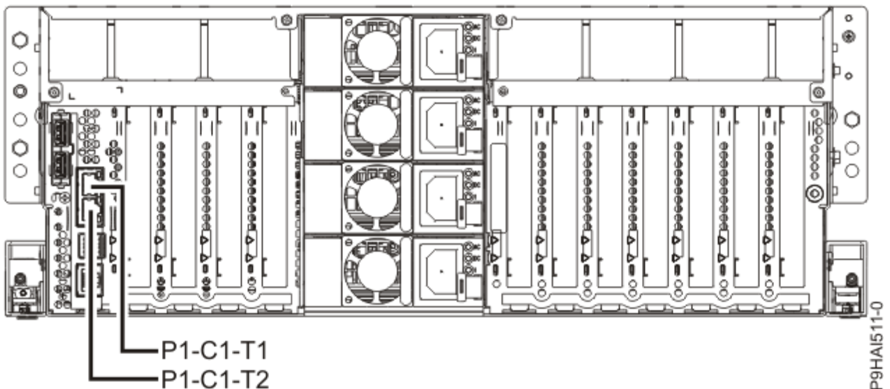
รูปที่ 27. 9009-41A, 9009-41G, 9009-42A, 9009-42G, 9223-42H และ 9223-42S ตำแหน่งพอร์ตของ HMC
