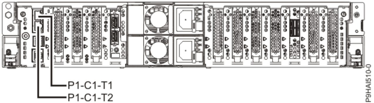
รูปที่ 26. 5105-22E, 9008-22L, 9009-22A, 9009-22G, 9223-22H และ 9223-22S ตำแหน่งพอร์ตของ HMC
