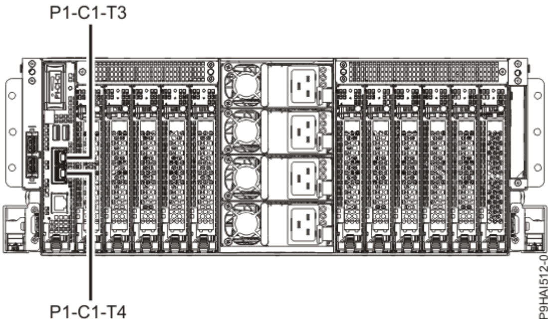
รูปที่ 28. ตำแหน่งพอร์ต HMC 9040-MR9
