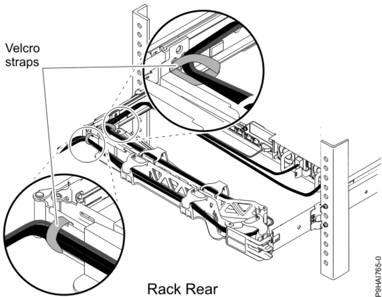
รูปที่ 23. ตัวรัด
