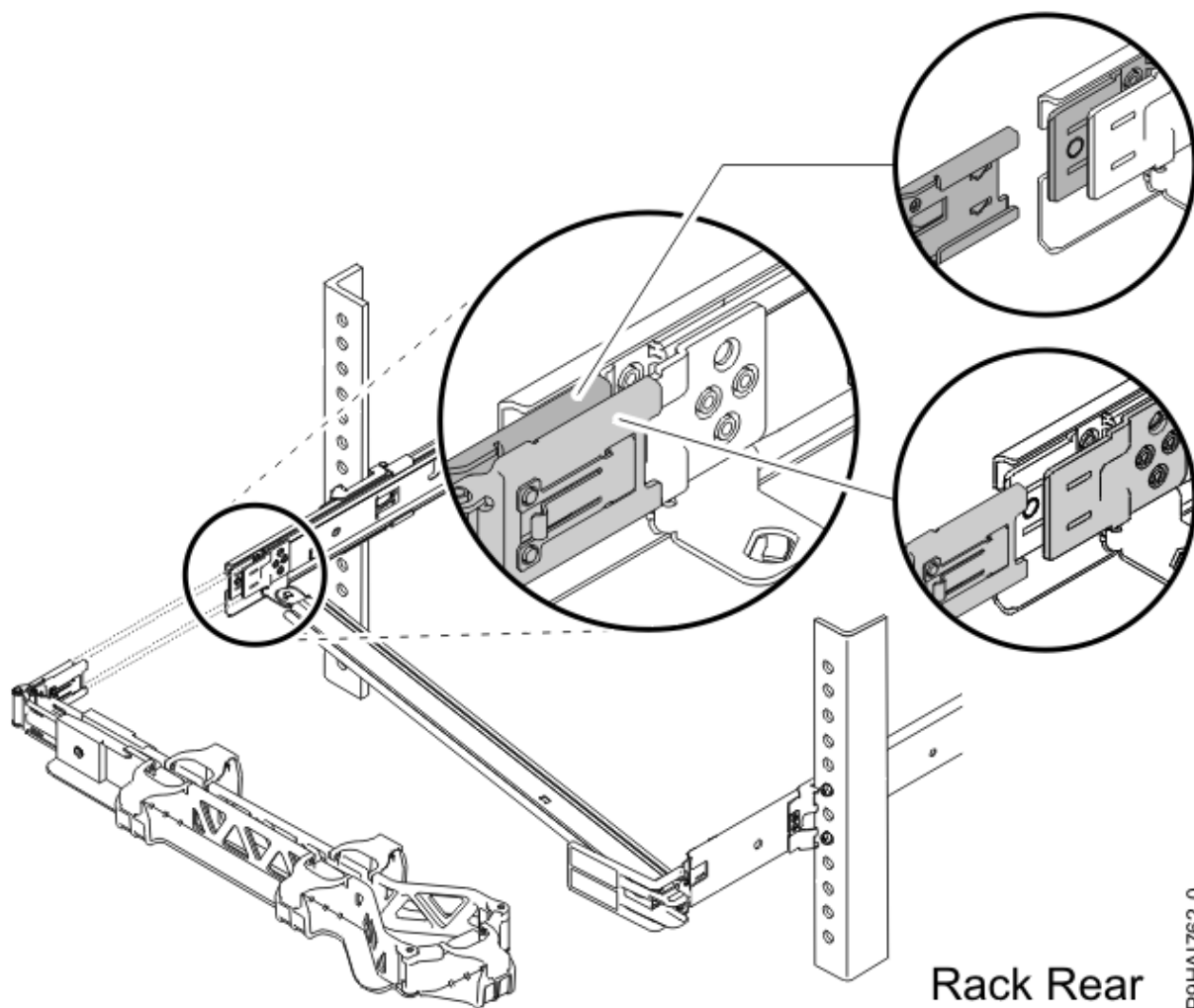
รูปที่ 20. การเชื่อมต่อแขนยึดสายเคเบิล
