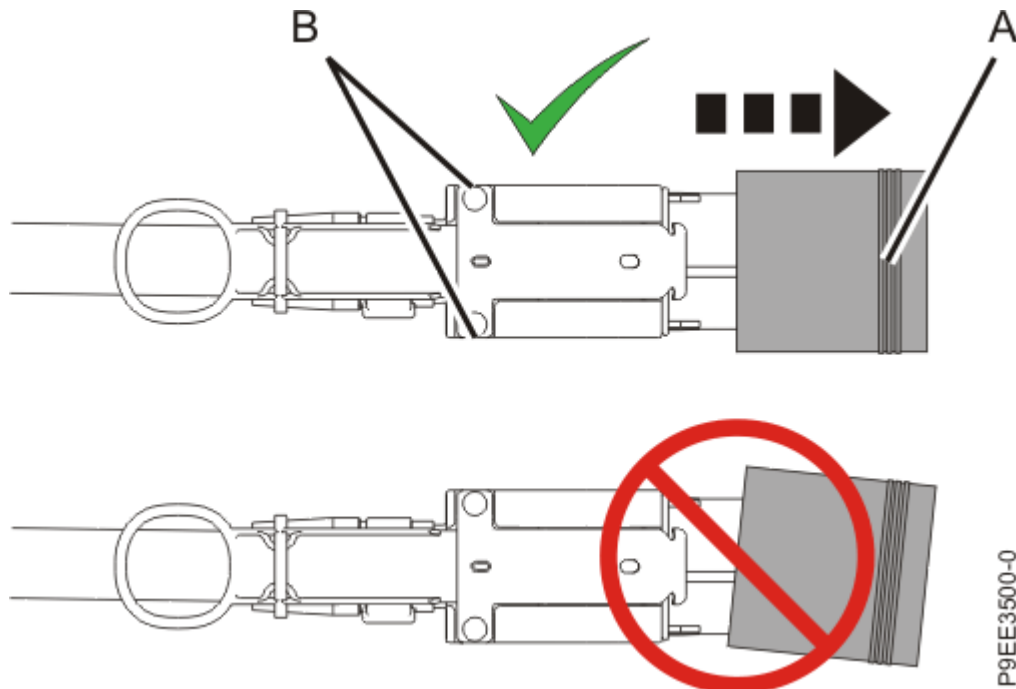
รูปที่ 5. การถอดฝาครอบป้องกันออกจากตัวเชื่อมต่อบน สายเคเบิลลิ้นชักส่วนขยาย
