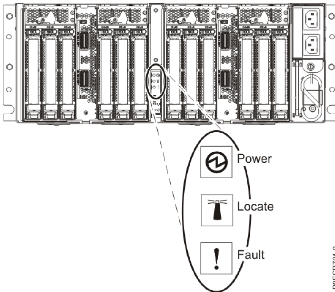
รูปที่ 9. ตัวบ่งชี้กำลังไฟ ด้านหลังสำหรับ ลินซ์กส่วนขยาย EMX0 PCIe3
