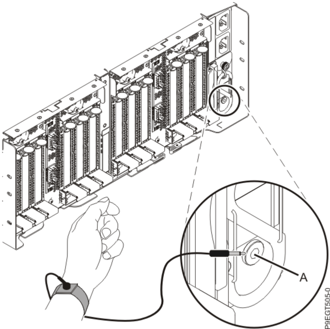
รูปที่ 1. ตำแหน่งของแฉีก ESD ทางด้านหลังของ ลื่นชักส่วนขยาย EMX0 PCIe3
