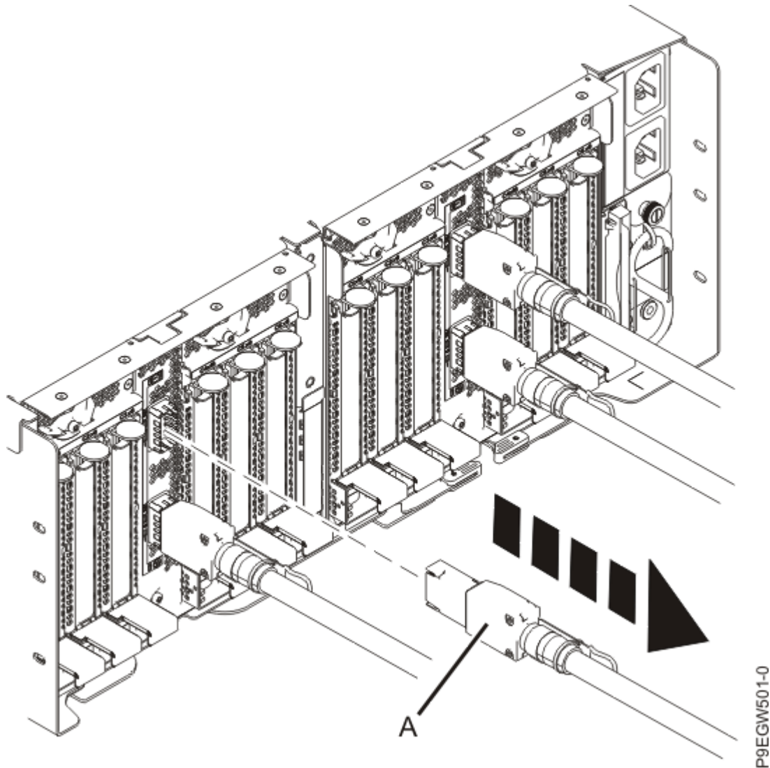
รูปที่ 4. การถอด สายเคเบิลลิ้นชักส่วนขยาย ออกจาก ลิ้นชักส่วนขยาย EMX0 PCIe3
