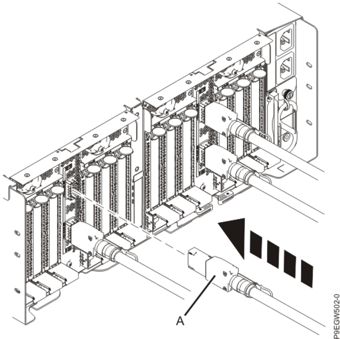
รูปที่ 7. การเปลี่ยน สายเคเบิลลิ้นชักส่วนขยาย ใน ลิ้นชักส่วนขยาย EMX0 PCIe3
