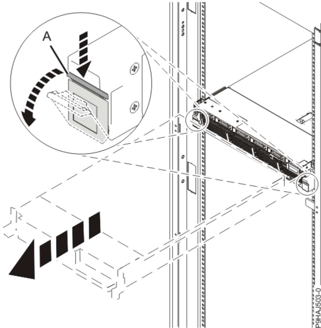
รูปที่ 11. การปลดแลตซ์ด้านข้าง
