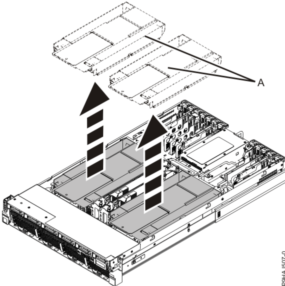
รูปที่ 4. การถอดตัวโหลเวียนอากาศ
