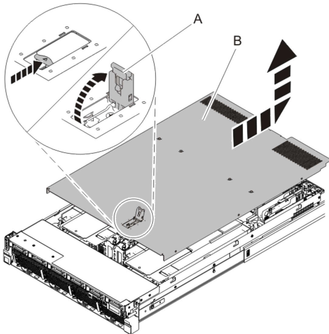
รูปที่ 12. การถอดฝาครอบการเข้าถึงเซอวิวิส
