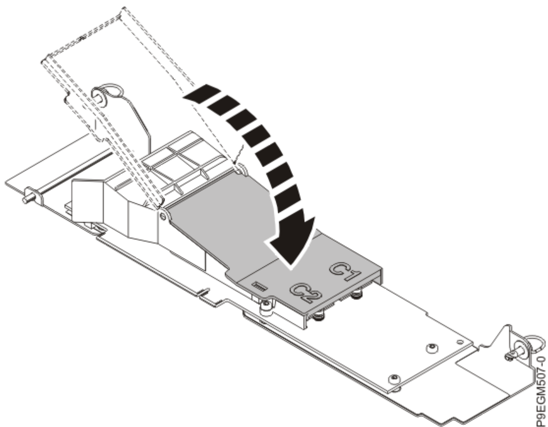
รูปที่ 7. การปิดฝาครอบสีดำของ NVMe M.2
