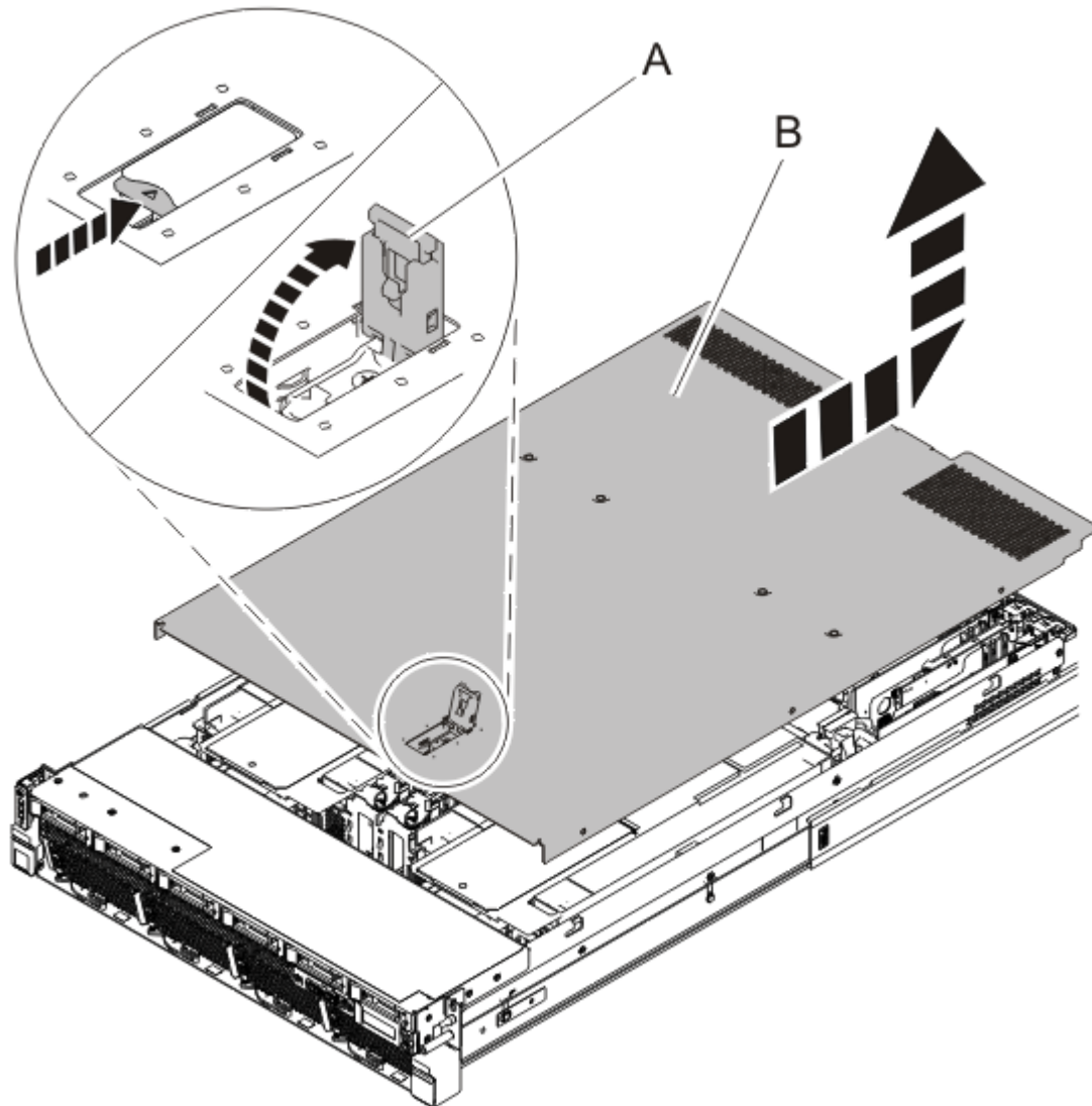
รูปที่ 3. การถอดฝาครอบการเข้าถึงเซอวิส
