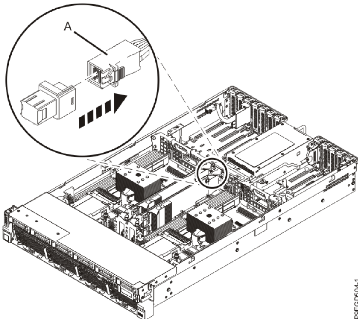
รูปที่ 21. การถอดสายเคเบิล SAS ด้านหลังออกจากอะแดปเตอร์ภายใน SAS RAID
