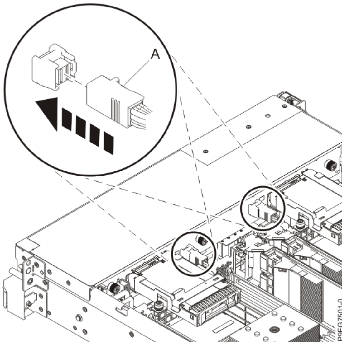
รูปที่ 10. การเชื่อมต่อสายเคเบิล SAS ด้านหน้า
