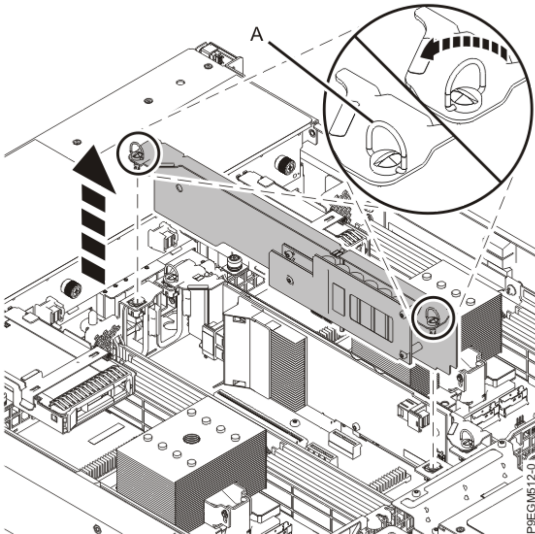
รูปที่ 23. การถอดโมดูลไฟสำรอง
