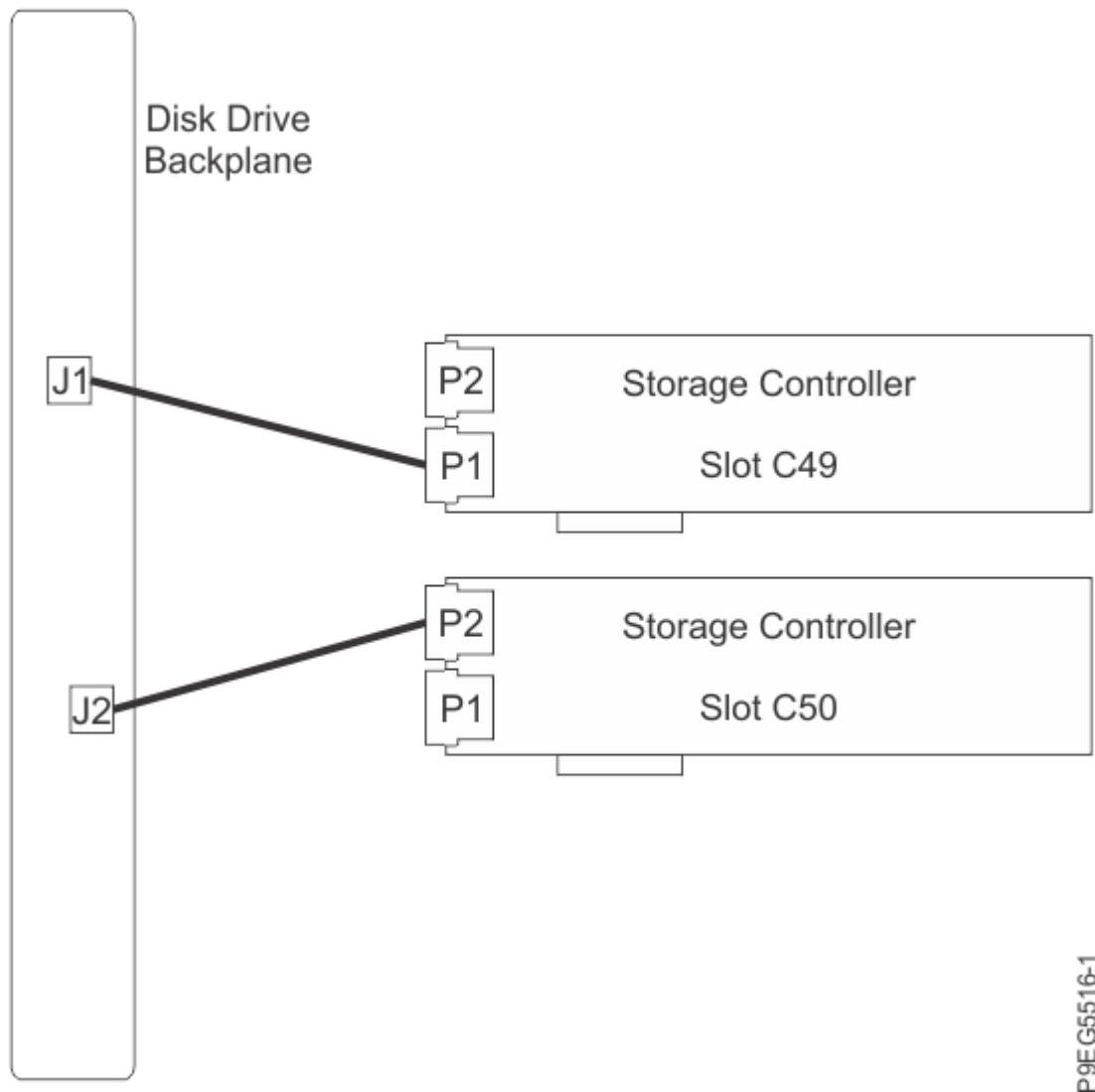
รูปที่ 6. การเชื่อมต่อสาย SAS อีกครั้งในคอนฟิกรูเรชัน ดิสก์แบบแยก
