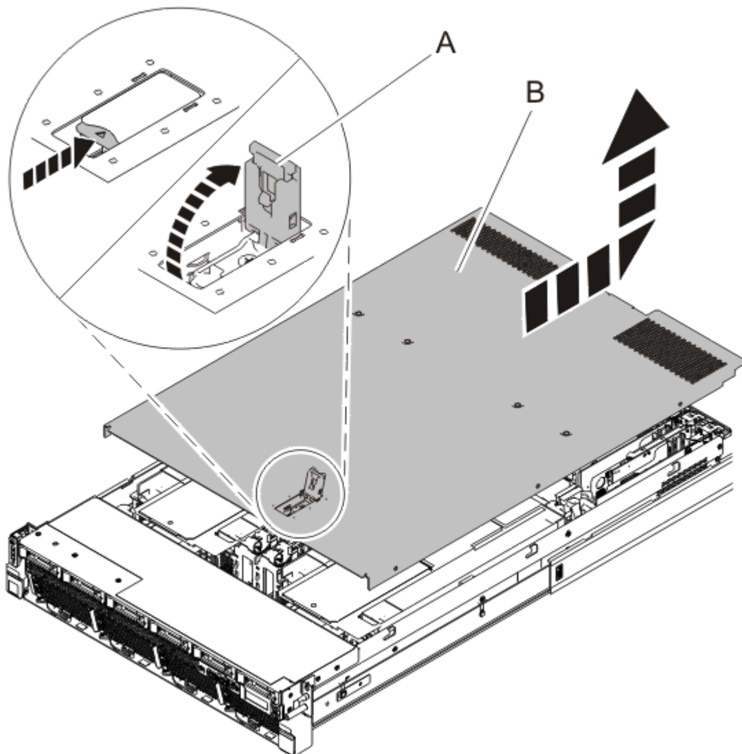
รูปที่ 18. การถอดฝาครอบการเข้าถึงเซอรัวิส
