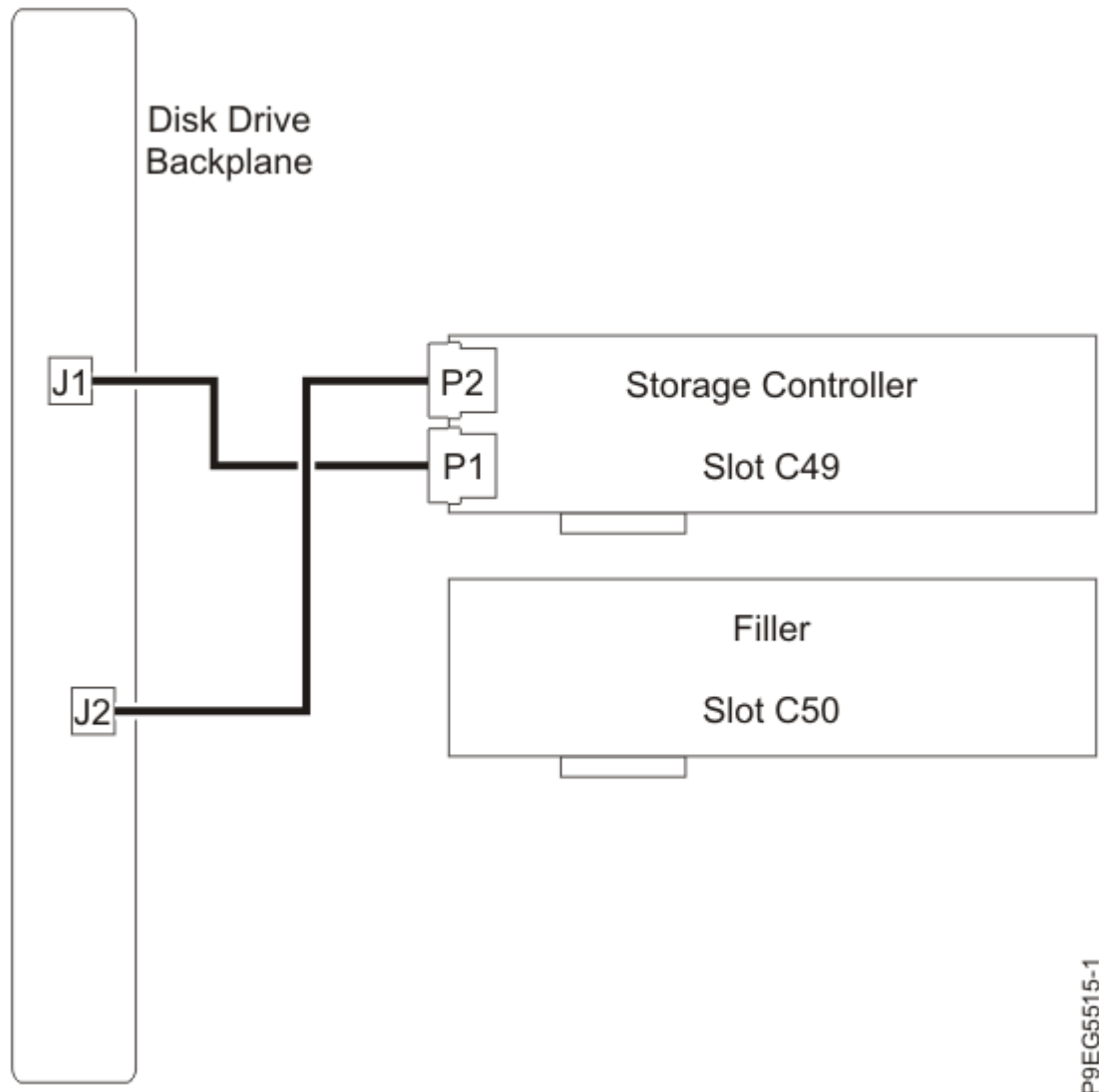
รูปที่ 24. การเชื่อมต่อสาย SAS อีกครั้งในคอนฟิกรูชัน หน่วยเก็บข้อมูลฐาน
