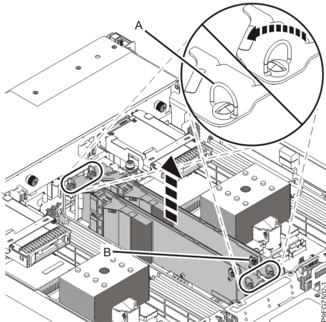
รูปที่ 22. การถอดอะแดปเตอร์ SAS RAID
