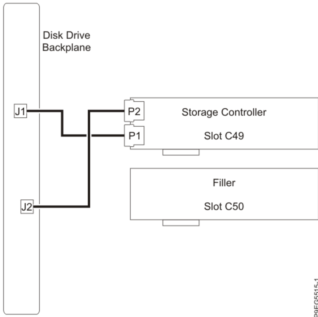
รูปที่ 5. การเชื่อมต่อสาย SAS อีกครั้งในคอนฟิกรูชัน หน่วยเก็บข้อมูลฐาน
