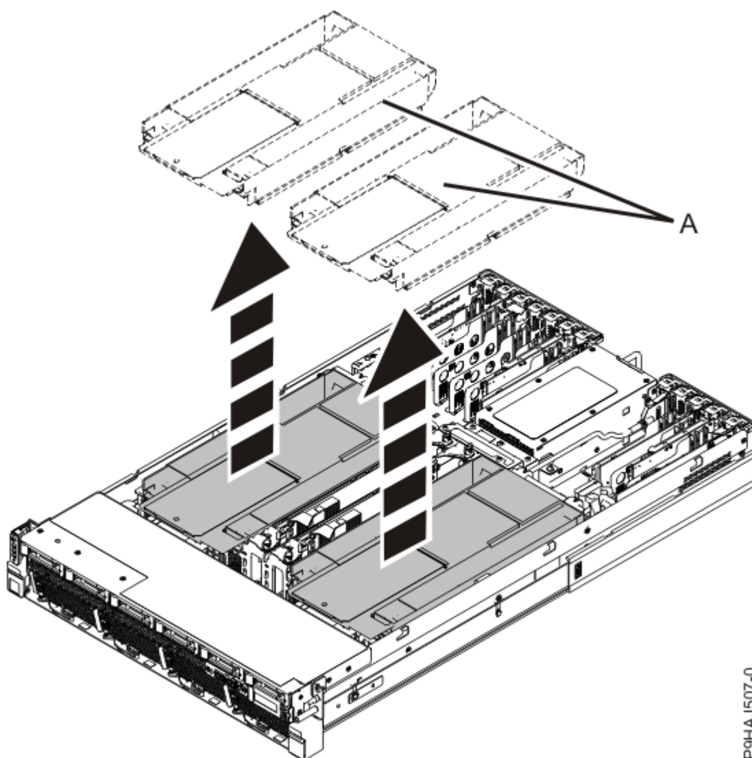
รูปที่ 19. การถอดตัวไหลเวียนอากาศ
