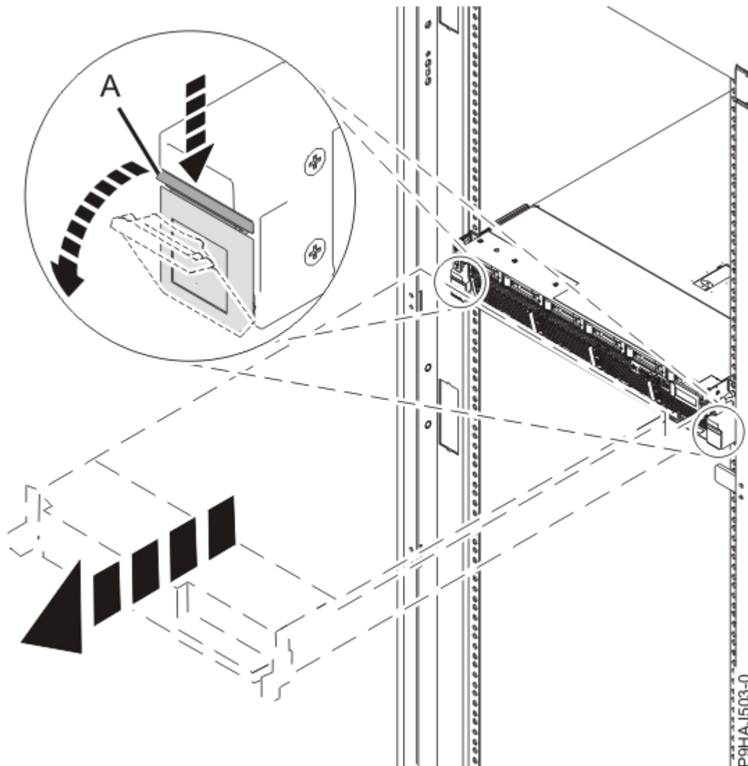
รูปที่ 17. การปลดแลตซ์ด้านข้าง
