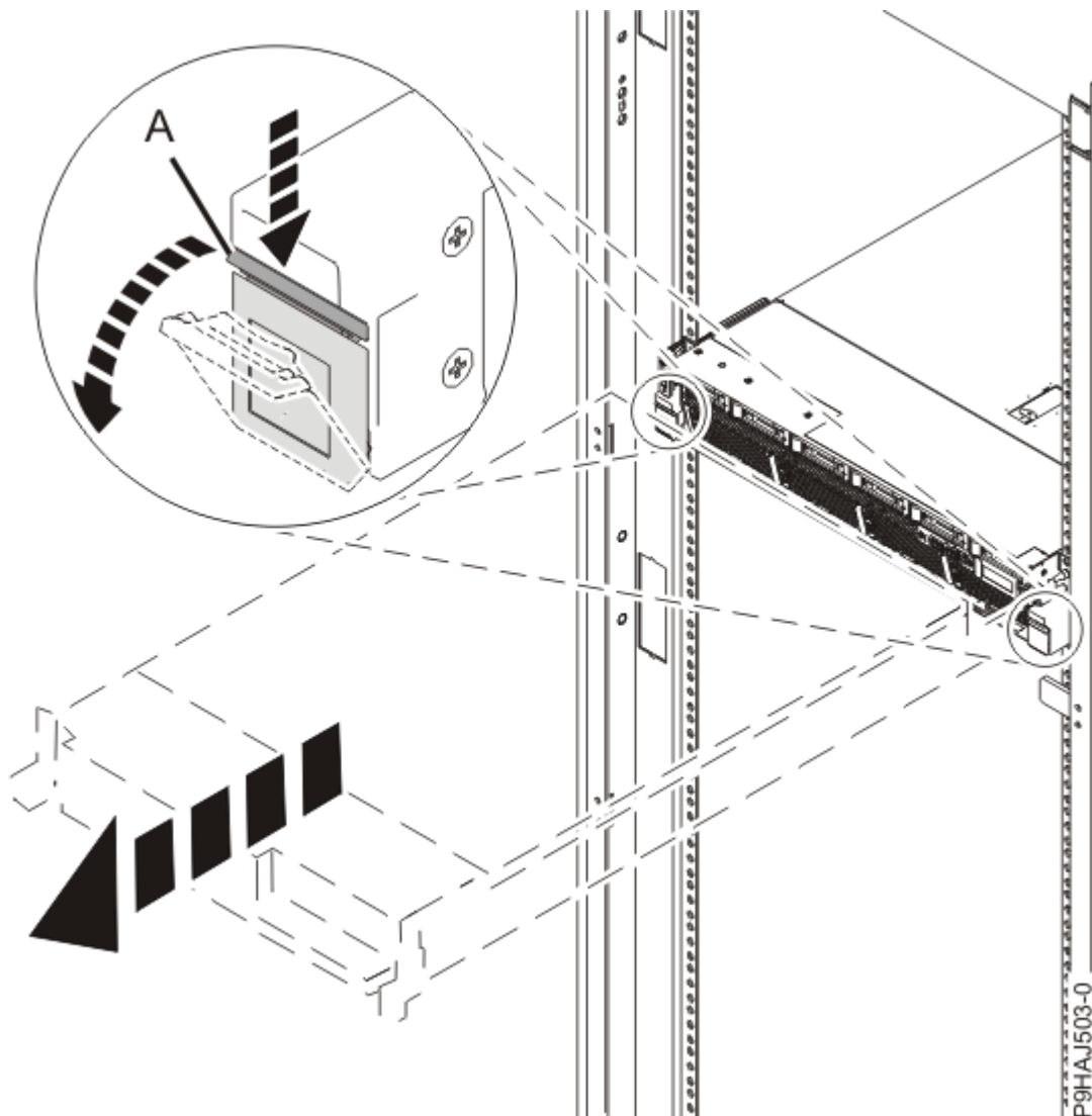
รูปที่ 2. การปลดแลตซ์ด้านข้าง
