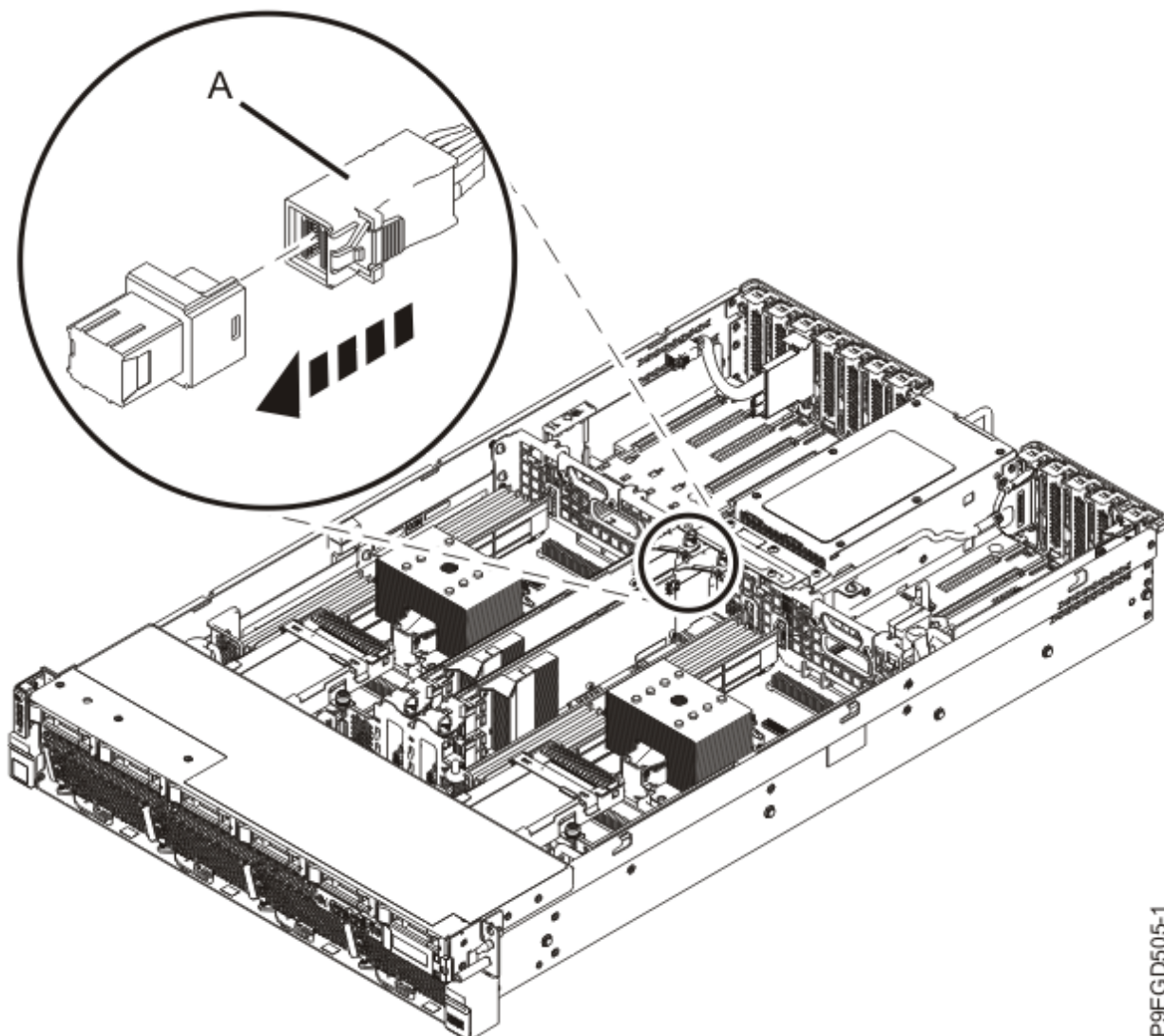
รูปที่ 9. การเชื่อมต่อสายเคเบิล SAS ด้านหลัง
