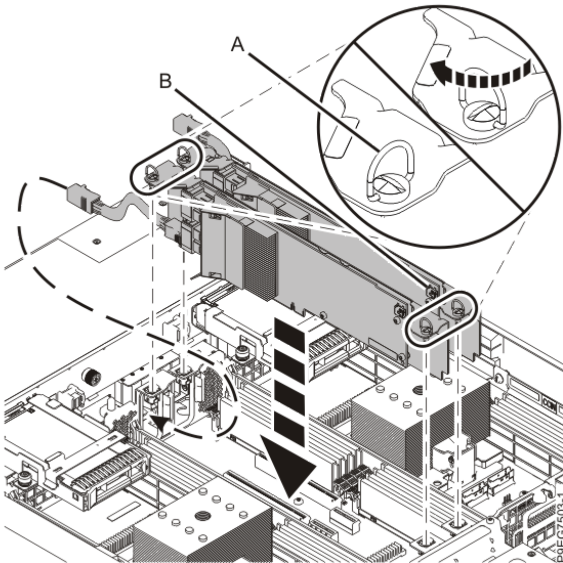
รูปที่ 27. การเปลี่ยนอะแดปเตอร์ SAS RAID
