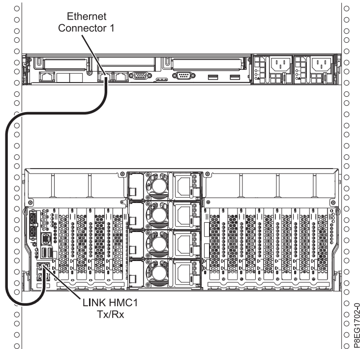
รูปที่ 12. การต่อพ่วง HMC กับระบบที่ถูกจัดการ
