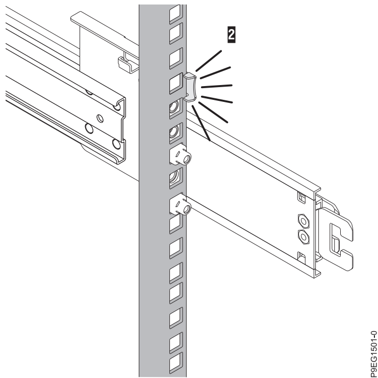
รูปที่ 3. การดันรางลงในหน้าแปลนของชั้นวางด้านหลังจนกว่าจะเข้าตำแหน่ง
