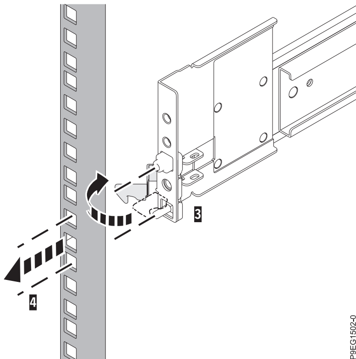
รูปที่ 4. การหมุนตัวยึดและการจัดแนวหมุด
