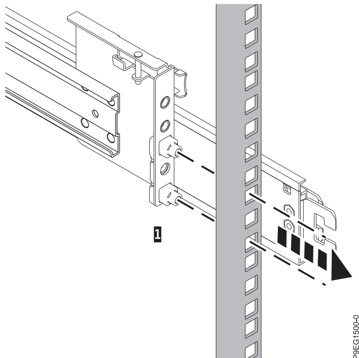
รูปที่ 2. การจัดแนวท้ายรางด้านซ้ายเข้ากับด้านหลังของชั้นวาง
