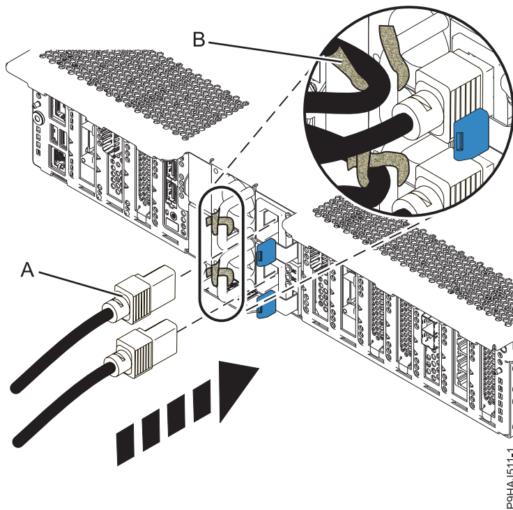
รูปที่ 21. การเชื่อมต่อสายไฟ
