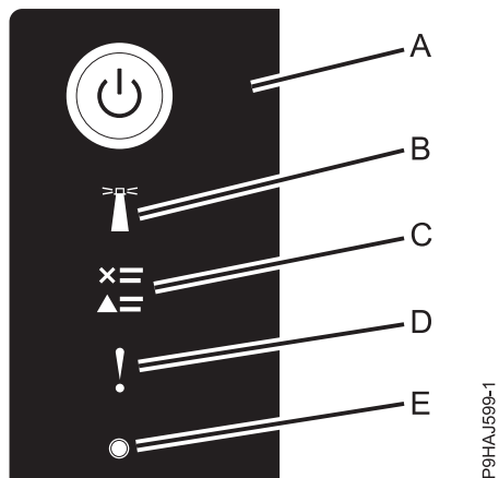
รูปที่ 9. คอนโทรลพาเนล LEDs
