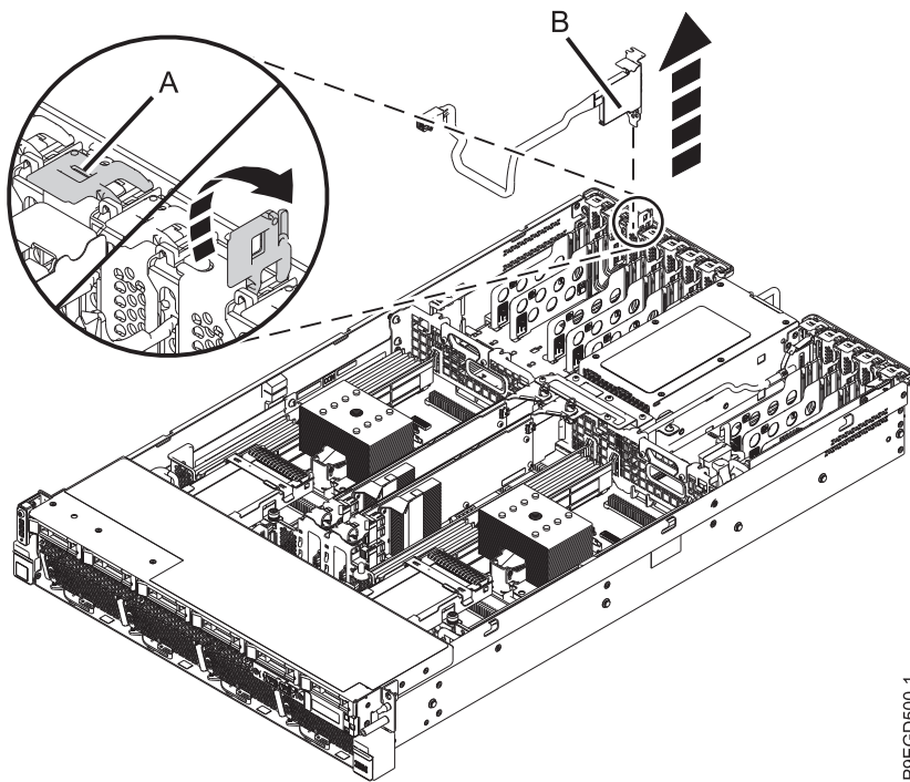
รูปที่ 4. การถอดอะแดปเตอร์สายเคเบิล SAS ด้านหลัง
