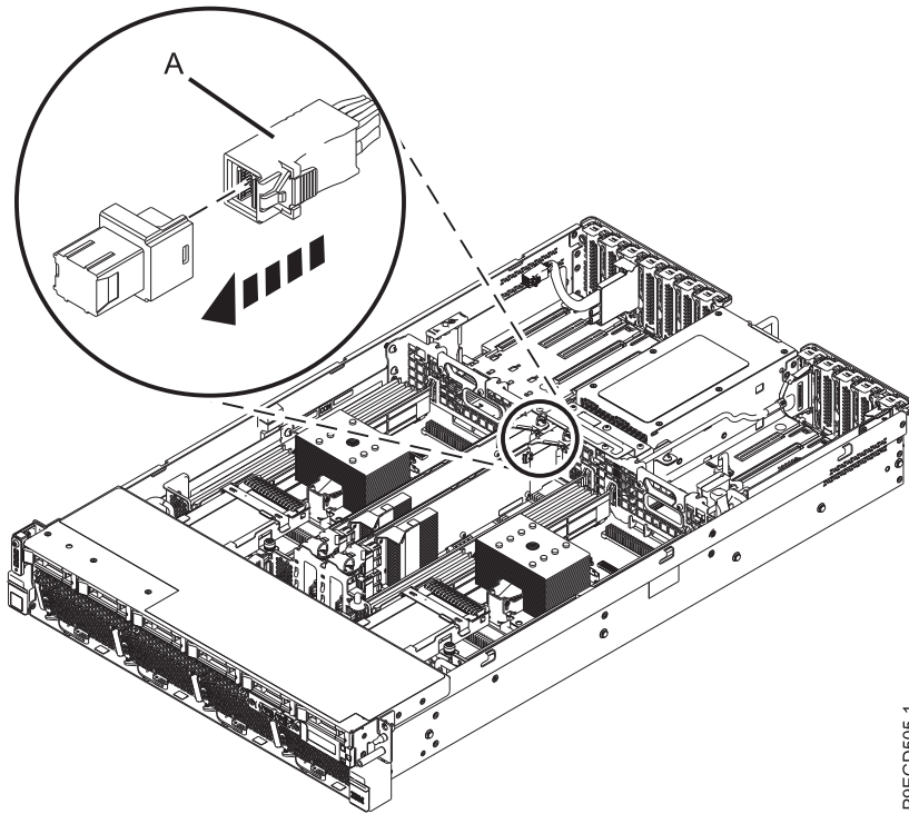
รูปที่ 7. การติดตั้งสายเคเบิล SAS ด้านหลัง
