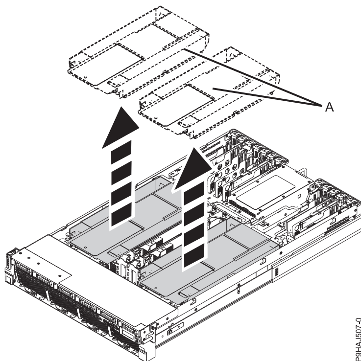
รูปที่ 16. การถอดตัวไหลเวียนอากาศ
