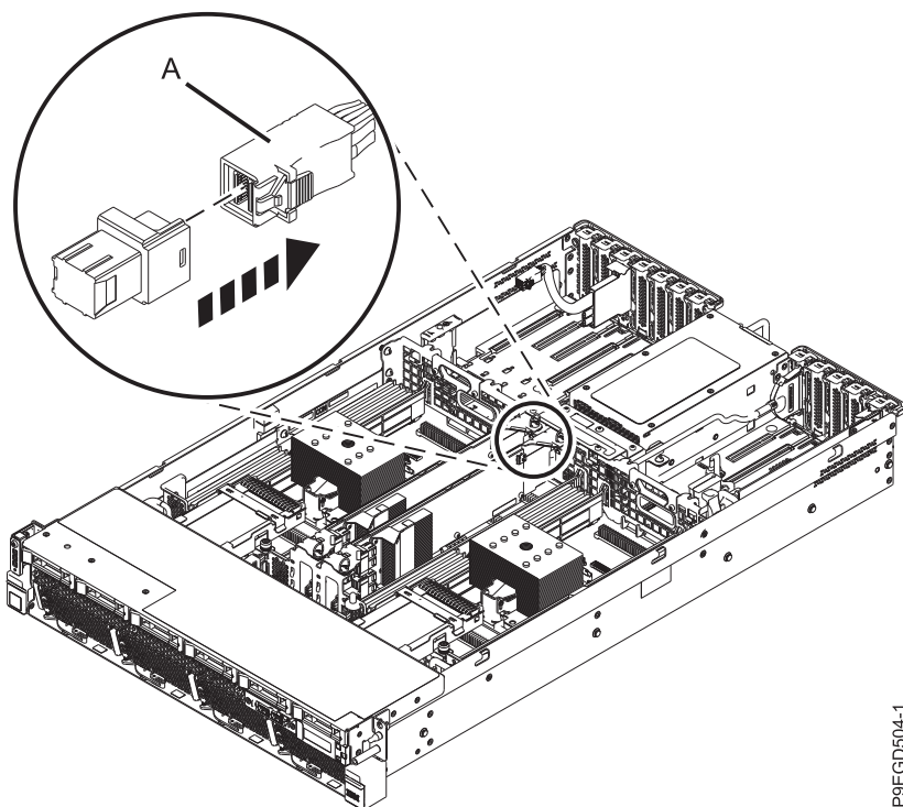
รูปที่ 3. การถอดสายเคเบิล SAS ด้านหลังออกจากอะแดปเตอร์ภายใน SAS RAID
