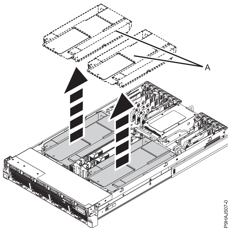
รูปที่ 2. การถอดตัวโหลเวียนอากาศ
