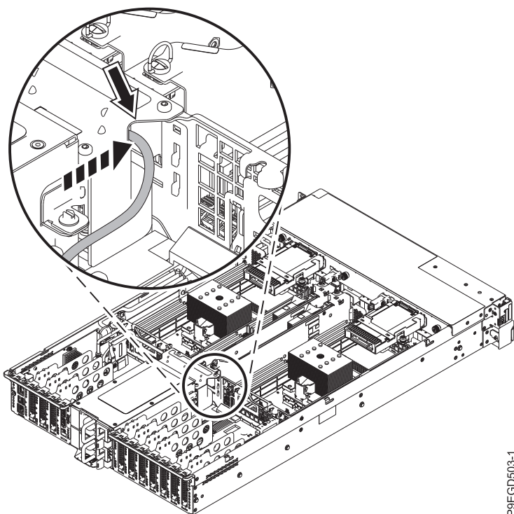
รูปที่ 6. การจัดเส้นทางสายเคเบิล SAS ด้านหลัง
