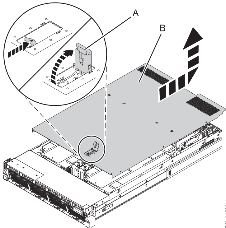
รูปที่ 14. การถอดฝาครอบการเข้าถึงเซอร์วิส
