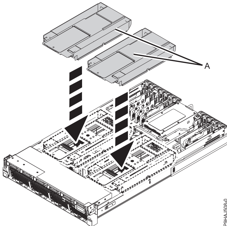
รูปที่ 17. การเปลี่ยนตัวไหลเวียนอากาศ
