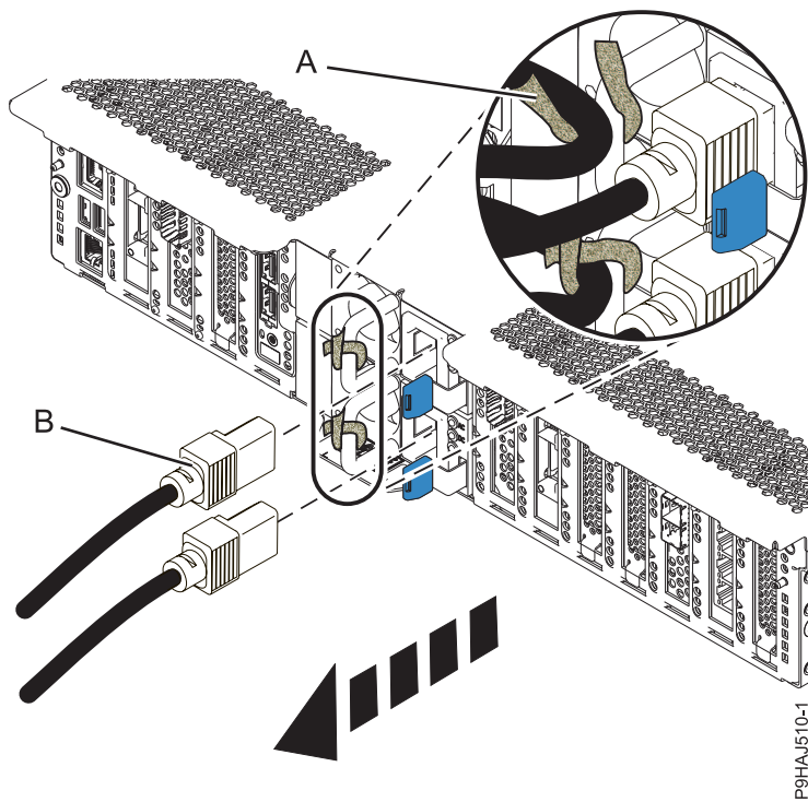
รูปที่ 20. การถอดสายไฟ
