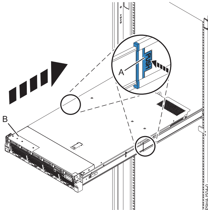
รูปที่ 19. การจัดตำแหน่งระบบในตำแหน่งการทำงาน
