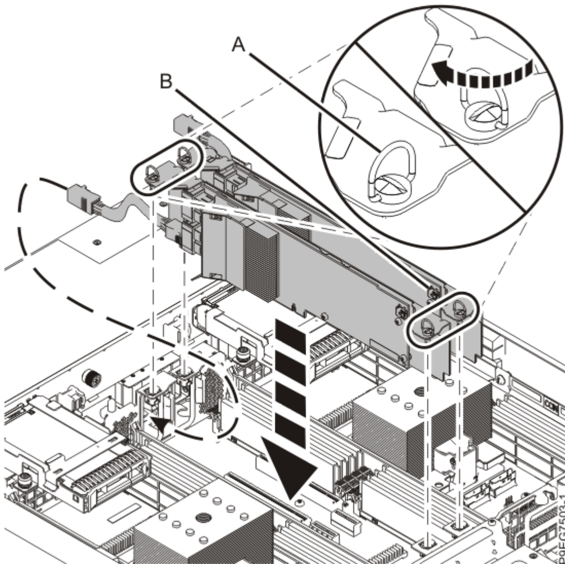
รูปที่ 12. การเปลี่ยนอะแดปเตอร์ SAS RAID
