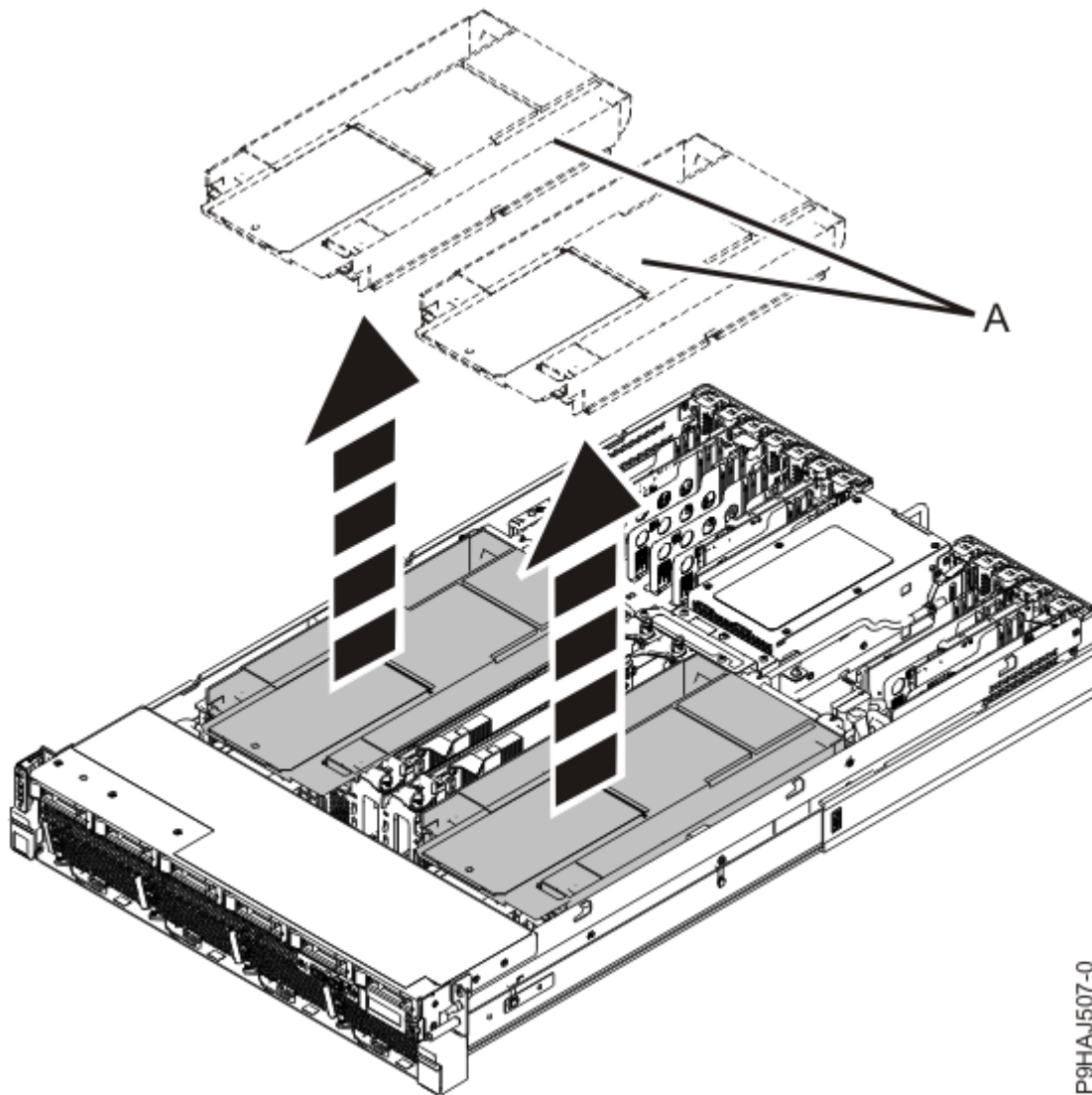
รูปที่ 5. การถอดตัวโหลเวียนอากาศ
