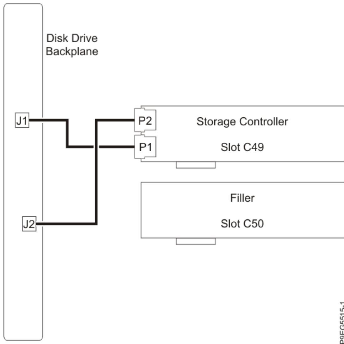
รูปที่ 9. การเชื่อมต่อสาย SAS อีกครั้งในคอนฟิเกอเรชัน หน่วยเก็บข้อมูลฐาน
