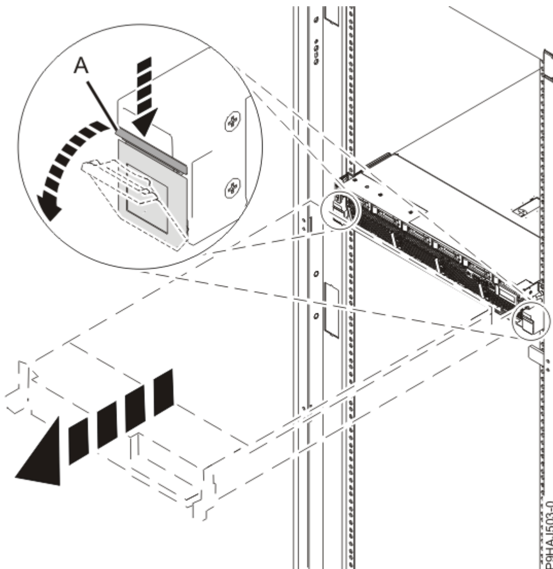
รูปที่ 2. การปลดแลตซ์ด้านข้าง
