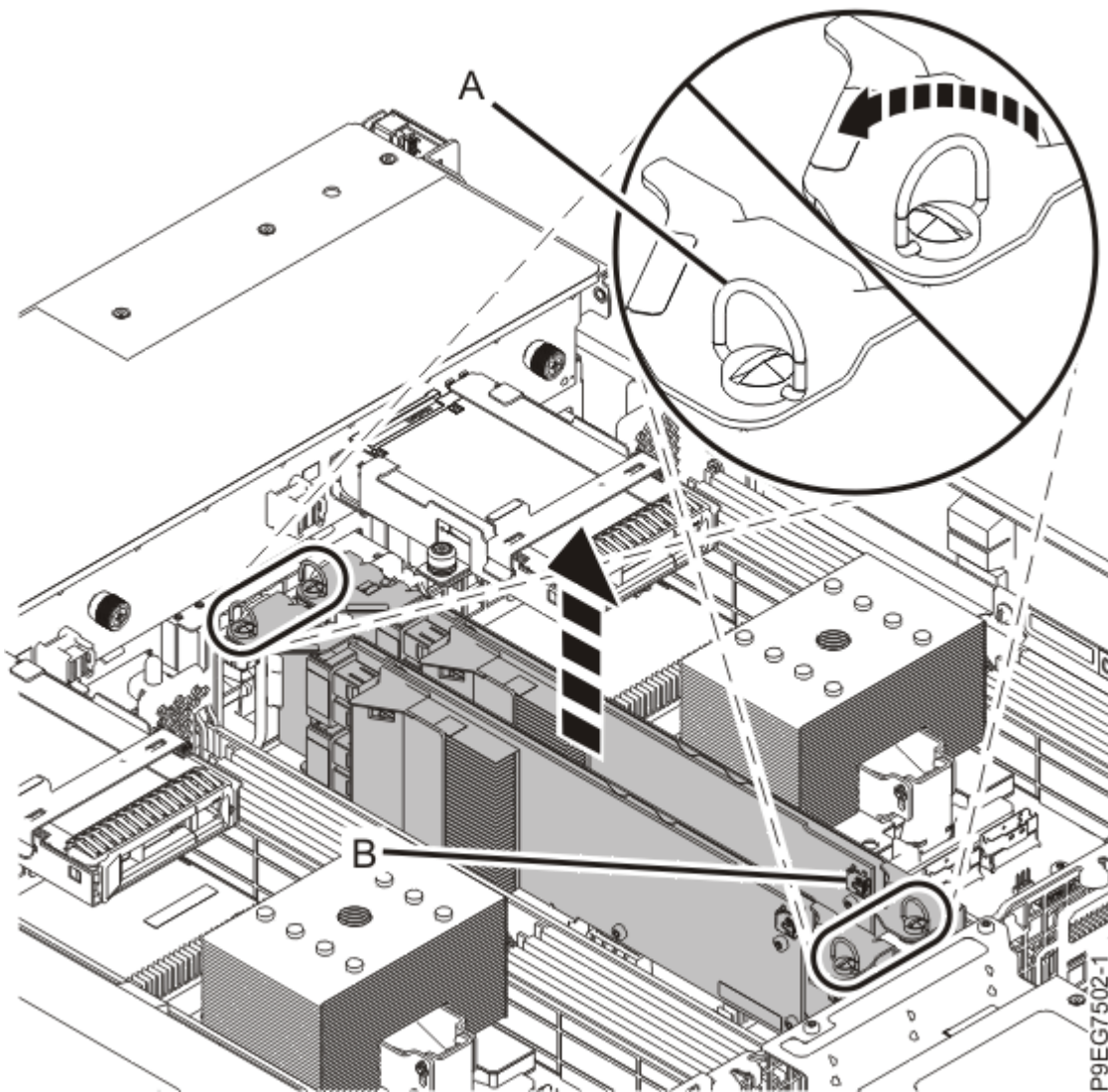
รูปที่ 7. การถอดอะแดปเตอร์ SAS RAID
