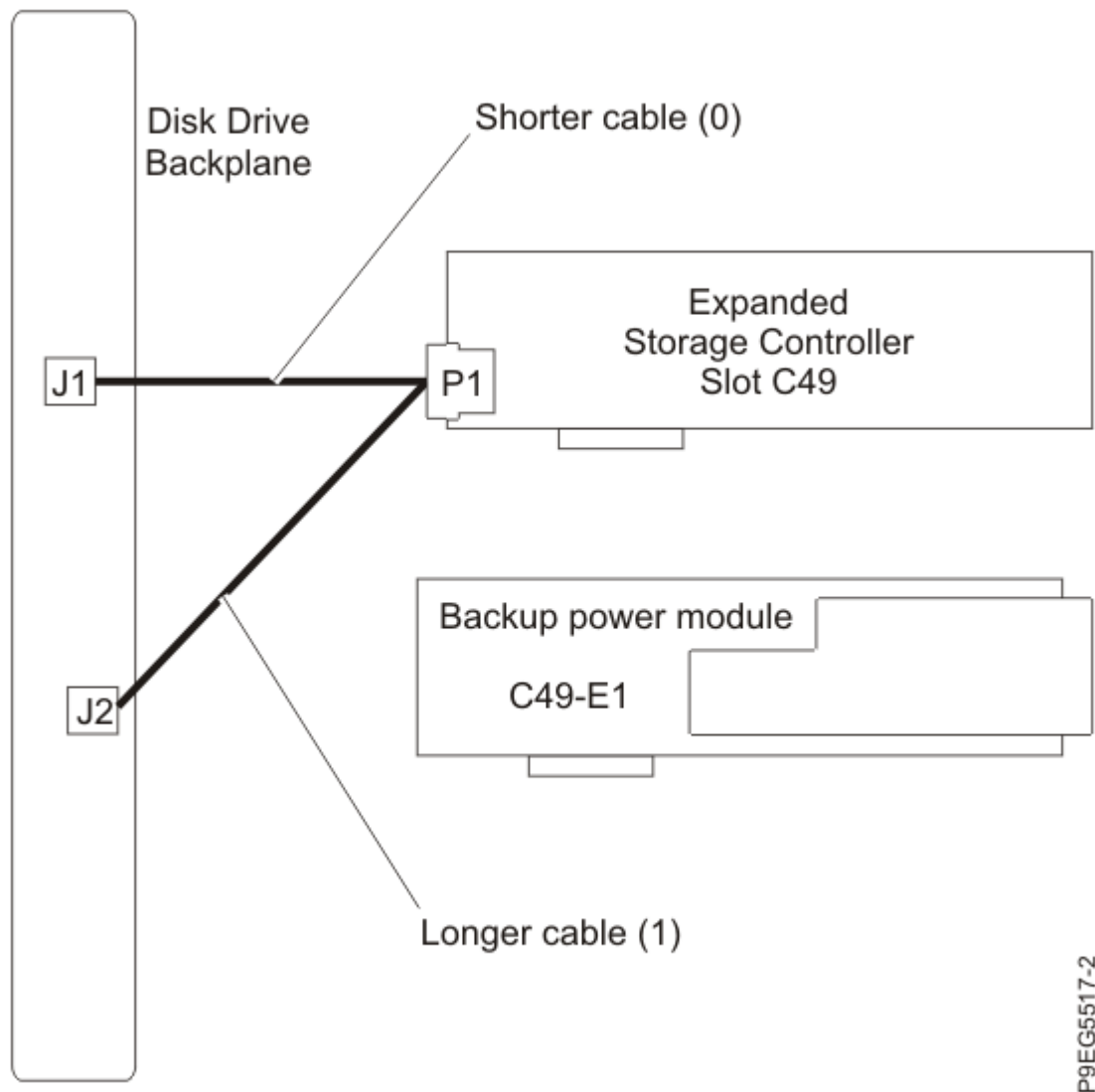
รูปที่ 11. การเชื่อมต่อสาย SAS แบบ "Y" ในคอนฟิกรูเรชันคอนโทรลเลอร์หน่วยเก็บข้อมูลประสิทธิภาพสูง
