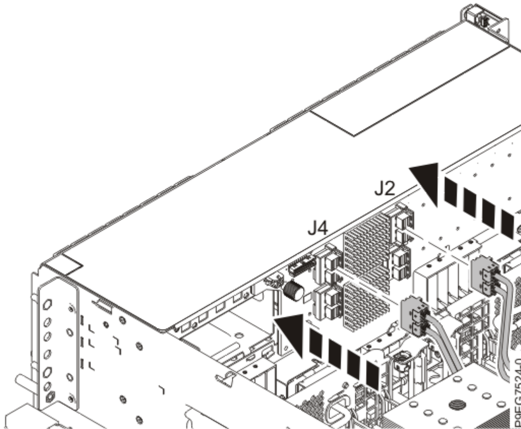
รูปที่ 12. การเสียบสายเคเบิล SAS ด้านหน้าสำหรับดิสก์ไดรฟ์ 12-drive expanded function or 18-drive expanded function ด้านหลัง
