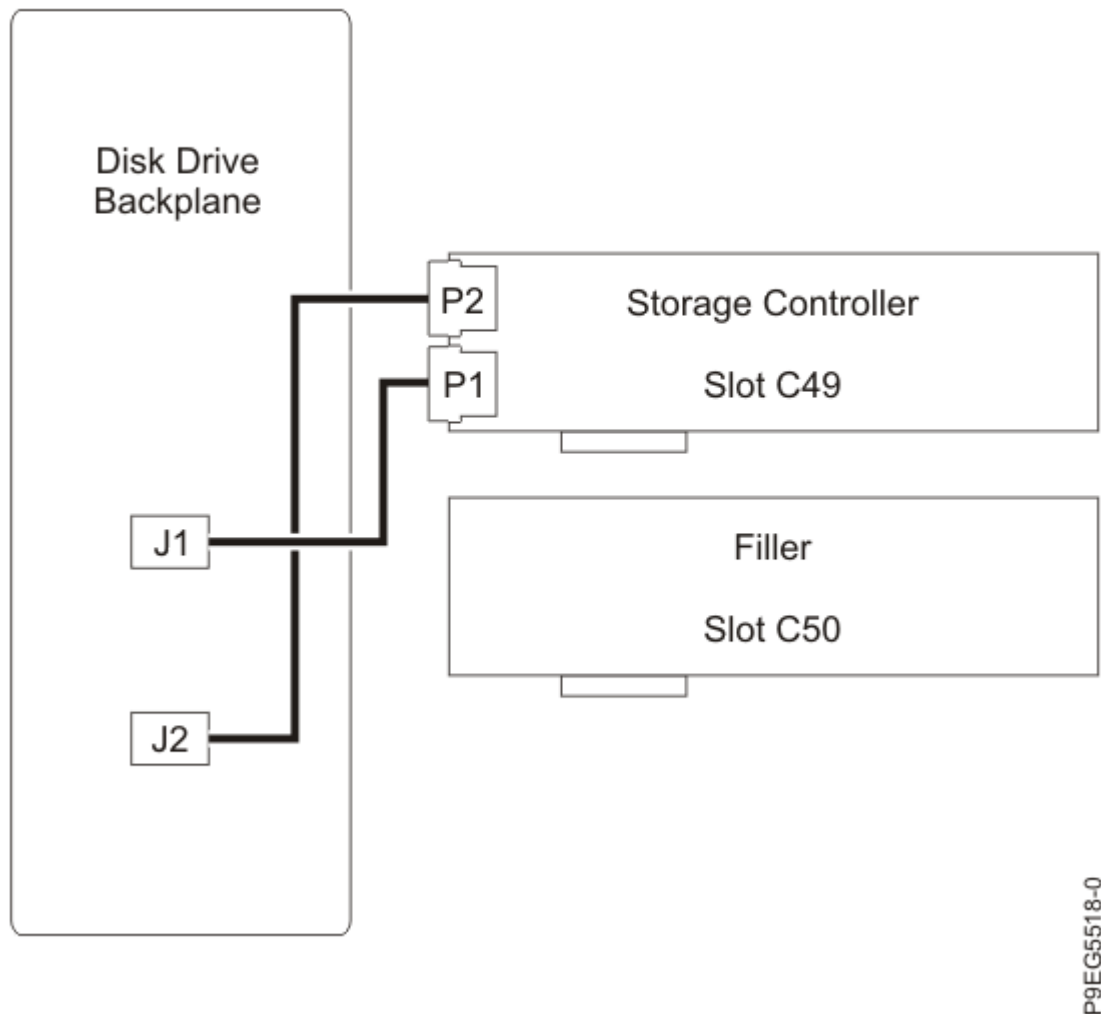
รูปที่ 13. การเชื่อมต่อสาย SAS อีกครั้งในคอนฟิเกอเรชัน หน่วยเก็บข้อมูลฐาน
