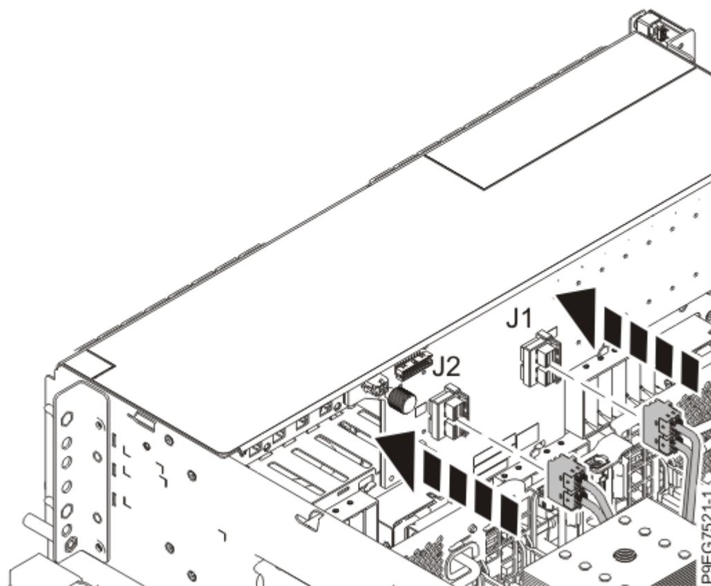
รูปที่ 11. การเสียบสายเคเบิล SAS ด้านหน้าใหม่อีกครั้งสำหรับดิสก์ไดรฟ์ base function ด้านหลัง
