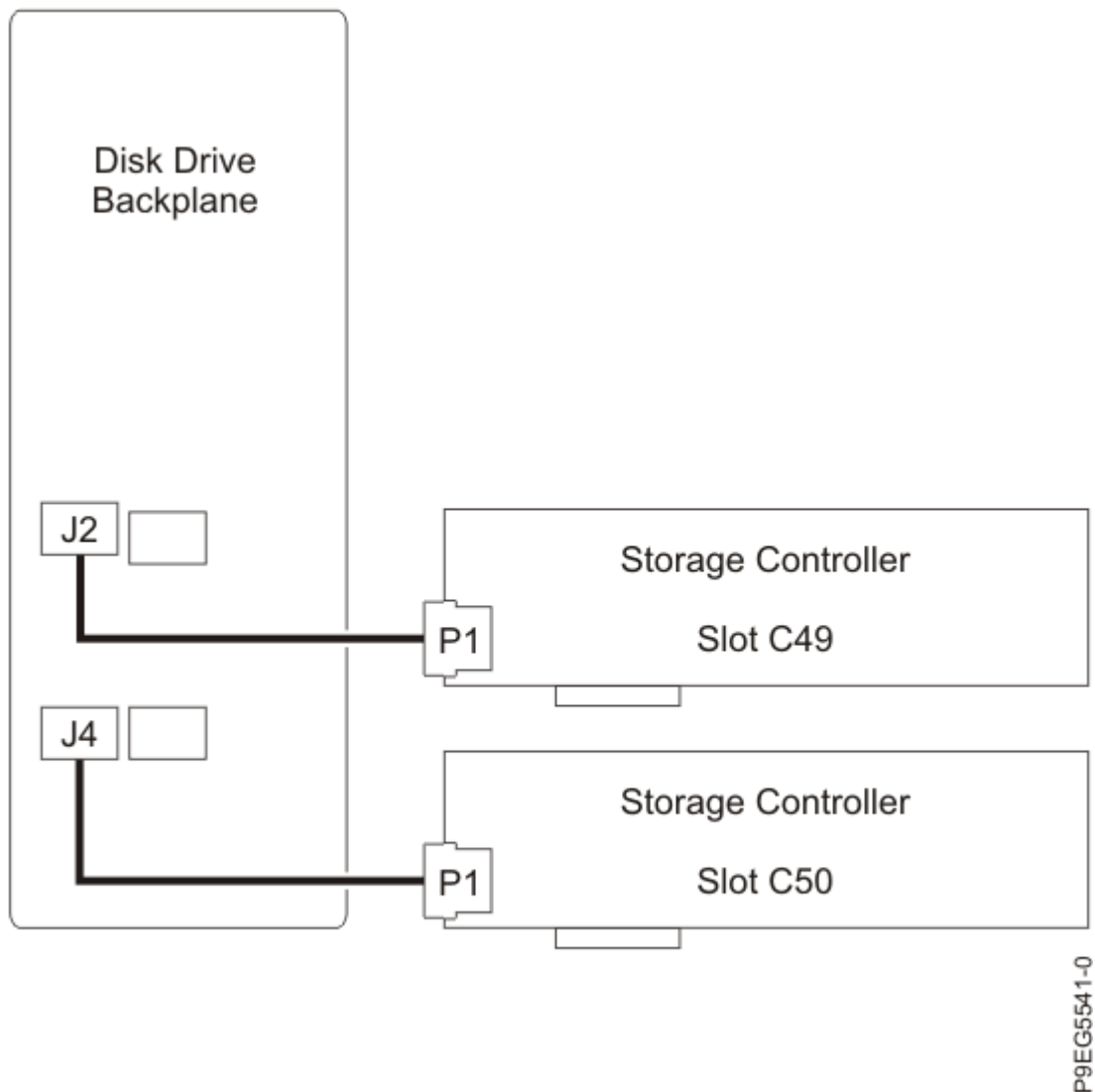
รูปที่ 15. การเชื่อมต่อสายเคเบิล SAS อีกครั้งในการกำหนดคอนฟิก 12-drive expanded function
