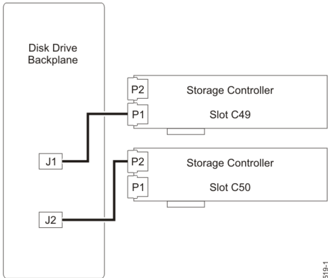
รูปที่ 14. การเชื่อมต่อสาย SAS อีกครั้งในคอนฟิกรูเรชัน ดิสก์แบบแยก
