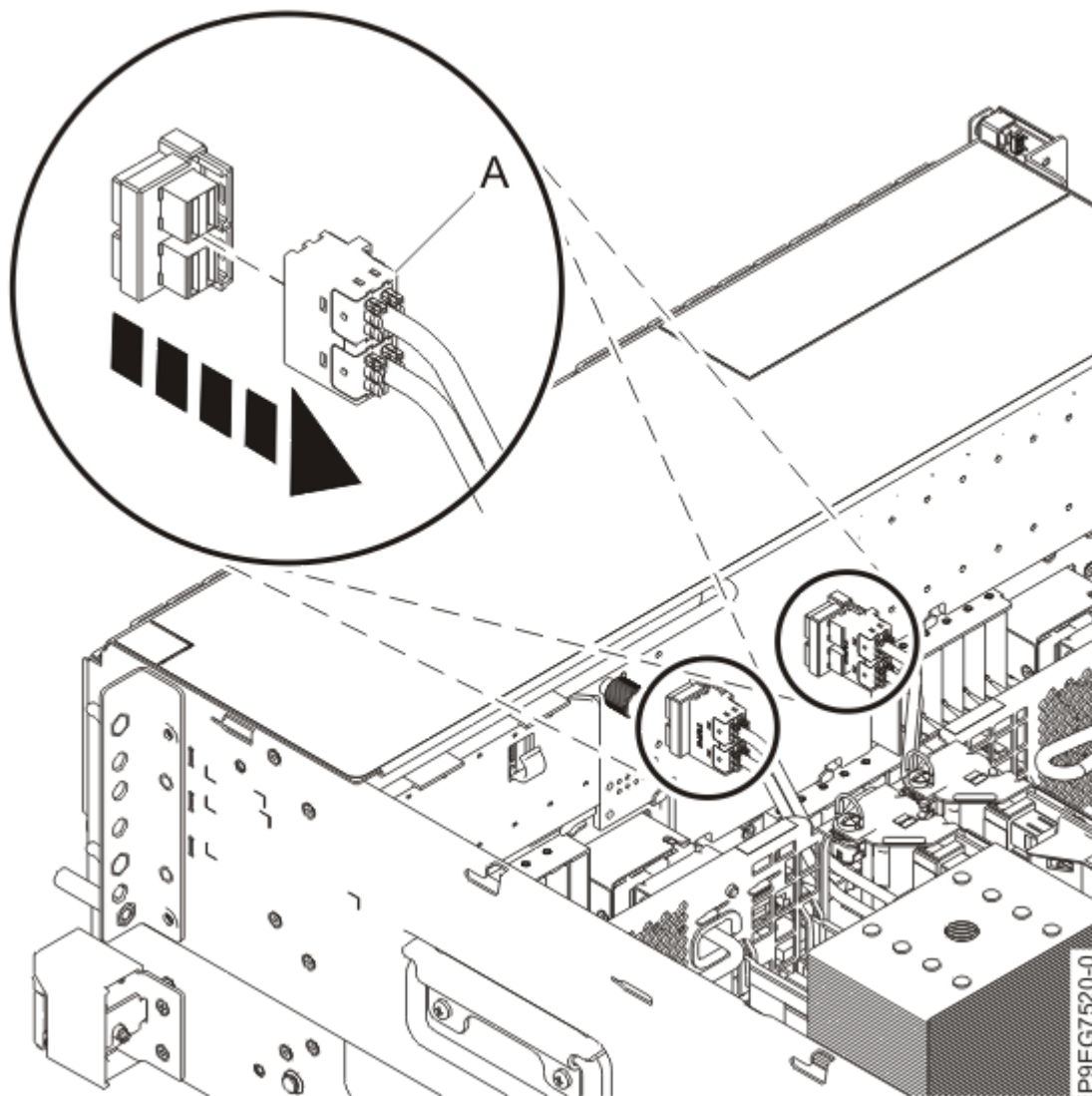
รูปที่ 9. การถอดสายเคเบิล SAS
