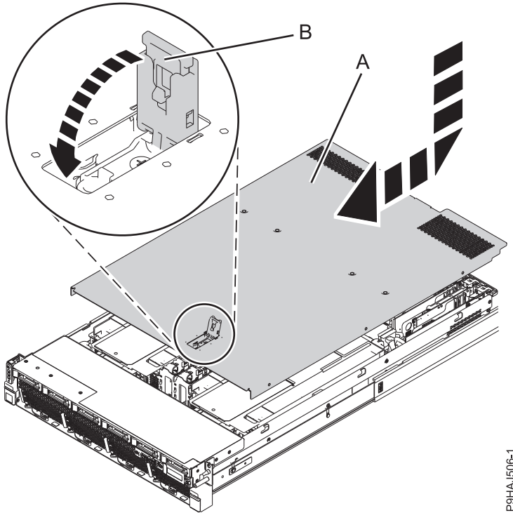
รูปที่ 36. การติดตั้ง ฝาครอบการเข้าถึงเซอร์วิส
