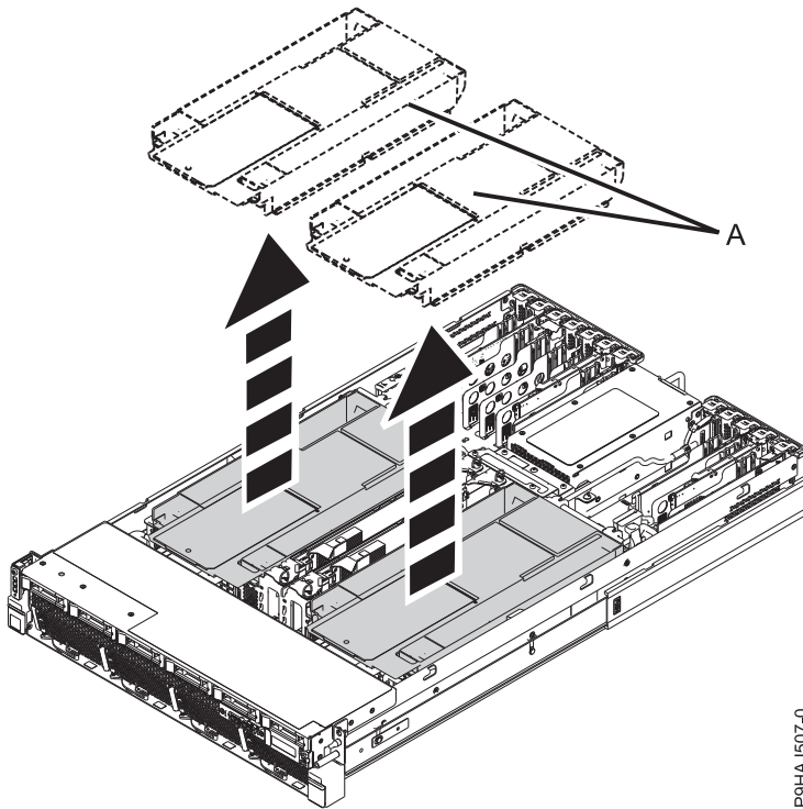
รูปที่ 2. การถอด ตัวไหลเวียนอากาศ
