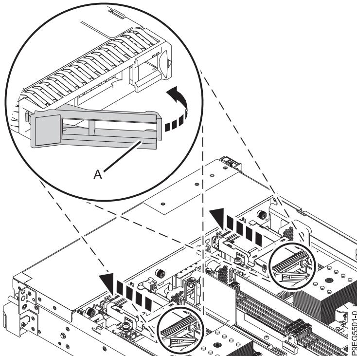
รูปที่ 20. การลือกไดร์ฟ
