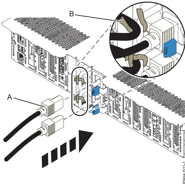
รูปที่ 42. การเชื่อมต่อสายไฟ
