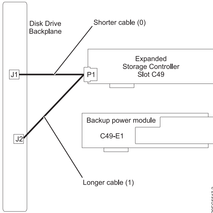
รูปที่ 16. การเชื่อมต่อสาย SAS แบบ “Y” ในคอนฟิกร์ชันคอนโทรลเลอร์หน่วยเก็บข้อมูล ประสิทธิภาพสูง
