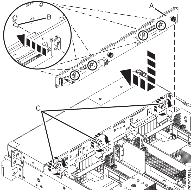
รูปที่ 11. การเปลี่ยนเบ็กเพลนของดิสก์ไดรฟ์
