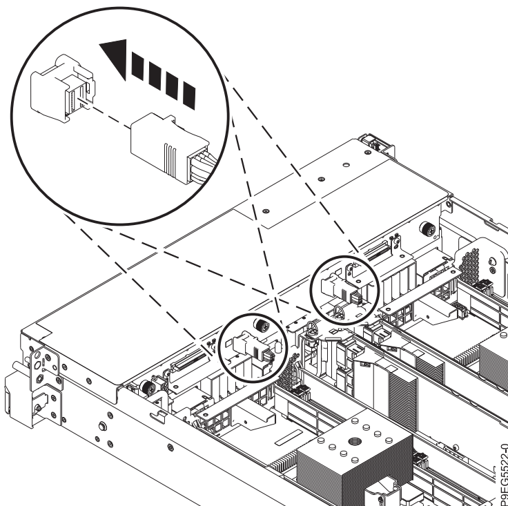
รูปที่ 13. การเชื่อมต่อสาย SAS ด้านหน้าอีกครั้ง
