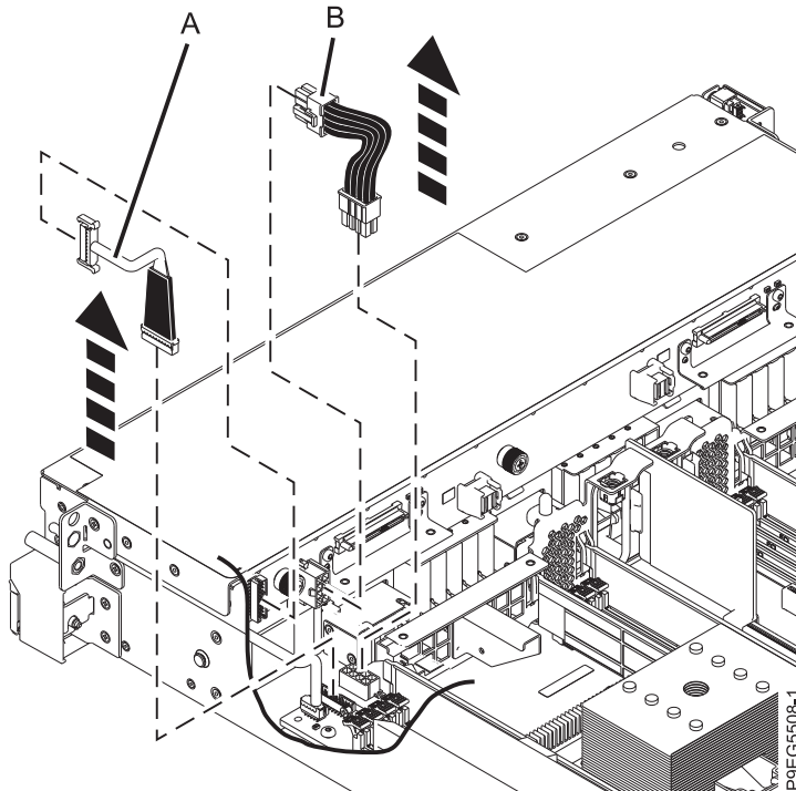
รูปที่ 9. การถอดสายสัญญาณและสายไฟ
