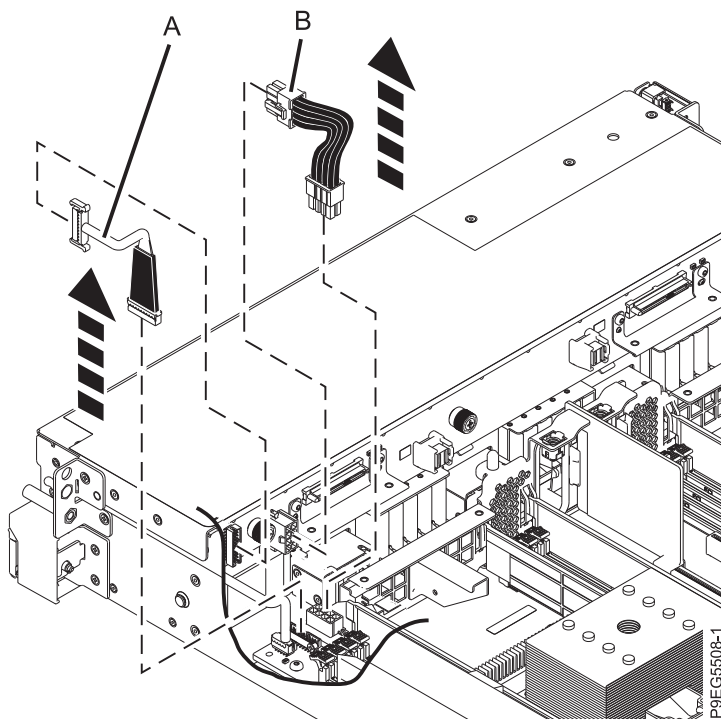
รูปที่ 24. การถอดสายสัญญาณและสายไฟ
