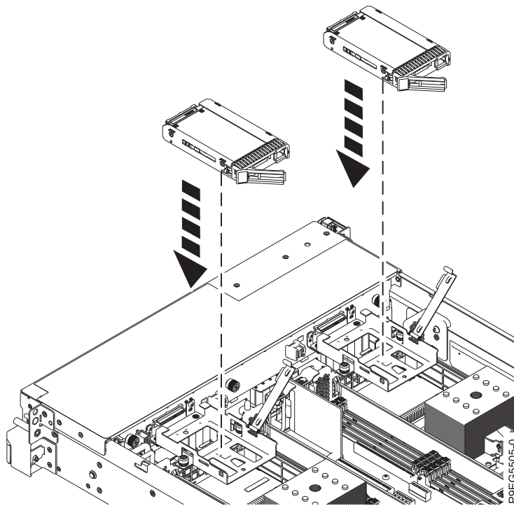
รูปที่ 19. การวางไดรฟ์ลงในถาดสำหรับไดรฟ์
