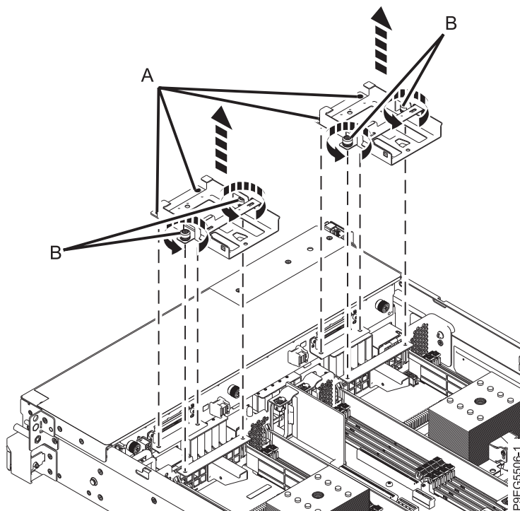
รูปที่ 6. การถอดถาดสำหรับไดรฟ์
