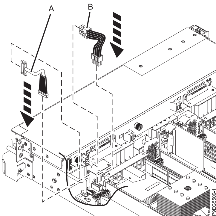
รูปที่ 12. การเชื่อมต่อสายสัญญาณและสายไฟ
