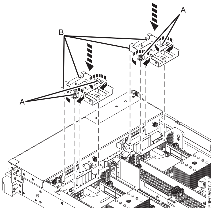
รูปที่ 18. การเปลี่ยนถาดสำหรับไดรฟ์
