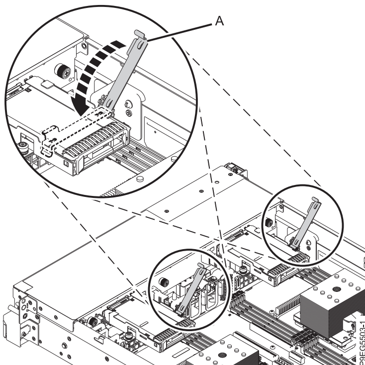
รูปที่ 21. การปิดที่ยึดไดร์ฟ
