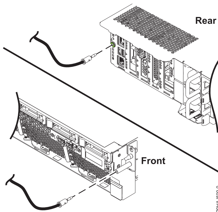
รูปที่ 1. ตำแหน่งของปลั๊ก ESD
