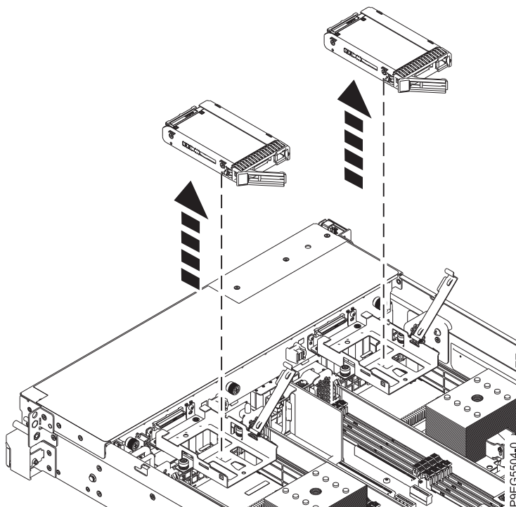
รูปที่ 5. การยกไดรฟ์
