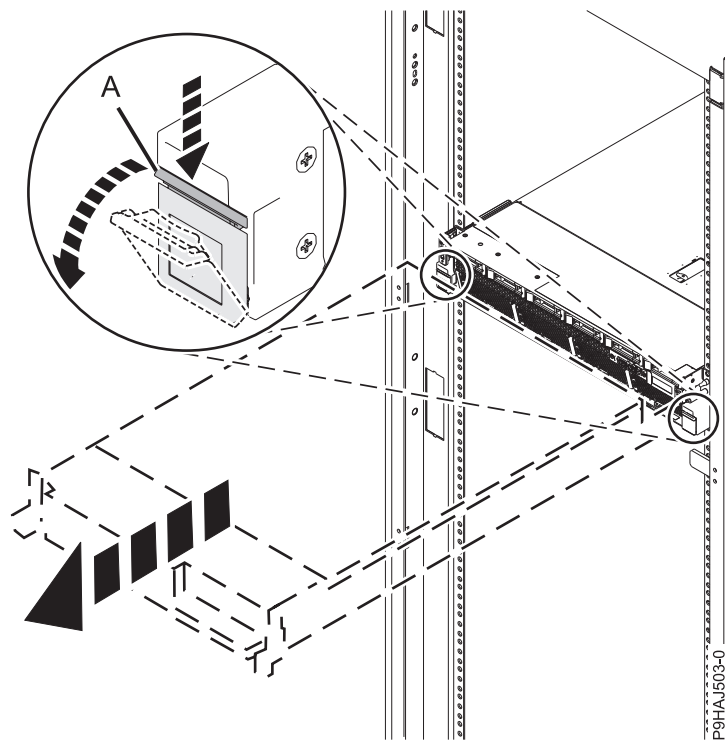
รูปที่ 39. การปลดแลตซ์ด้านข้าง
