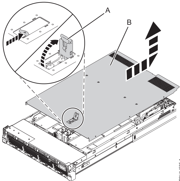
รูปที่ 35. การถอดฝาครอบการเข้าถึงเซิร์ฟเวอร์
