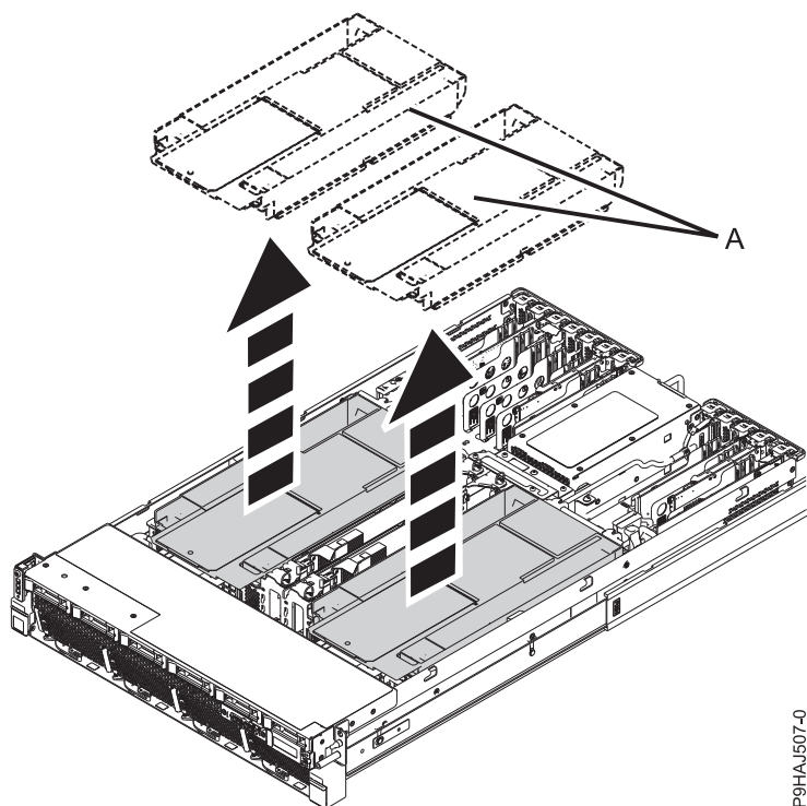
รูปที่ 23. การถอดตัวโหลเวียนอากาศ
