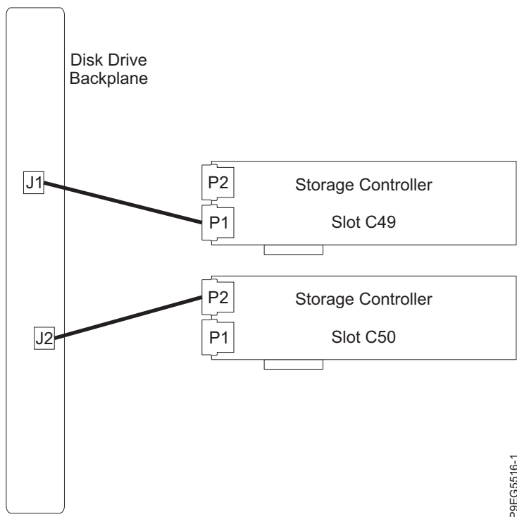
รูปที่ 15. การเชื่อมต่อสาย SAS อีกครั้งในคอนฟิกรูระดับดิสก์แบบแยก
