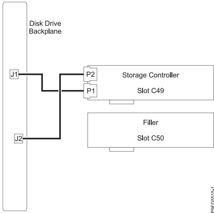
รูปที่ 14. การเชื่อมต่อสาย SAS อีกครั้งในคอนฟิกรेशनหน่วยเก็บข้อมูลฐาน
