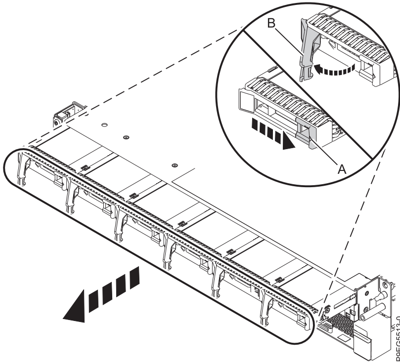
รูปที่ 7. การถอดไดรฟ์ด้านหน้าบางส่วน
