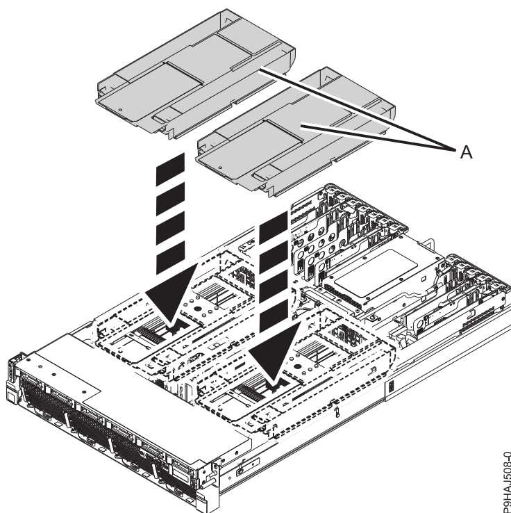
รูปที่ 38. การเปลี่ยนตัวไหลเวียนอากาศ
