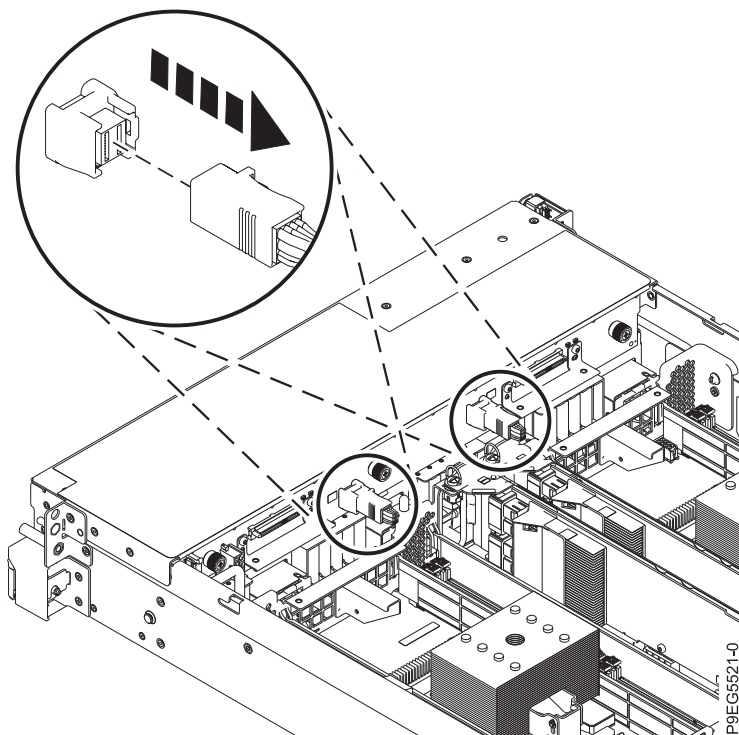
รูปที่ 8. การปลดสาย SAS ด้านหน้า
