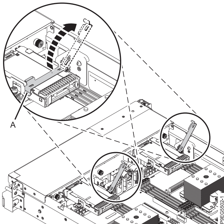
รูปที่ 3. การเปิดที่ยึดไดรฟ์
