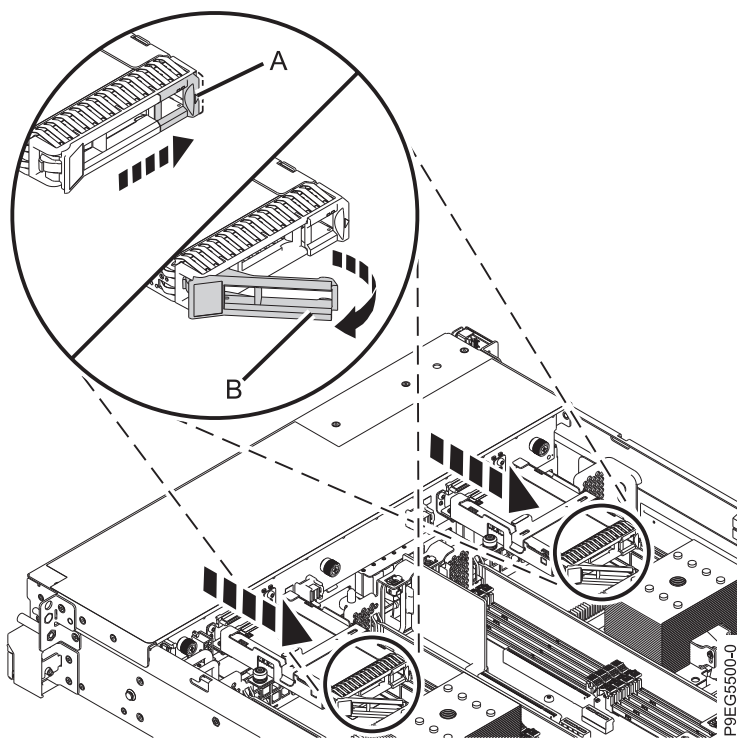
รูปที่ 4. การปลดแลตซ์
