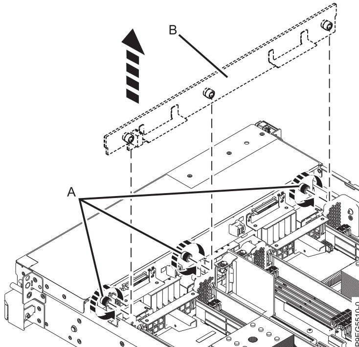
รูปที่ 10. การคลายสกรูแบ็กเพลนดิสก์ไดรฟ์
