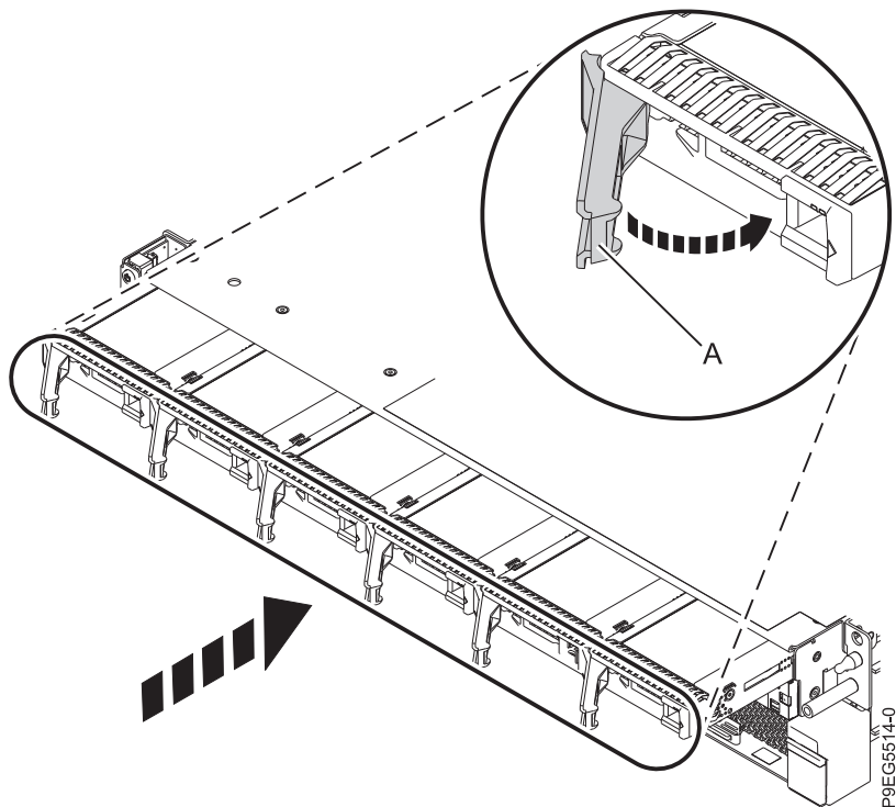
รูปที่ 17. การเปลี่ยนไดรฟ์ด้านหน้า
