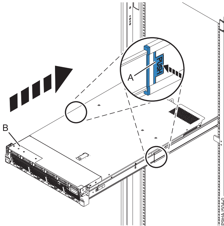
รูปที่ 40. การจัดตำแหน่งระบบในตำแหน่งการทำงาน
