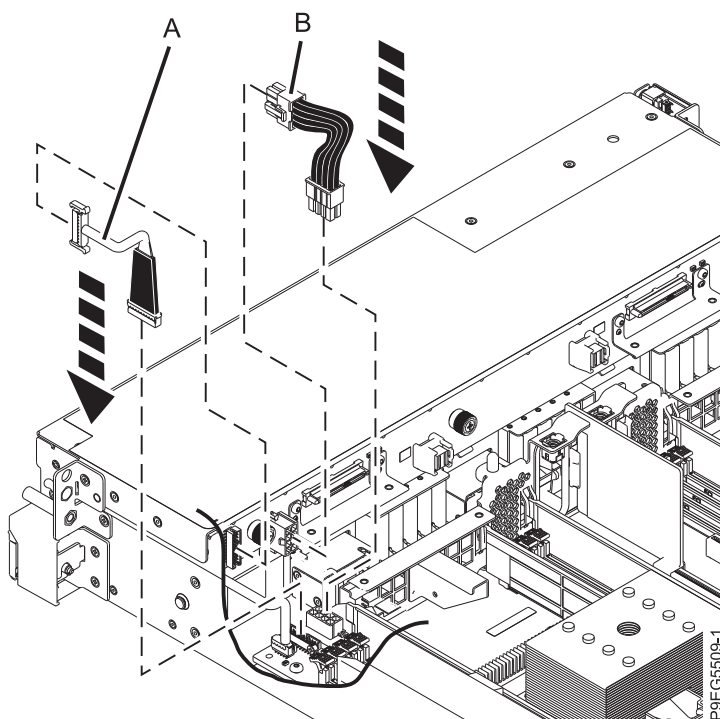
รูปที่ 25. การเชื่อมต่อสายสัญญาณและสายไฟ
