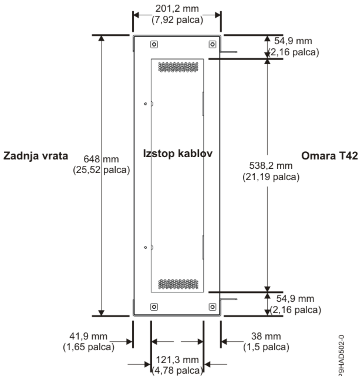
Slika 5. Razširitev zadnjega dela omare, koda možnosti FC ERG0 (pogled od zgoraj navzdol)
