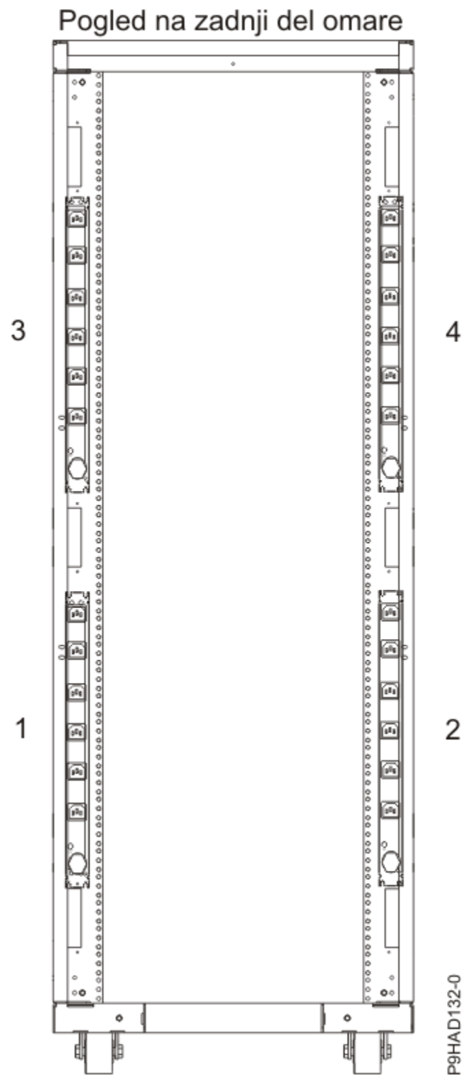
Slika 50. Navpični položaji napajalnih distribucijskih enot
