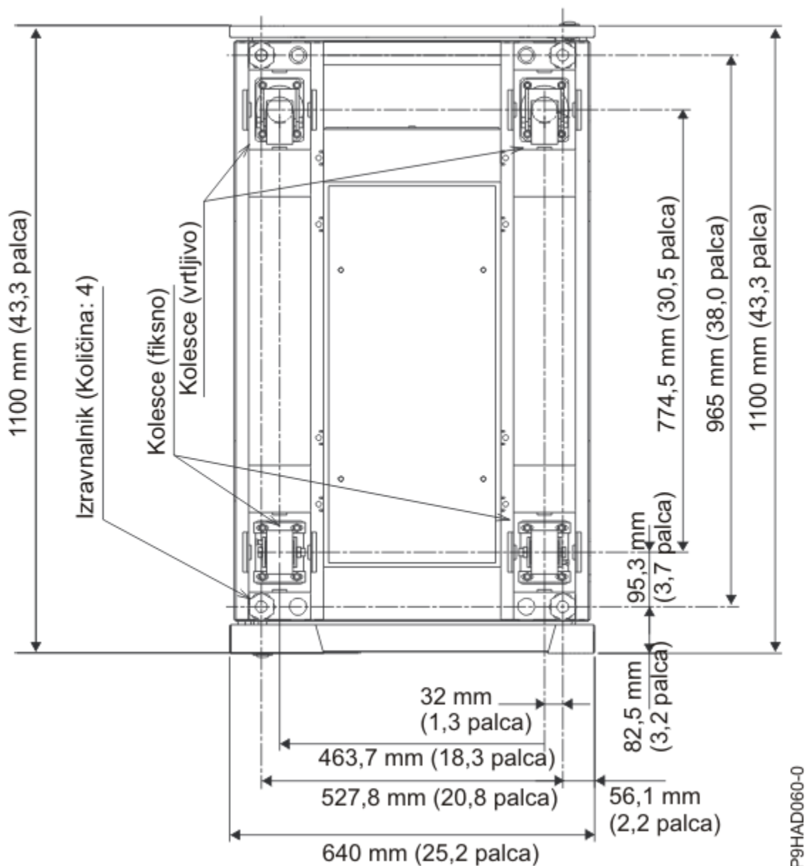
Slika 4. Lokacije kolesc in izravnalnikov
