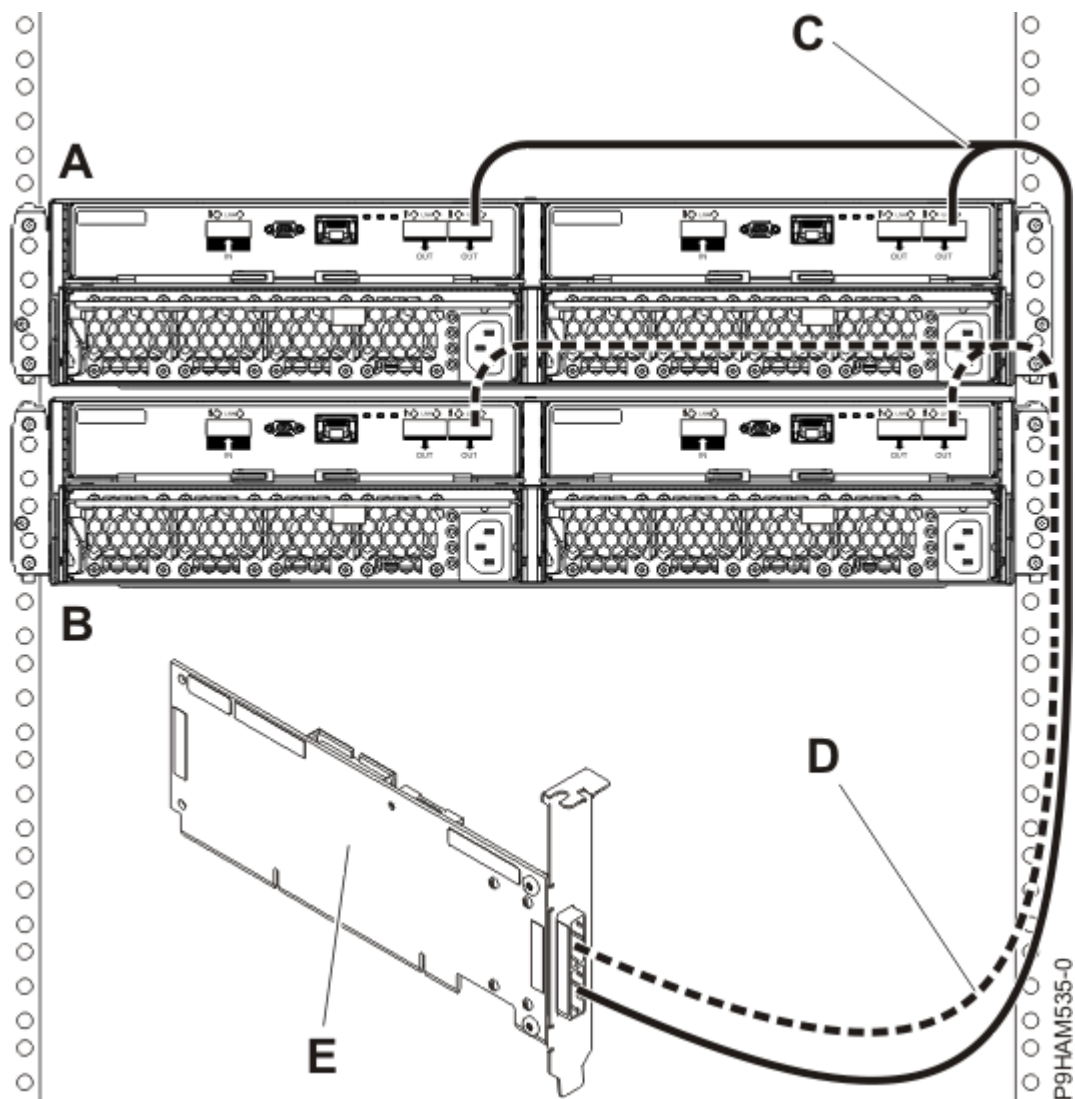
Slika 67. Povezava v načinu 1 dveh ohišij 5887 s kablji YO z enim vmesnikom SAS
