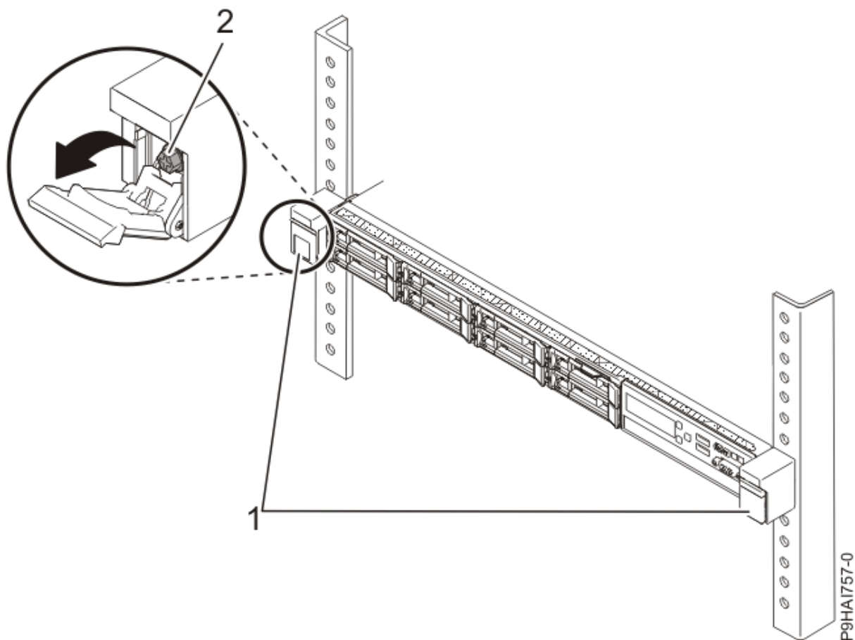
Slika 15. Prednje vodilo omare in nožice
