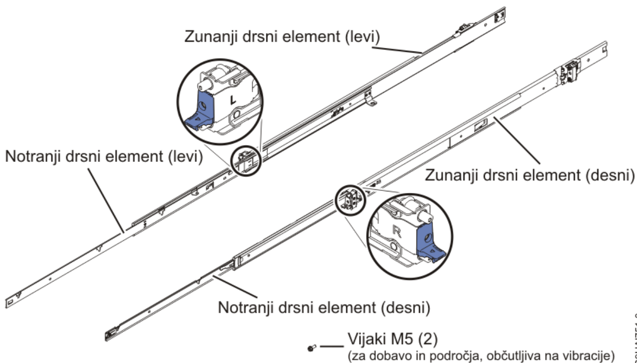
Slika 10. Vsebina škatle z vodili
