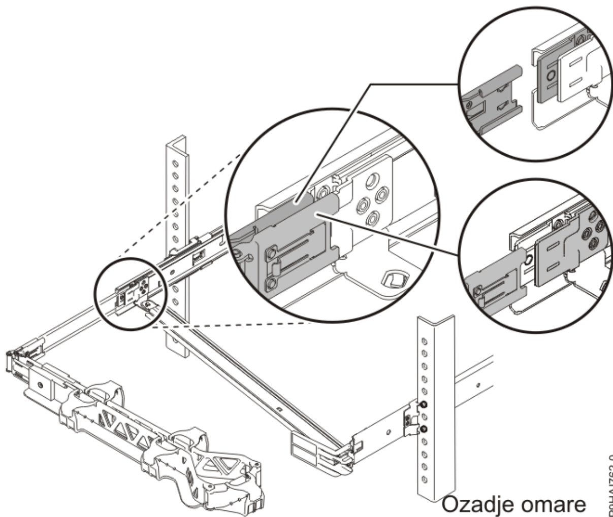
Slika 20. Povezava roke za napeljavo kablov
