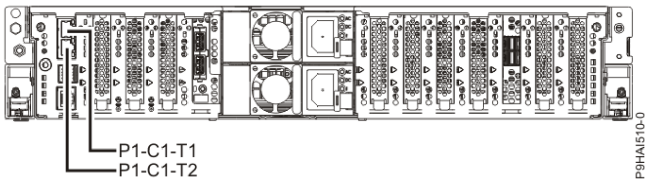
Slika 26. Lokacije vrat na HMC-ju 5105-22E, 9008-22L, 9009-22A, 9009-22G, 9223-22H in 9223-22S
