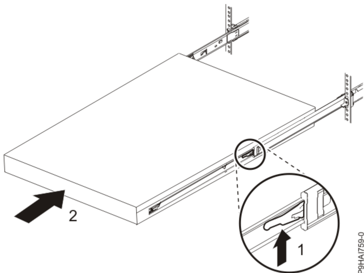
Slika 17. Sprostitutveni zatiči in strežnik
