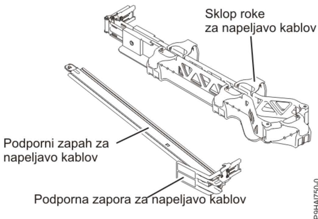
Slika 9. Vsebina škatle z roko za napeljavo kablov
