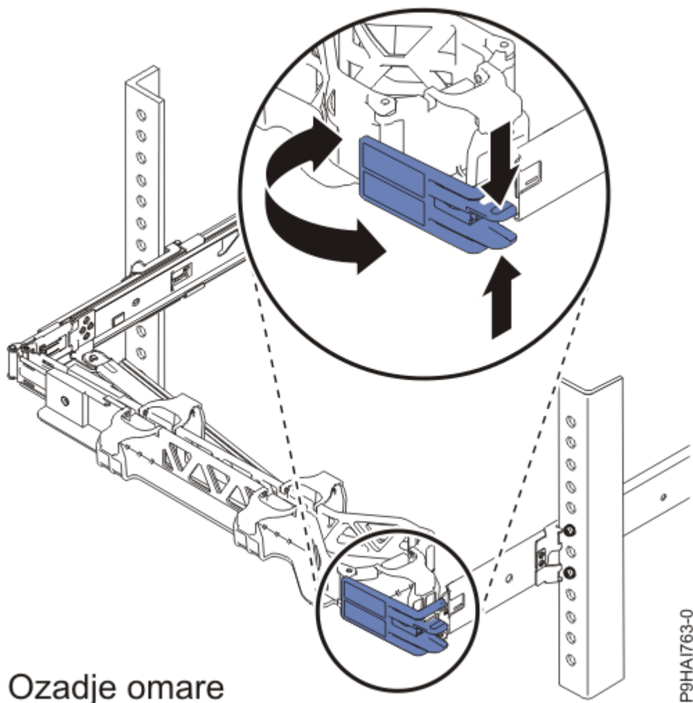
Slika 21. Podporni zaustavitveni nosilec za napeljavo kablov
