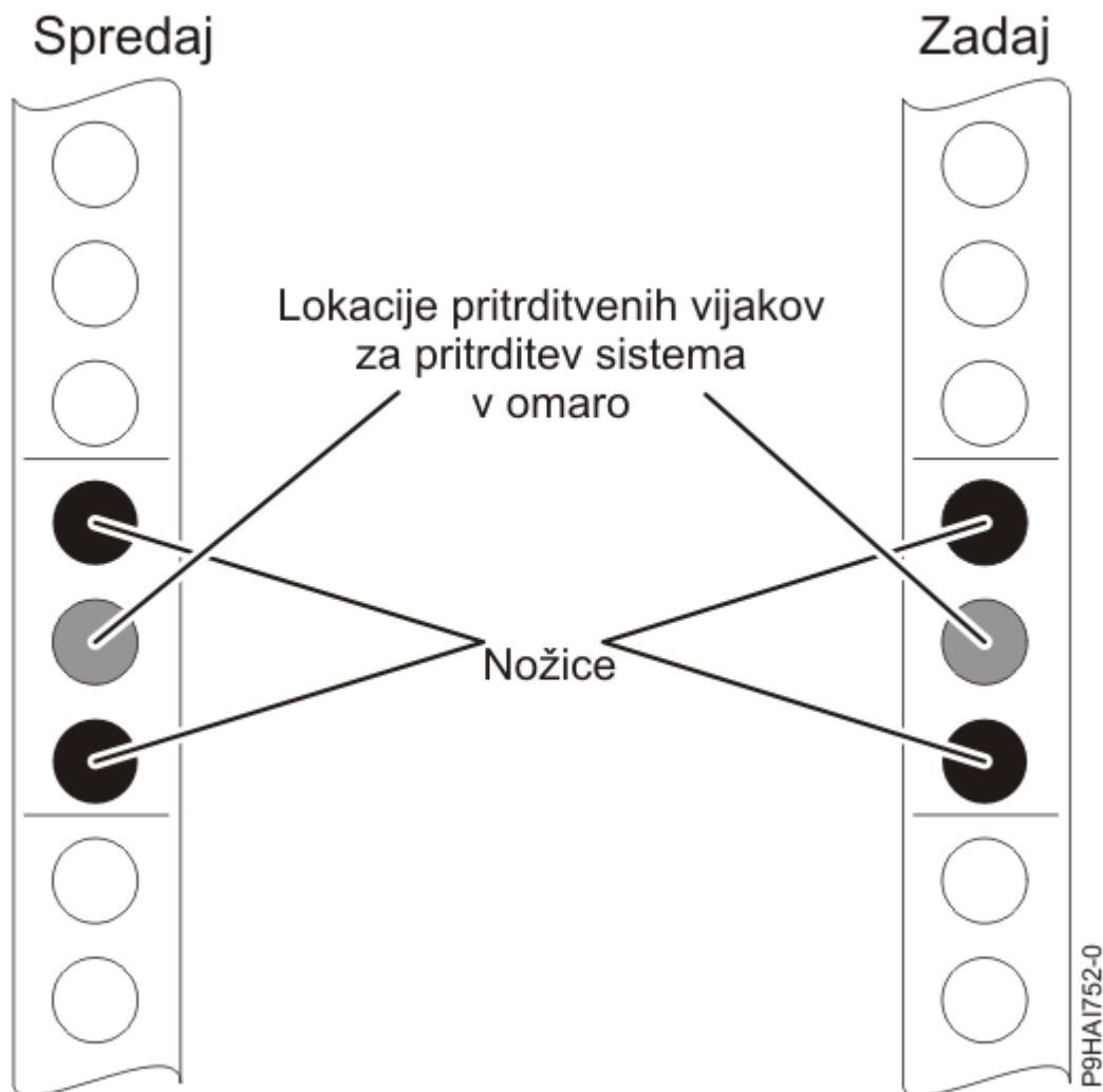
Slika 11. Identificiranje prostora v omaro
