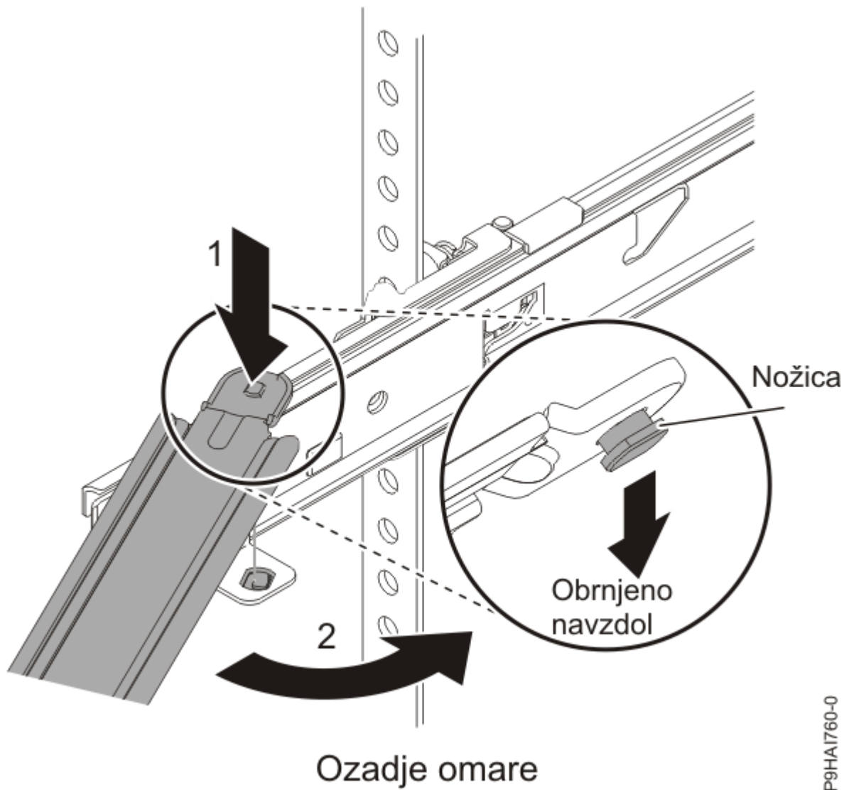
Slika 18. Povezava podporne roke
