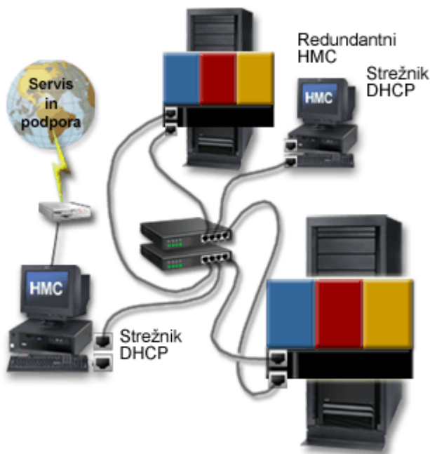
Slika 25. Zasebno omrežje z enim HMC kot strežnikom DHCP
