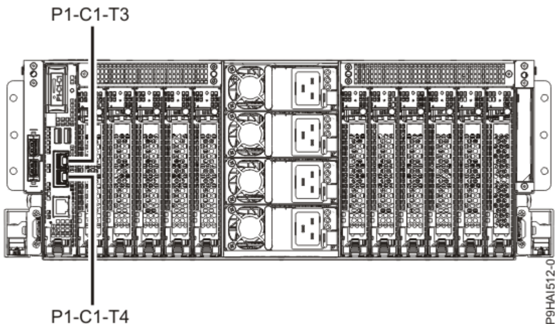
Slika 28. Lokacije vrat na HMC-ju 9040-MR9
