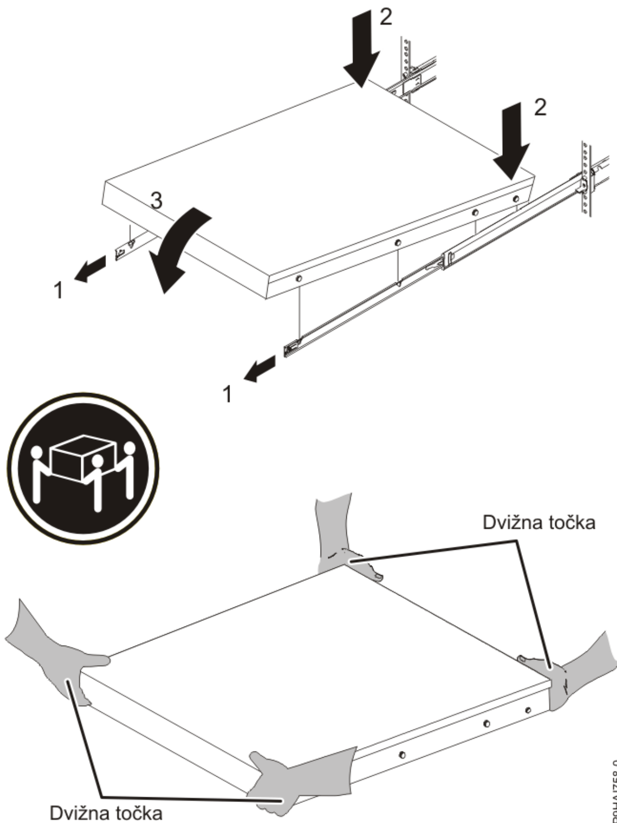
Slika 16. Drsna vodila so iztegnjena, glave žebličkov so poravnane z režami v vodilih in dvižnimi točkami
