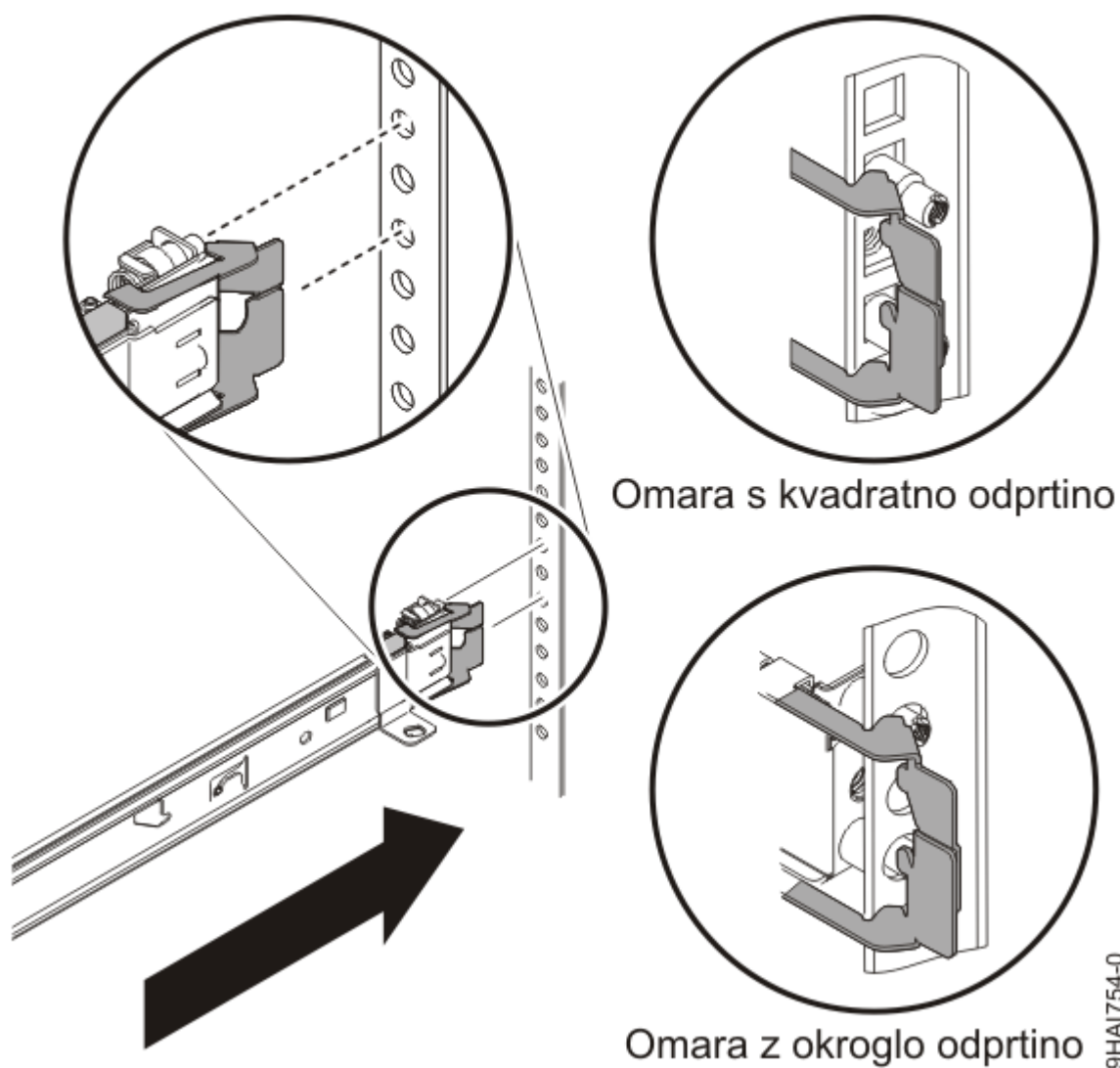
Slika 13. Nožice poravnajte z luknjami v zadnjem delu omare
