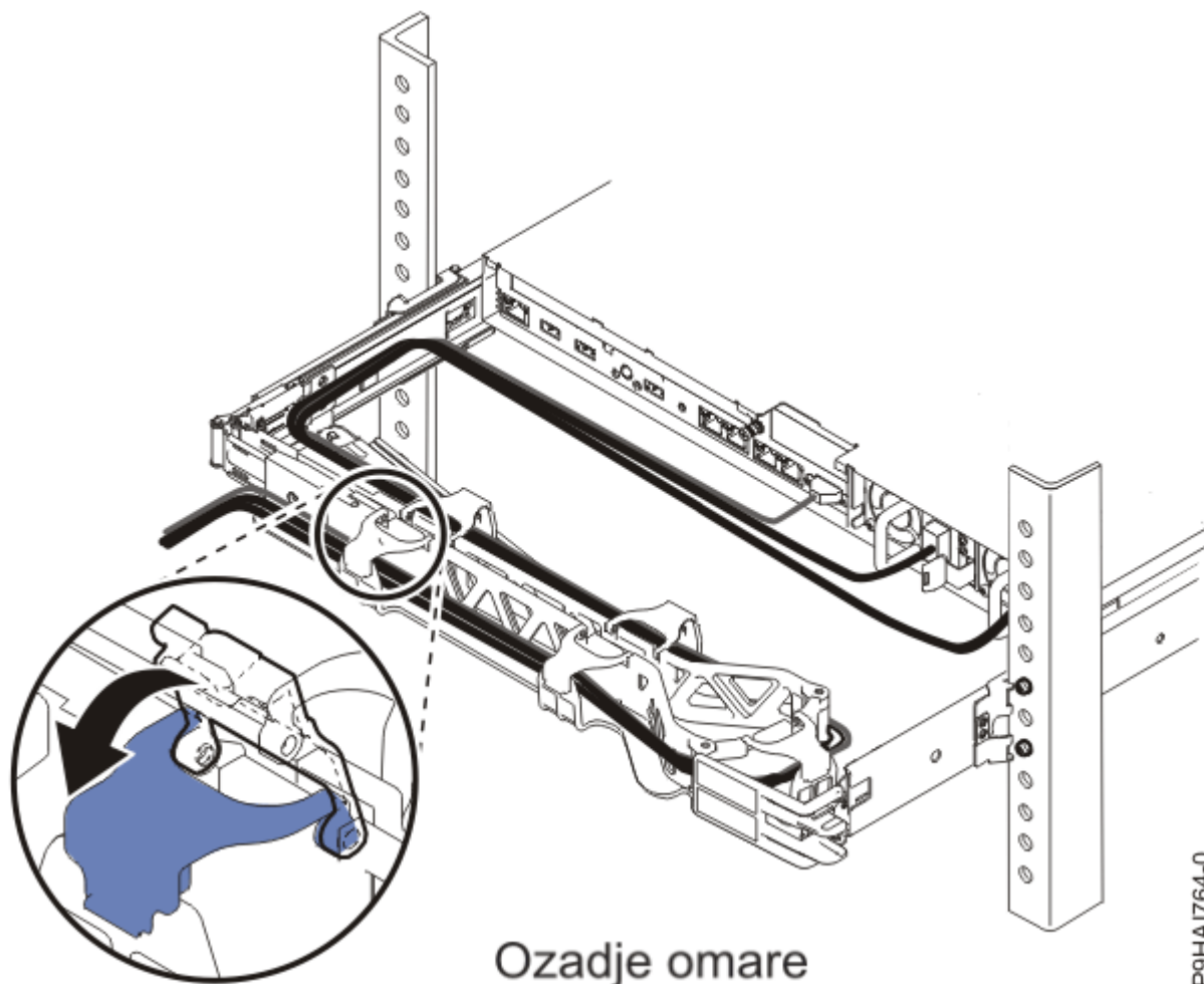
Slika 22. Priklapljanje napajalnega kabla in napeljevanje kabla
