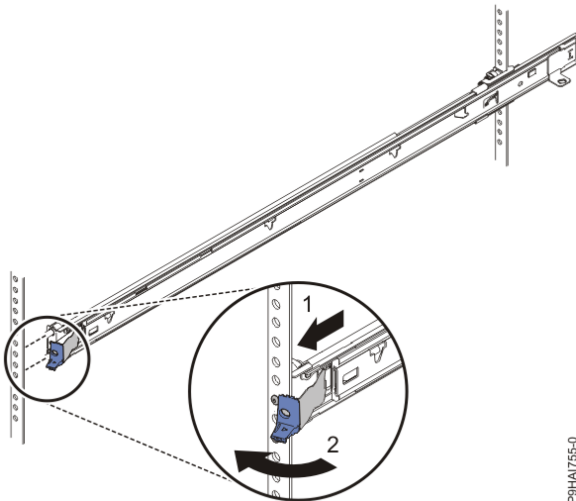
Slika 14. Zatič prednjega drsnega vodila
