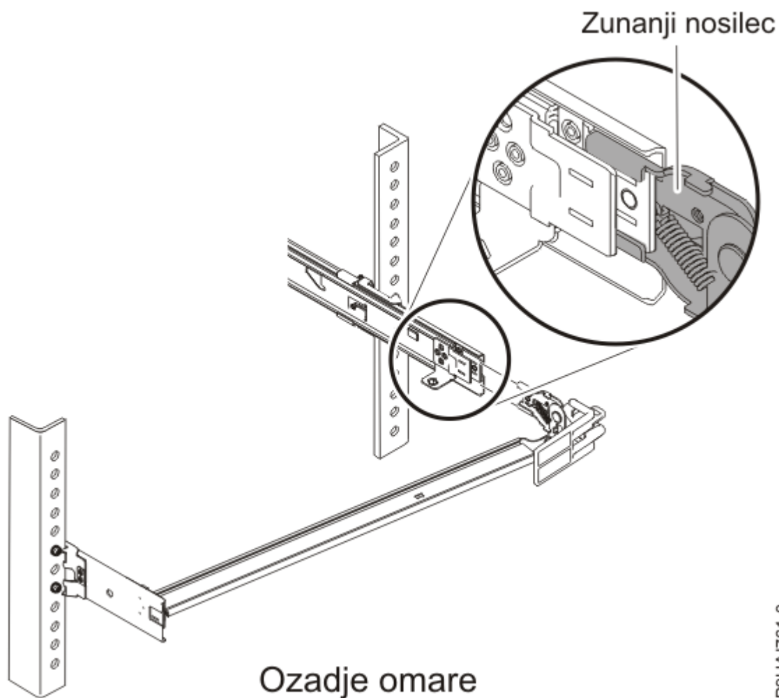
Slika 19. Povezovanje zaustavitvenega nosilca z drsnim vodilom
