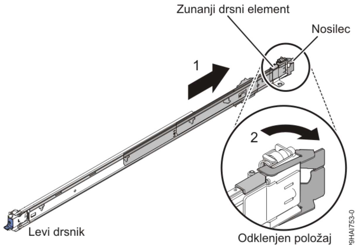
Slika 12. Drsno vodilo in zunanji drsni element
