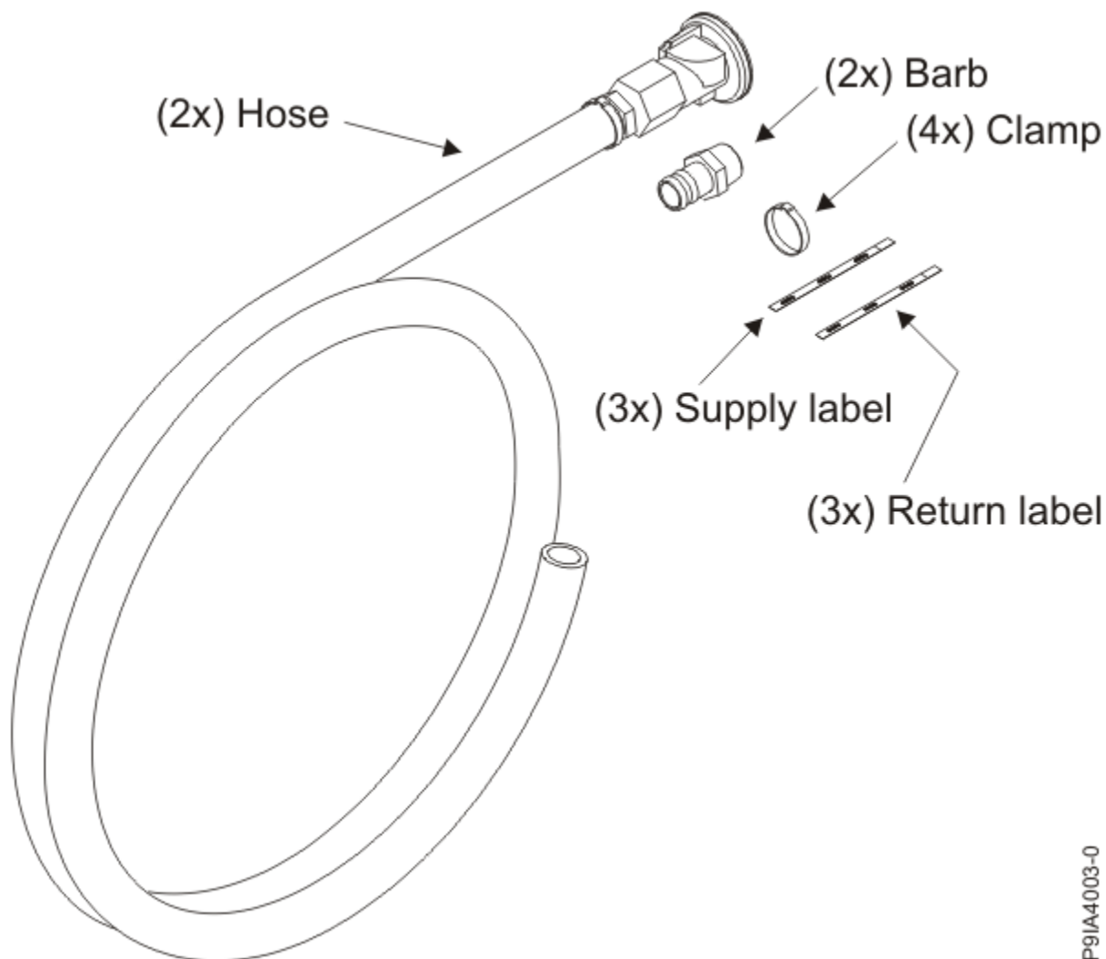
Slika 26. Komplet cevi
