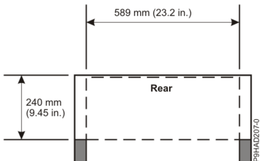
Slika 35. Prostor na zadnji strani omare za modela 9080-M9S
