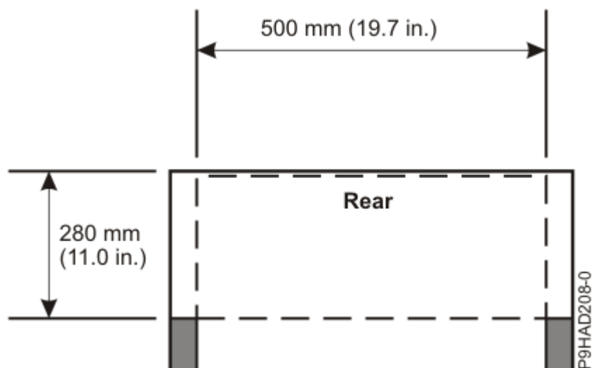
Slika 34. Prostor na zadnji strani omare za modela 9040-MR9
