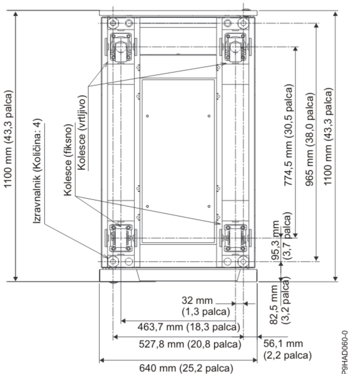
Slika 3. Lokacije koles in izravnalnikov
