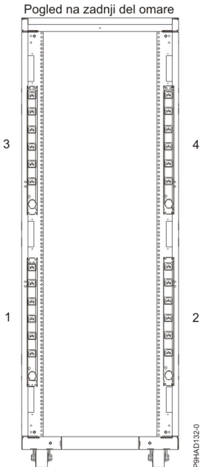
Slika 39. Navpični položaji napajalnih distribucijskih enot
