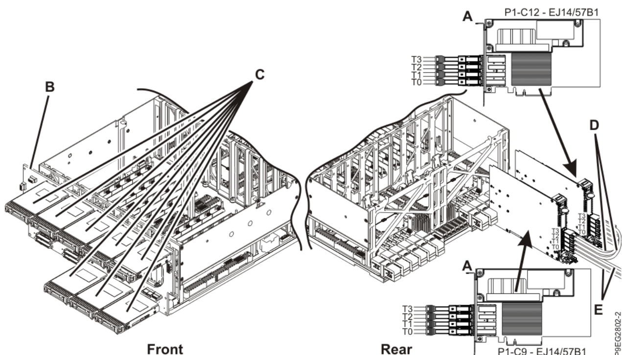
Slika 3. Deli podsistema SAS v sistemu 9040-MR9 s konfiguracijo shrambe razširjene funkcionalnosti
