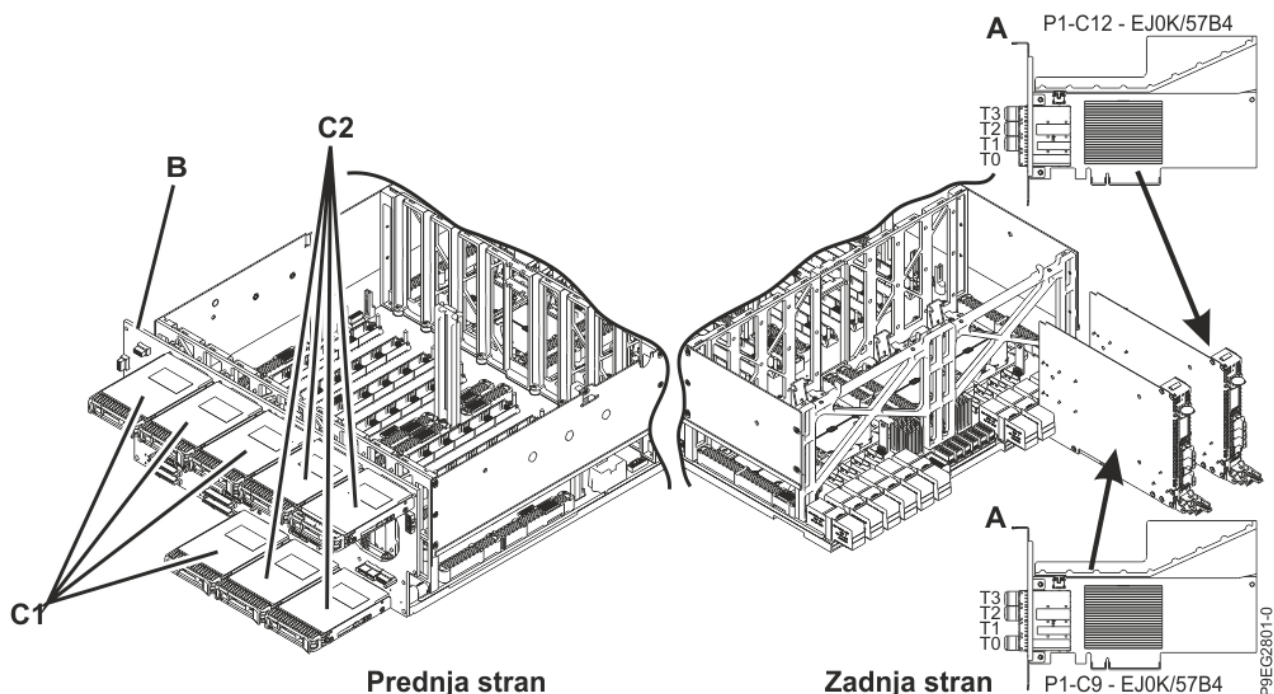
Slika 2. Deli podsistema SAS v sistemu 9040-MR9 s konfiguracijo shrambe osnovna komponenta s funkcijo deljenega diska
