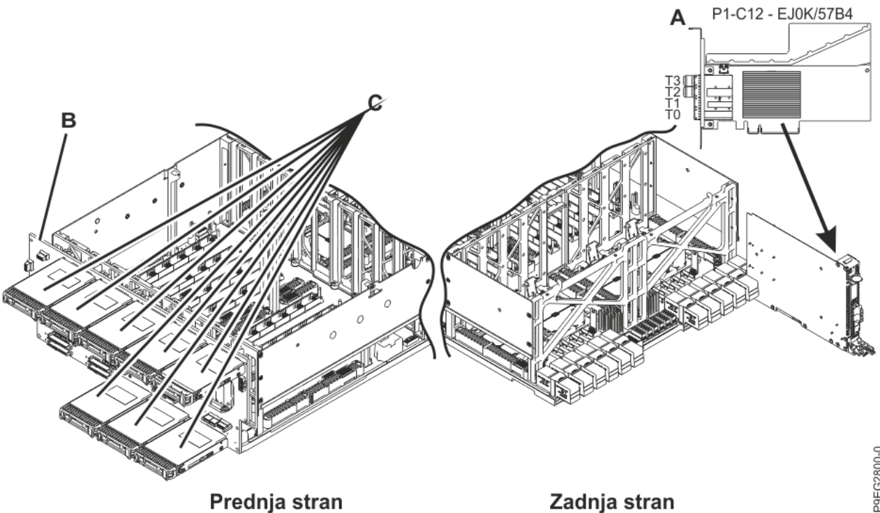
Slika 1. Deli podsistema SAS v sistemu 9040-MR9 s konfiguracijo shrambe osnovna komponenta
