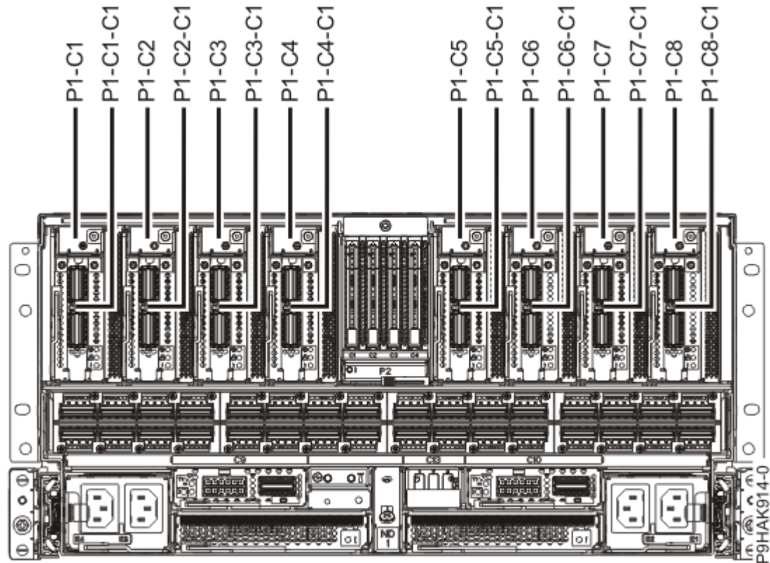
Slika 1. Pogled od zadaj na vgradni sistem 9080-M9S z lokacijskimi kodami rež PCIe
