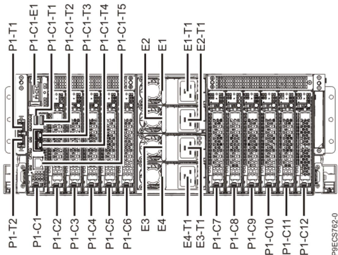
Slika 1. Pogled od zadaj na vgradni sistem 9040-MR9 z lokacijskimi kodami rež PCIe
