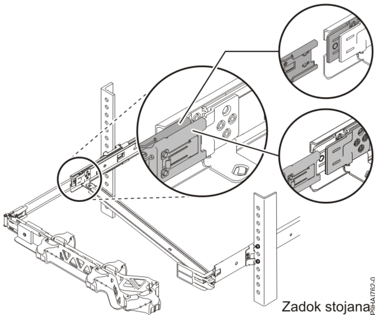
Obrázok 20. Pripojenie ramena na organizáciu káblov
