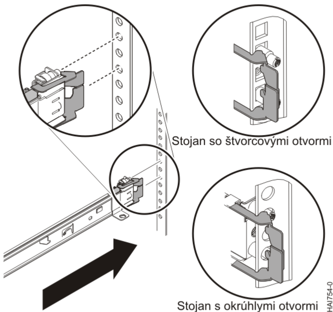
Obrázok 13. Zarovnajte kolíky s otvormi na zadnej strane stojana
