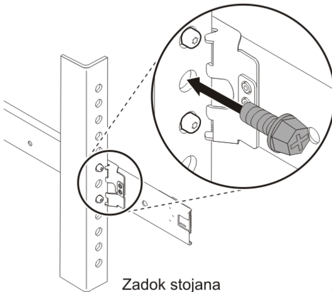
Obrázok 24. Zabezpečenie servera pri preprave
