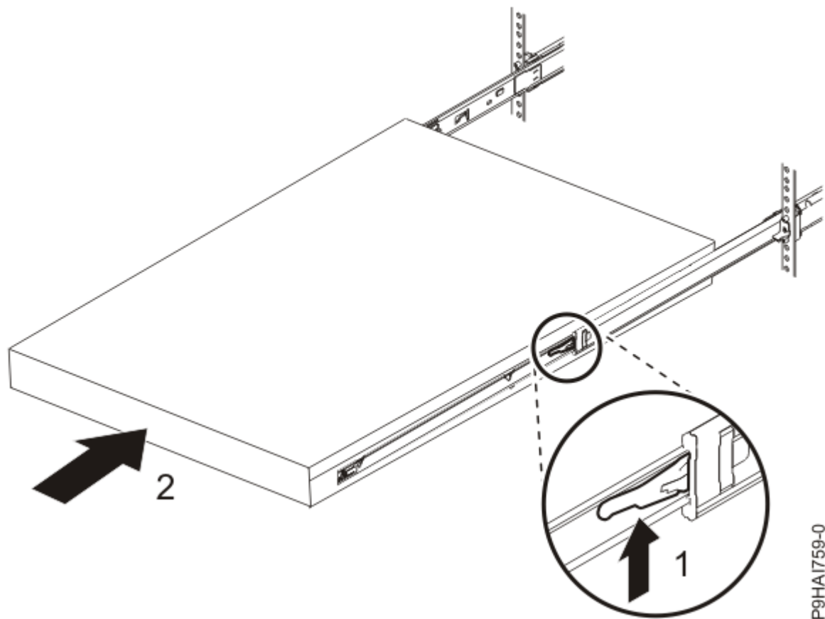
Obrázok 17. Uvoľňovacie úchytky a server
