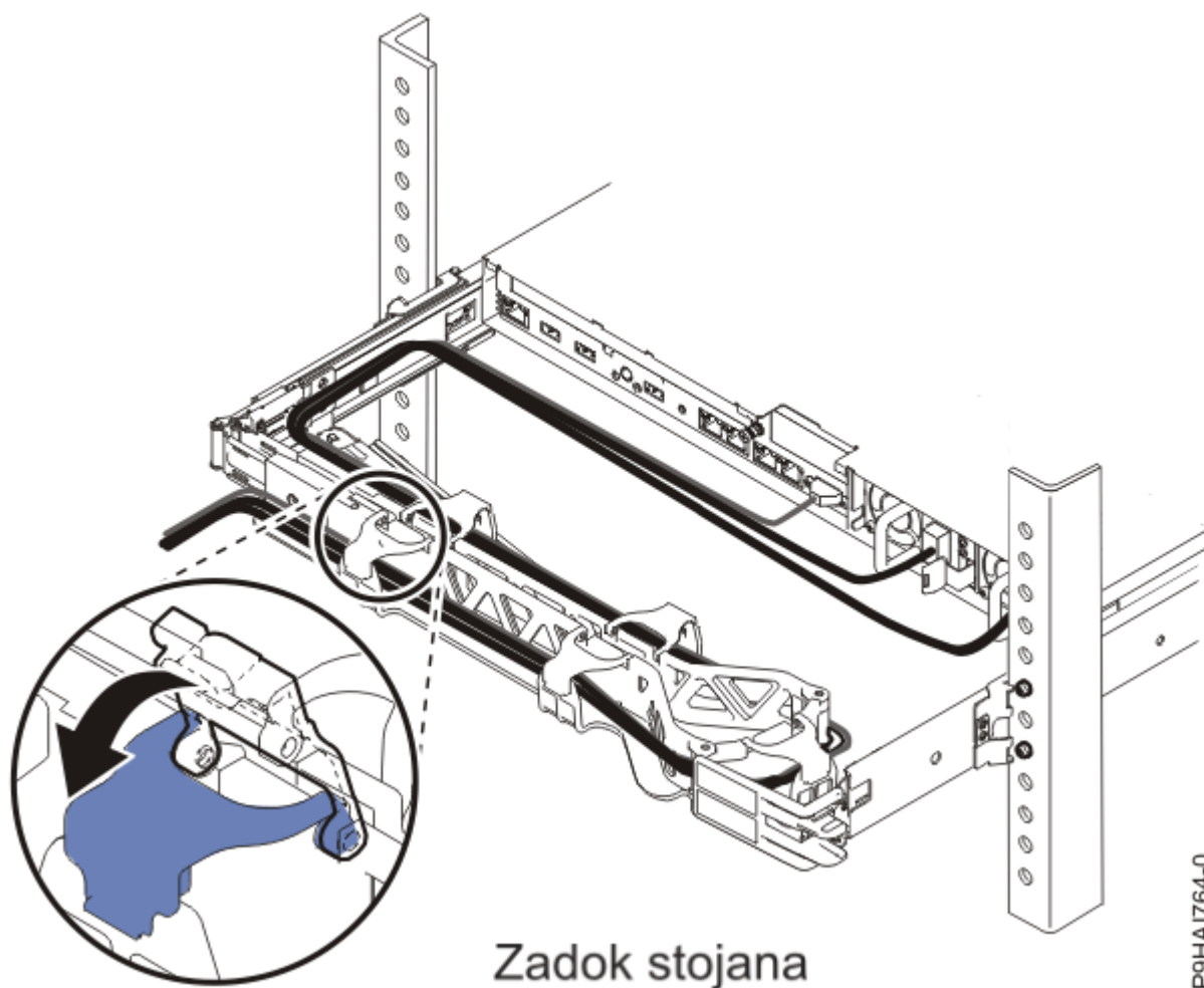
Obrázok 22. Pripojenie napájacieho kábla a vedenie kábla
