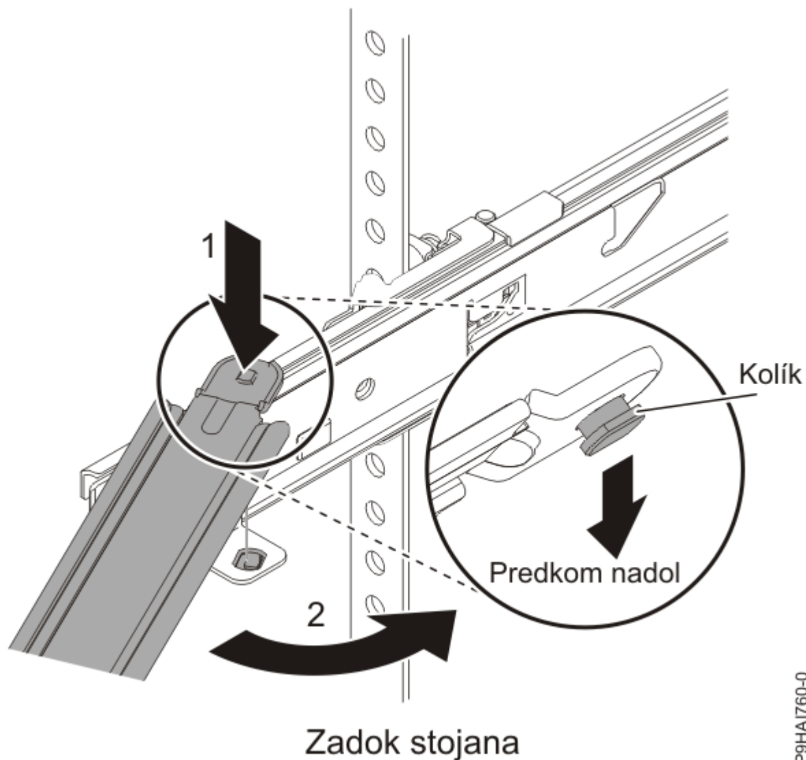
Obrázok 18. Pripojenie podporného ramena
