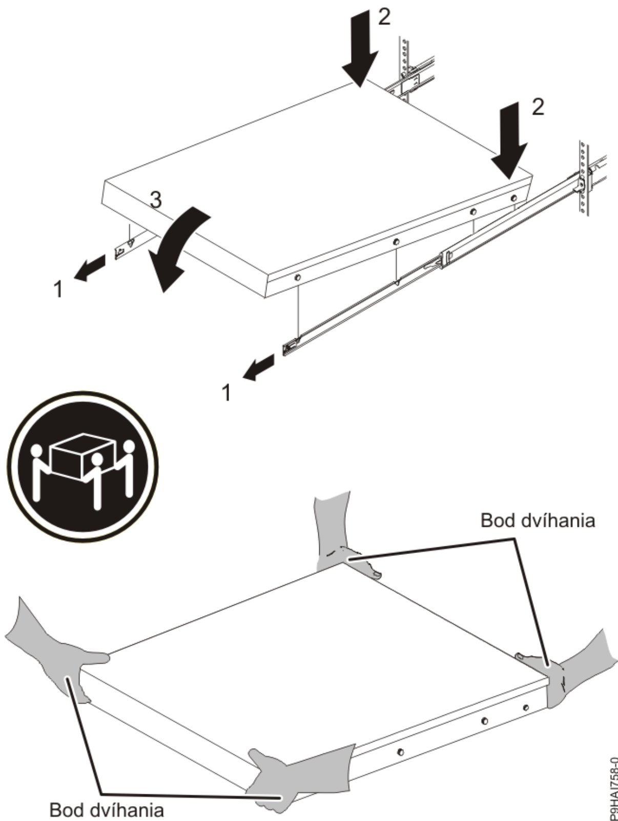
Obrázok 16. Vysunuté posuvné koľajničky, hlavičky kolíkov servera zarovnané s otvormi v koľajničke a dvíhacie body
