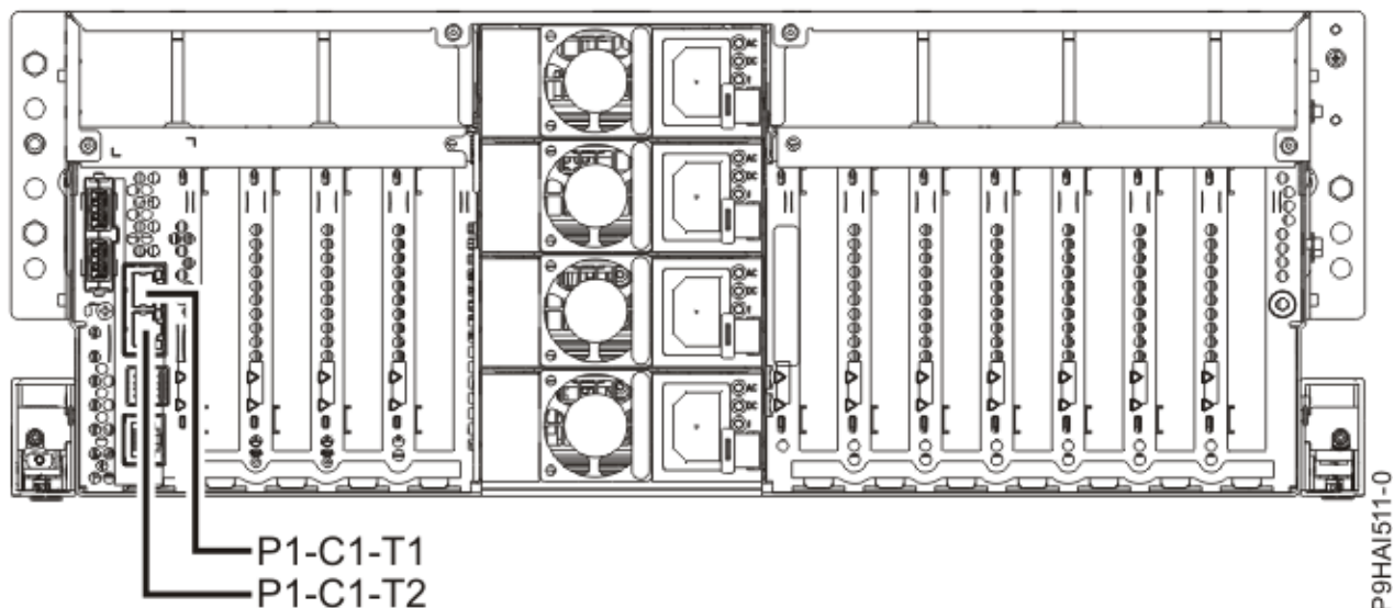
Obrázok 27. Umiestnenia portov konzoly HMC 9009-41A, 9009-41G, 9009-42A, 9009-42G, 9223-42H a 9223-42S
