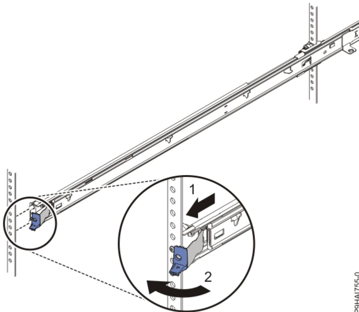
Obrázok 14. Predná blokovacia úchytka posuvnej koľajničky
