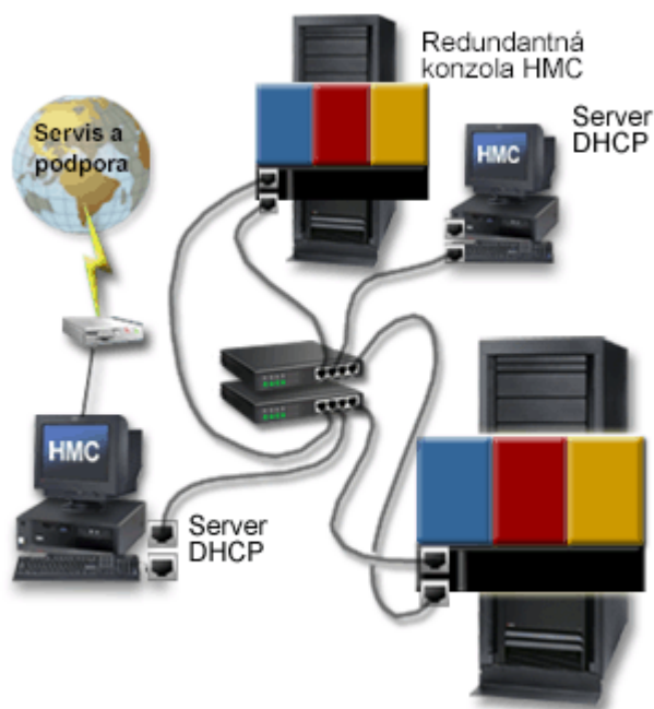
Obrázok 25. Súkromná sieť s jednou konzolou HMC ako serverom DHCP
