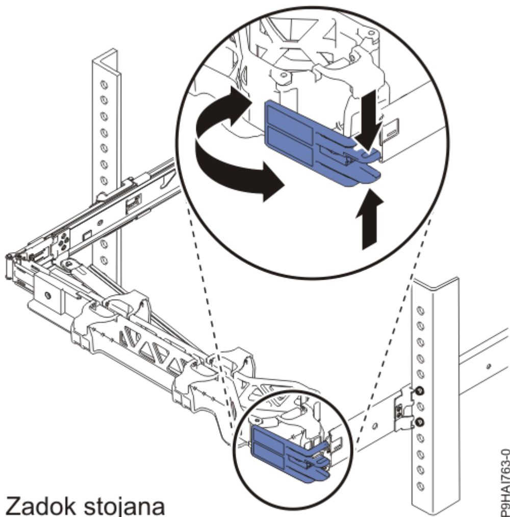
Obrázok 21. Podporná zarážka pre organizáciu káblov
