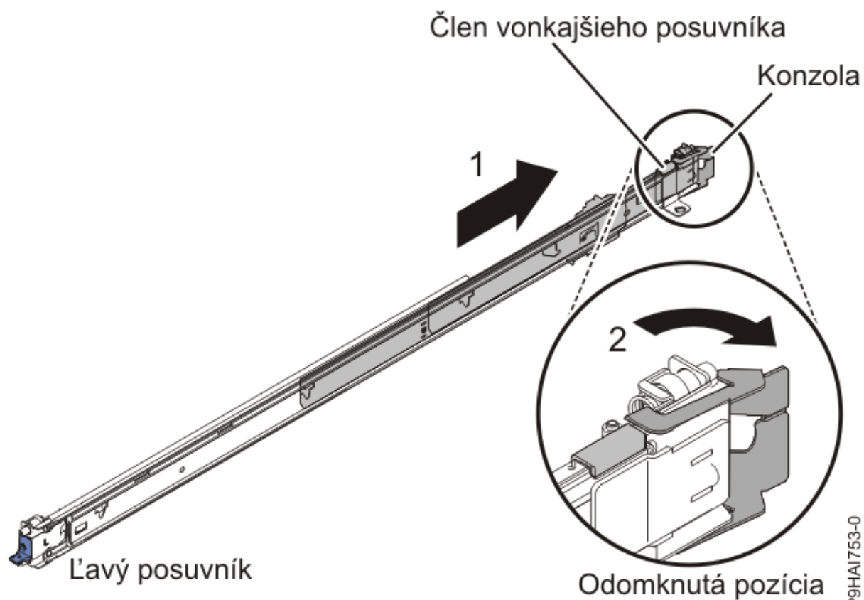
Obrázok 12. Posuvná koľajnička a člen vonkajšieho posuvníka
