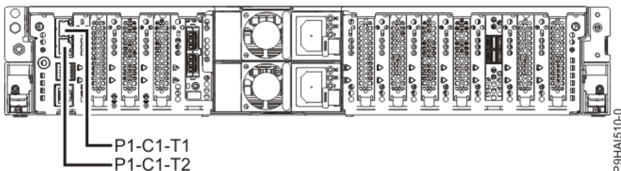
Obrázok 26. Umiestnenia portov konzoly HMC 5105-22E, 9008-22L, 9009-22A, 9009-22G, 9223-22H a 9223-22S
