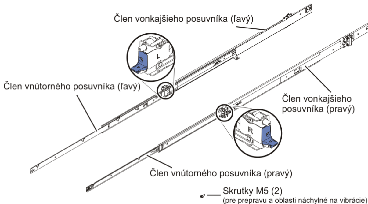
Obrázok 10. Obsah škatule s koľajničkami
