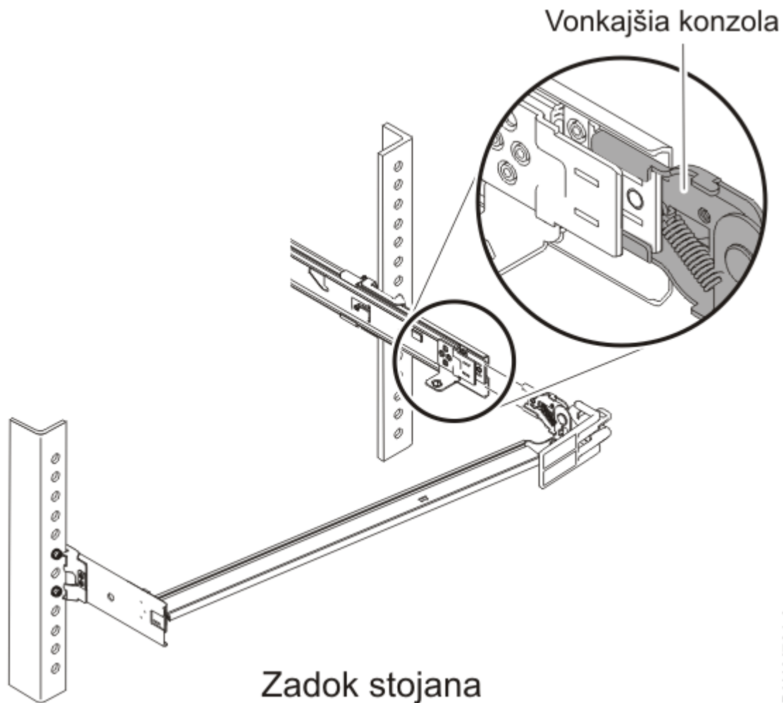
Obrázok 19. Pripojenie blokovej konzoly k posuvnej koľajničke
