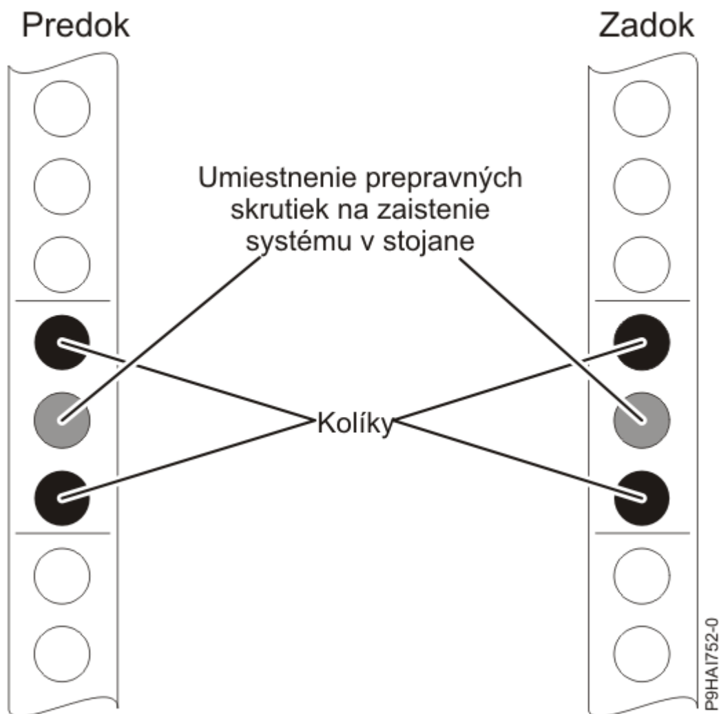
Obrázok 11. Identifikácia priestoru v stojane
