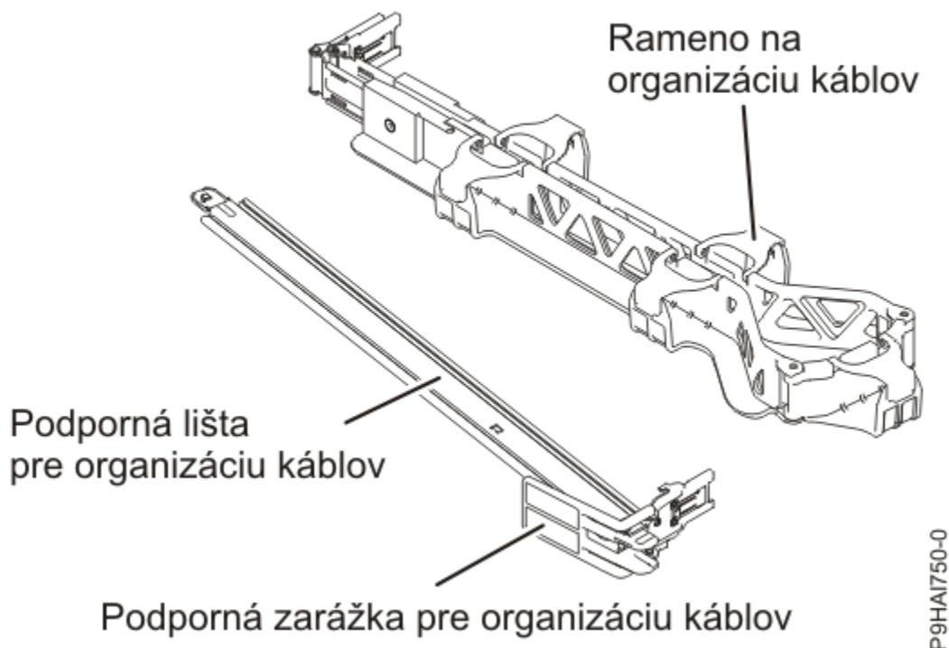
Obrázok 9. Obsah škatule s ramenom na organizáciu káblov
