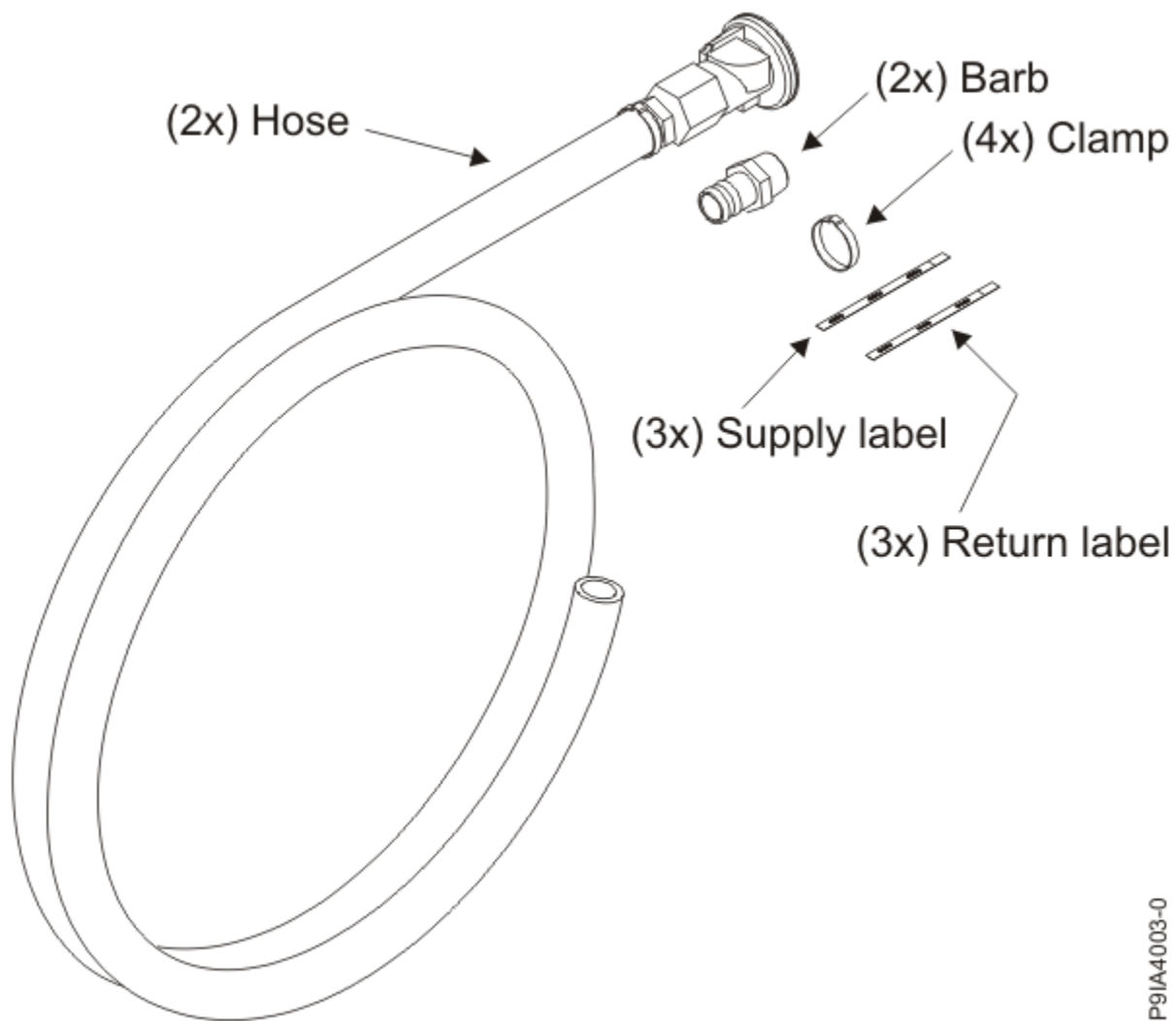
Obrázok 26. Súprava hadíc
