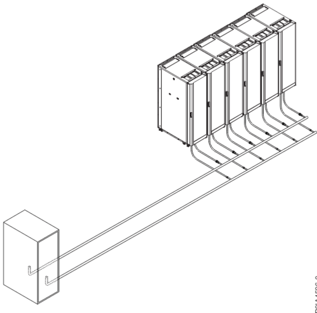
Obrázok 25. Typický rozšírený rozvádzač
