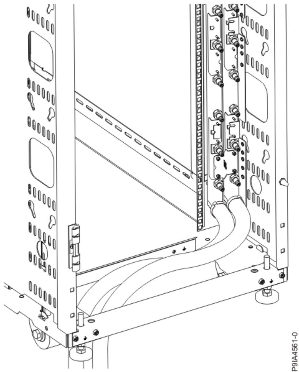
Figura 21. Locații de ieșire furtunuri în partea de jos
