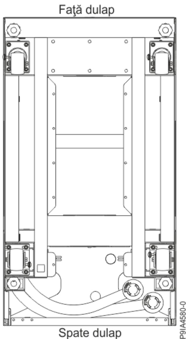
Figura 37. Locațiile de ieșire pentru furtunuri în partea de jos (vedere de jos)
