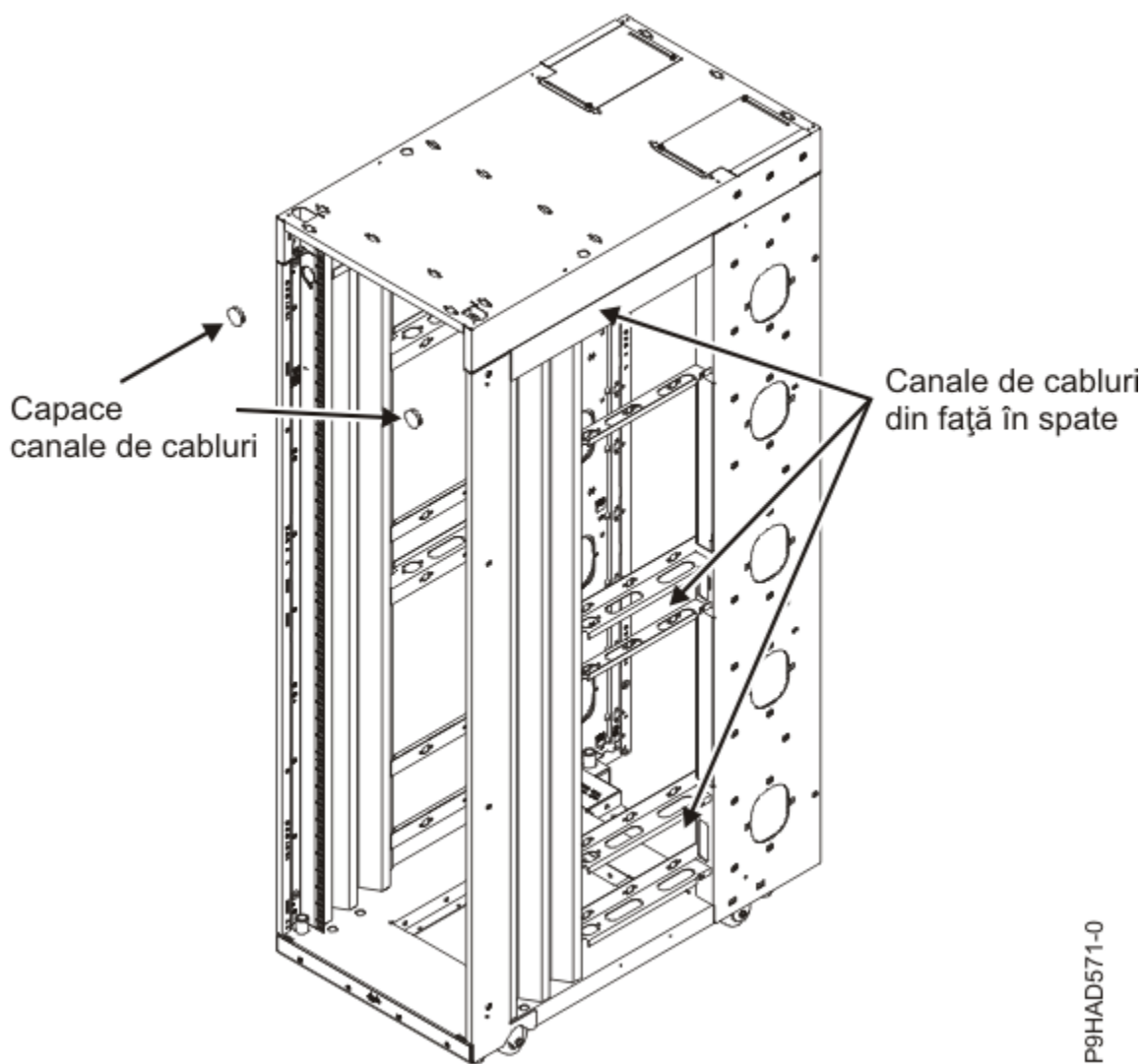
Figura 26. Cablarea în dulap
