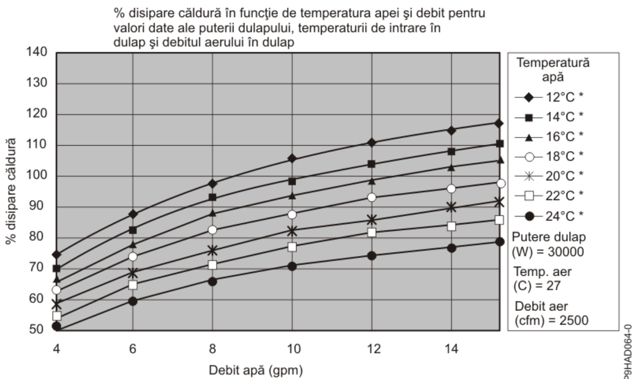
Figura 31. Performanța tipică a schimbătorului de căldură, 30 kW sarcină termică
