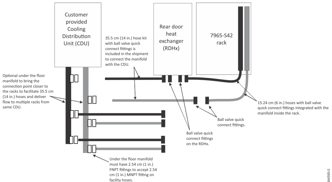
Figura 48. Schemă CDU cu furtunurile rețelei de apă pentru colector și RDHx ce se conectează la un colector de sub podea
