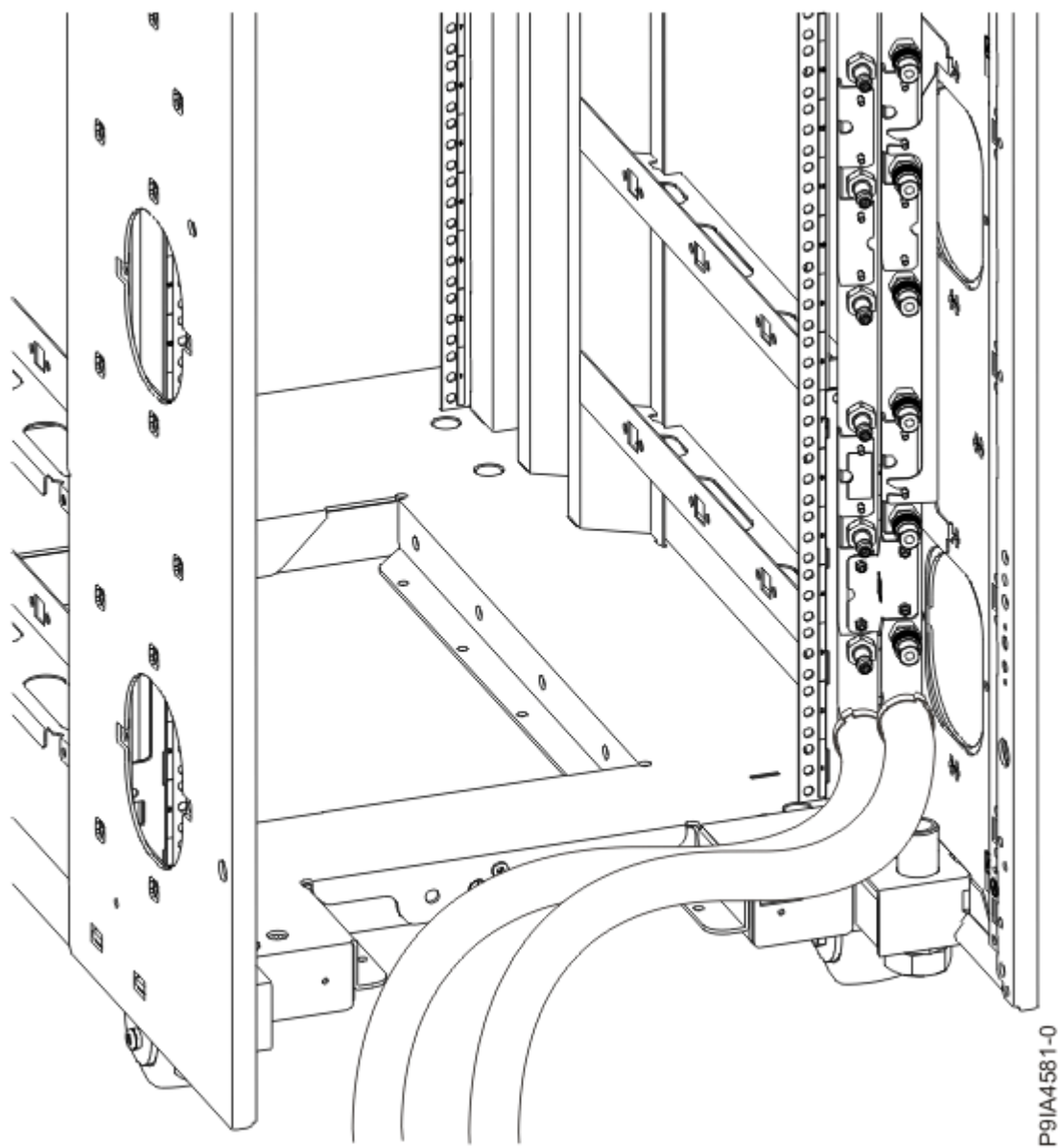
Figura 36. Locațiile de ieșire pentru furtunuri în partea de jos
