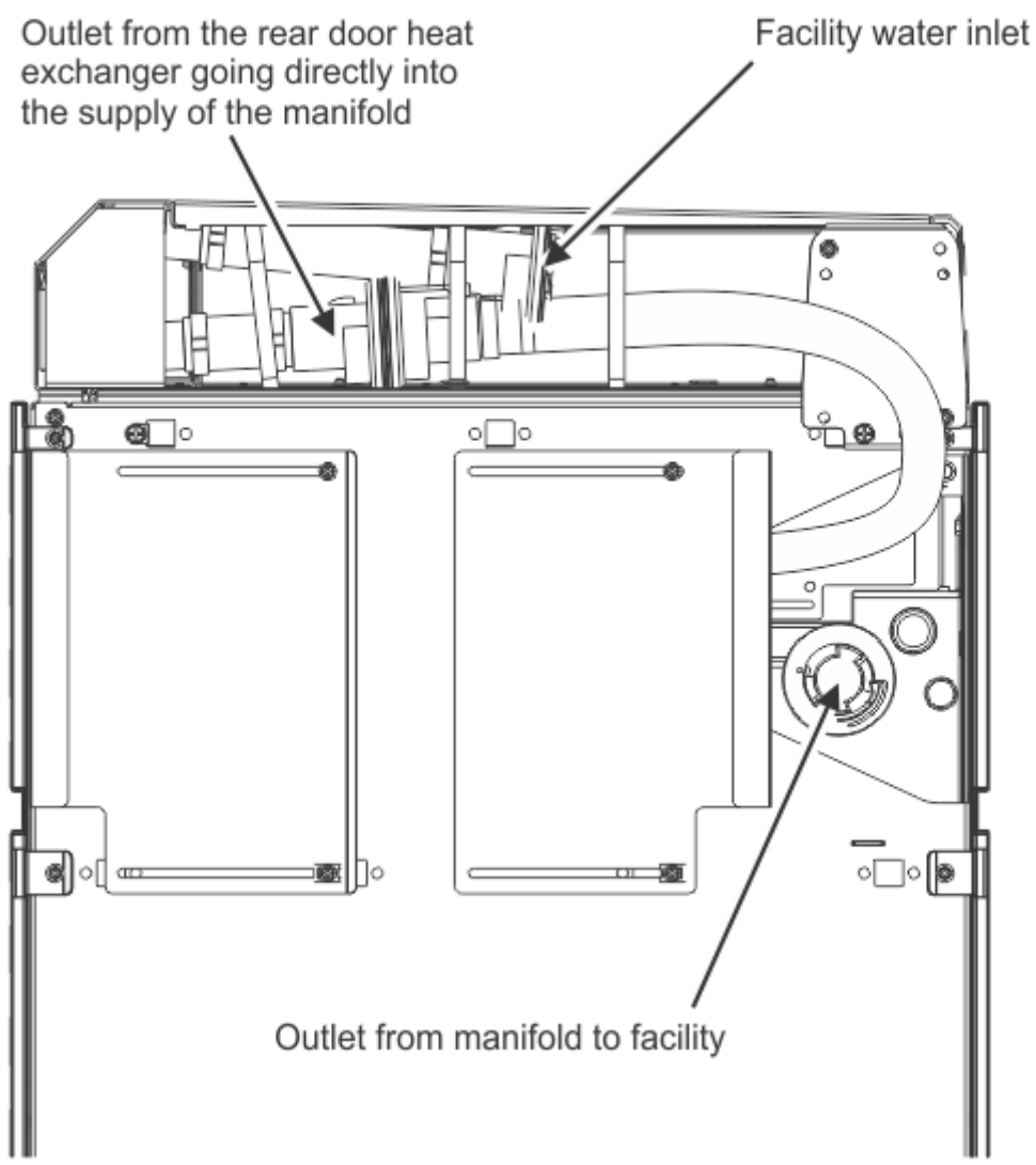
Figura 45. Configurație cu ieșirea sus (vedere de sus în jos)
