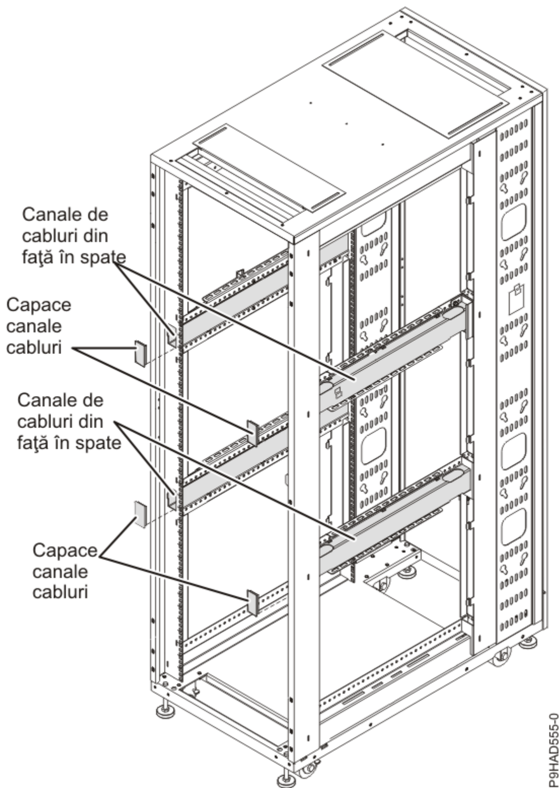
Figura 10. Cablarea în dulap
