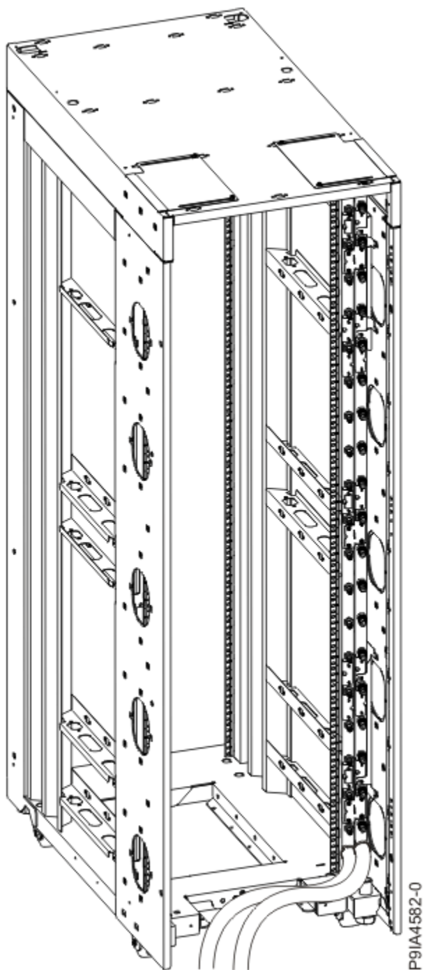
Figura 33. Dulap și colector cu furtunuri de alimentare și retur care ies prin partea de jos a dulapului
