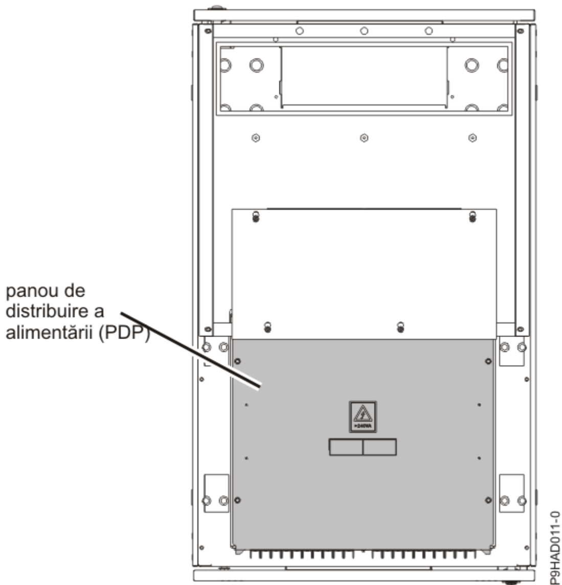
Figura 4. FC EPB8 - panou de distribuire a alimentării (vizualizare de sus în jos)
