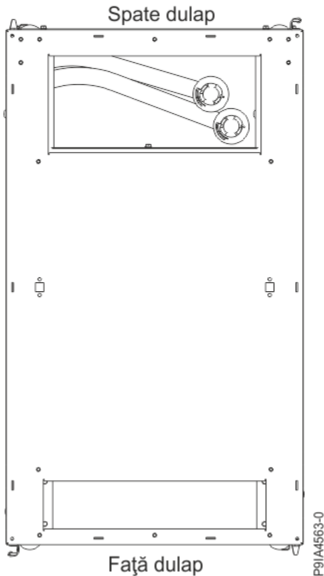
Figura 20. Locațiile de ieșire ale furtunului în partea de sus (vedere de sus)
