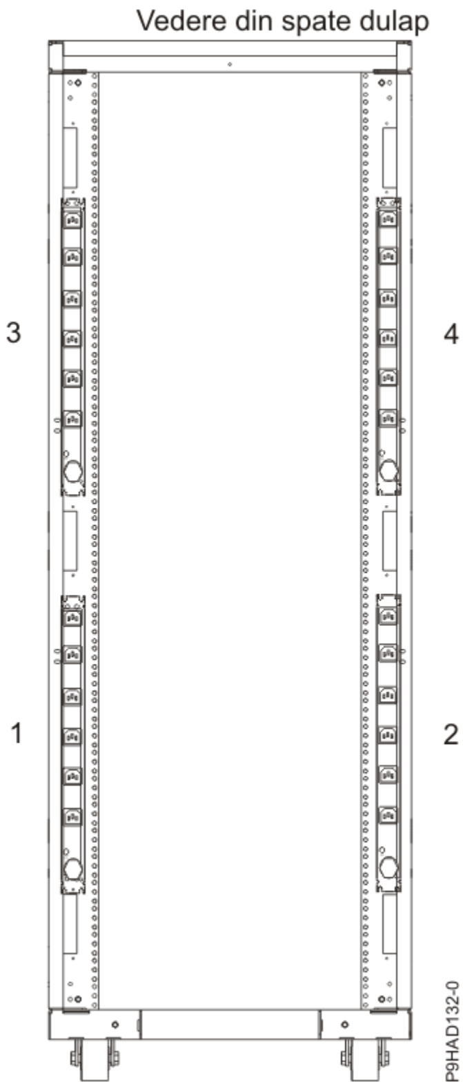
Figura 54. Locații verticale pentru Unitatea de distribuție alimentare
