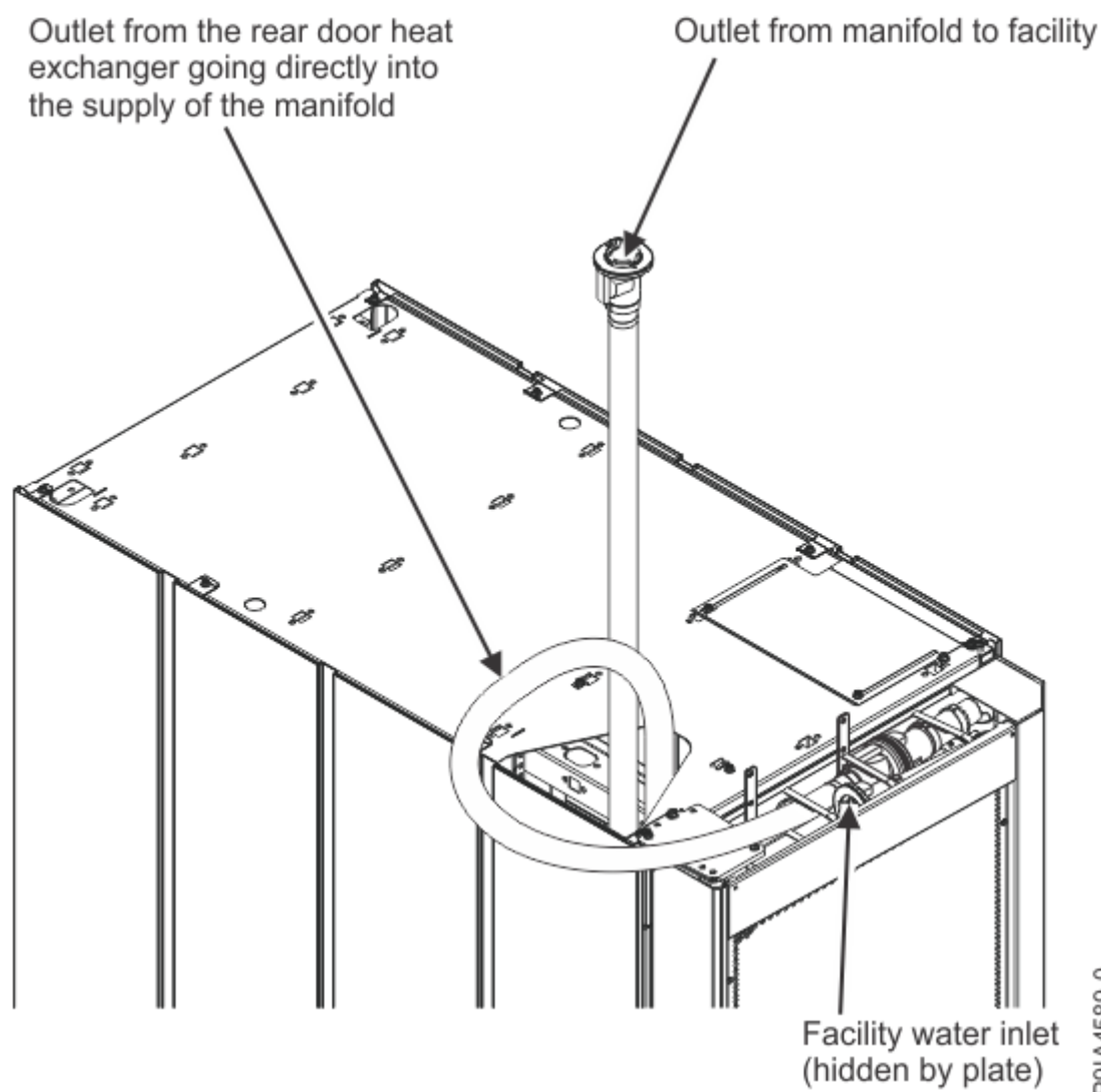
Figura 44. Configurație cu ieșirea sus
