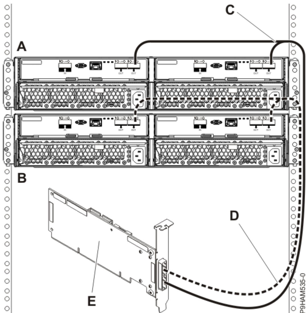
Figura 71. Conexiune mod 1 a două incinte de stocare 5887 folosind cabluri YO la un singur adaptor SAS
