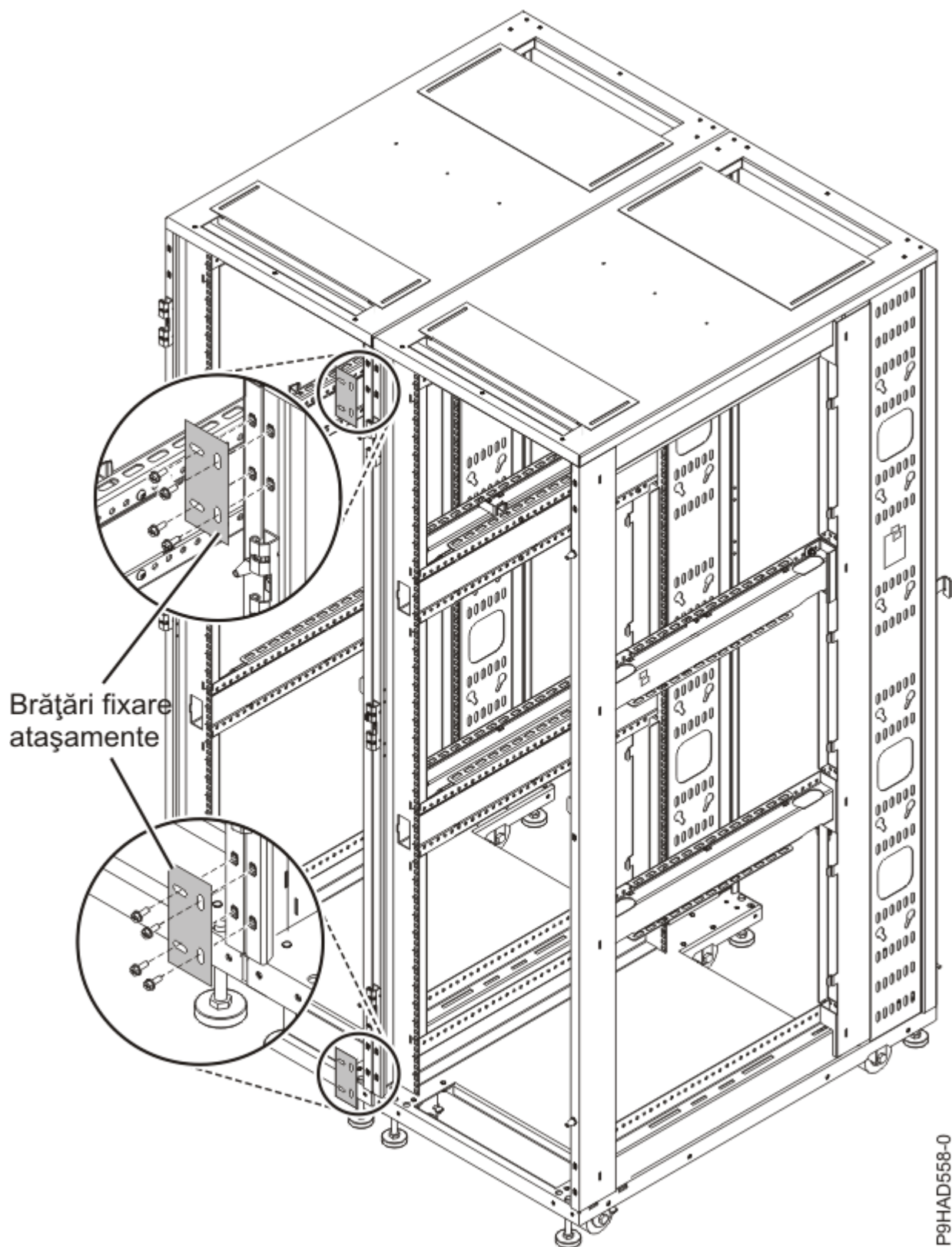
Figura 14. Inele de legătură
