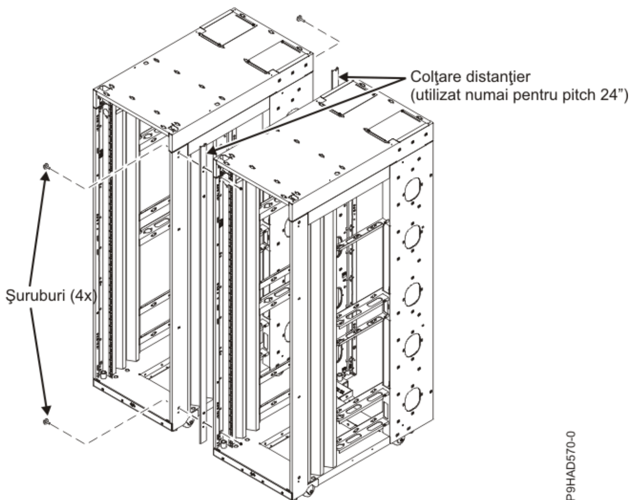
Figura 29. Atașarea mai multor dulapuri cu colțare distanțier
