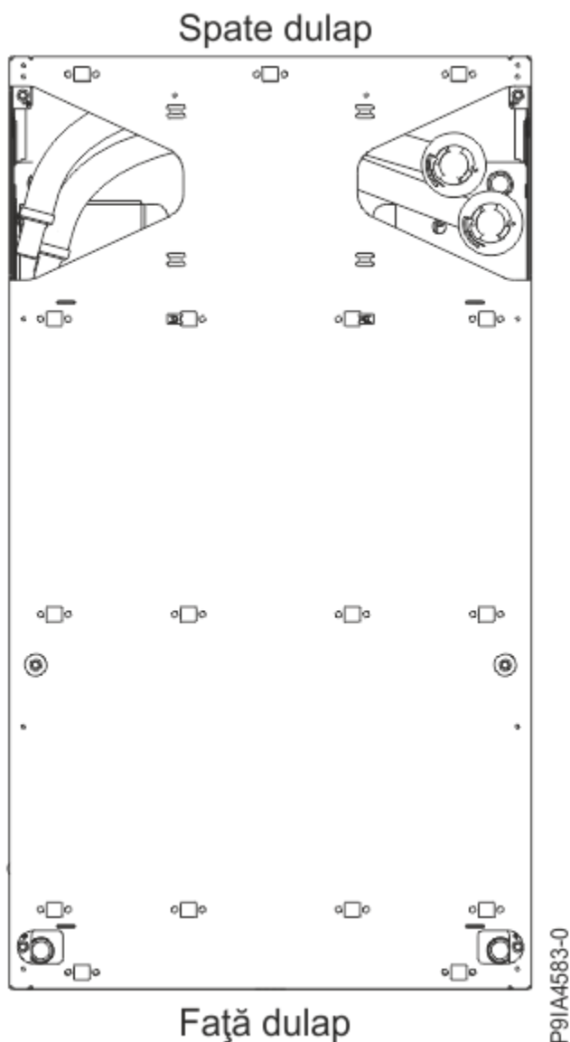
Figura 35. Locațiile de ieșire pentru furtunuri în partea de jos (vedere de sus)
