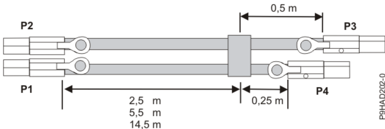
Figura 62. Lungimile de cablu pentru ansamblul cablu YO extern SAS
