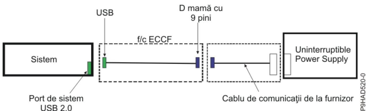
Figura 53. Cablarea UPS pentru
