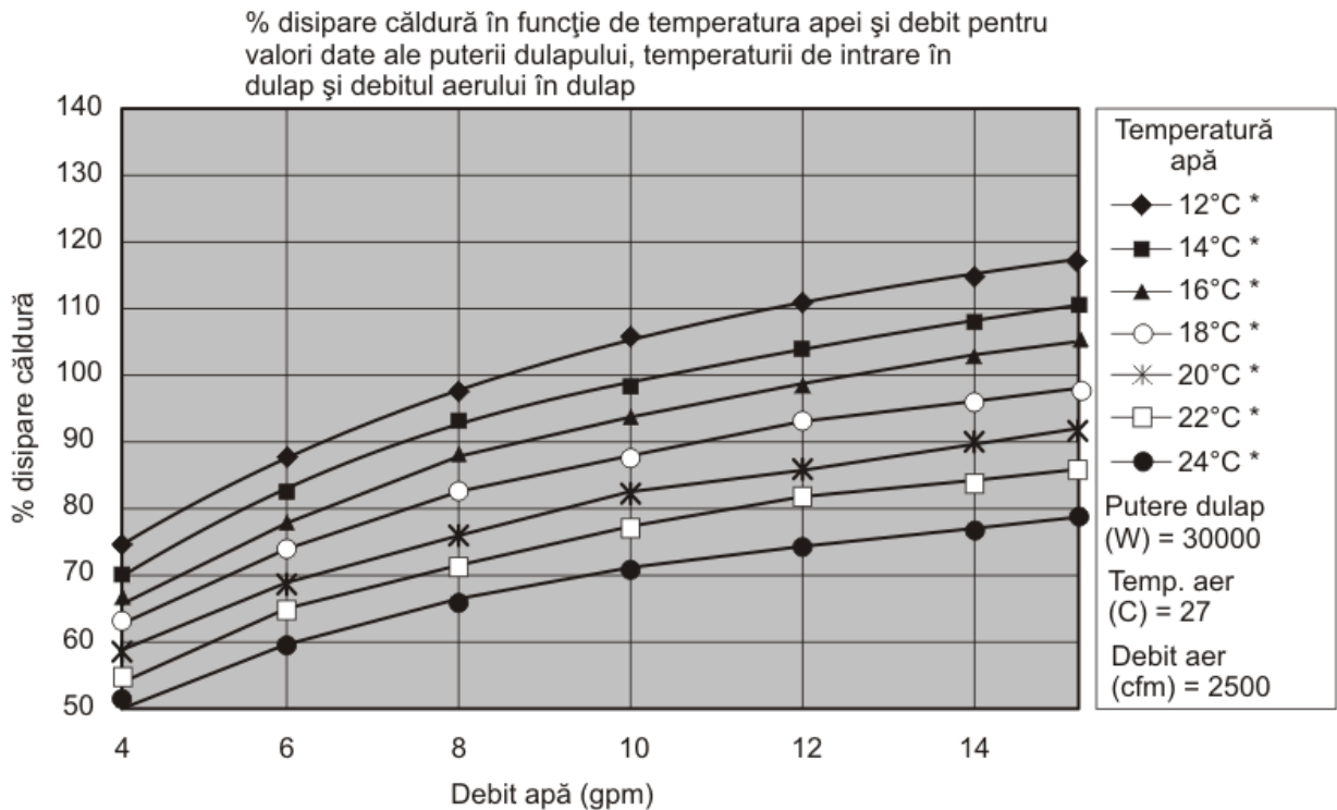
Figura 16. Performanța tipică a schimbătorului de căldură, 30 kW sarcină termică
