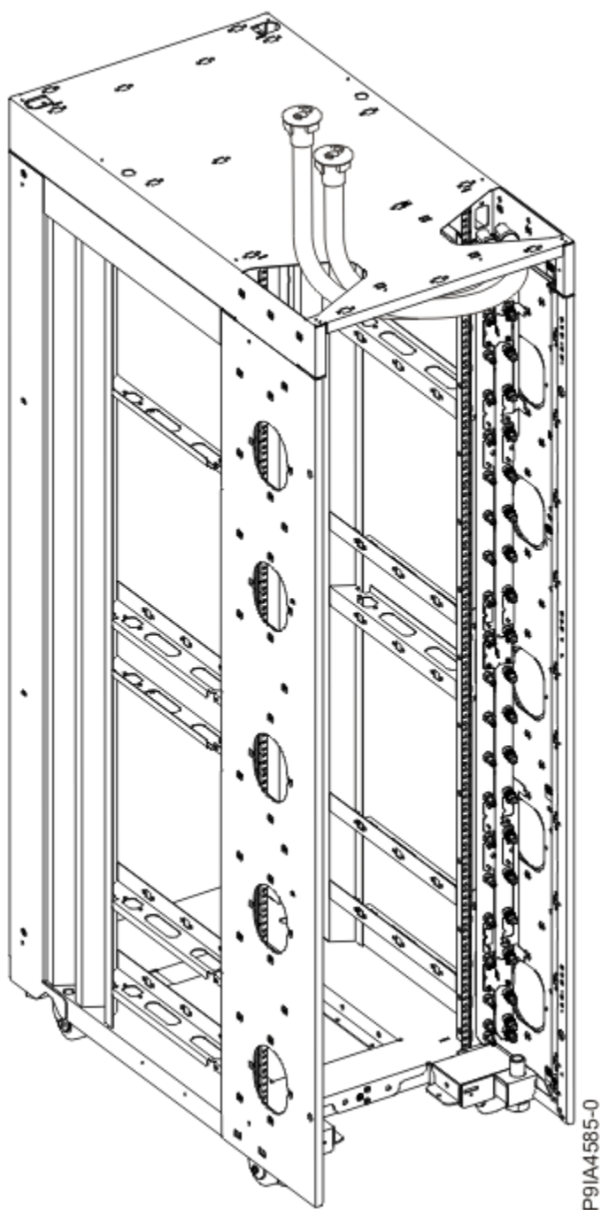
Figura 32. Dulap și colector cu furtunuri de alimentare și retur care ies prin partea de sus a dulapului
