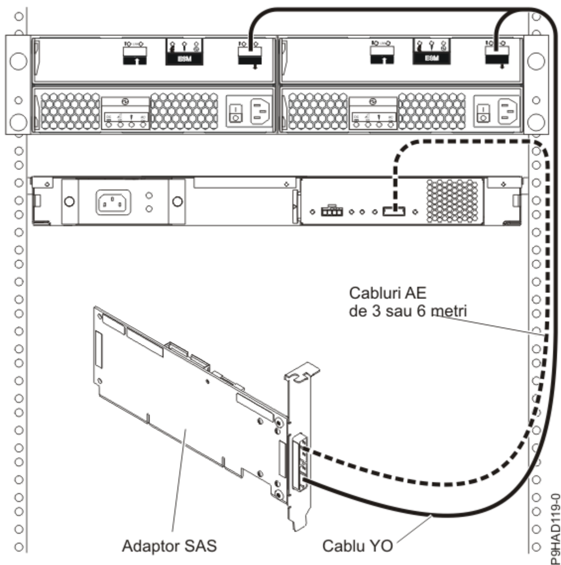
Figura 64. Adaptor SAS la un sertar de expansiune pentru discuri sau un sertar de expansiune pentru medii
