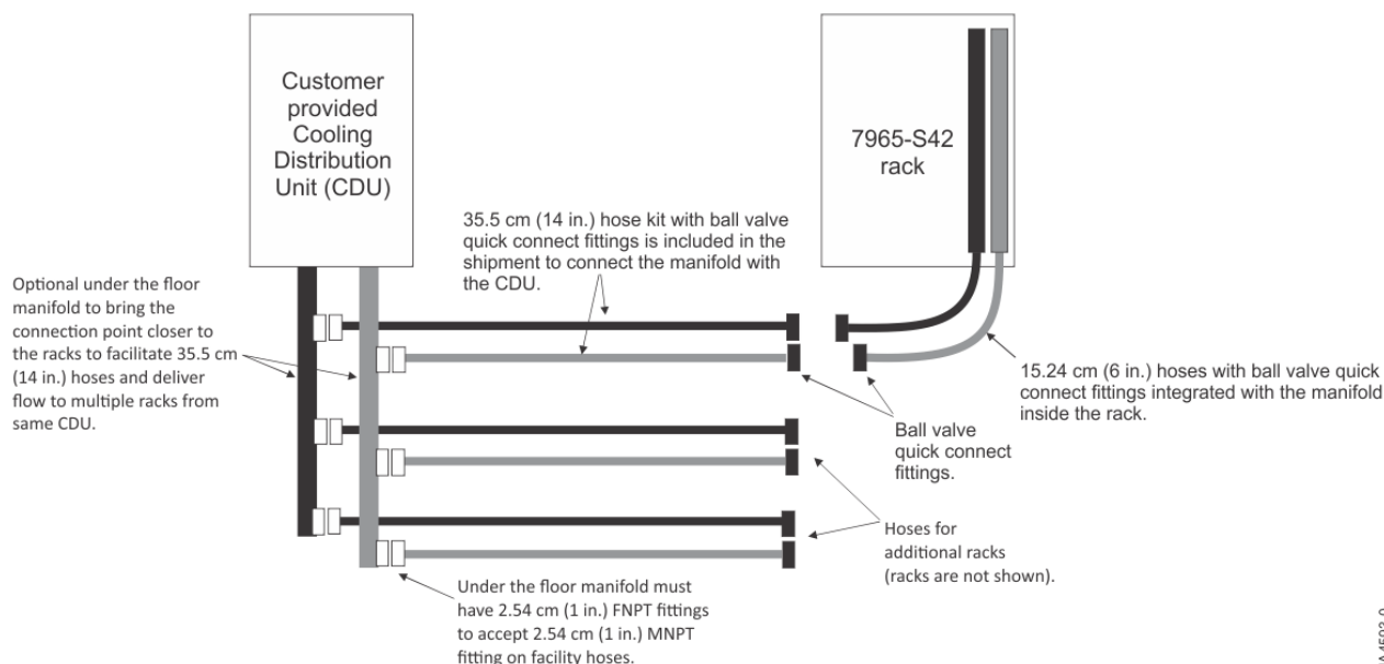
Figura 41. Schemă CDU cu furtunurile rețelei de apă ce se conectează la un colector de sub podea
