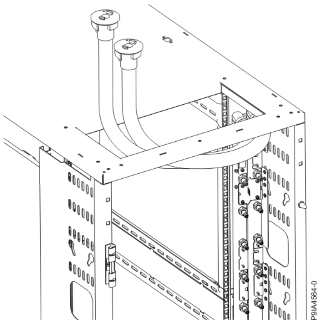
Figura 19. Locații de ieșire furtunuri în partea de sus
