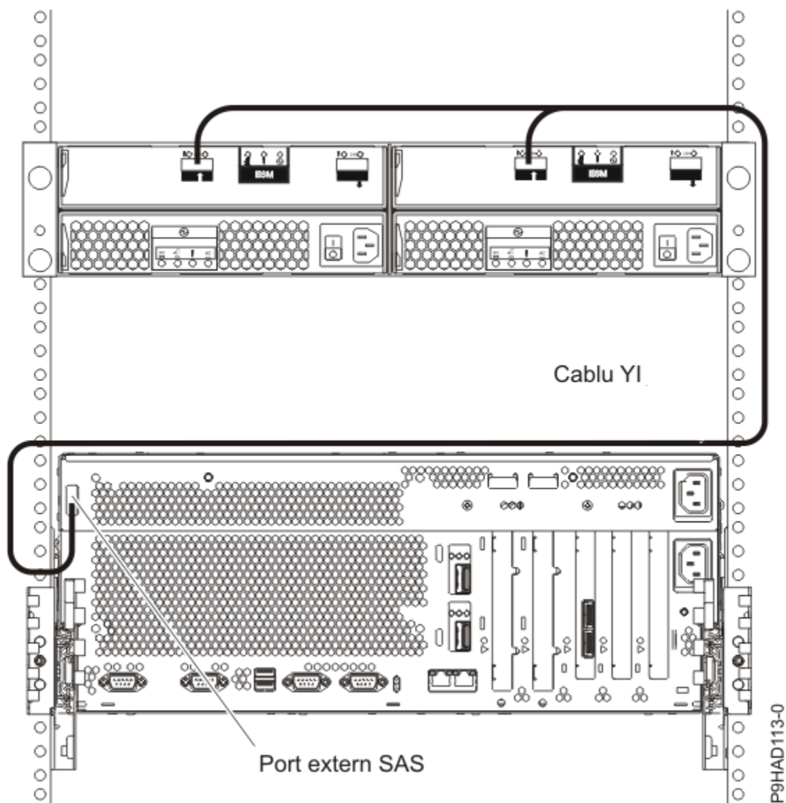
Figura 65. Port de adaptor SAS extern de sistem la un sertar de expansiune pentru discuri
