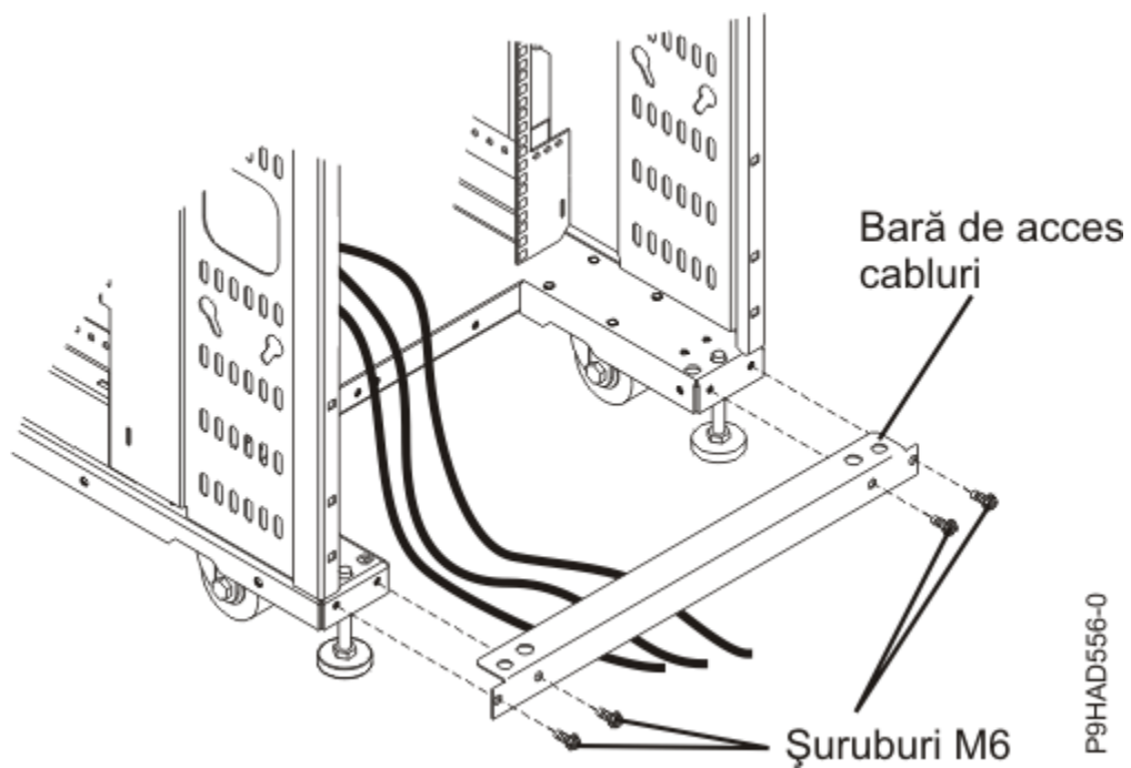
Figura 11. Bară de acces cabluri
