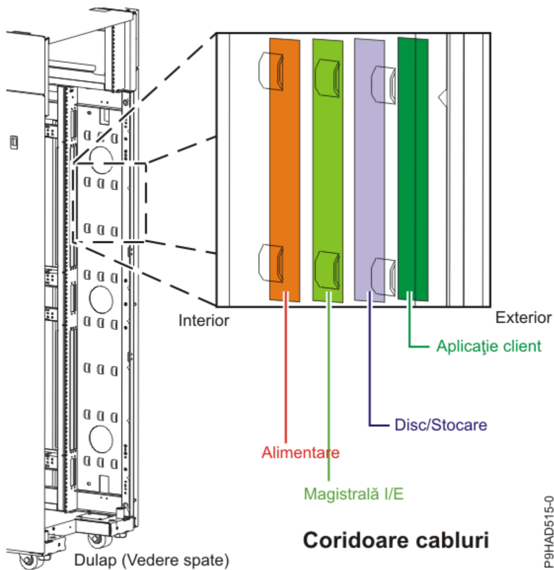
Figura 58. Clemele punții de pozare a cablurilor
