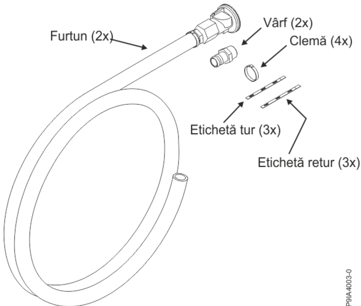
Figura 23. Kitul de furtun
