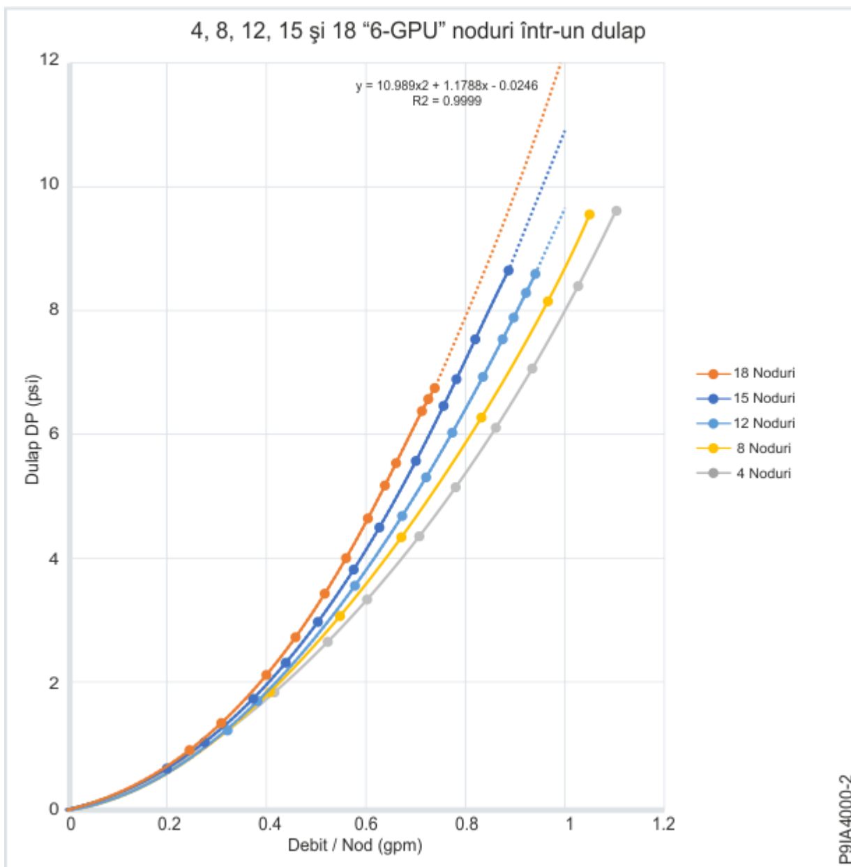
Figura 2. Debitul de apă în funcție de scăderea presiunii
