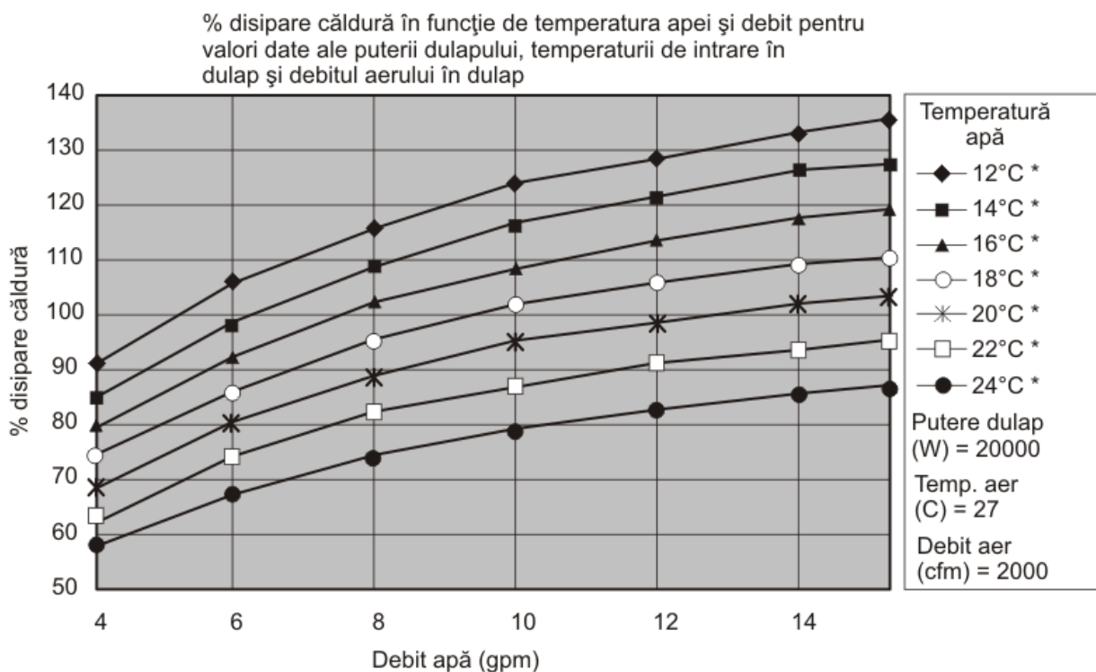
Figura 30. Performanța tipică a schimbătorului de căldură, 20 kW sarcină termică
