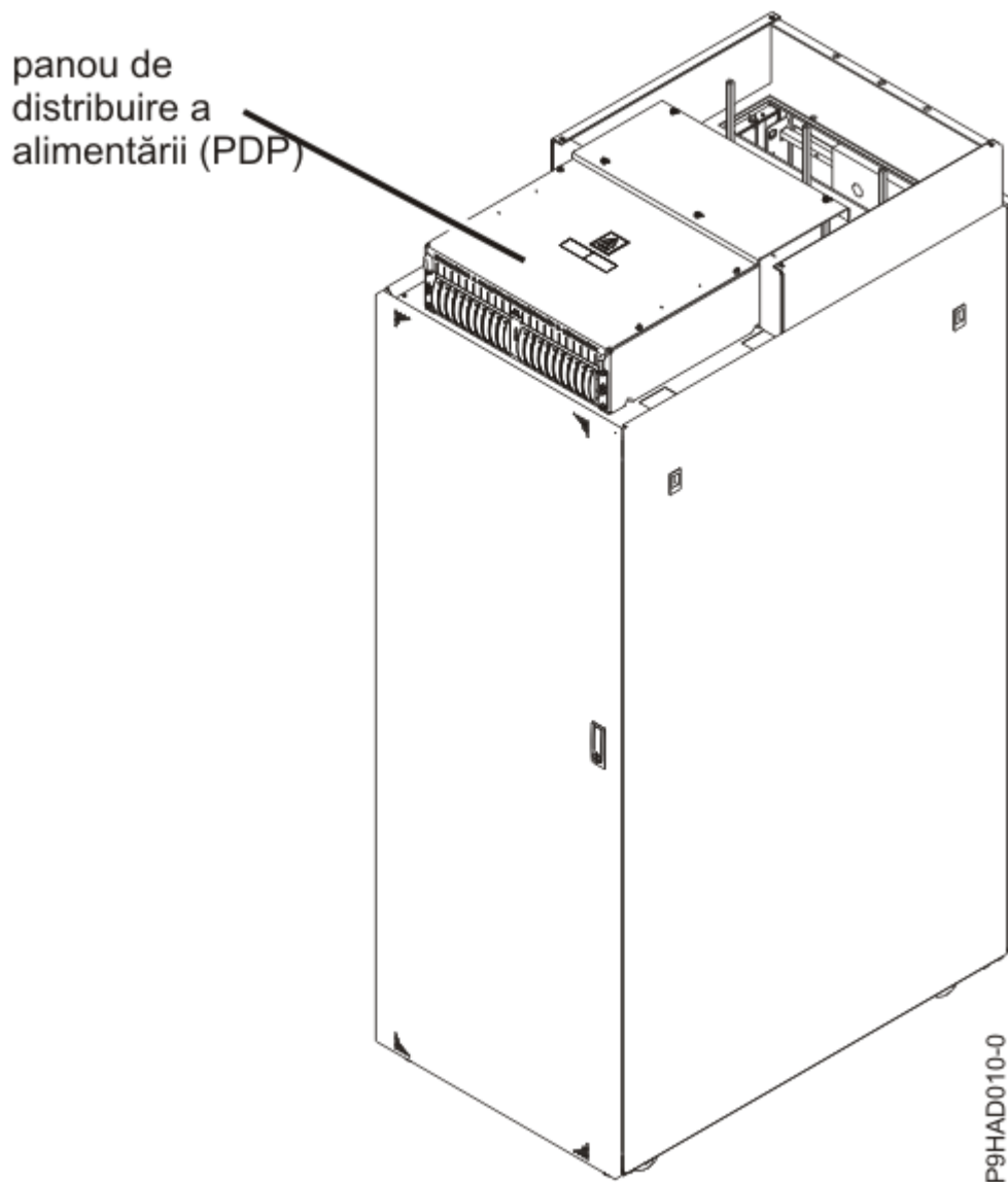
Figura 3. FC EPB8 - panou de distribuție a alimentării
