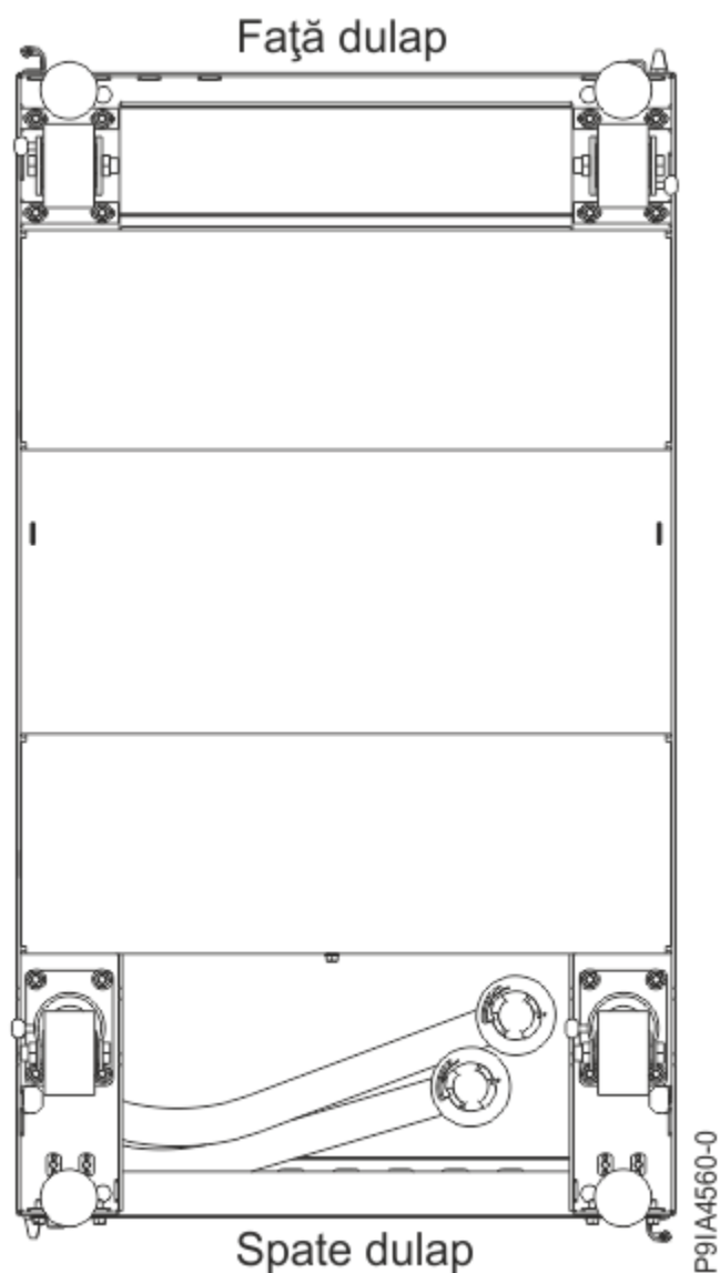
Figura 22. Locațiile de ieșire ale furtunului în partea de jos (vedere de jos)
