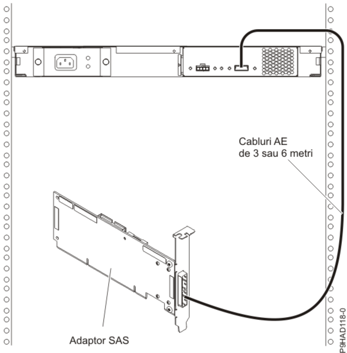
Figura 63. Adaptor SAS la un sertar de expansiune pentru medii
