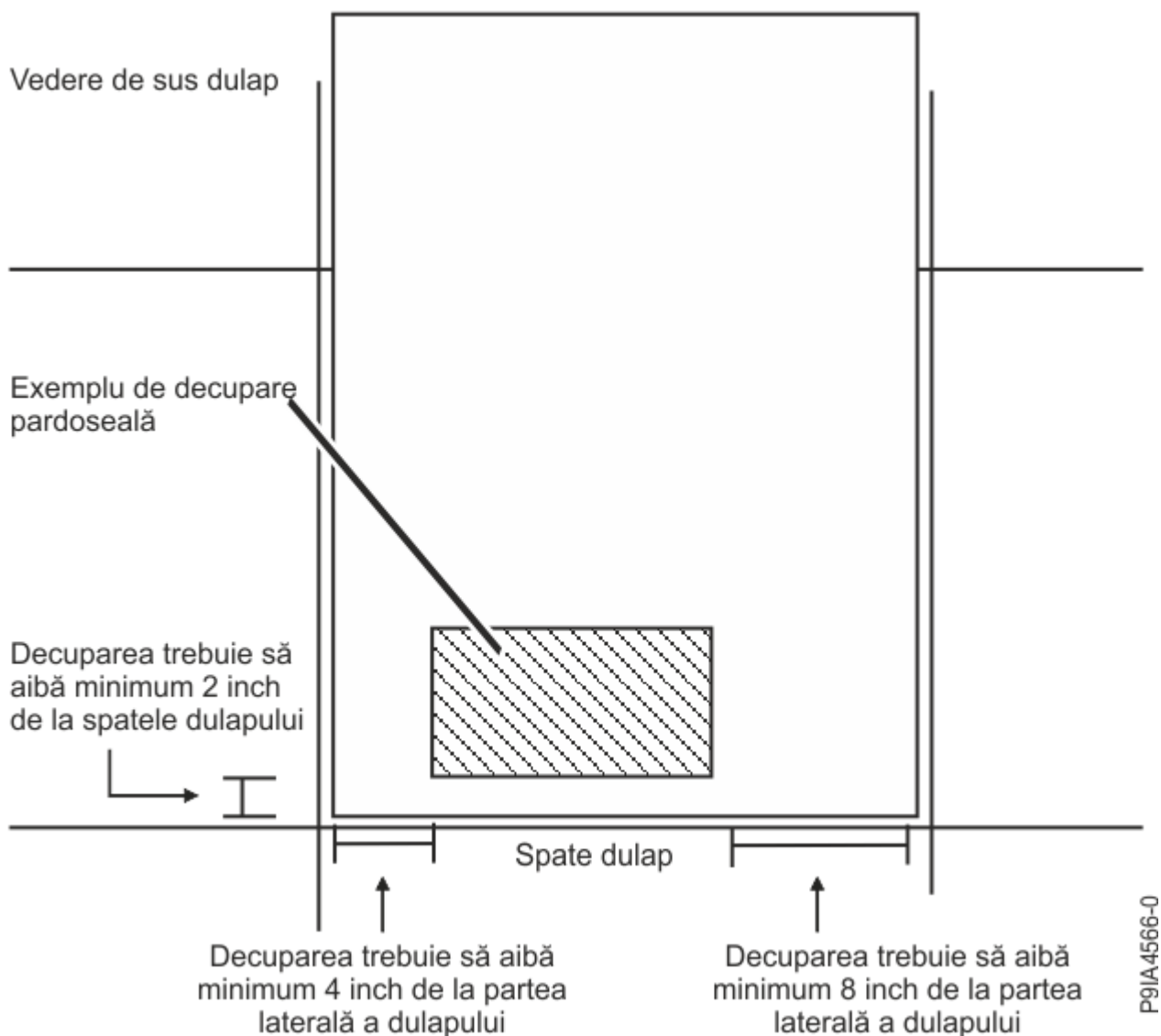
Figura 24. Decuparea în podea
