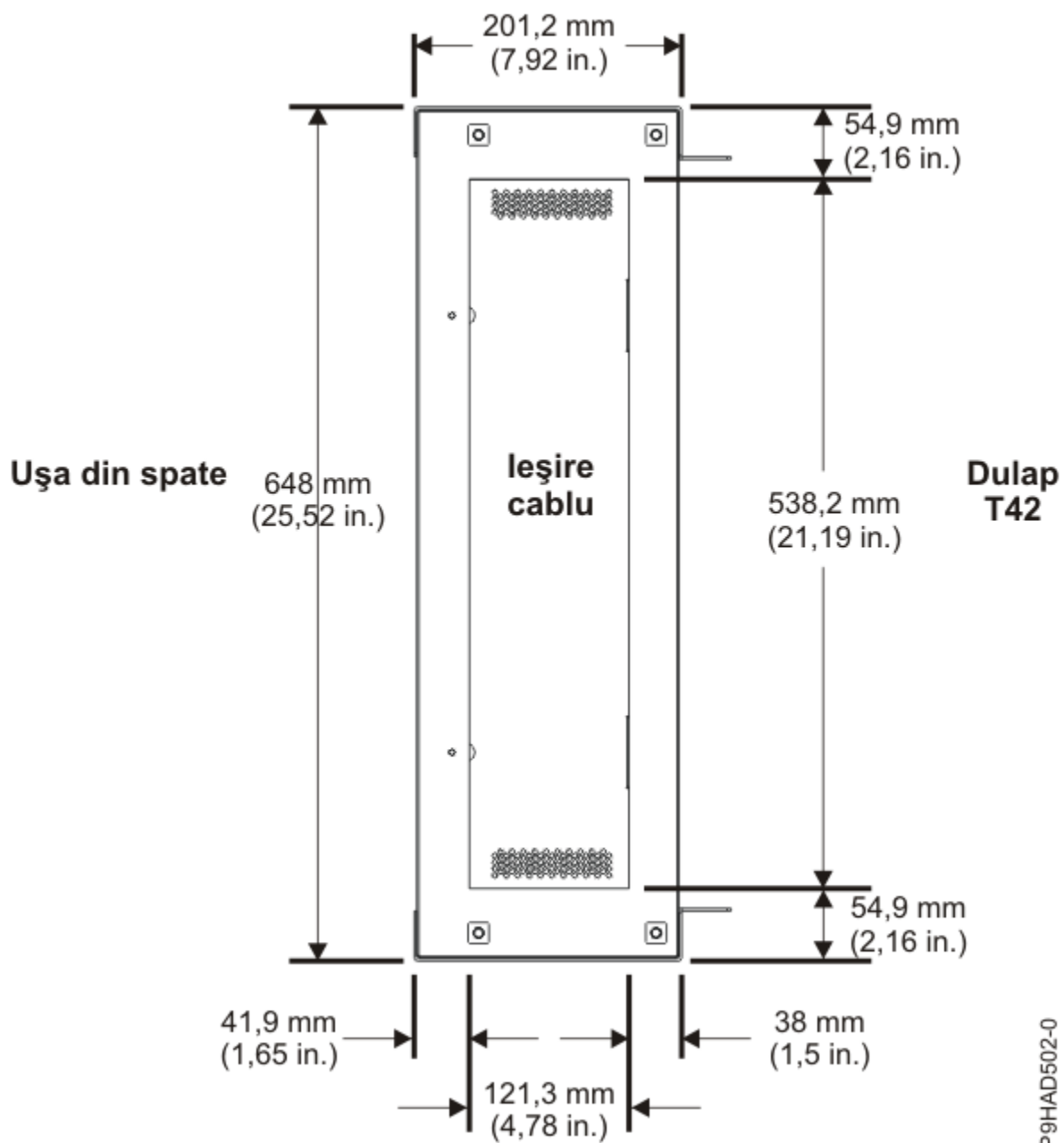
Figura 7. Extenderul de dulap spate FC ERG0 (vizualizare de sus în jos)
