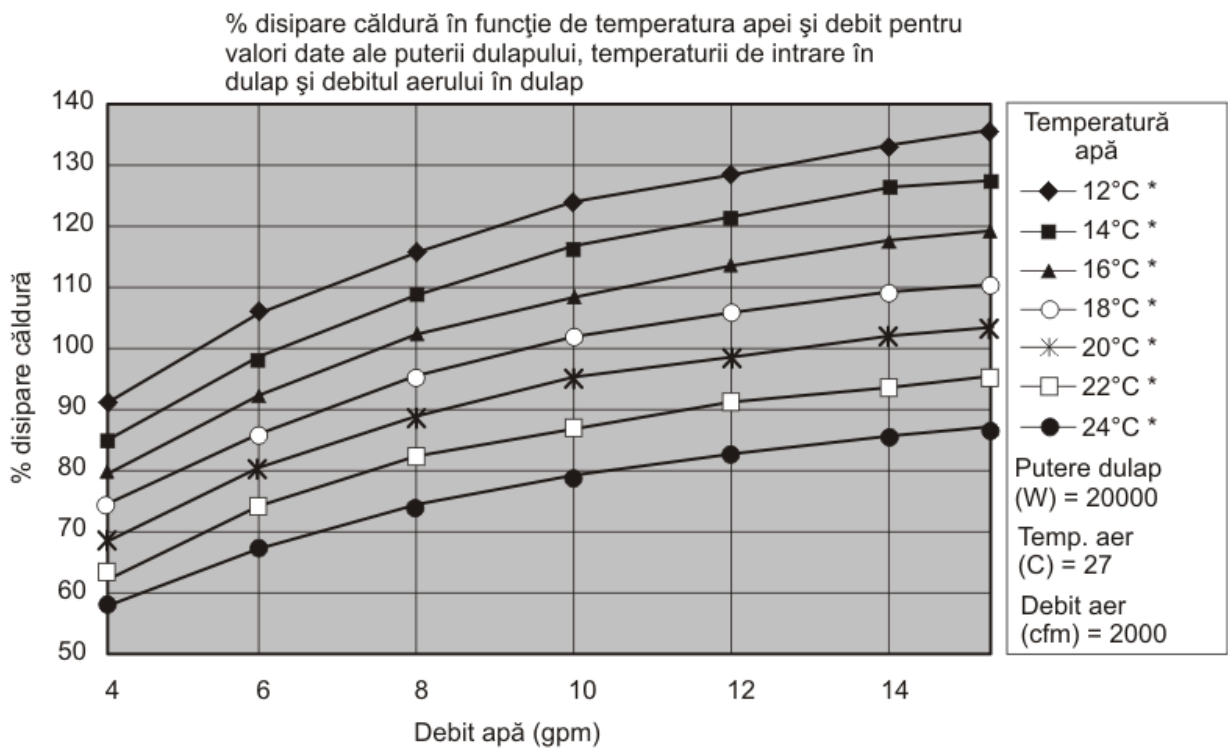
Figura 15. Performanța tipică a schimbătorului de căldură, 20 kW sarcină termică
