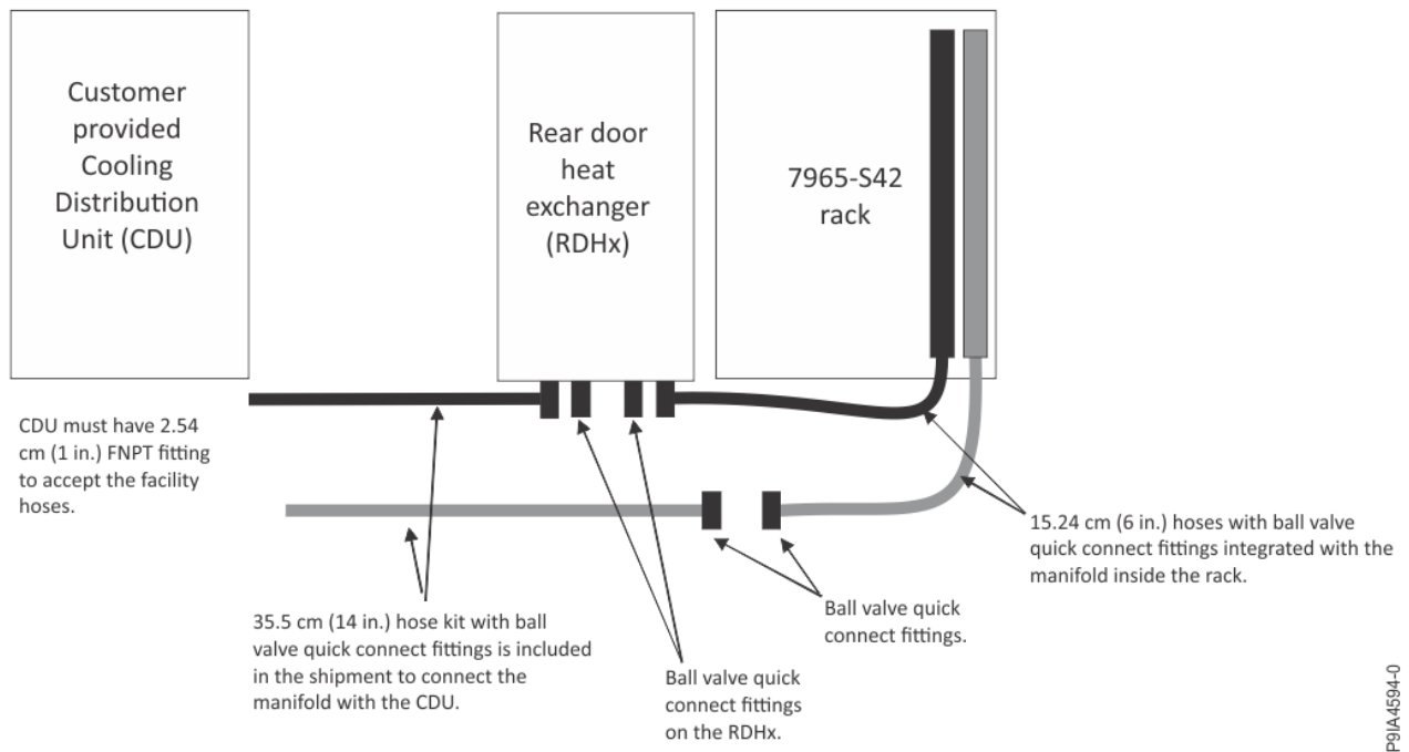
Figura 47. Schemă CDU cu furtunurile rețelei de apă pentru colector și RDHx ce se conectează direct la CDU
