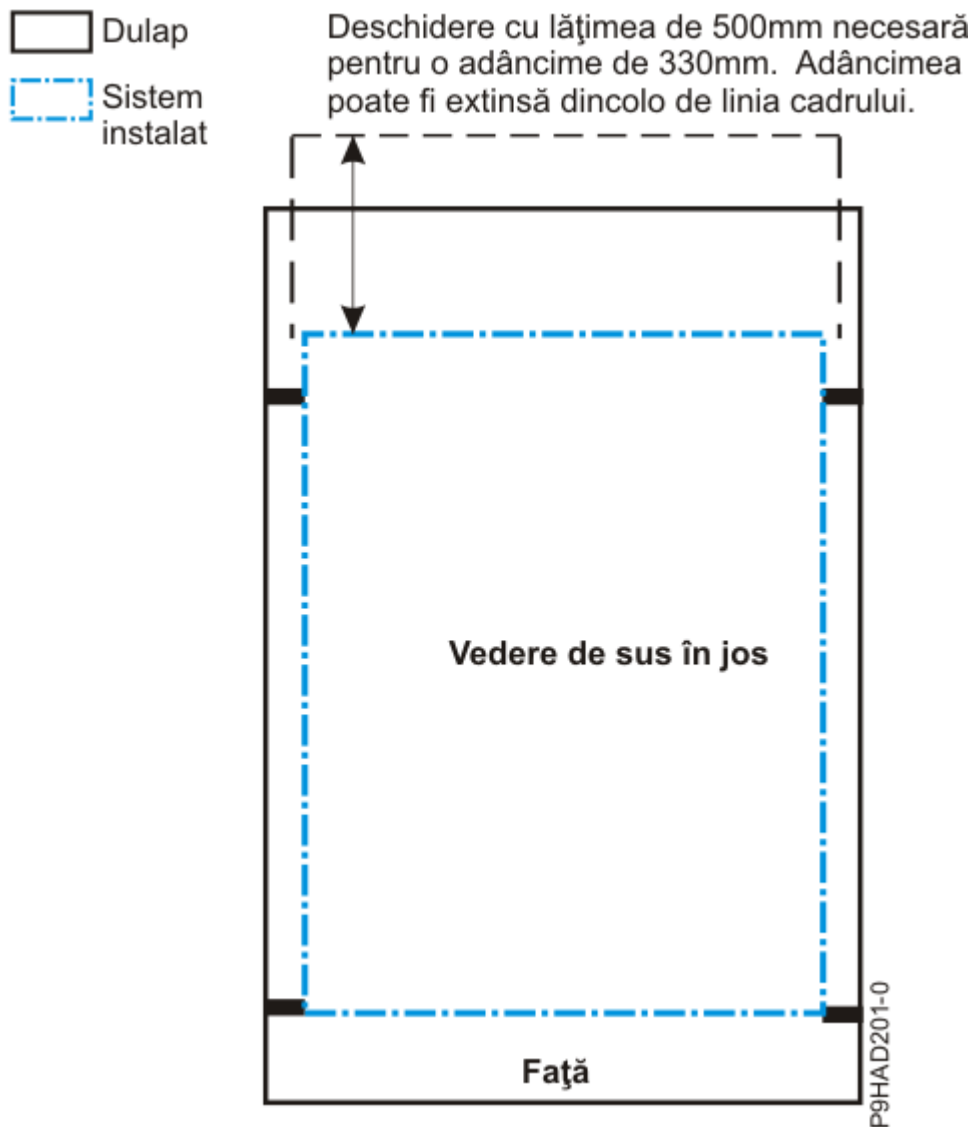
Figura 51. Dimensiuni de bordură de montare critice
