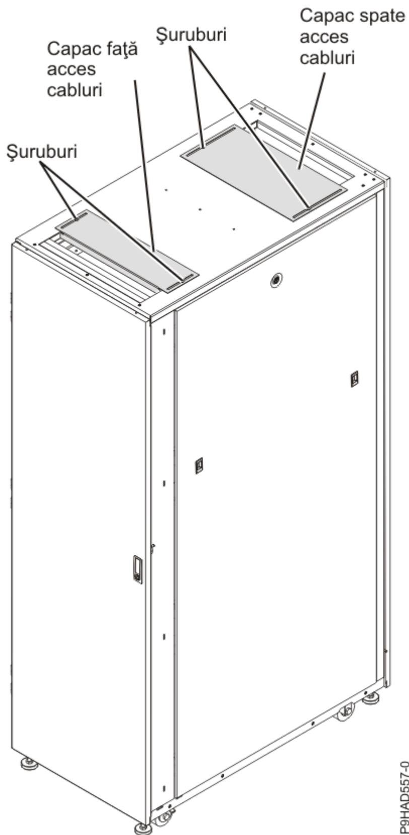
Figura 12. Capace de acces cabluri
