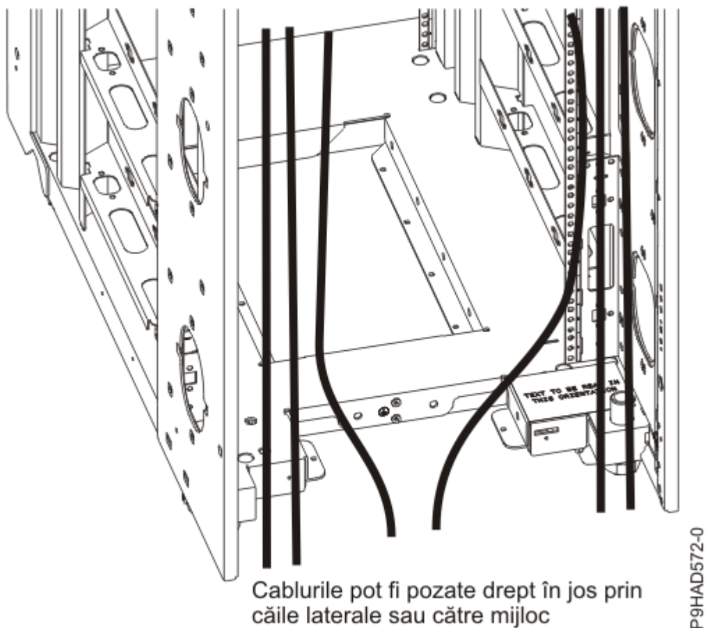
Figura 27. Cablarea sub podea
