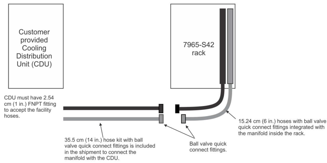
Figura 40. Schemă CDU cu furtunurile rețelei de apă ce se conectează direct la CDU
