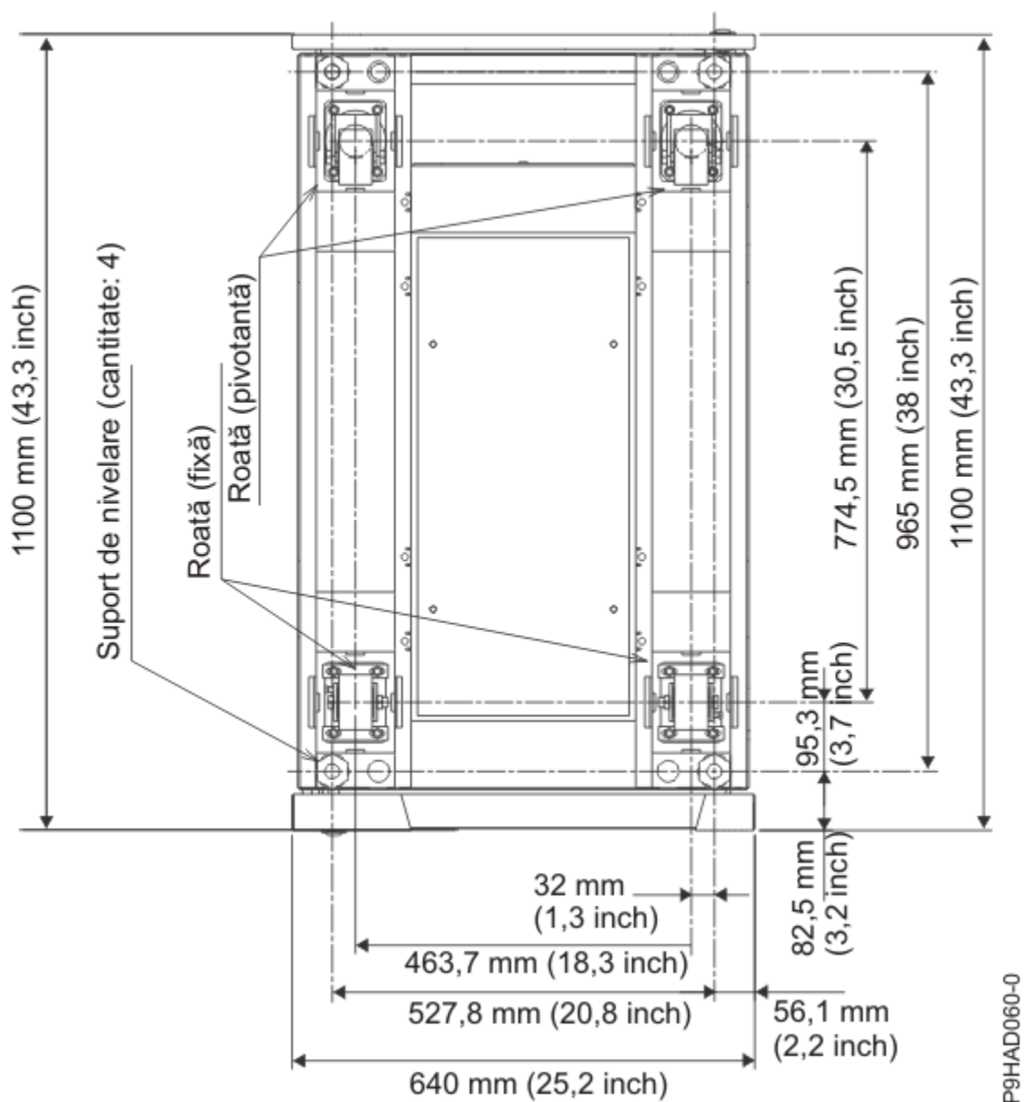
Figura 6. Locațiile roților și nivelatoarelor
