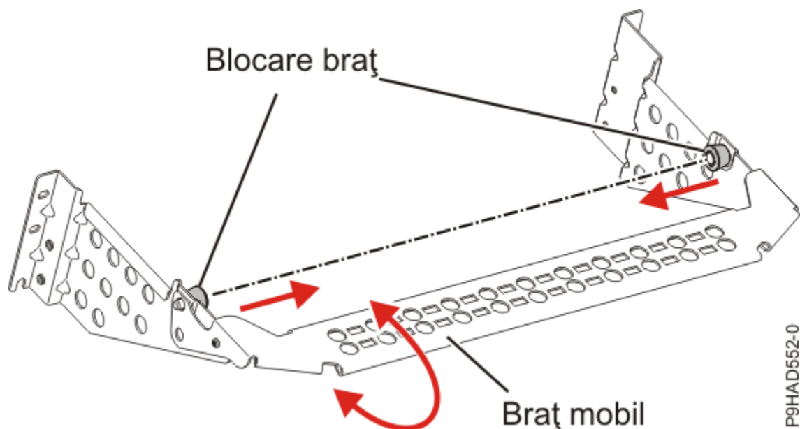
Figura 60. Colțar pentru pozarea cablurilor
