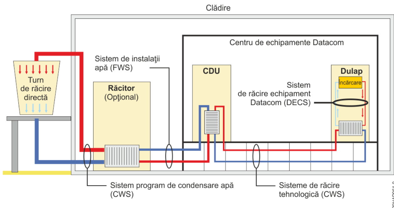
Figura 84. Exemplu de bucle și sisteme de răcire cu lichid într-un centru de date
