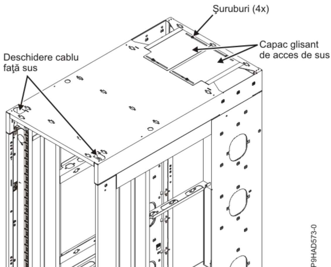
Figura 28. Pozare cablare
