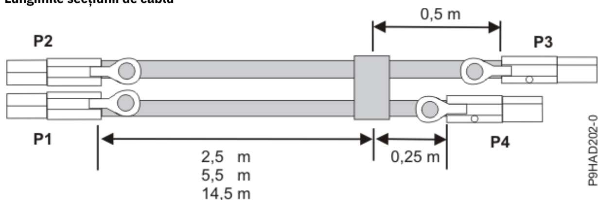
Figura 61. Lungimile de cablu pentru ansamblul cablu X extern SAS
