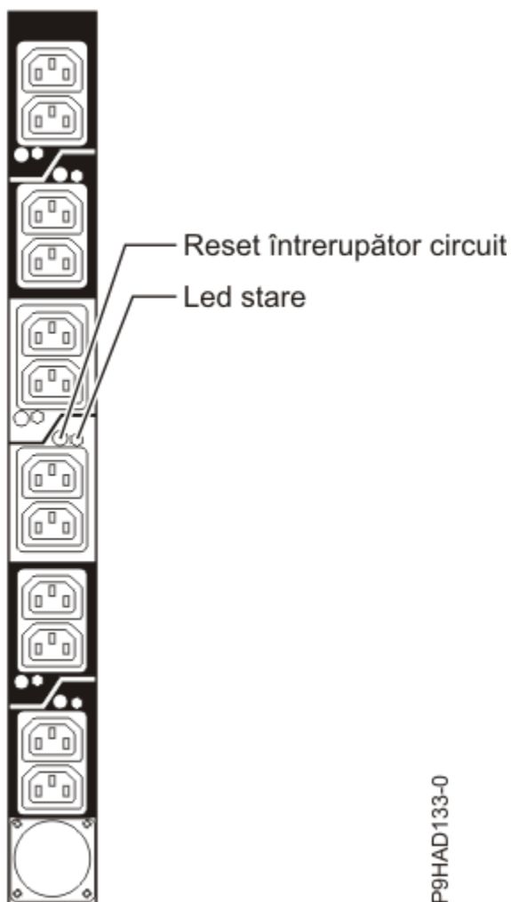
Figura 55. Desen priză PDU
