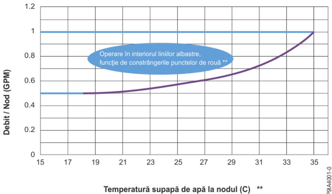
Figura 1. Debitul de apă în funcție de temperatură
