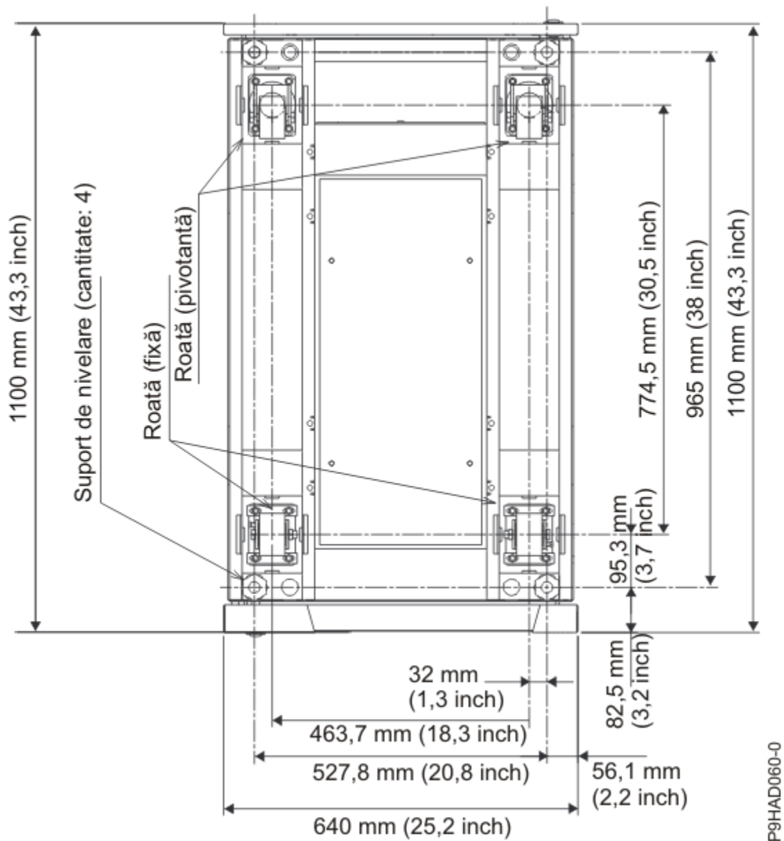
Figura 5. Locațiile roților și nivelatoarelor
