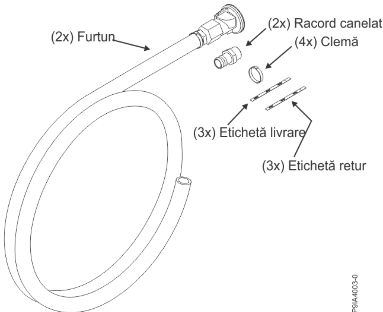
Figura 26. Kit furtun
