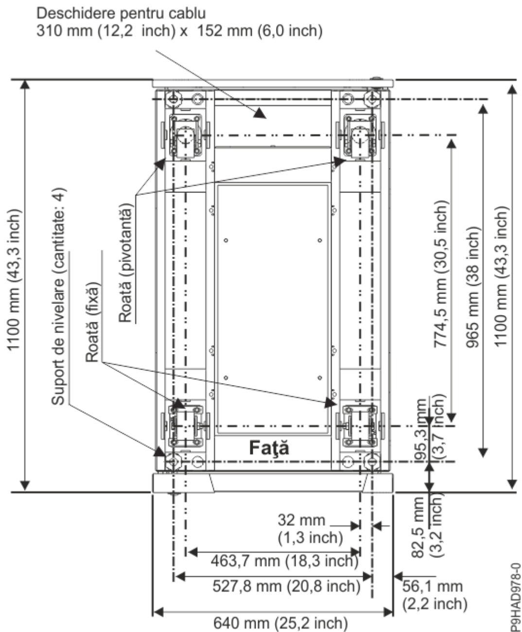
Figura 4. Locațiile roților și nivelatoarelor
