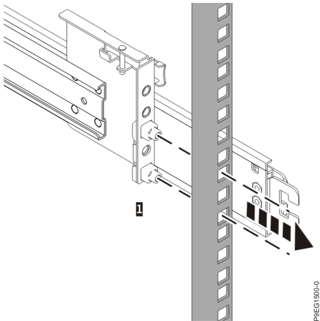
Figura 2. Aliniați capătul șinei din stânga la spatele dulapului
