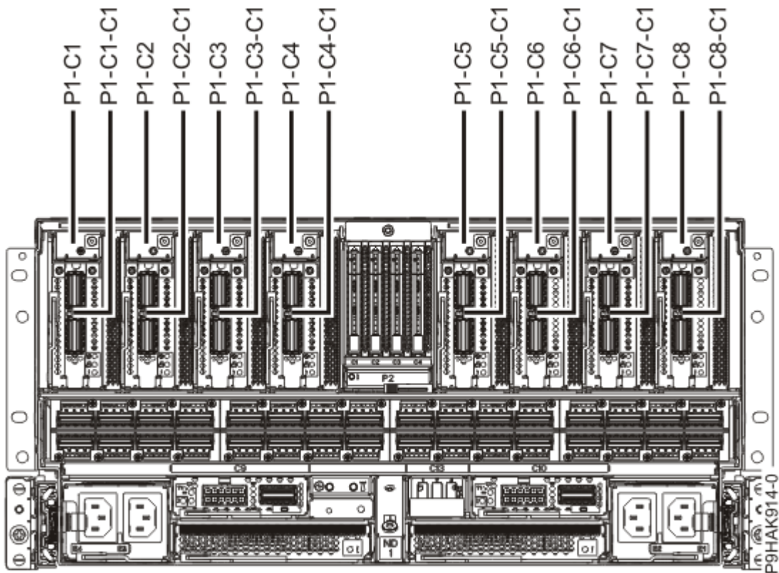
Figura 1. Vedere din spate a sistemului 9080-M9S montat în dulap, cu codurile de locație ale sloturilor PCIe Tabela 2 la pagina 2 listează locațiile de sloturi DE adaptor și detalii pentru sistemele 9080-M9S.
