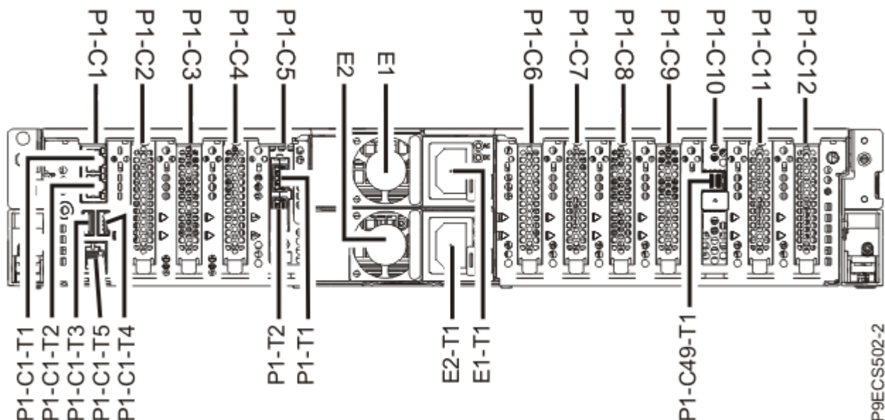
Figura 2. Vederea din spate a unui sistem montat în dulap 9008-22L, 9009-22A sau 9223-22H cu codurile de locație pentru sloturile PCIe
