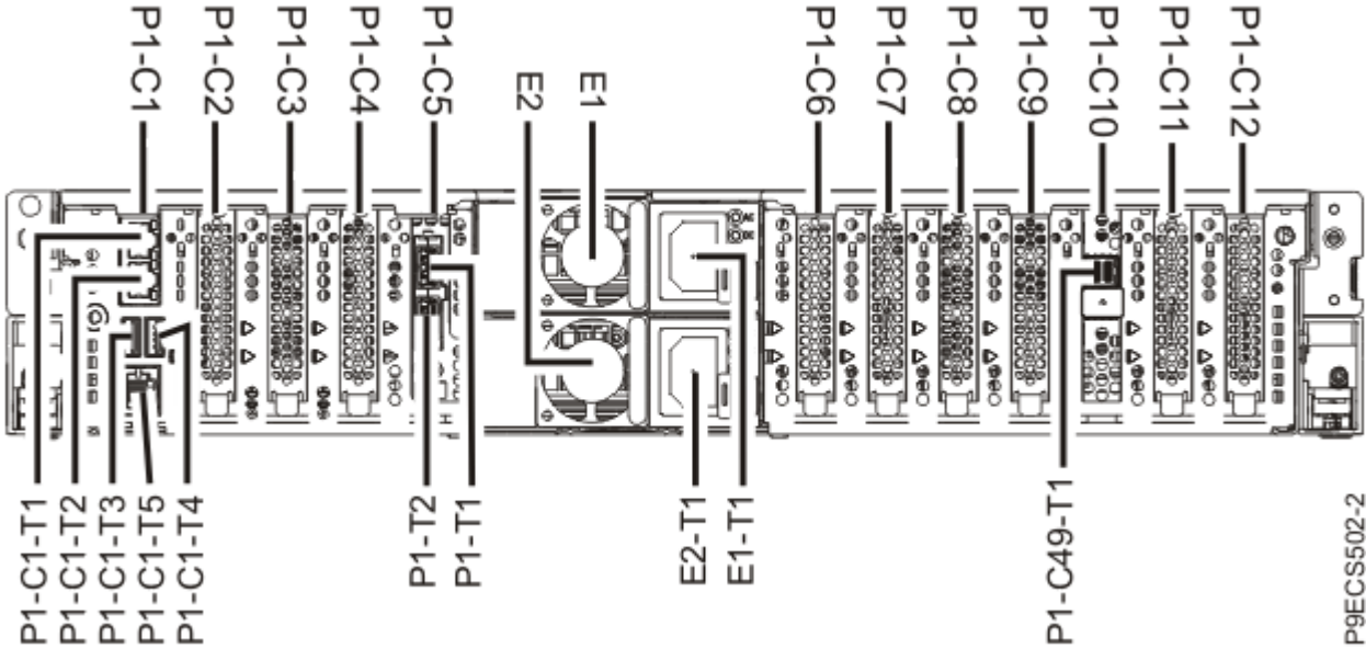
Figura 1. Vederea din spate a unui sistem montat în dulap 5105-22E, 9009-22G sau 9223-22S cu codurile de locație pentru sloturile PCIe4
