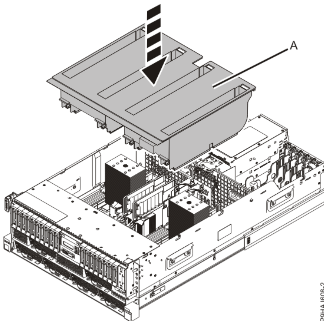
Figura 33. Substituir a conduta de ventilação num sistema montado em bastidor
