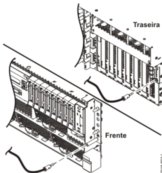
Figura 23. Localização das tomadas ESD
