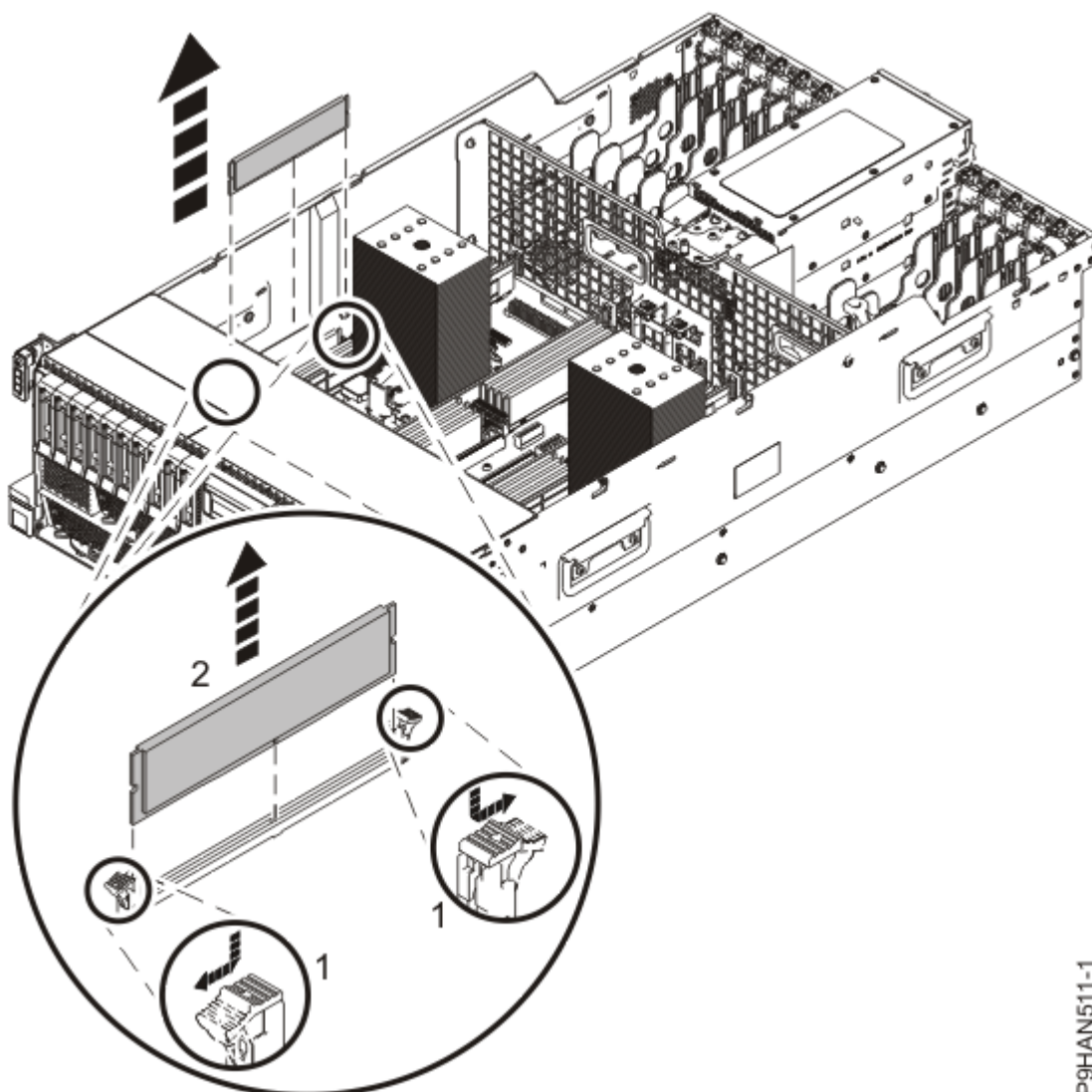
Figura 31. Remover um módulo de memória
