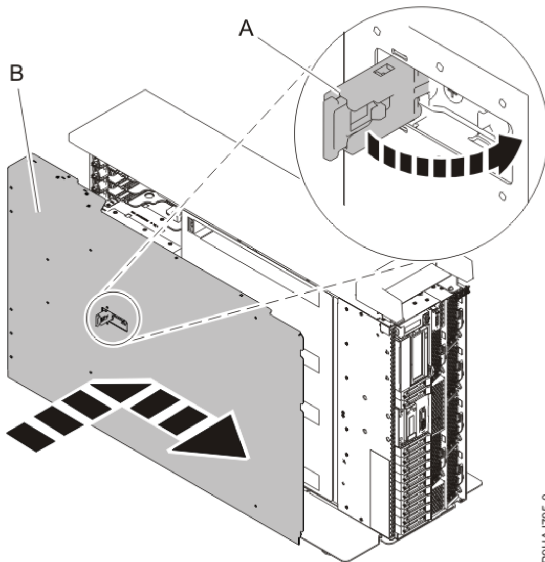
Figura 36. Instalar a tampa de acesso a assistência
