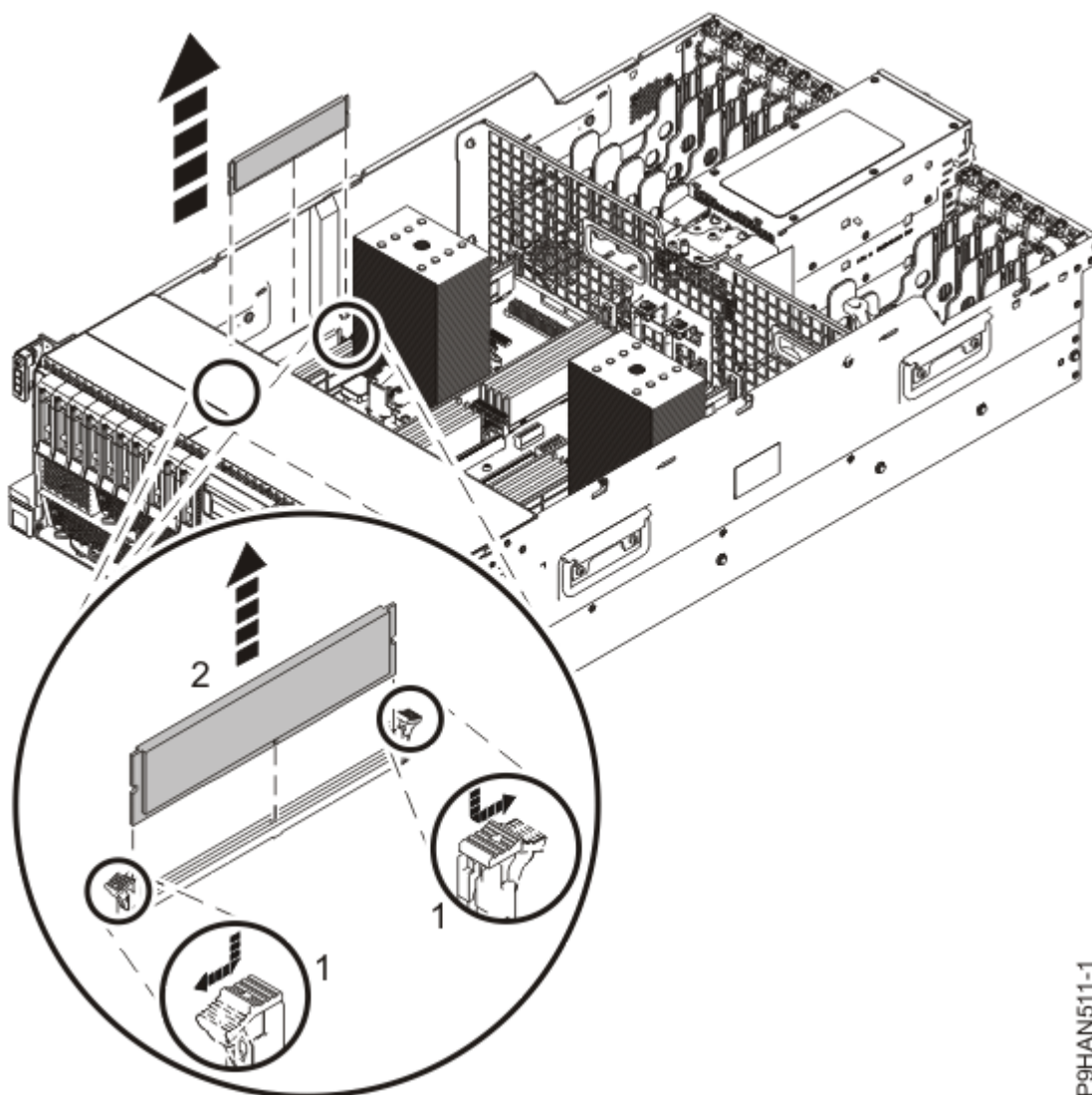
Figura 51. Remover um módulo de memória
