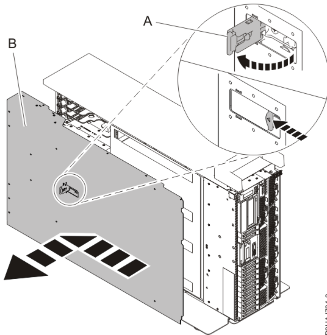
Figura 25. Remover a tampa de acesso para assistência
