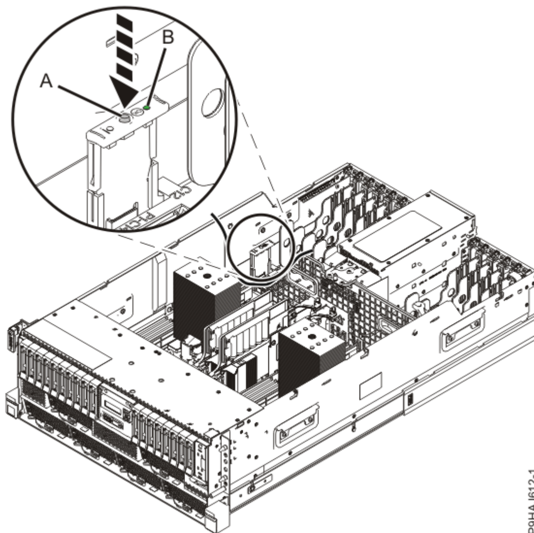
Figura 26. Activar o LED de identificação para um sistema montado em bastidor
