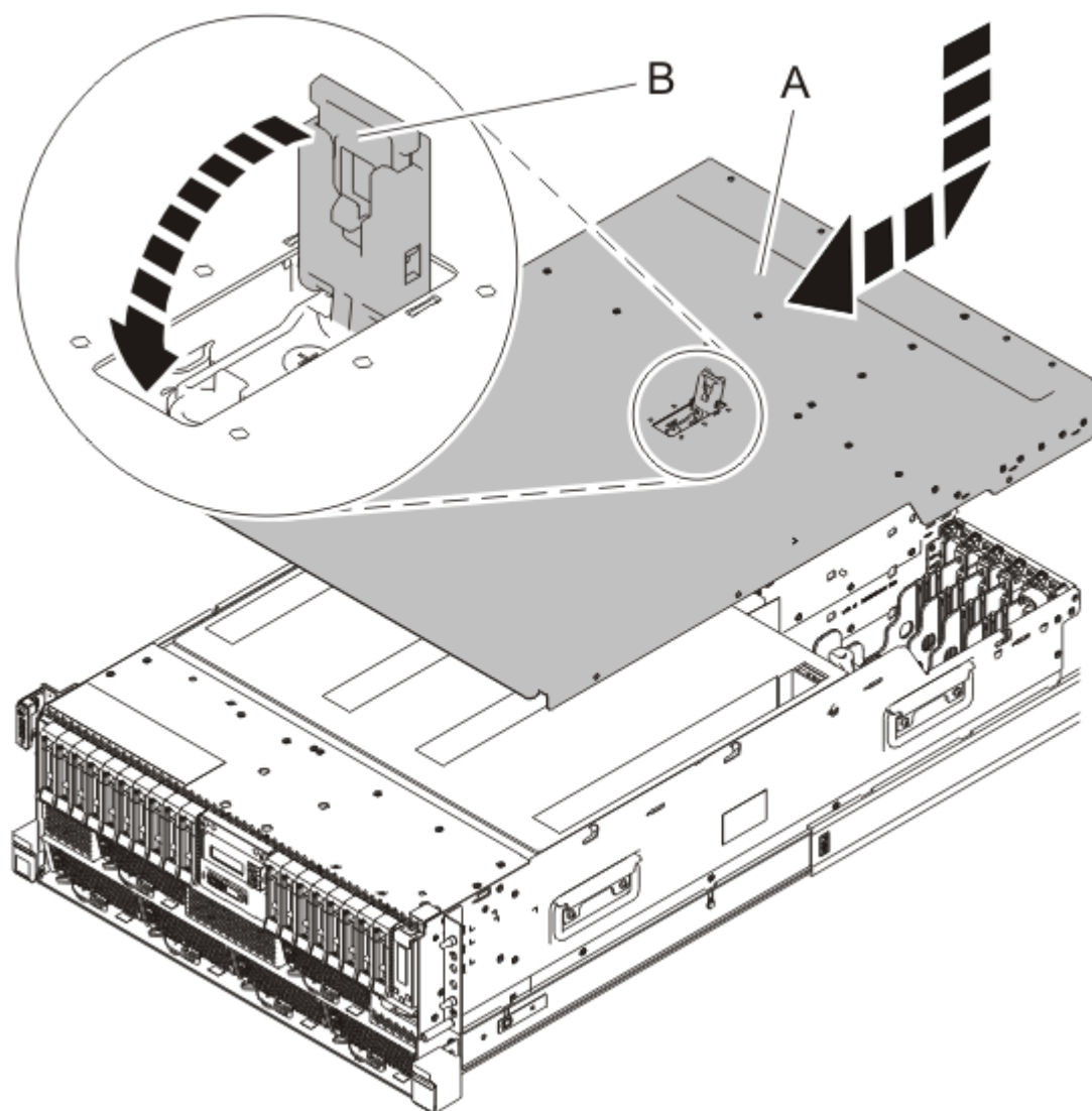
Figura 35. Instalar a tampa de acesso a assistência
