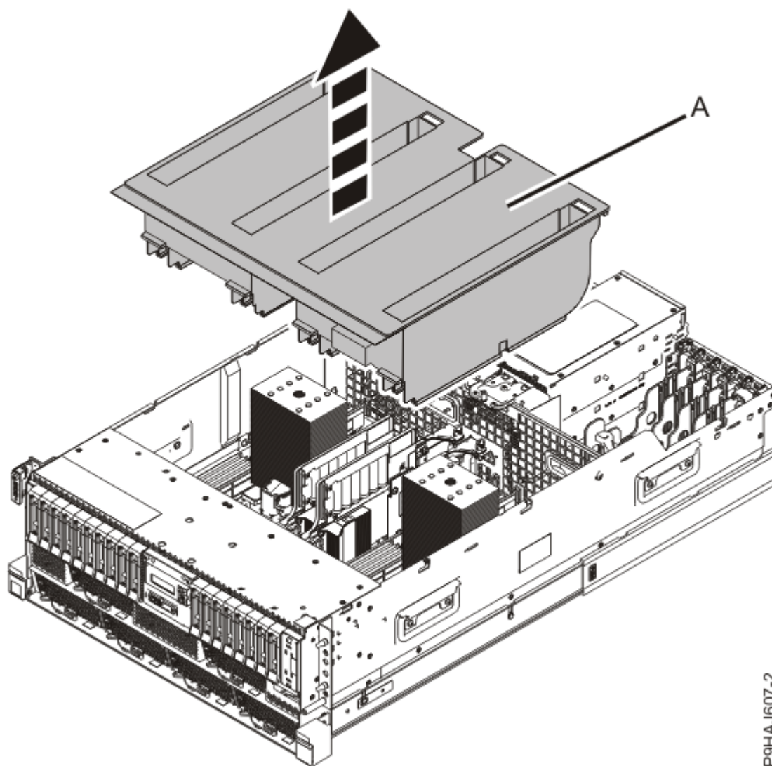
Figura 49. Remover a conduta de ventilação de um sistema montado em bastidor
