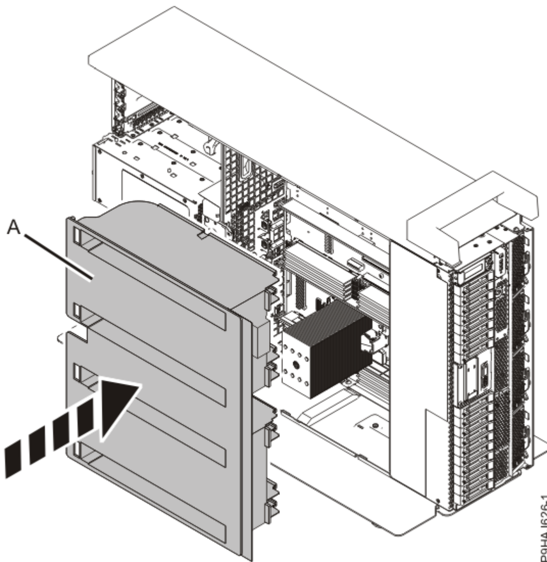
Figura 34. Substituir a conduta de ventilação num sistema autónomo
