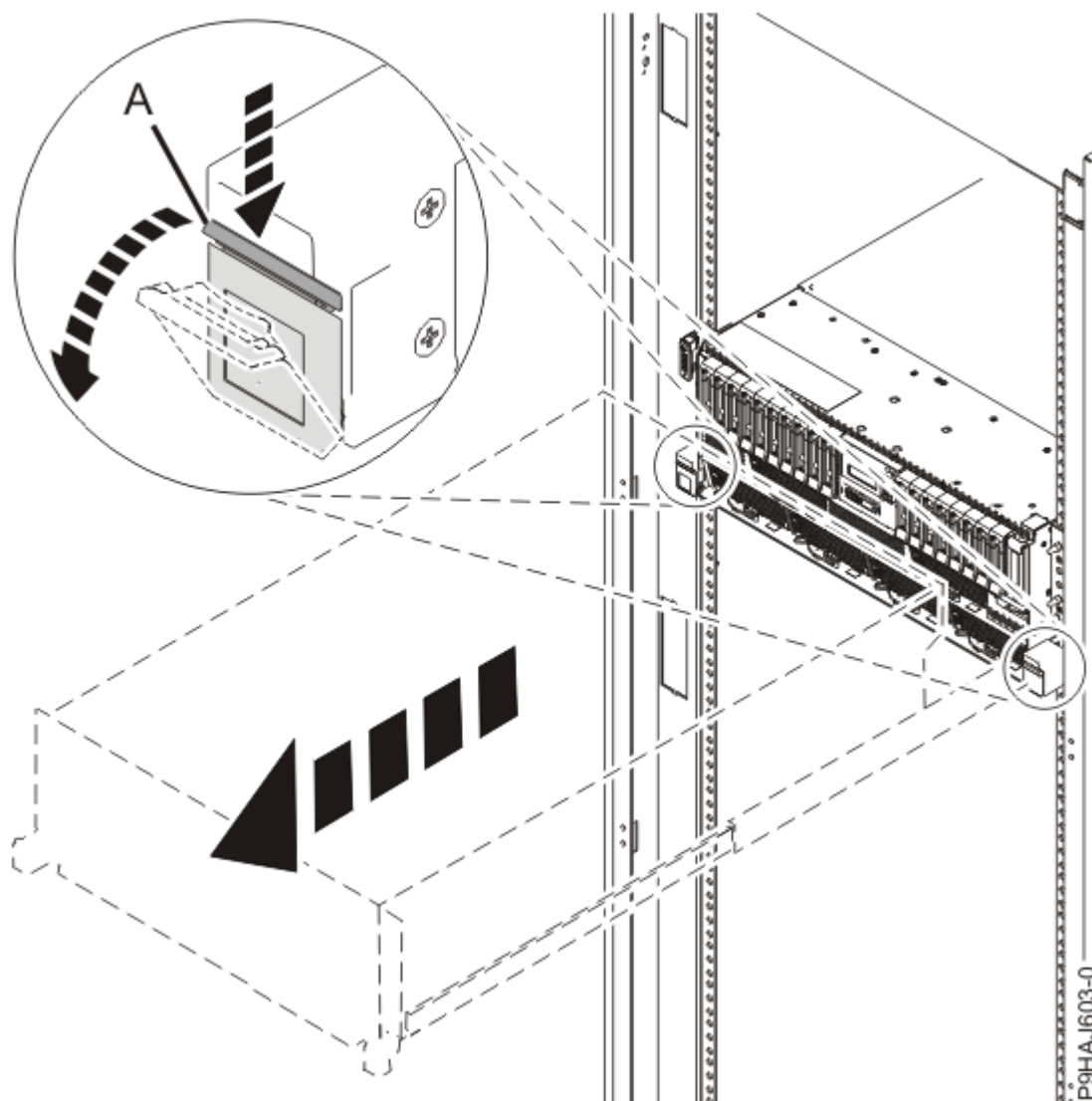
Figura 45. Soltar as patilhas laterais
