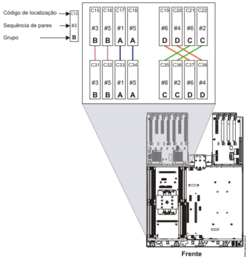
Figura 40. Sequência de ligação, um processador do sistema, sistema montado em bastidor
