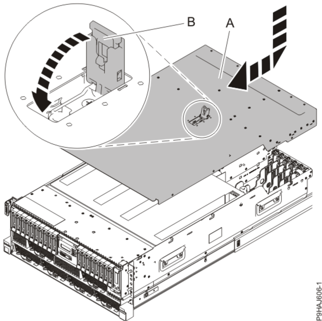
Figura 54. Instalar a tampa de acesso a assistência
