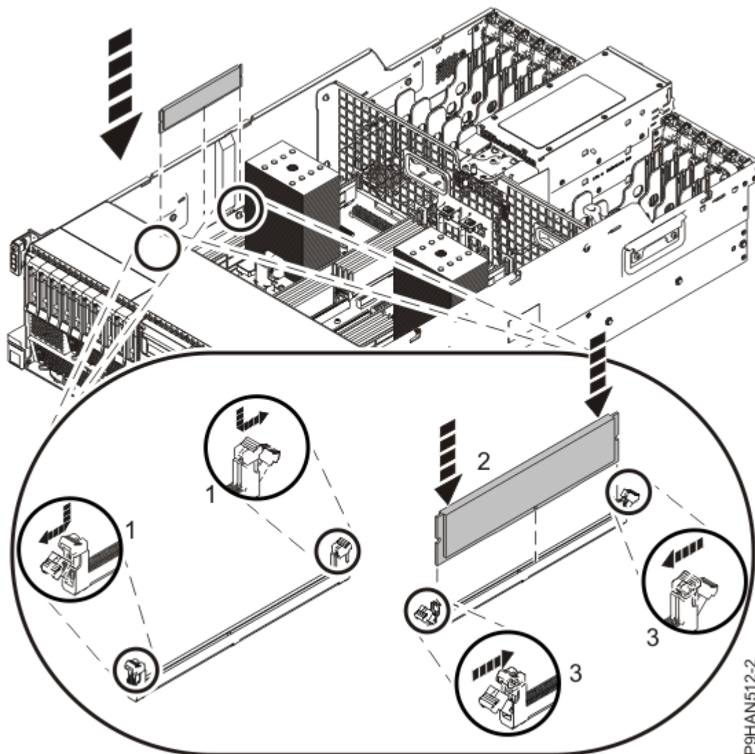
Figura 12. Instalar um módulo de memória
