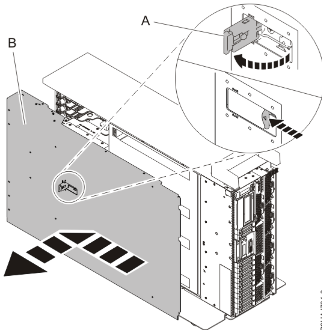
Figura 48. Remover a tampa de acesso para assistência
