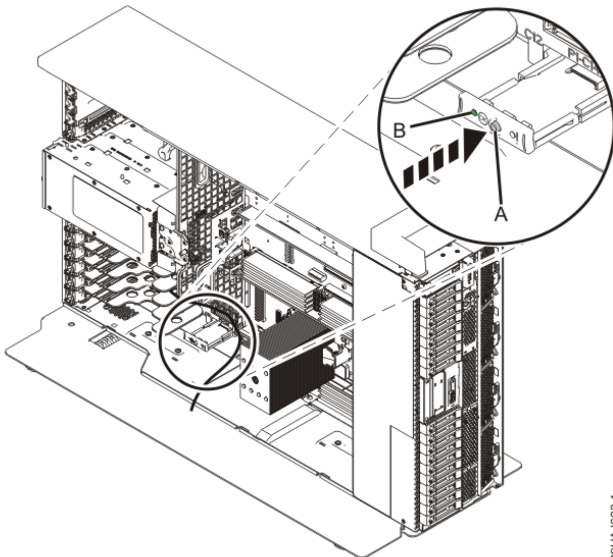
Figura 27. Activar o LED de identificação para um sistema autónomo
