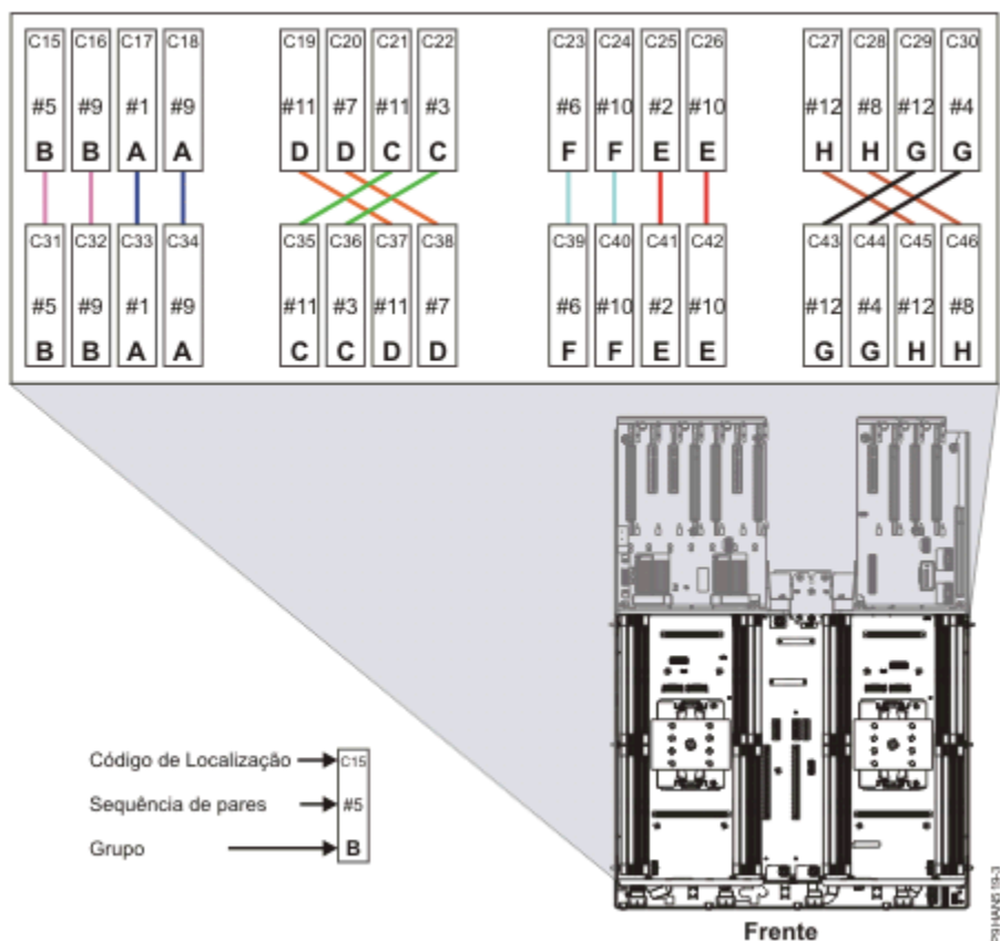
Figura 42. Sequência de ligação, dois processadores de sistema
