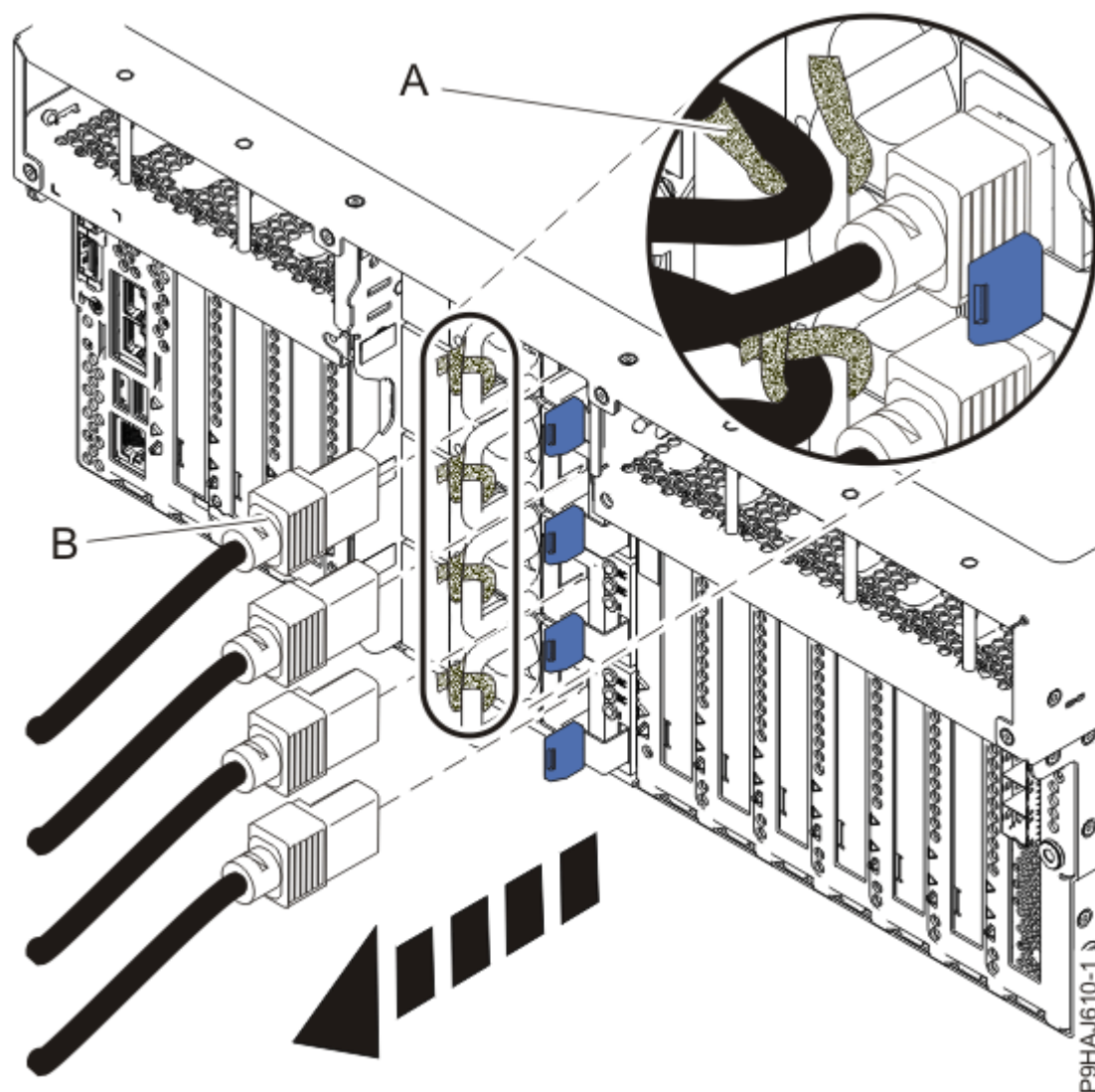
Figura 43. Remover os cabos de alimentação de um servidor instalado em bastidor
