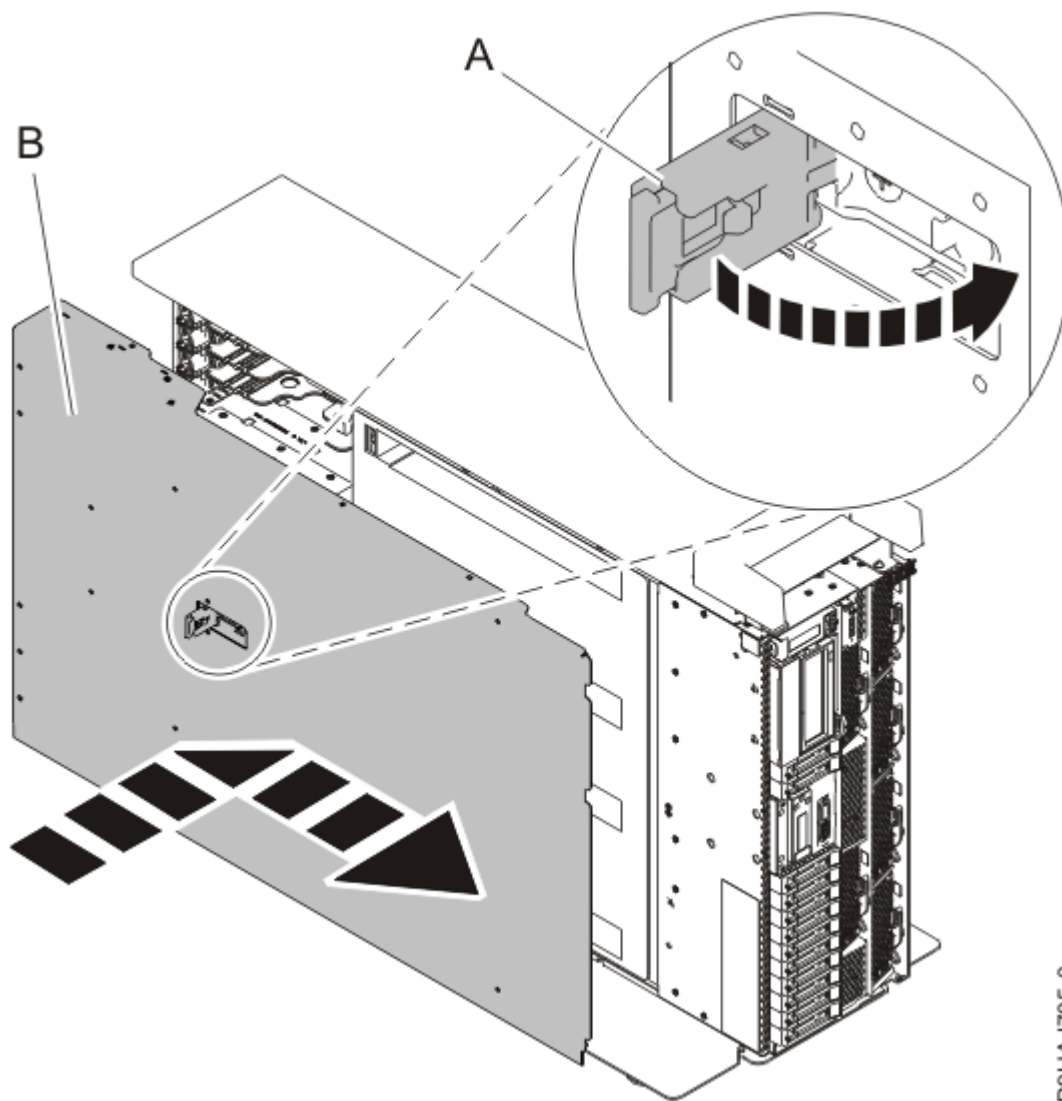
Figura 16. Instalar a tampa de acesso a assistência
