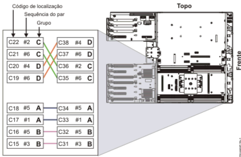
Figura 41. Sequência de ligação, um processador do sistema, sistema autónomo
