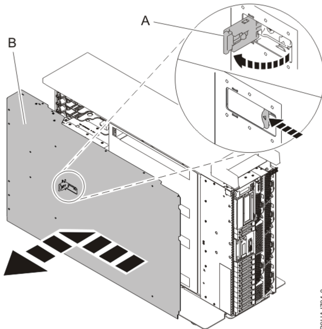
Figura 9. Remover a tampa de acesso para assistência
