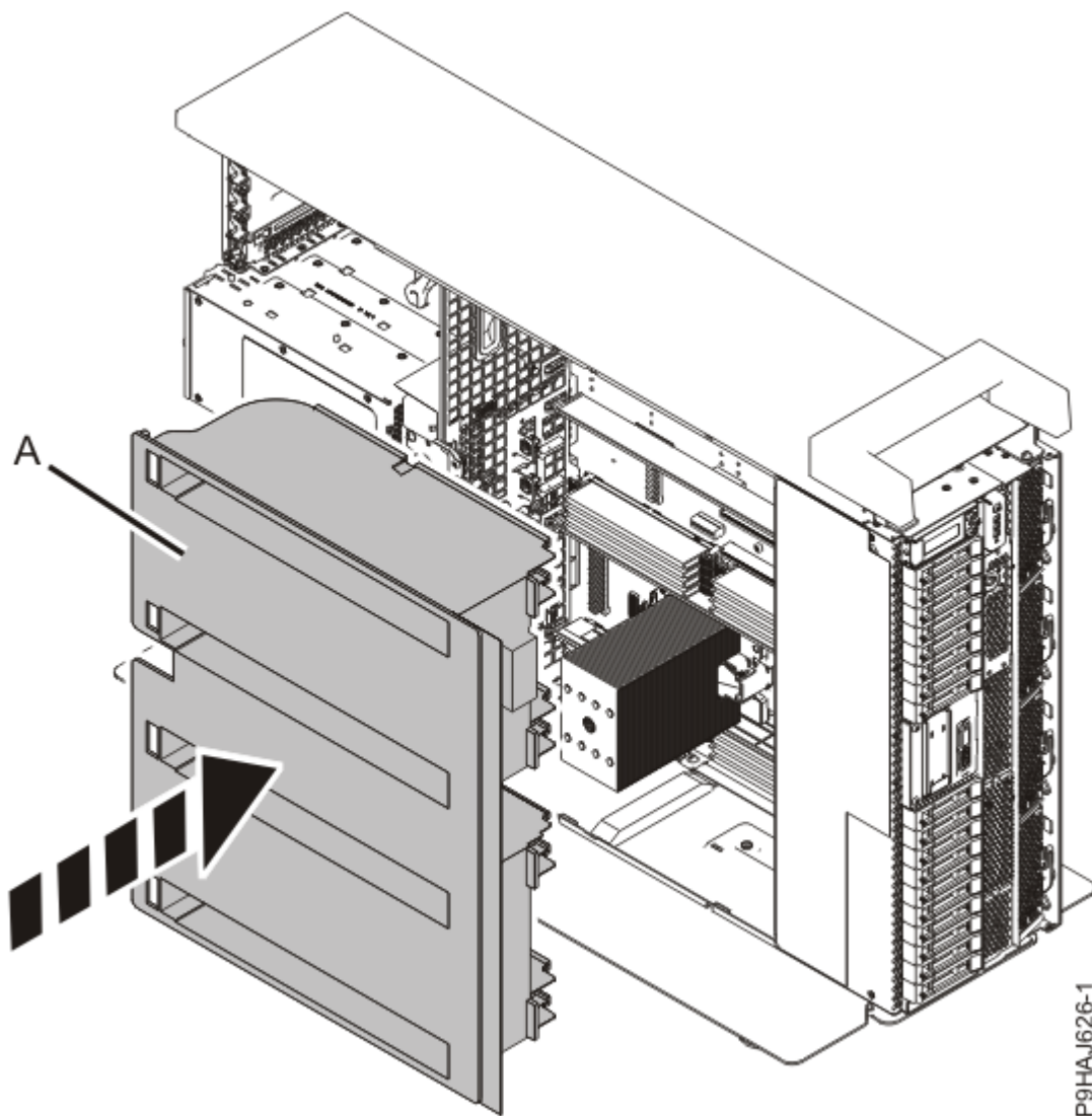
Figura 53. Substituir a conduta de ventilação num sistema autónomo
