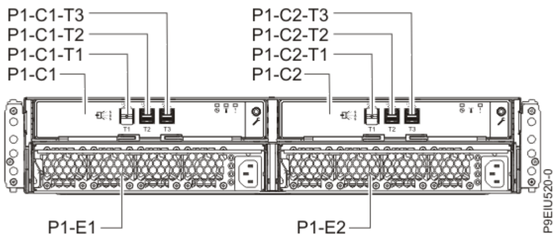
Figura 3. Vista posterior das unidades de expansão
