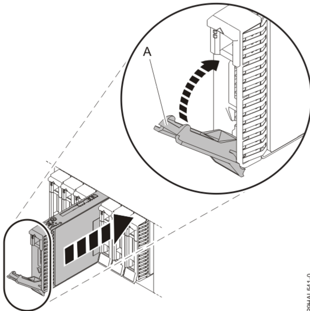
Figura 20. Instalar uma unidade num sistema
