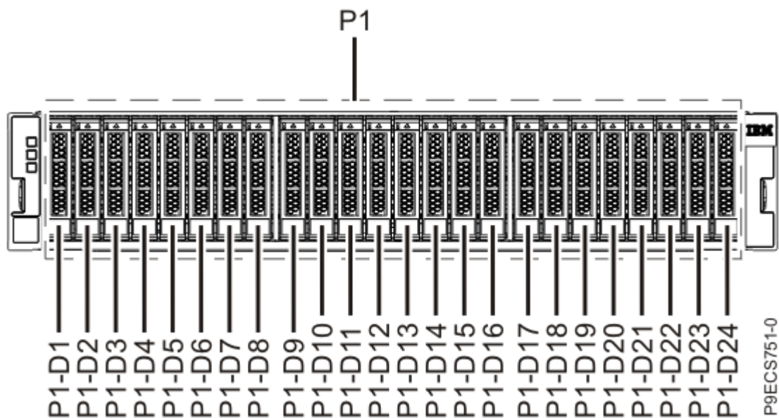
Figura 2. Vista anterior da unidade de expansão ESLS que mostra as localizações das unidade
