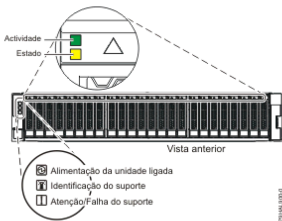
Figura 12. Vista anterior da unidade de expansão que mostra os indicadores de assistência
