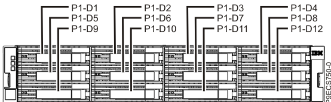
Figura 1. Vista anterior da unidade de expansão ESLL que mostra as localizações das unidade
