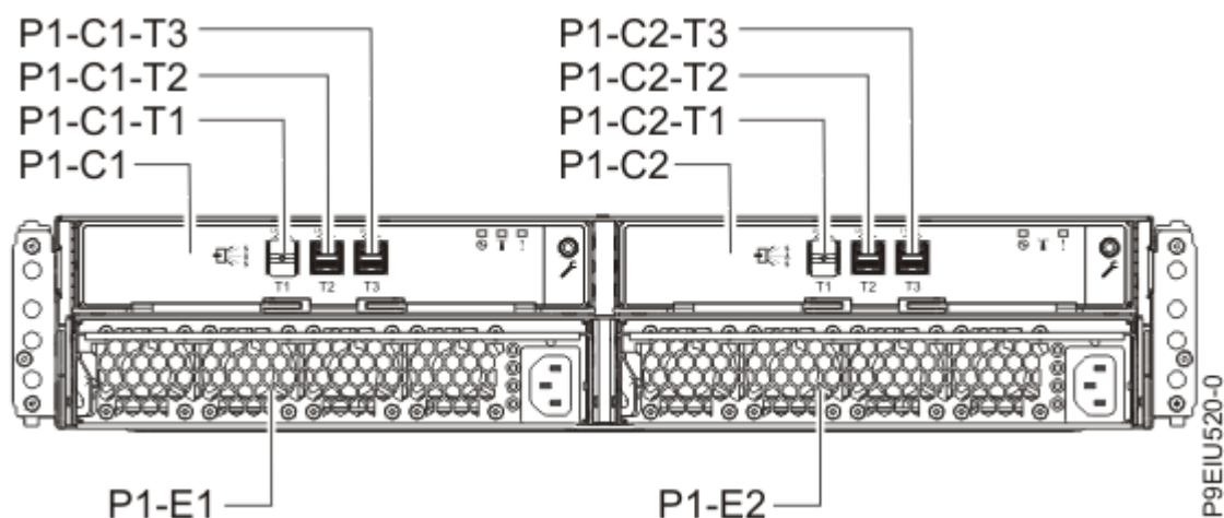
Figura 11. Vista posterior das unidades de expansão
