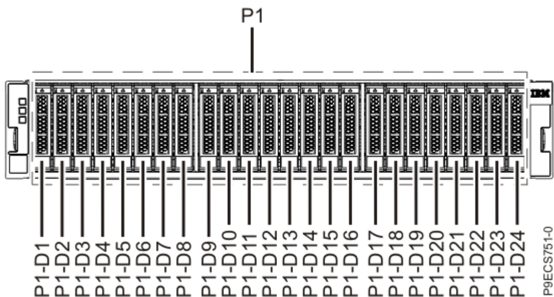
Figura 10. Vista anterior da unidade de expansão ESLS que mostra as localizações das unidade
