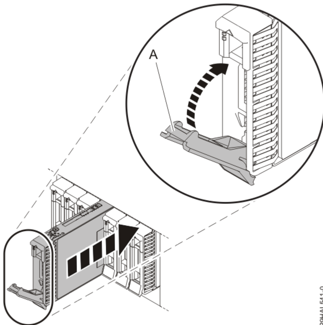
Figura 8. Instalar uma unidade num sistema
