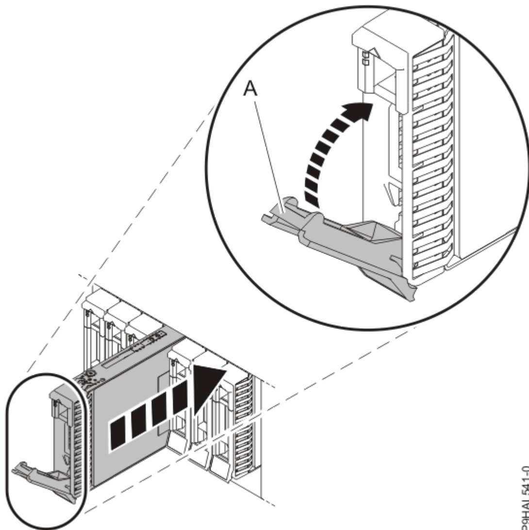
Figura 18. Substituir uma unidade num suporte
