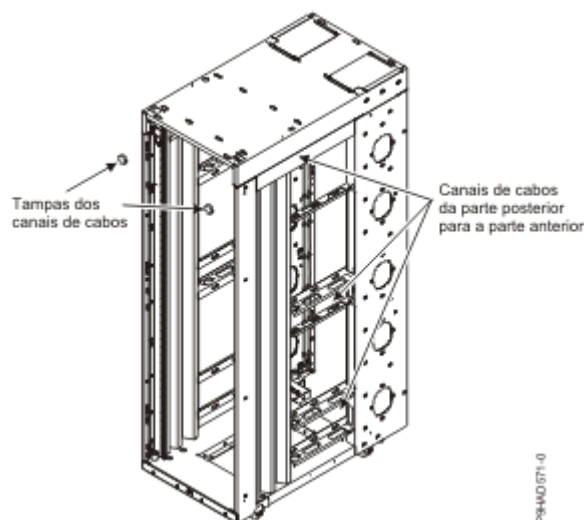
Figura 15. Cablagem no bastidor
