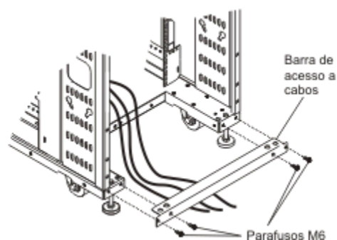
Figura 9. Barra de acesso de cabos
