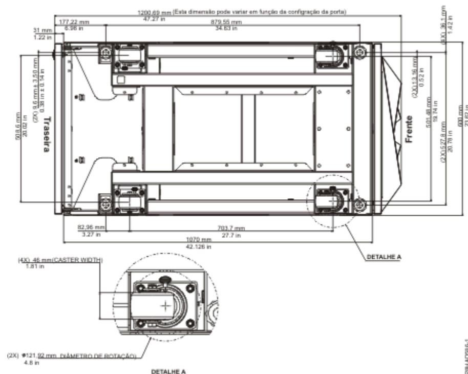
Figura 14. Localizações dos rodízios e parafusos de nivelamento
