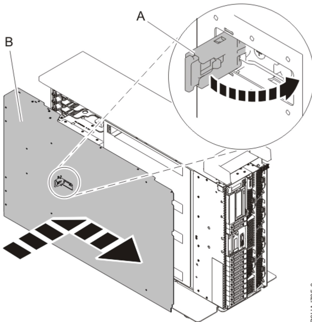
Figura 19. Instalar a tampa de acesso para assistência
