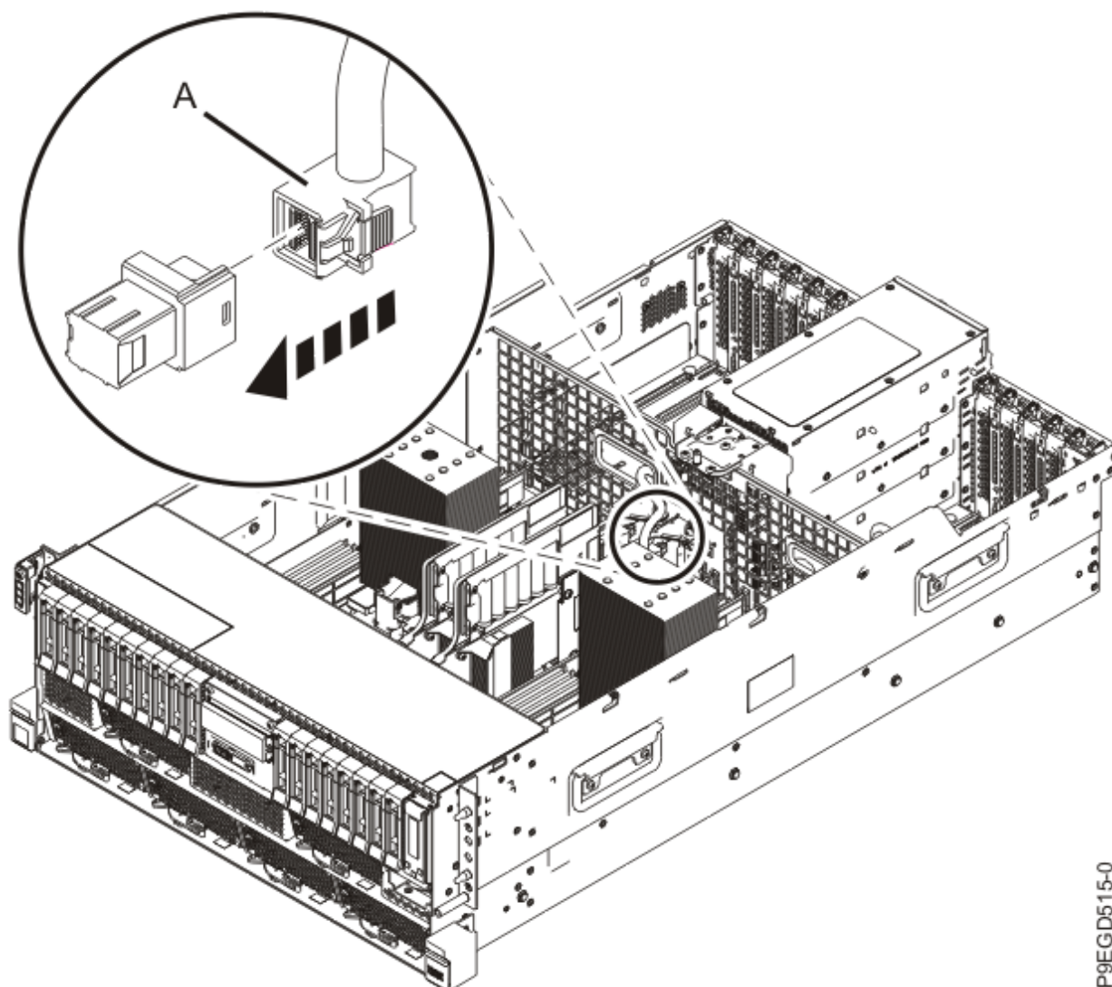
Figura 38. Voltar a ligar os cabos SAS posteriores
