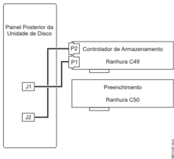
Figura 33. Voltar a ligar o cabo SAS numa configuração de armazenamento base
