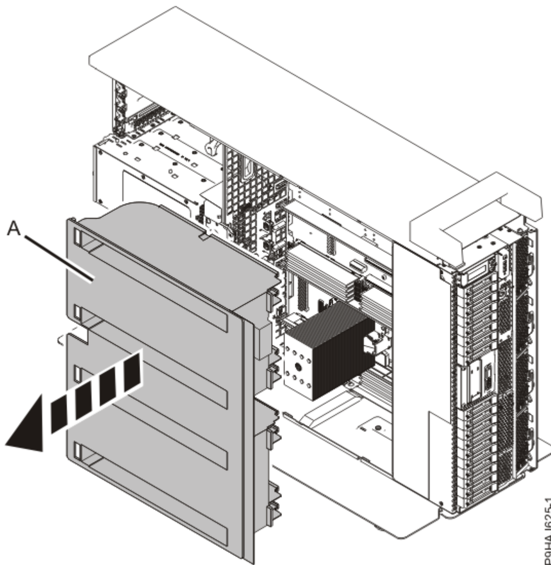
Figura 29. Remover a conduta de ventilação de um sistema autónomo
