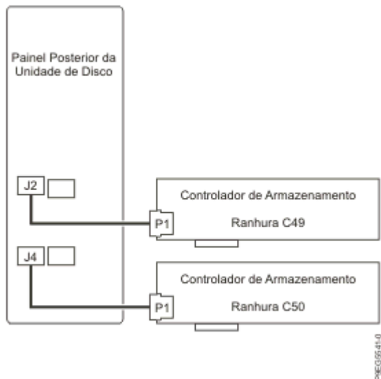
Figura 35. Voltar a ligar o cabo SAS na configuração do função expandida de 12 unidades
