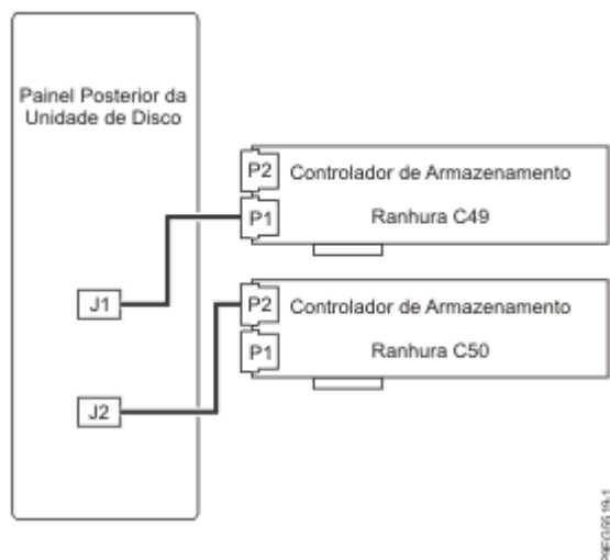
Figura 34. Voltar a ligar o cabo SAS numa configuração de disco dividido
