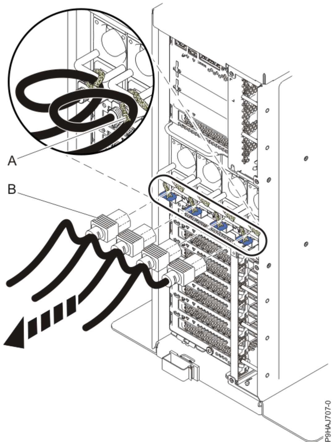
Figura 24. Remover os cabos de alimentação de um servidor autónomo
