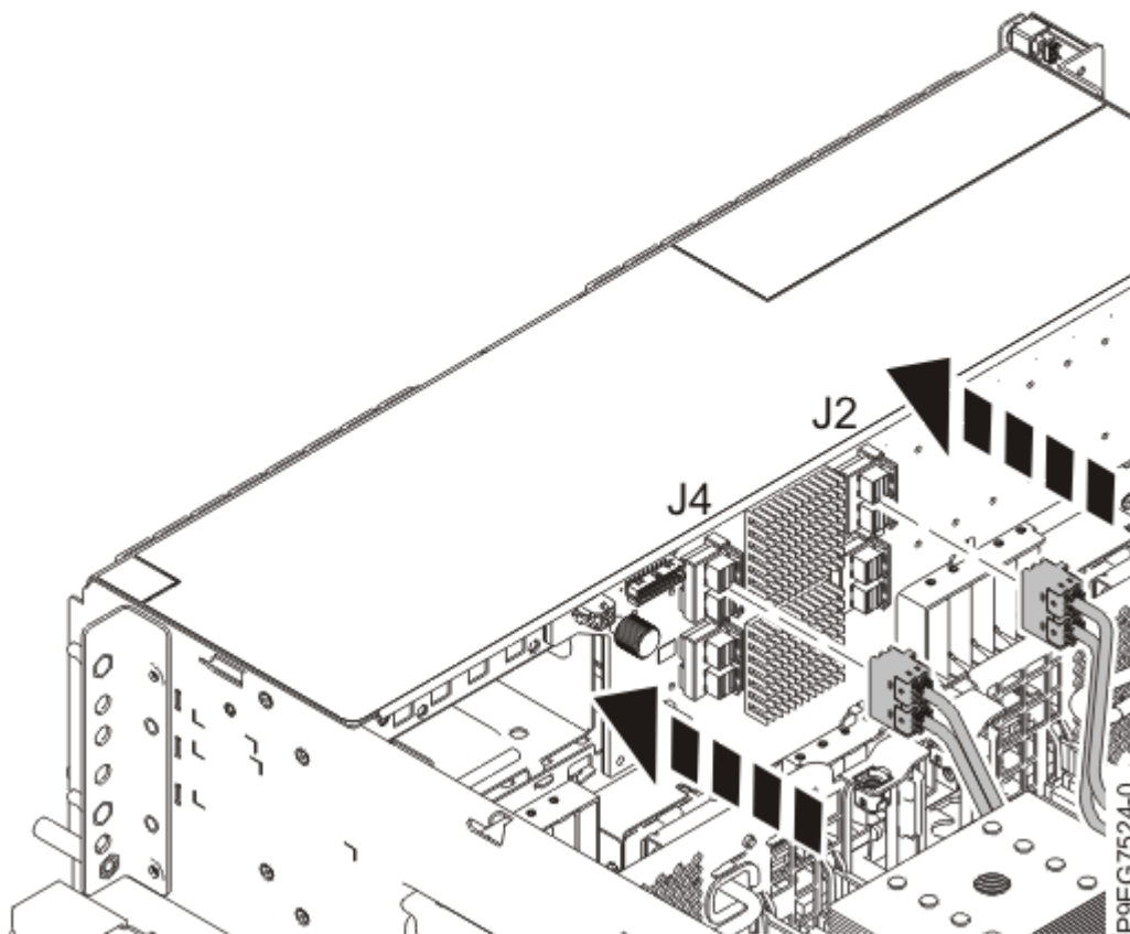
Figura 40. Voltar a ligar os cabos SAS frontais para o painel posterior da unidade de disco função expandida de 12 unidades ou função expandida de 18 unidades
