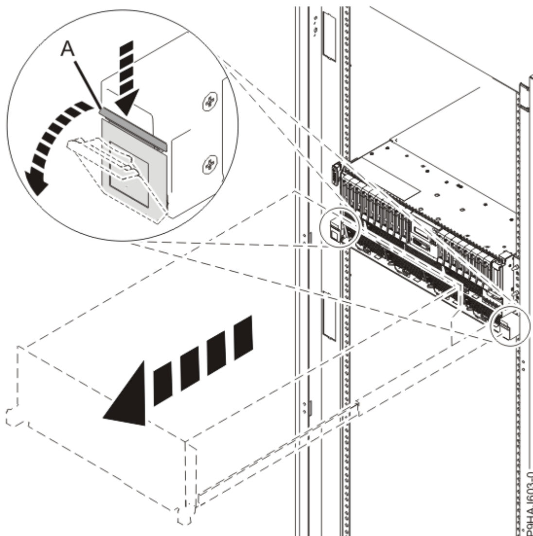
Figura 25. Soltar as patilhas laterais
