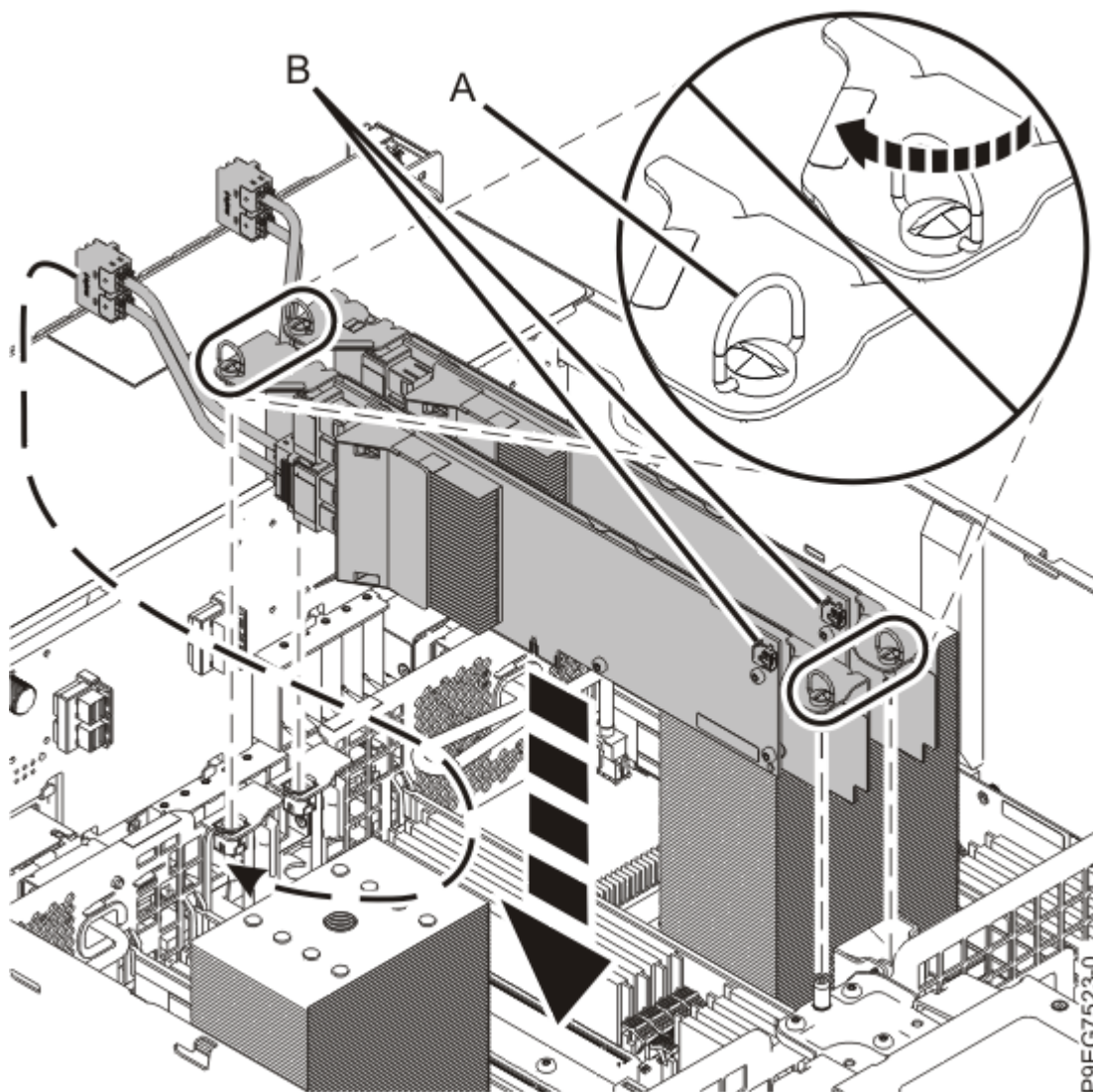
Figura 12. Encaixar o adaptador SAS RAID
