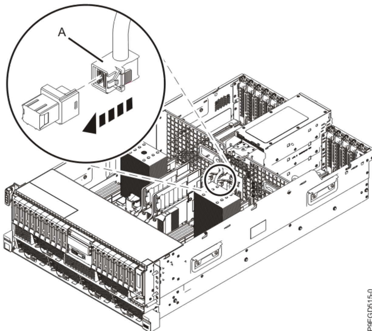
Figura 13. Voltar a ligar os cabos SAS posteriores
