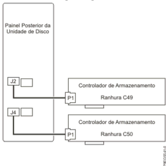
Figura 11. Voltar a ligar o cabo SAS na configuração do função expandida de 18 unidades
