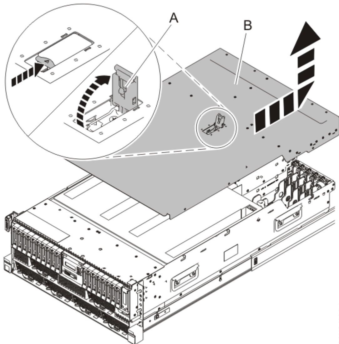
Figura 4. Remover a tampa de acesso para assistência de um sistema montado em bastidor
