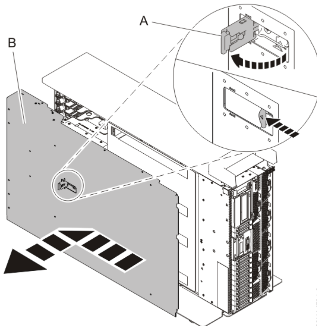
Figura 5. Remover a tampa de acesso para assistência
