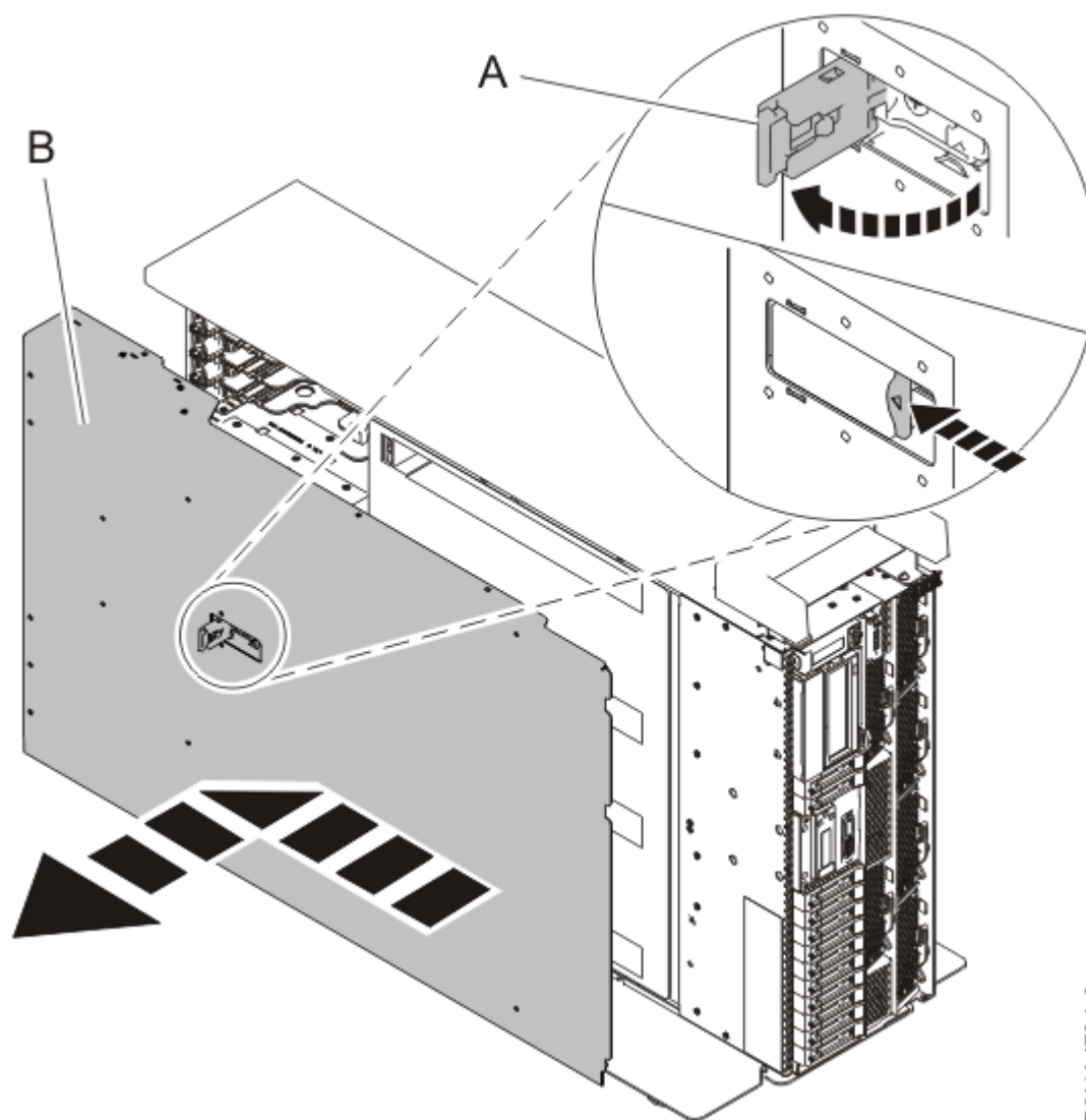
Figura 27. Remover a tampa de acesso para assistência
