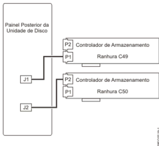
Figura 9. Voltar a ligar o cabo SAS numa configuração de disco dividido
