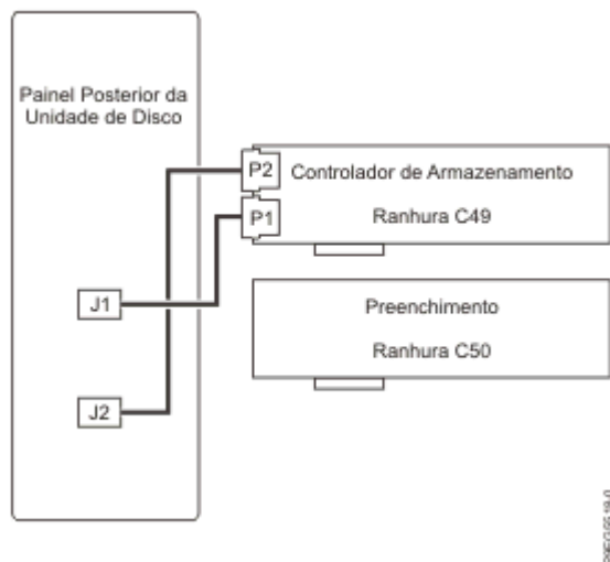
Figura 8. Voltar a ligar o cabo SAS numa configuração de armazenamento base
