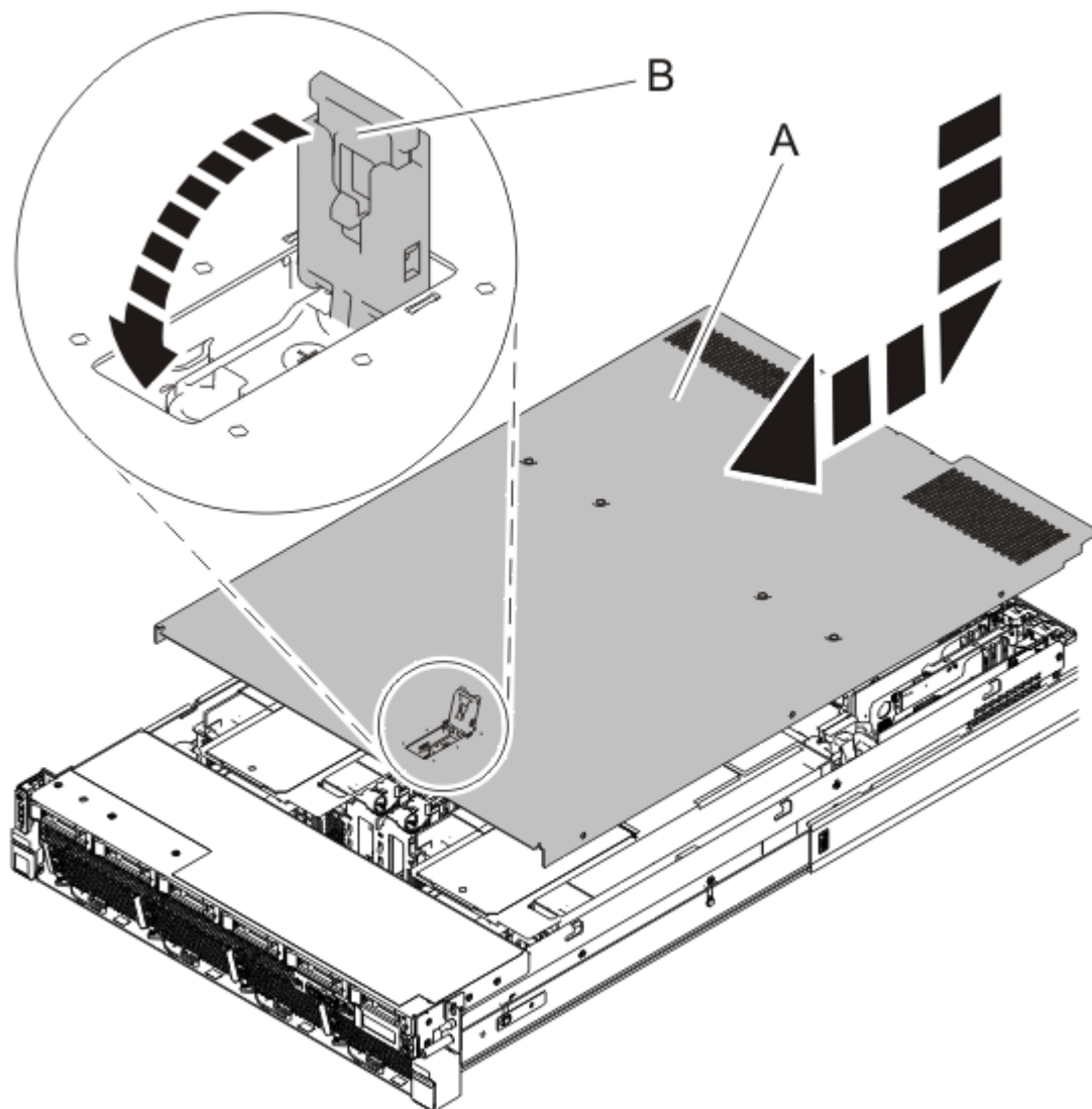
Figura 7. Instalar a tampa de acesso para assistência
