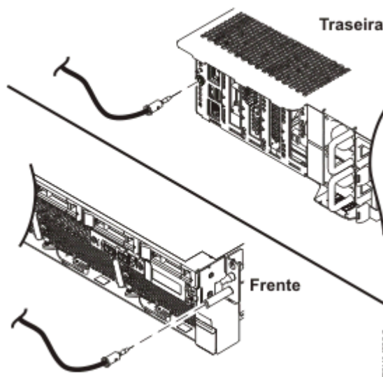
Figura 3. Localização das tomadas ESD
