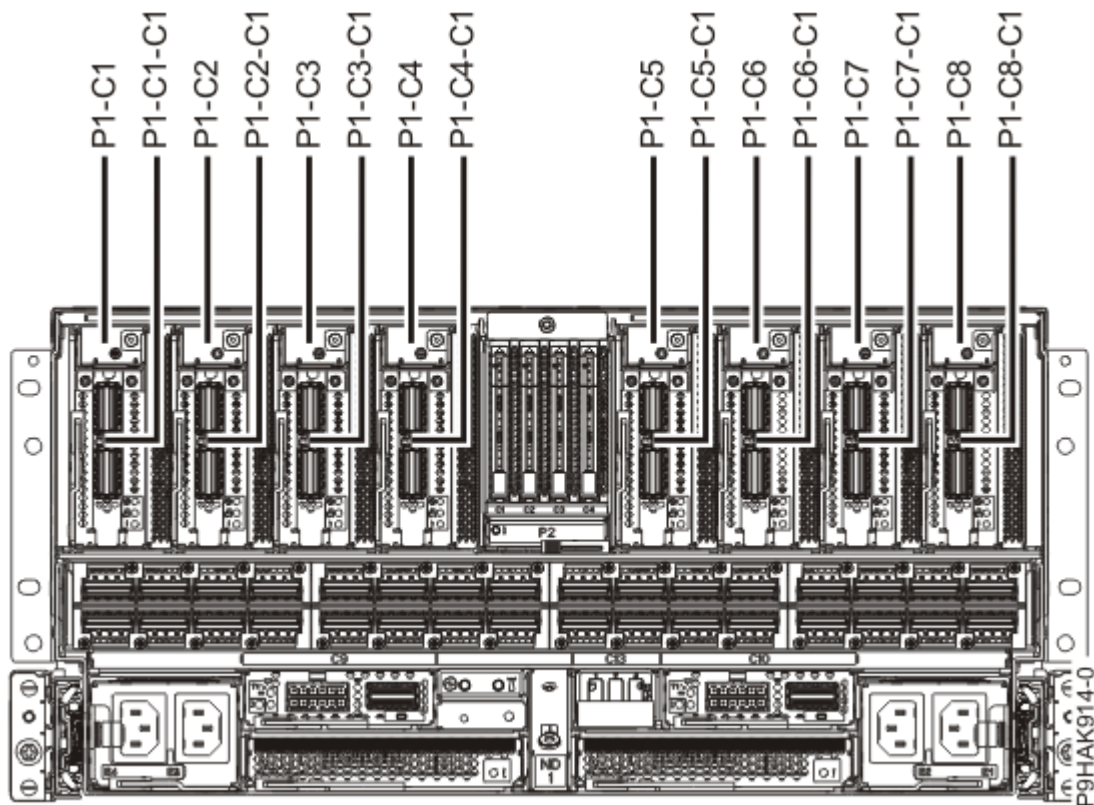
Figura 1. A vista posterior do sistema 9080-M9S montado em bastidor com códigos de localizações de ranhuras do PCIe
