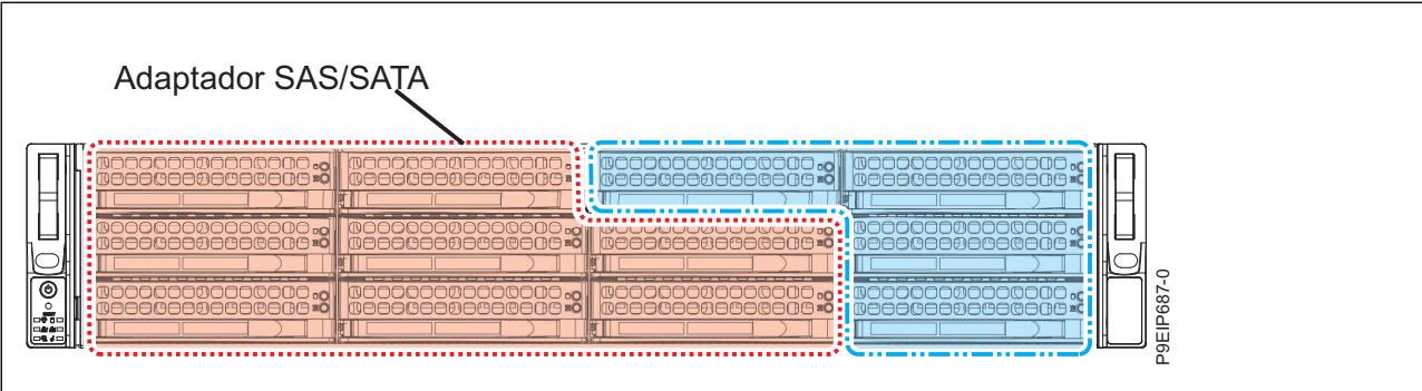
Figura 5. Até oito unidades SAS ou SATA conectadas a um adaptador SAS/SATA, até quatro unidades SAS ou SATA conectadas ao controlador integrado e até dois DOMs
