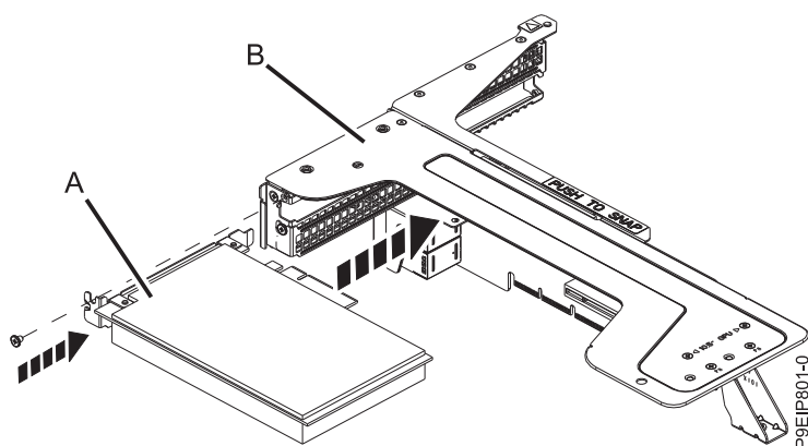
Figura 56. Inserindo um adaptador na posição 2 do riser PCIe
