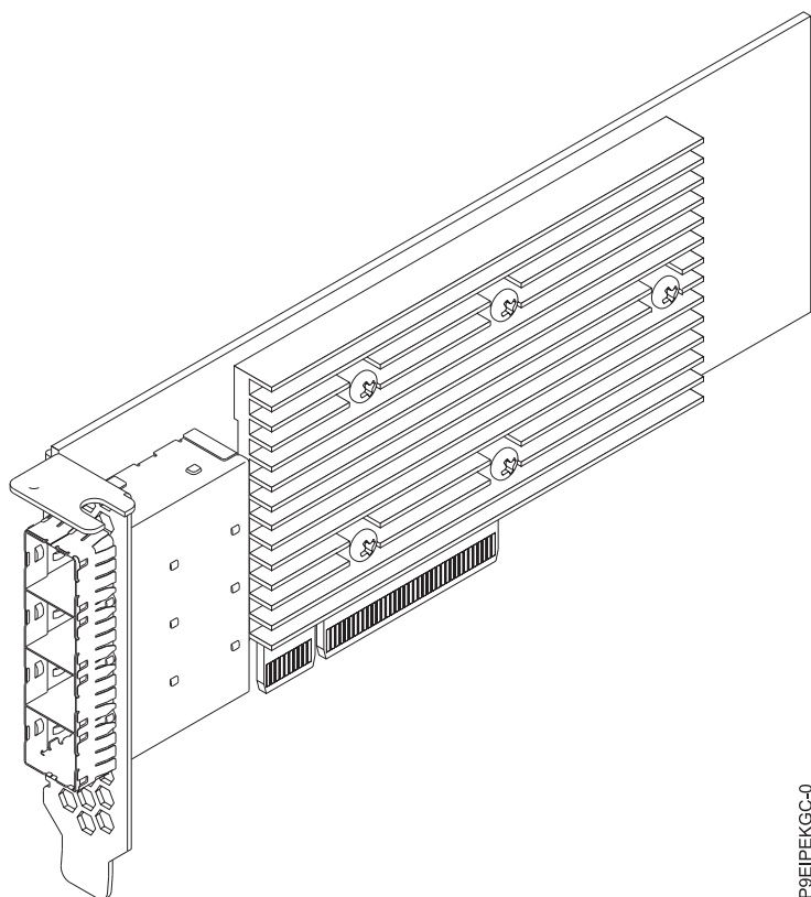
Figura 50. Broadcom (LSI) 9305-16E SAS3 HBA PCIe3.0 x8 LP
