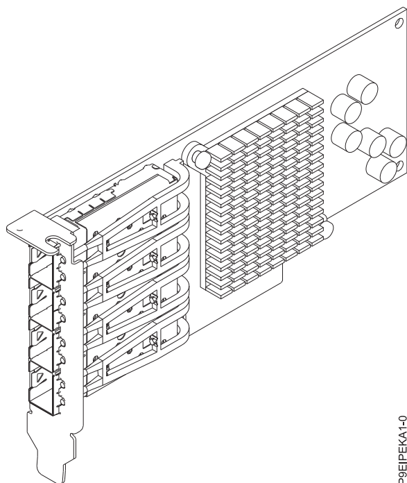
Figura 26. Adaptador Ethernet Cavium (Qlogic) BCM57840 PCIe3.0 x8 LP com 4 portas SFP+ de 10 Gb
