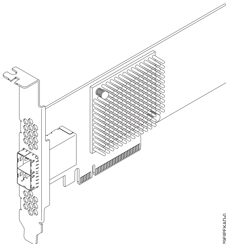
Figura 44. Adaptador Broadcom (LSI) 9300-8E SAS3 HBA PCIe3.0 x8 LP
