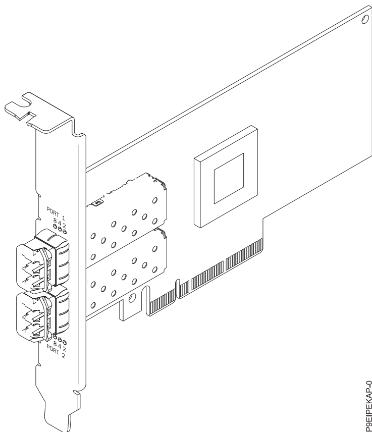
Figura 36. Adaptador Mellanox MCX415A-CCAT ConnectX-4 EN de 100 GbE com uma porta QSFP28 PCIe3.0 x16 LP
