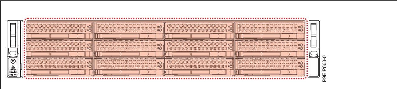
Figura 6. Até 12 unidades SAS ou SATA ou uma combinação de HDDs SAS e SSDs SATA (12 unidades no total), adaptador SAS/SATA e até dois DOMs
