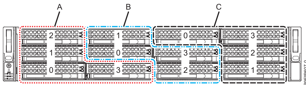
Figura 9. Mapeamento de porta para compartimento de unidade
