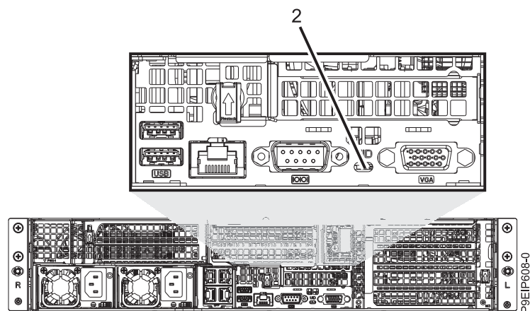
Figura 64. LEDs na parte traseira do sistema
