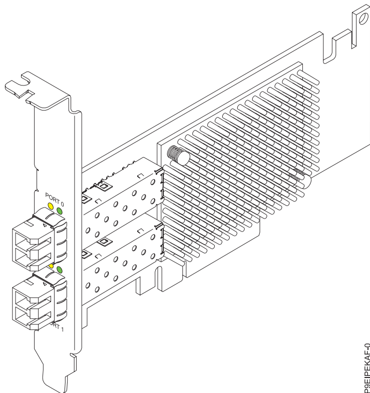
Figura 31. Placa Fibre Channel PCIe3.0 x8 LP Emulex LPE16002B-M6-O com porta dual e 16 Gb
