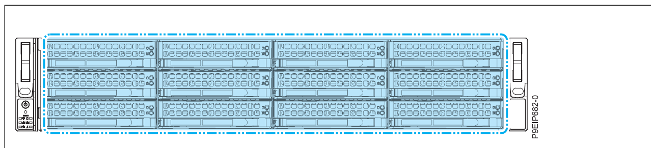
Figura 3. Até 12 unidades SAS ou SATA e até dois DOMs
