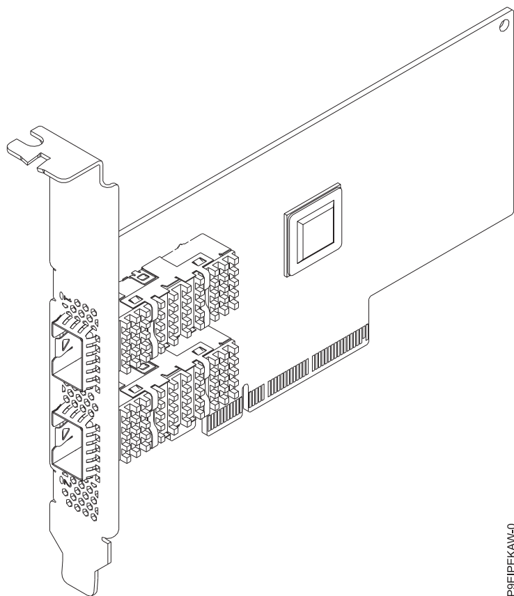
Figura 40. Adaptador Mellanox MCX414A-BCAT ConnectX-3 Pro EN com porta dual 40/56 GbE PCIe3.0 x8 LP
