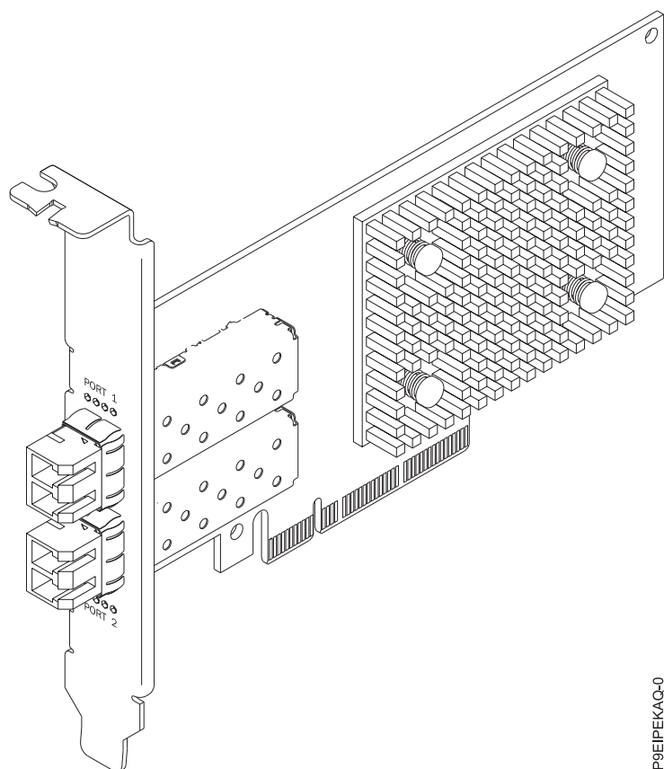
Figura 37. Adaptador Adaptador Fibre Channel PCIe3 x8 LP Qlogic QLE2692OP com porta dual e 16 Gb
