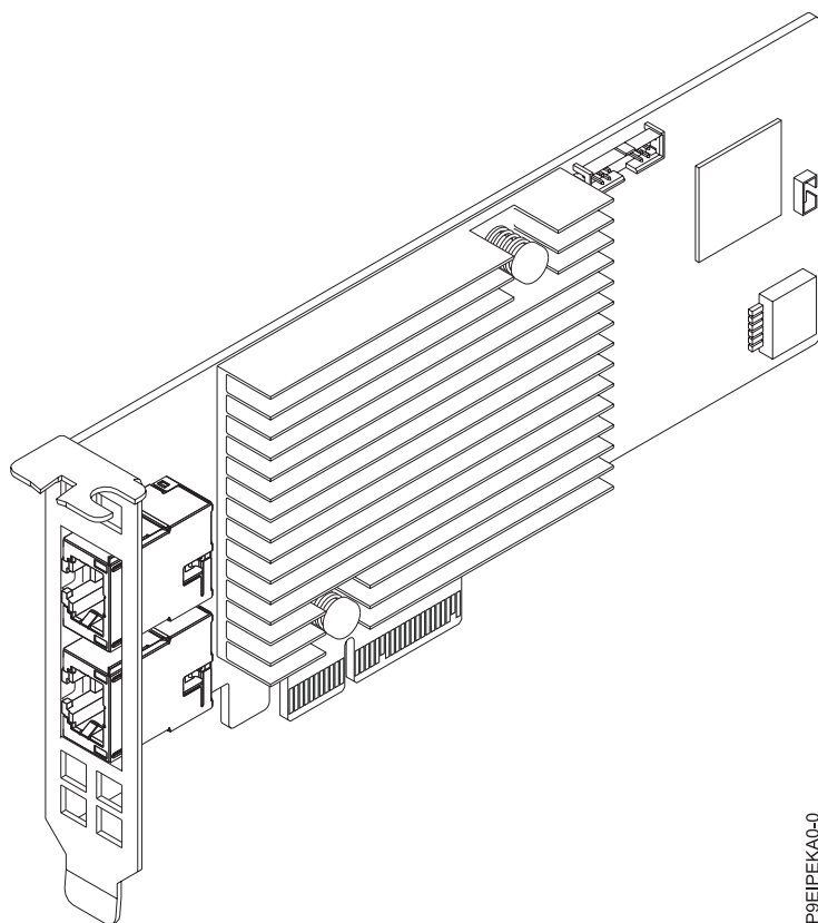
Figura 25. Adaptador de rede convergido PCIe3 x4 Intel x550 10GBase-T com portas duais RJ45
