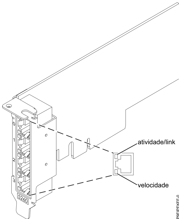
Figura 47. Placa da interface de rede PCIe x4 LP Broadcom 5719 QP 1G (1G/100M/10M)
