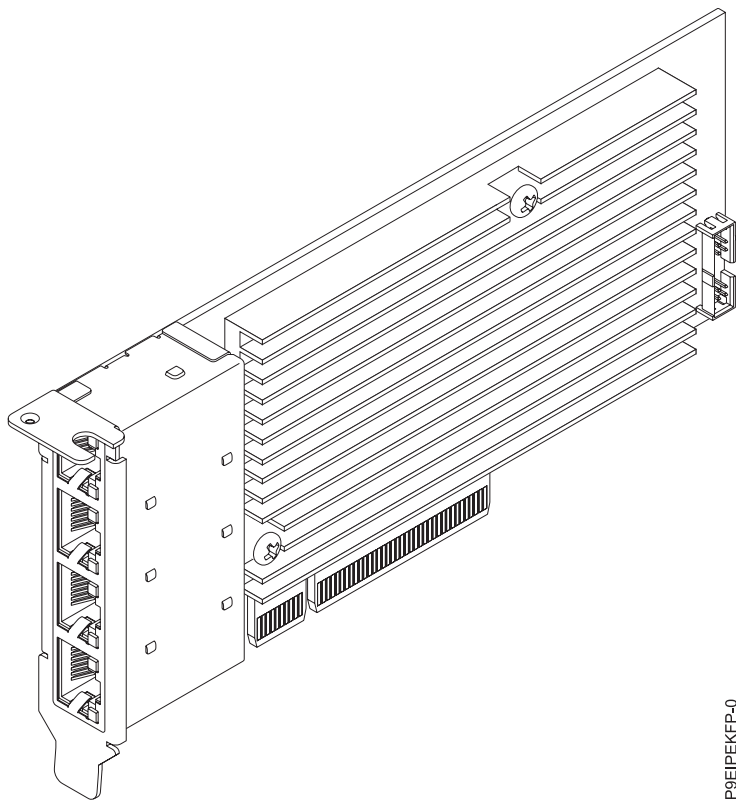
Figura 49. Adaptador de rede convergido Intel XL710/X557 10GBase-T com portas quádruplas (velocidades de 10G/1G/100M) PCIe3.0 x8 LP
