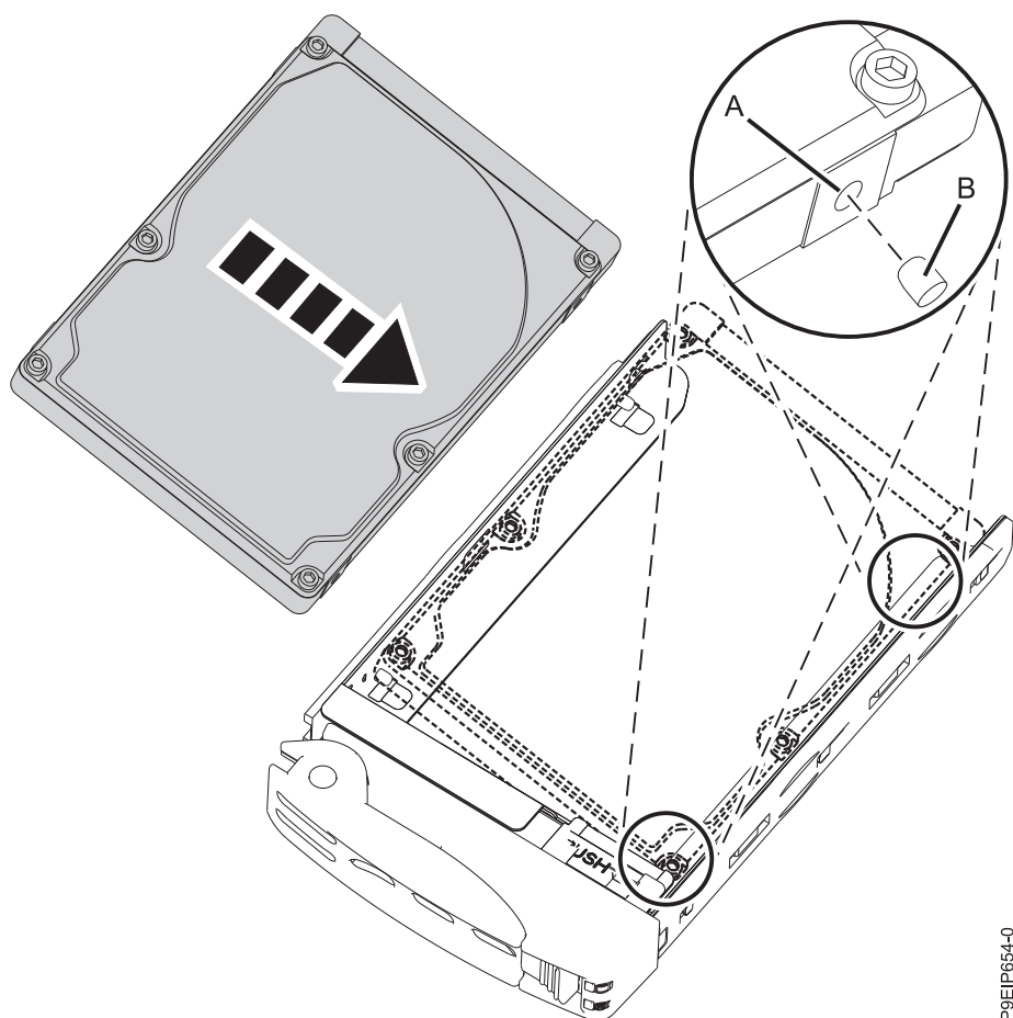
Figura 17. Inserindo a unidade traseira na bandeja
