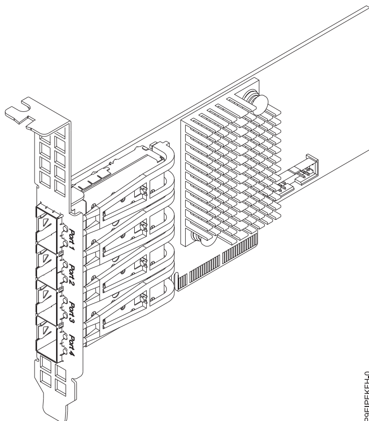
Figura 48. Adaptador de rede convergido Ethernet Intel XL710 com portas quádruplas 10G/1G SFP+ PCIe3.0 x8 LP
