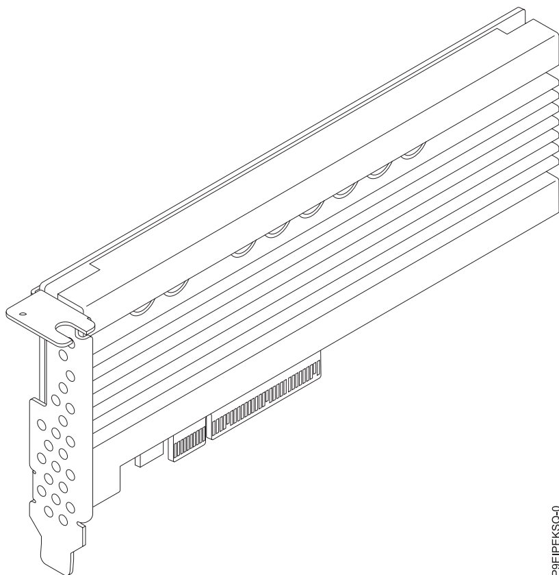
Figura 51. Adaptador Samsung PM1725a NVMe 1,6 TB 5DWPD PCIe3.0 x8 LP
