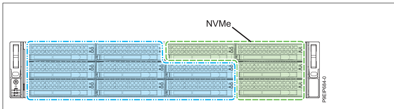
Figura 4. Até 8 unidades SAS ou SATA ou uma combinação de HDDs SAS e SSDs SATA (oito unidades no total), quatro unidades NVMe conectadas a um adaptador NVMe e até dois DOMs
