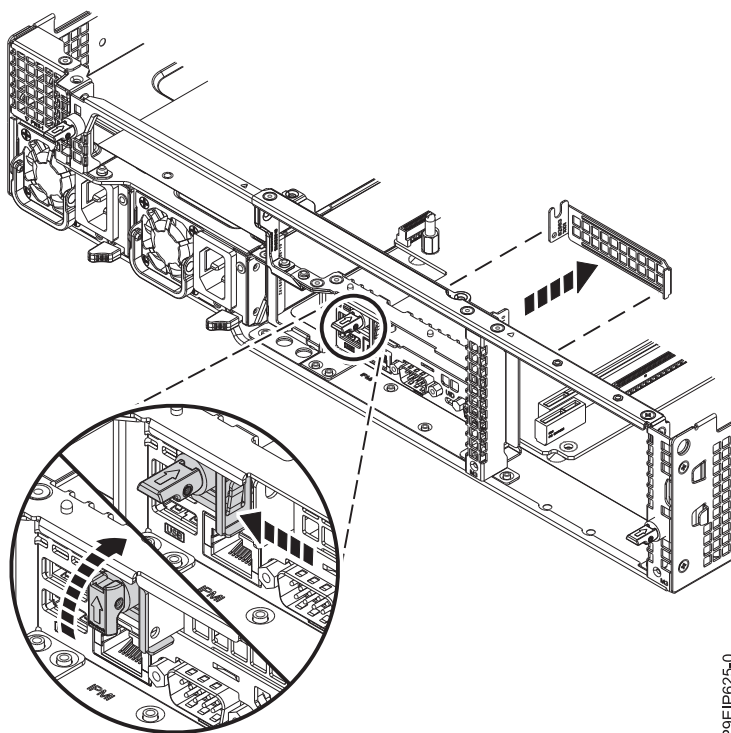
Figura 58. Liberando o suporte sobre trilhos
