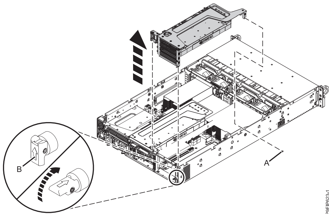
Figura 60. Removendo o riser PCIe
