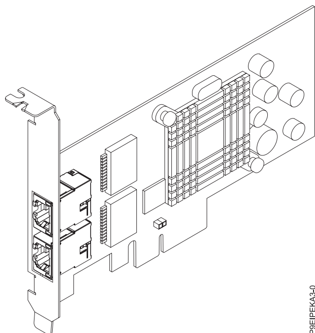
Figura 28. IControladora Ethernet Intel 82575EB com porta dual Gigabit PCIe x4.0 LP
