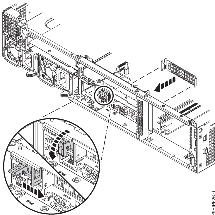
Figura 59. Deslizando o retentor do suporte sobre trilhos para a posição fechada
