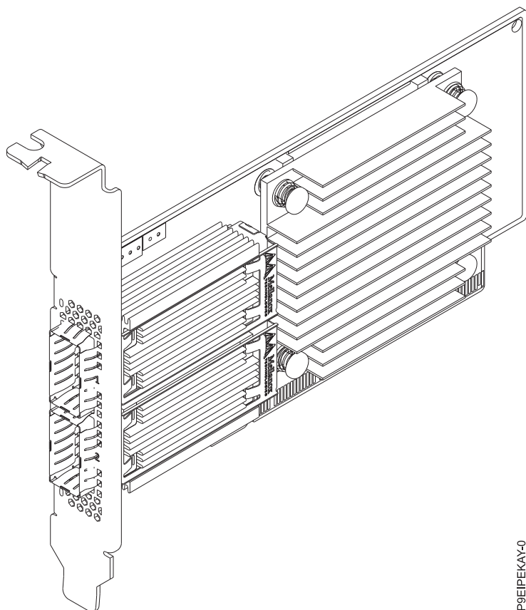
Figura 41. Adaptador Mellanox MCX556A-EDAT ConnectX-5 VPI EDR InfiniBand 100 Gb/s e 100 GbE com porta dual QSFP28 PCIe4.0 x16 LP
