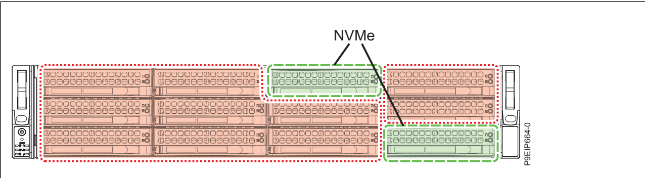
Figura 7. Até 10 unidades SAS ou SATA ou uma combinação de HDDs SAS e SSDs SATA (10 unidades no total), adaptador SAS/SATA, duas unidades NVMe conectadas a um adaptador NVMe e até dois DOMs
