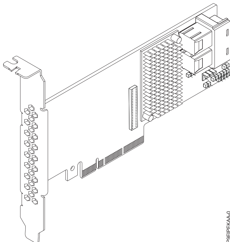
Figura 29. Controlador Broadcom (LSI) MegaRAID 9361-8i SAS3 com 8 portas internas (1 GB de cache) PCIe3.0 x8 LP com cabos
