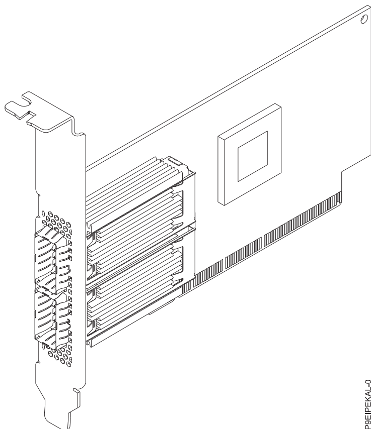
Figura 34. Adaptador Mellanox MCX456A-ECAT ConnectX-4 VPI EDR InfiniBand 100 Gb/s e 100 GbE com porta dual QSFP28 PCIe3.0 x16 LP
