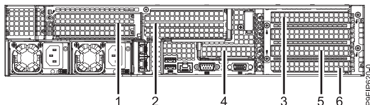
Figura 24. Vista posterior de um sistema 9006-22P com slots PCIe indicados
