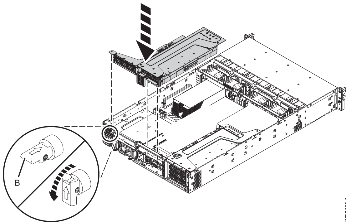
Figura 57. Inserindo o riser da posição 1 e 2
