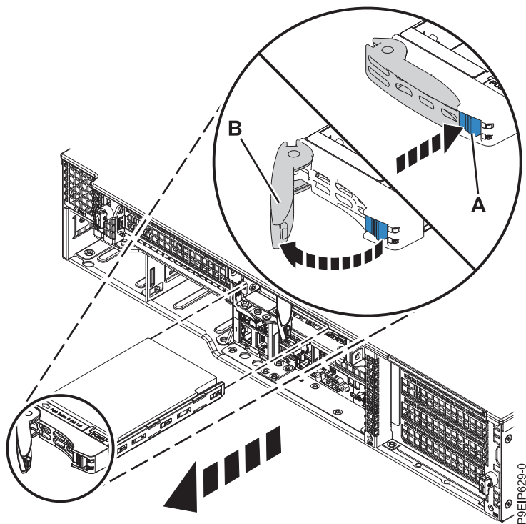
Figura 16. Removendo uma unidade traseira
