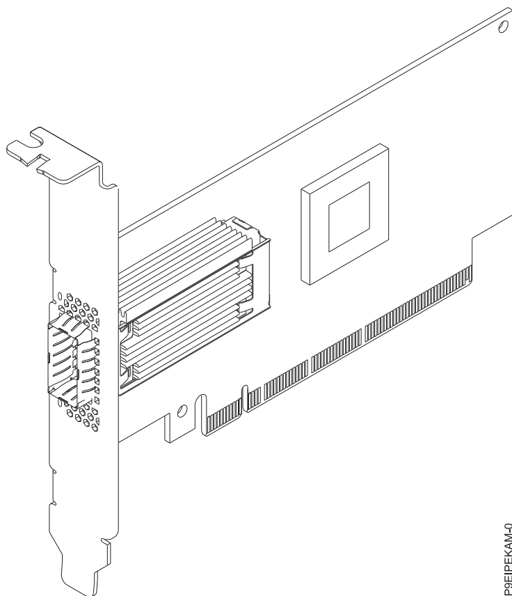
Figura 35. Mellanox MCX415A-CCAT ConnectX-4 EN de 100 GbE com uma porta QSFP28 PCIe3.0 x16 LP
