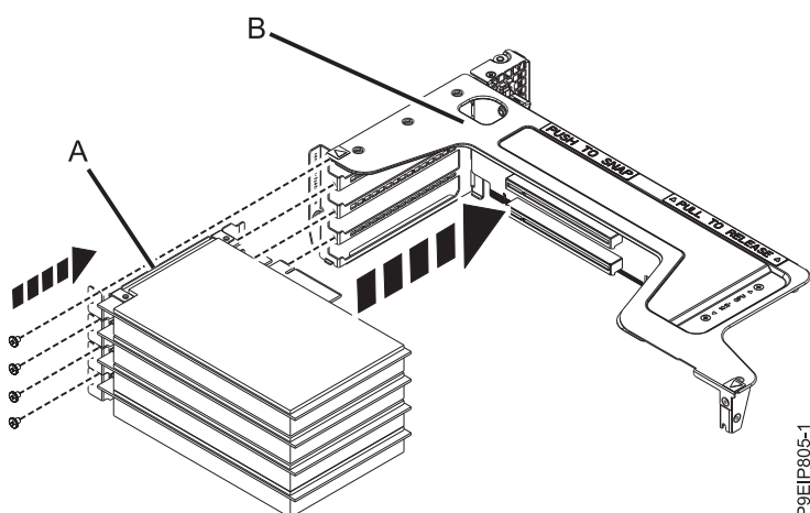
Figura 61. Inserindo um adaptador PCIe no riser
