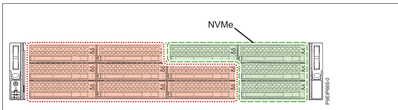
Figura 8. Até oito unidades SAS ou SATA ou uma combinação de HDDs SAS e SSDs SATA (oito unidades no total), adaptador SAS/SATA, quatro unidades NVMe conectadas a um adaptador NVMe e até dois DOMs
