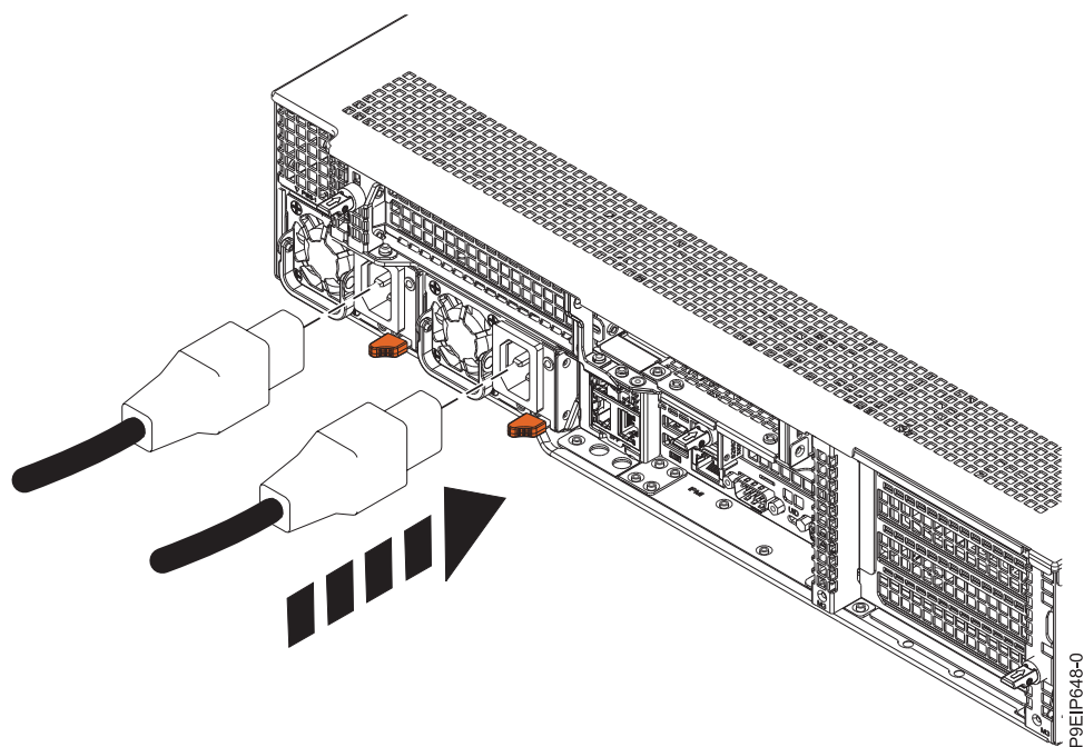
Figura 72. Conectando os cabos de energia ao sistema
