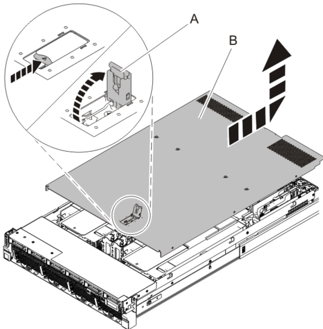
Figura 30. Removendo a Tampa de Acesso de Serviço
