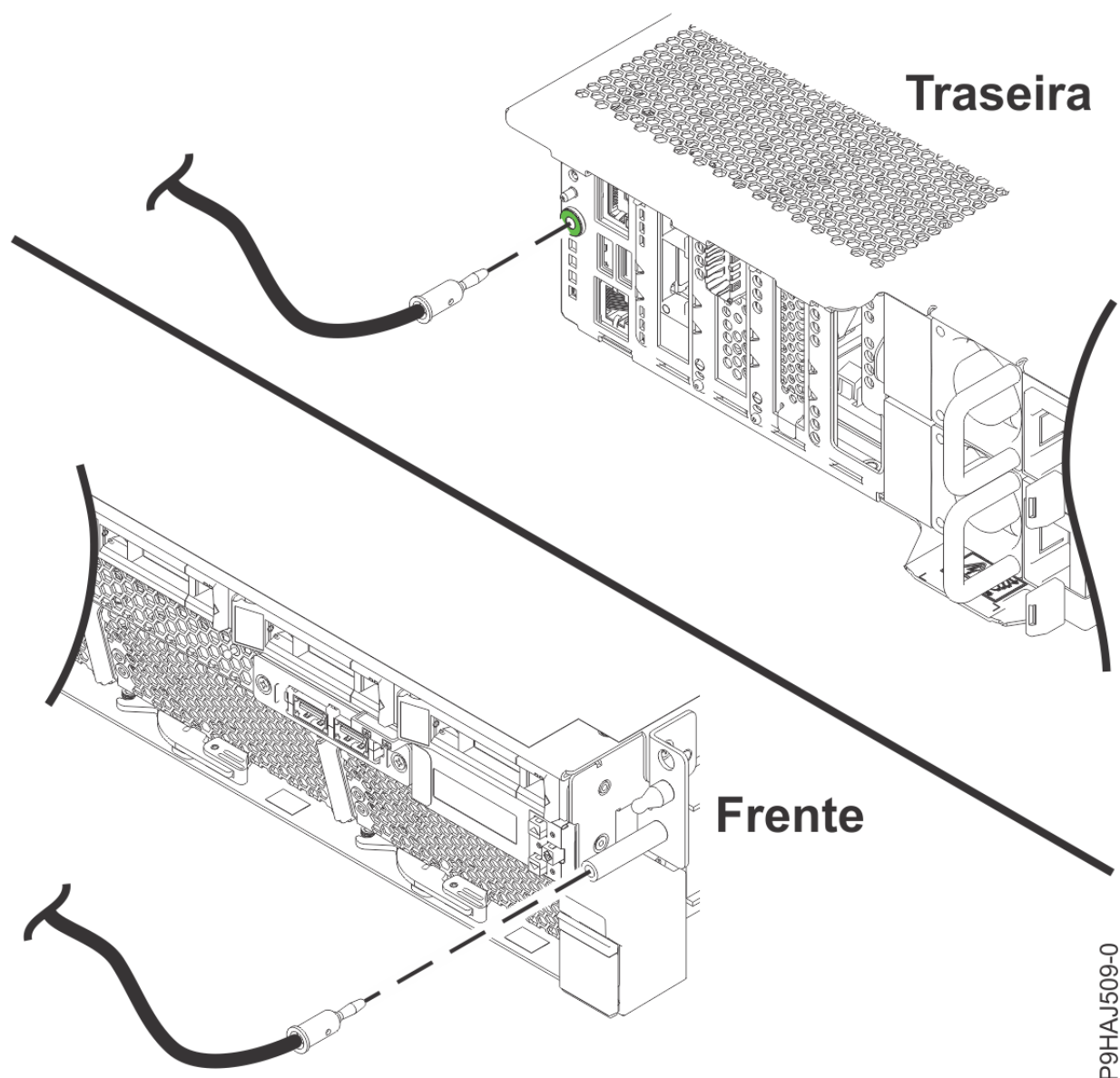
Figura 38. Local dos plugues do ESD
