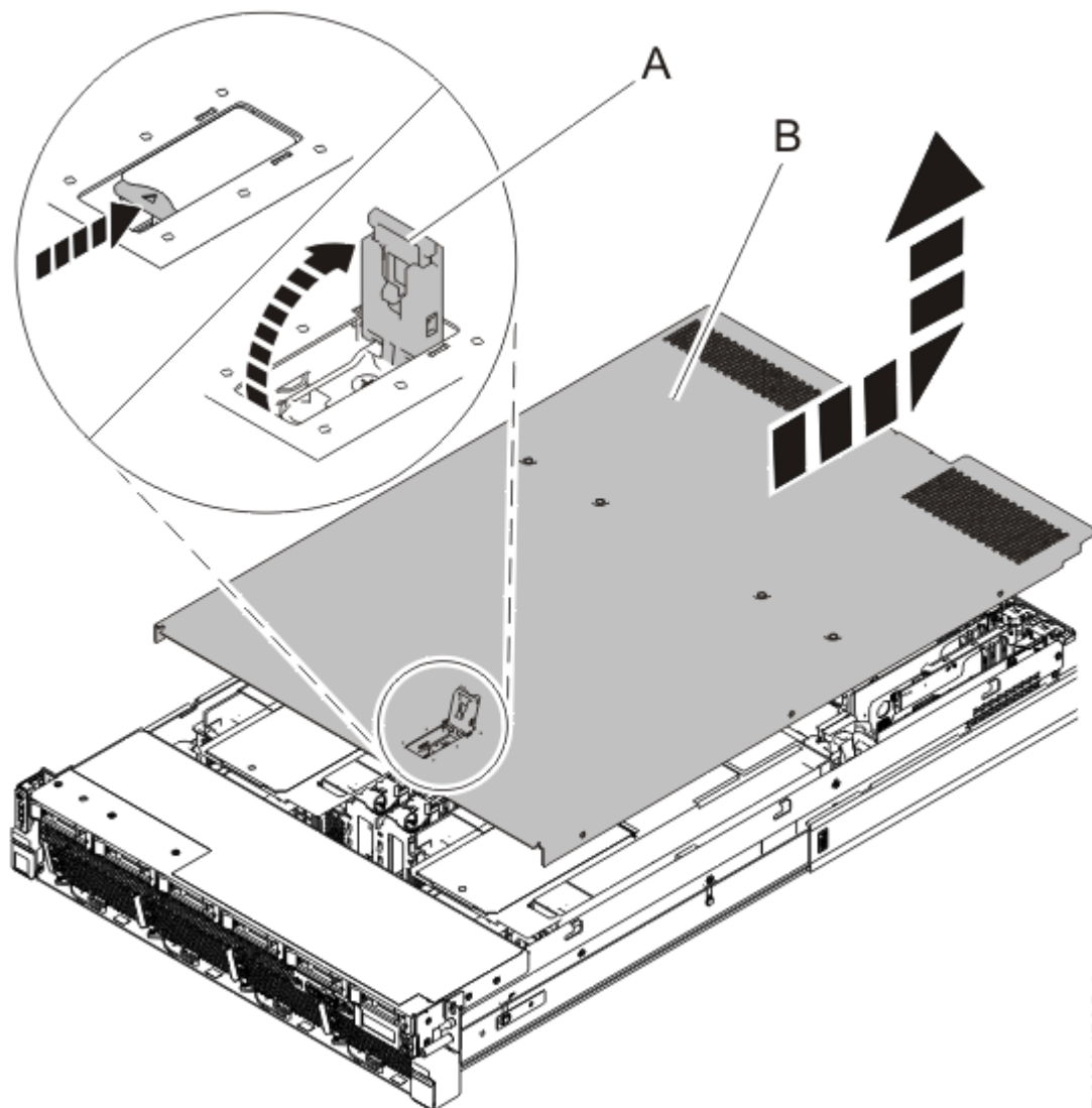
Figura 39. Removendo a Tampa de Acesso de Serviço
