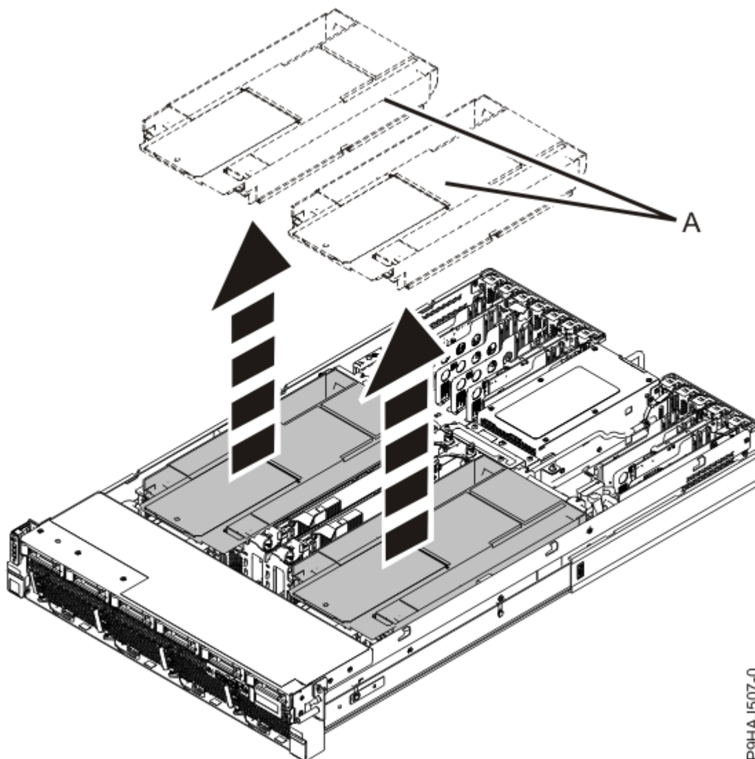
Figura 5. Removendo a placa defletora de ar
