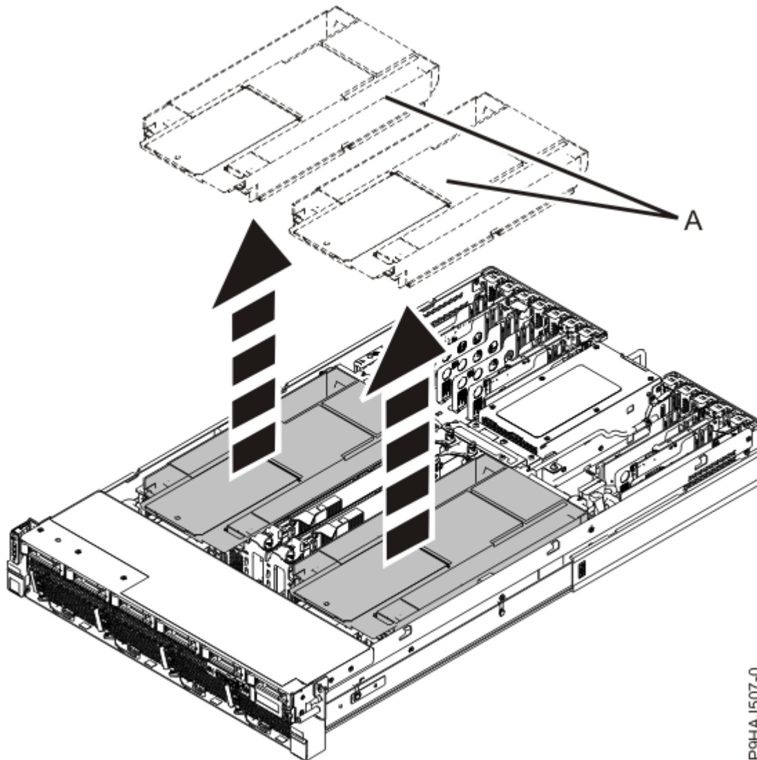
Figura 40. Removendo a placa defletora de ar
