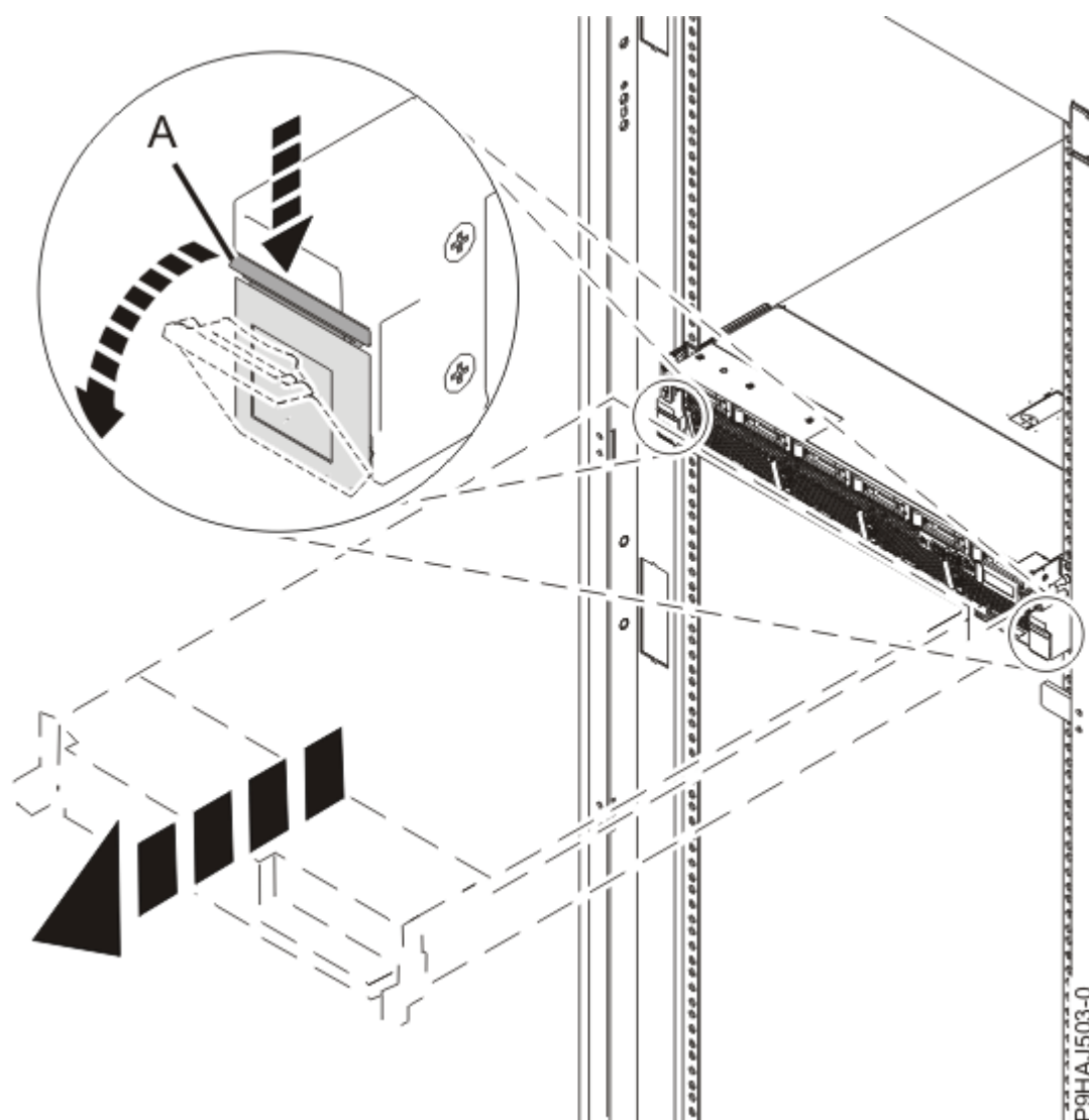
Figura 28. Liberando as Travas Laterais
