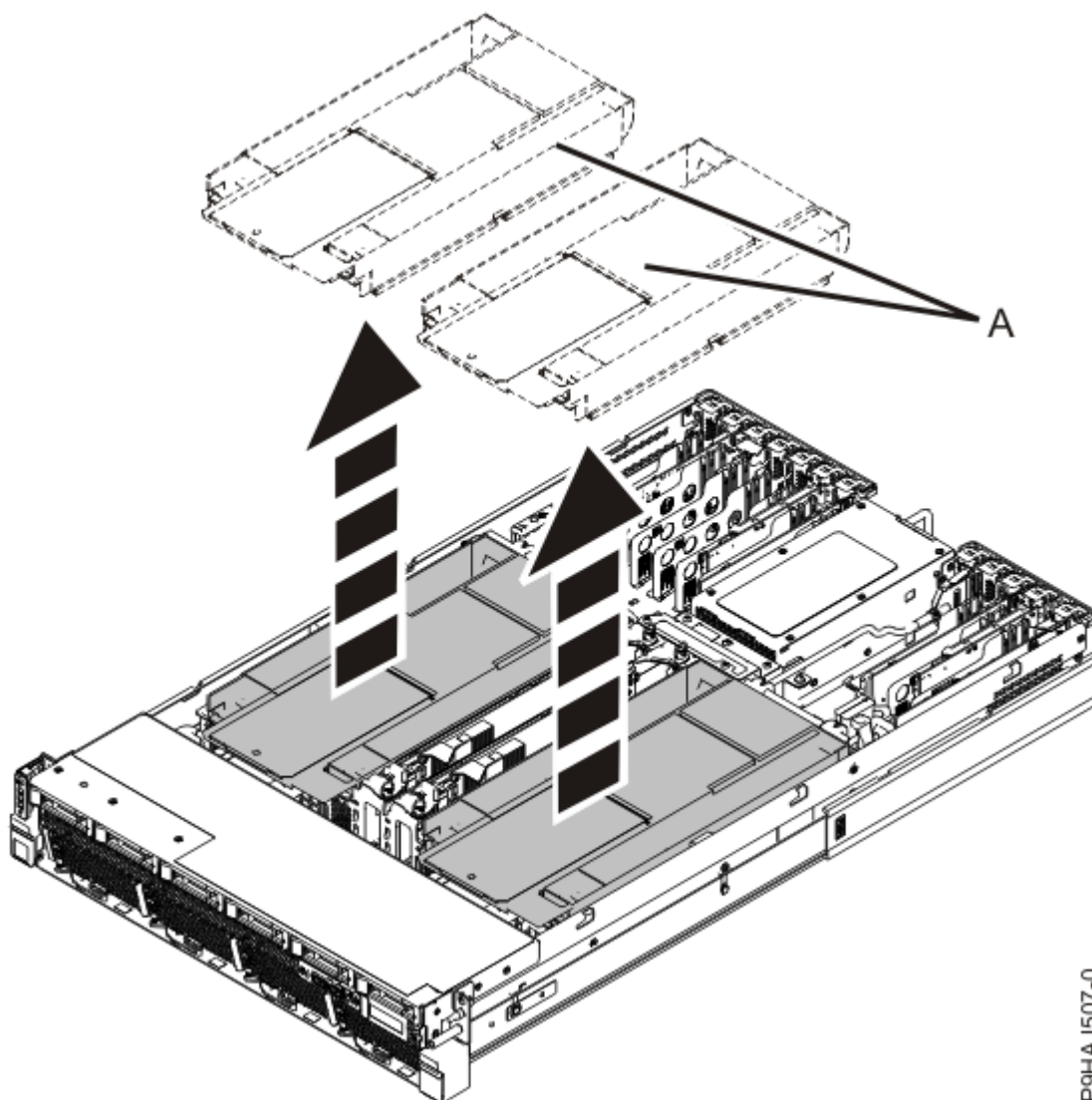
Figura 31. Removendo a placa defletora de ar
