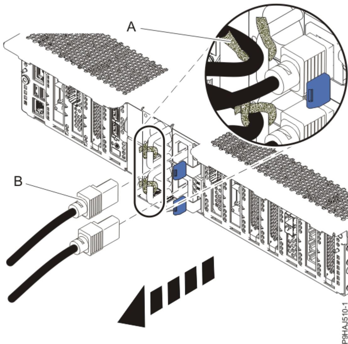
Figura 1. Removendo os Cabos de Energia
