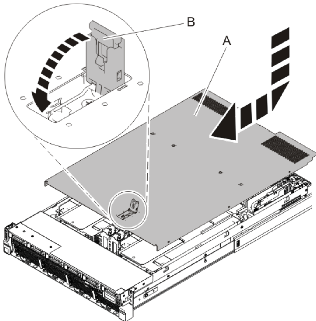
Figura 34. Instalando a Tampa de Acesso de Serviço
