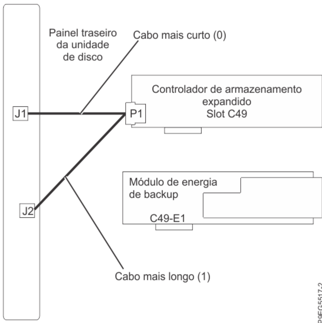
Figura 19. Reconnectando o cabo SAS em "Y" em uma configuração de controlador de armazenamento de alto desempenho
