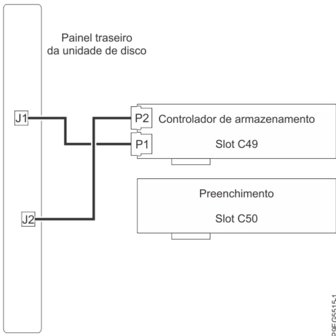
Figura 17. Reconectando o cabo SAS em uma configuração de armazenamento de base
