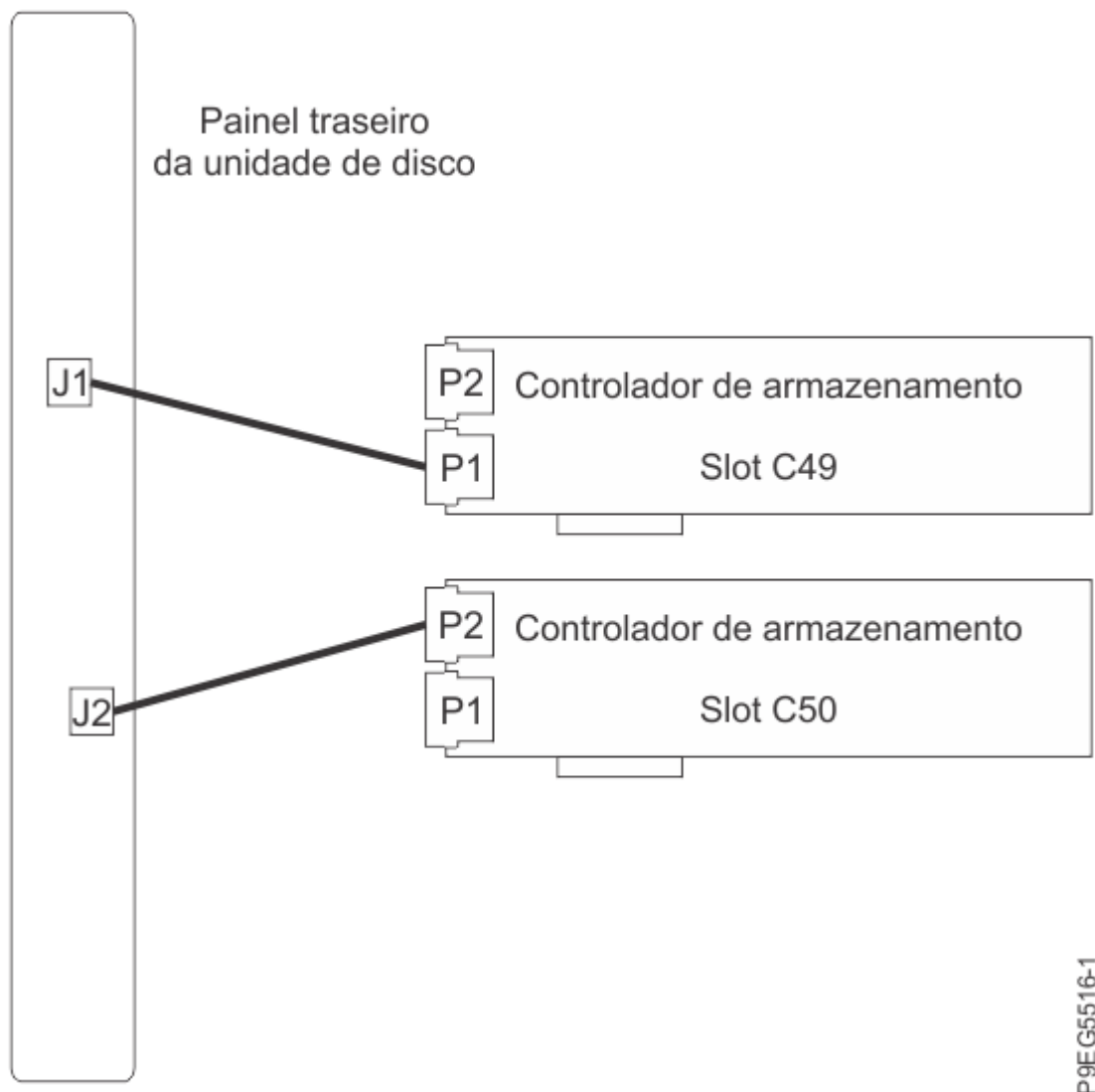
Figura 18. Reconectando o cabo SAS em uma configuração de divisão de disco
