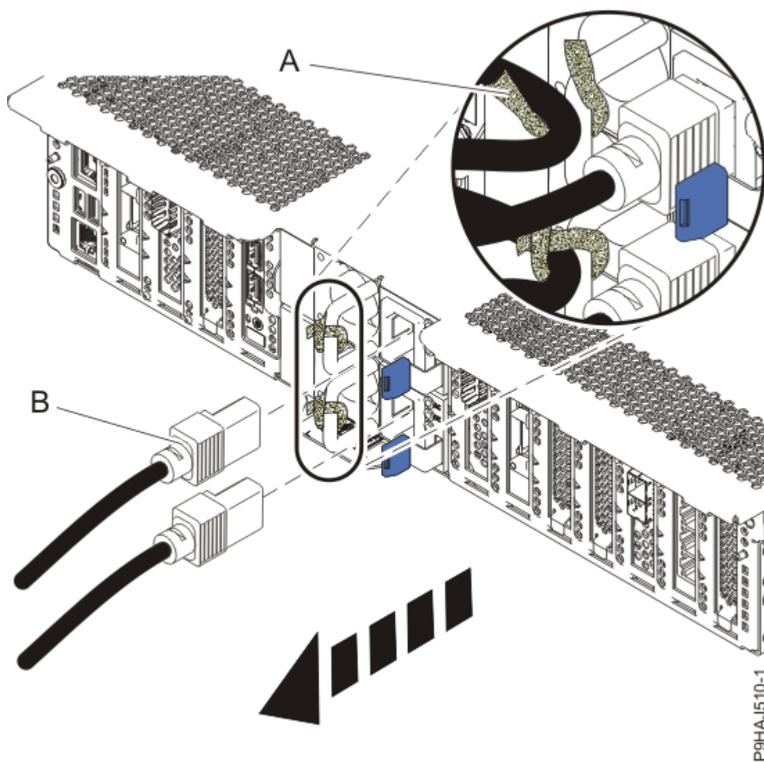
Figura 27. Removendo os Cabos de Energia
