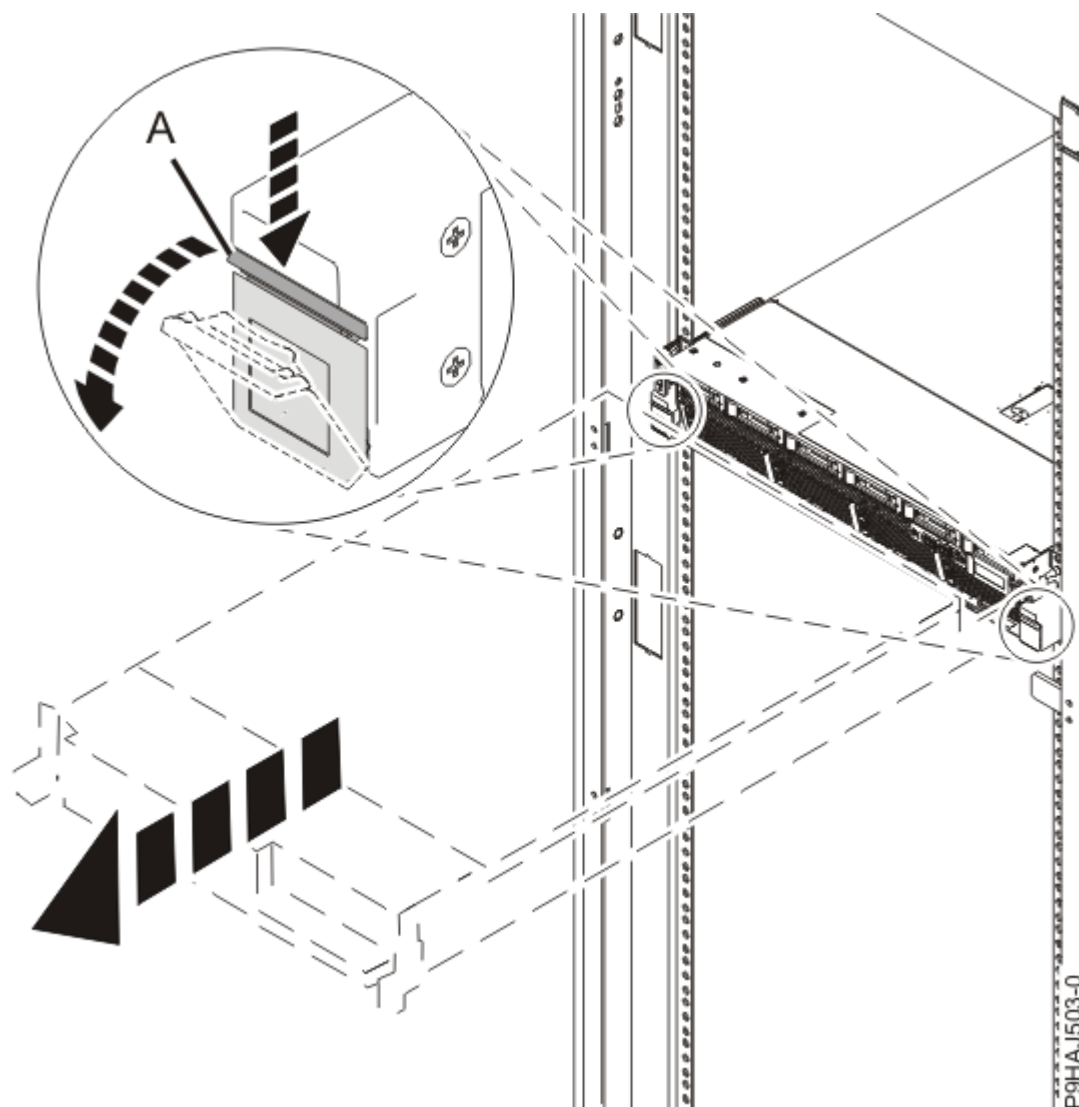
Figura 37. Liberando as Travas Laterais
