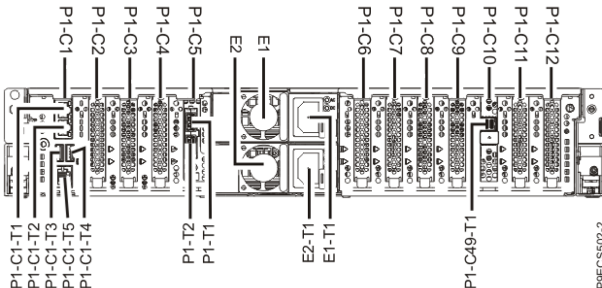
Figura 1. Vista posterior de um sistema 5105-22E, 9009-22G ou 9223-22S montado em rack com os códigos dos locais de slots PCIe4
