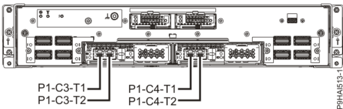
Rysunek 13. Położenie portów konsoli HMC w serwerach 9080-M9S
