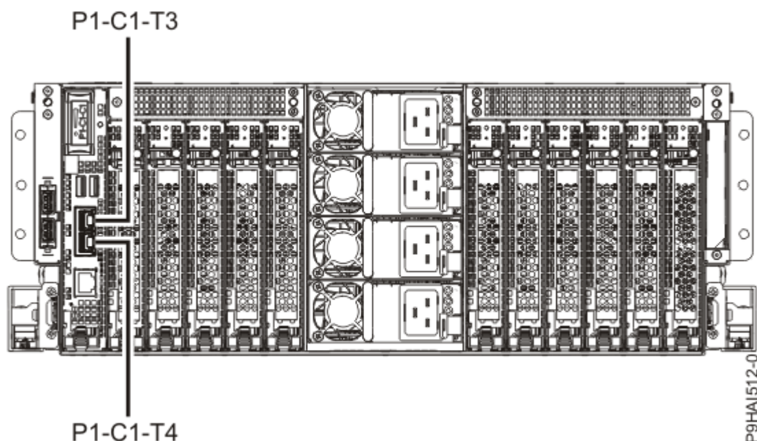
Rysunek 12. Położenie portów konsoli HMC w serwerach 9040-MR9
