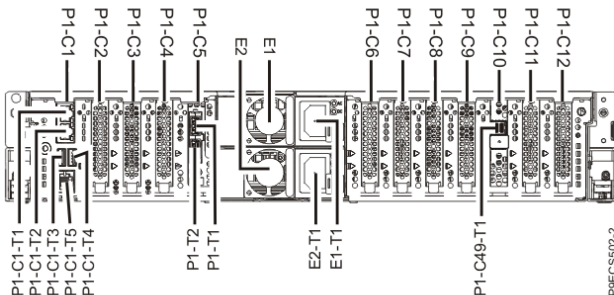
Rysunek 1. Widok z tyłu serwera stelażowego 5105-22E, 9009-22G lub 9223-22S z kodami połączenia gniazd PCIe4
