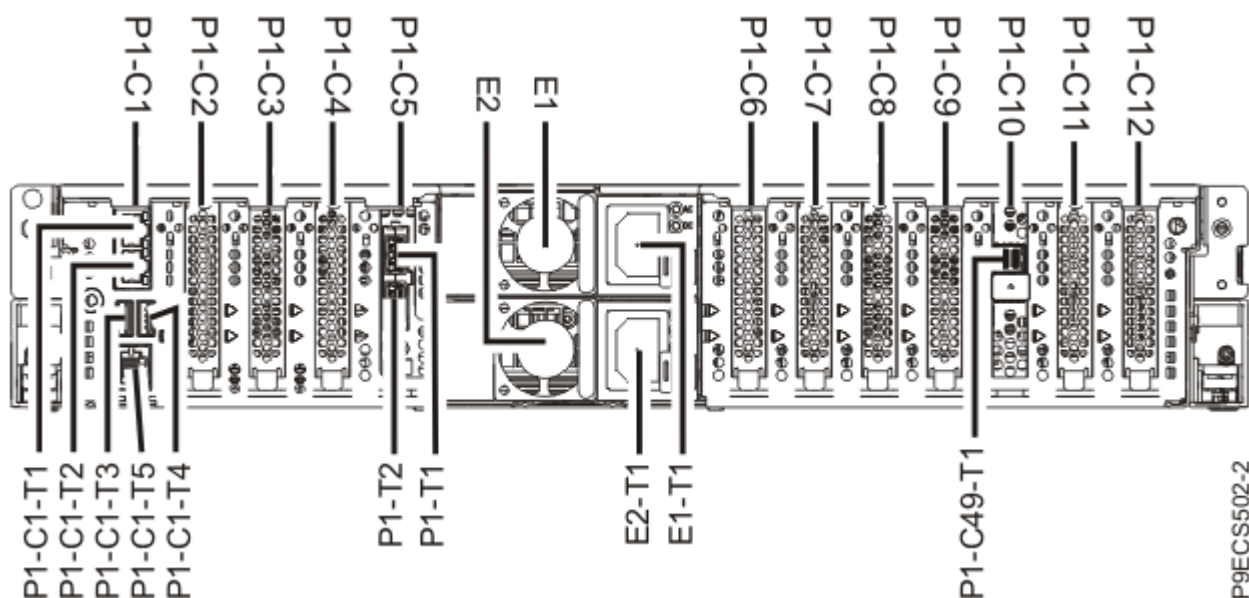
Rysunek 2. Widok z tyłu serwera stelażowego 9008-22L, 9009-22A lub 9223-22H z kodami położenia gniazd PCIe
