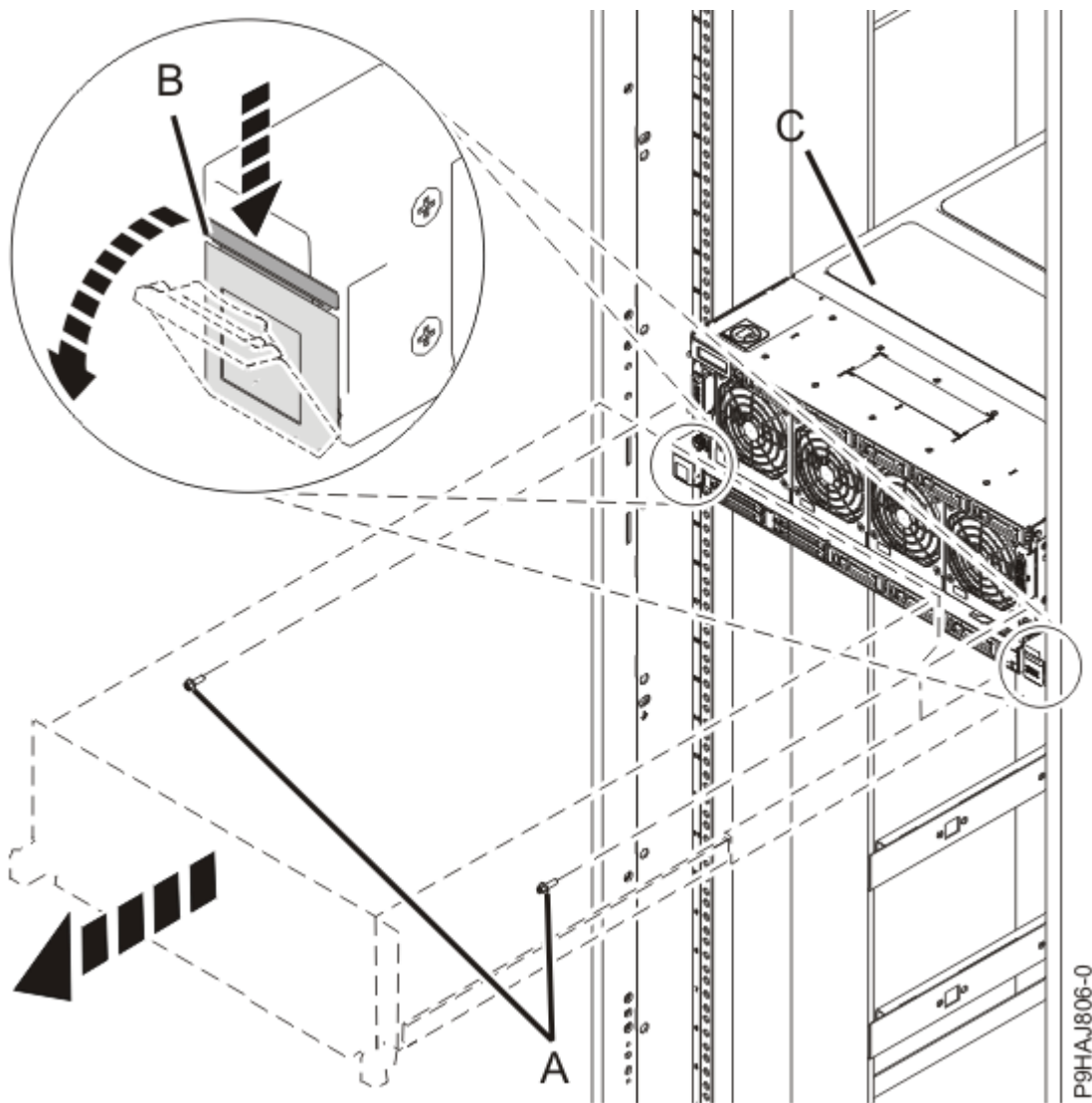
그림 2. 시스템을 서비스 위치에 배치
