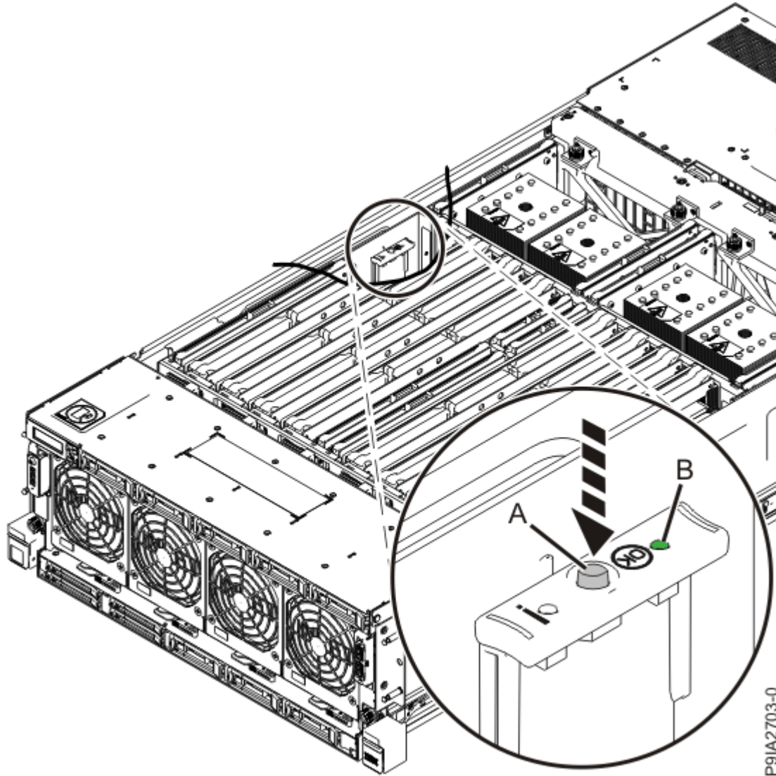
그림 4. 식별 LED 활성화
