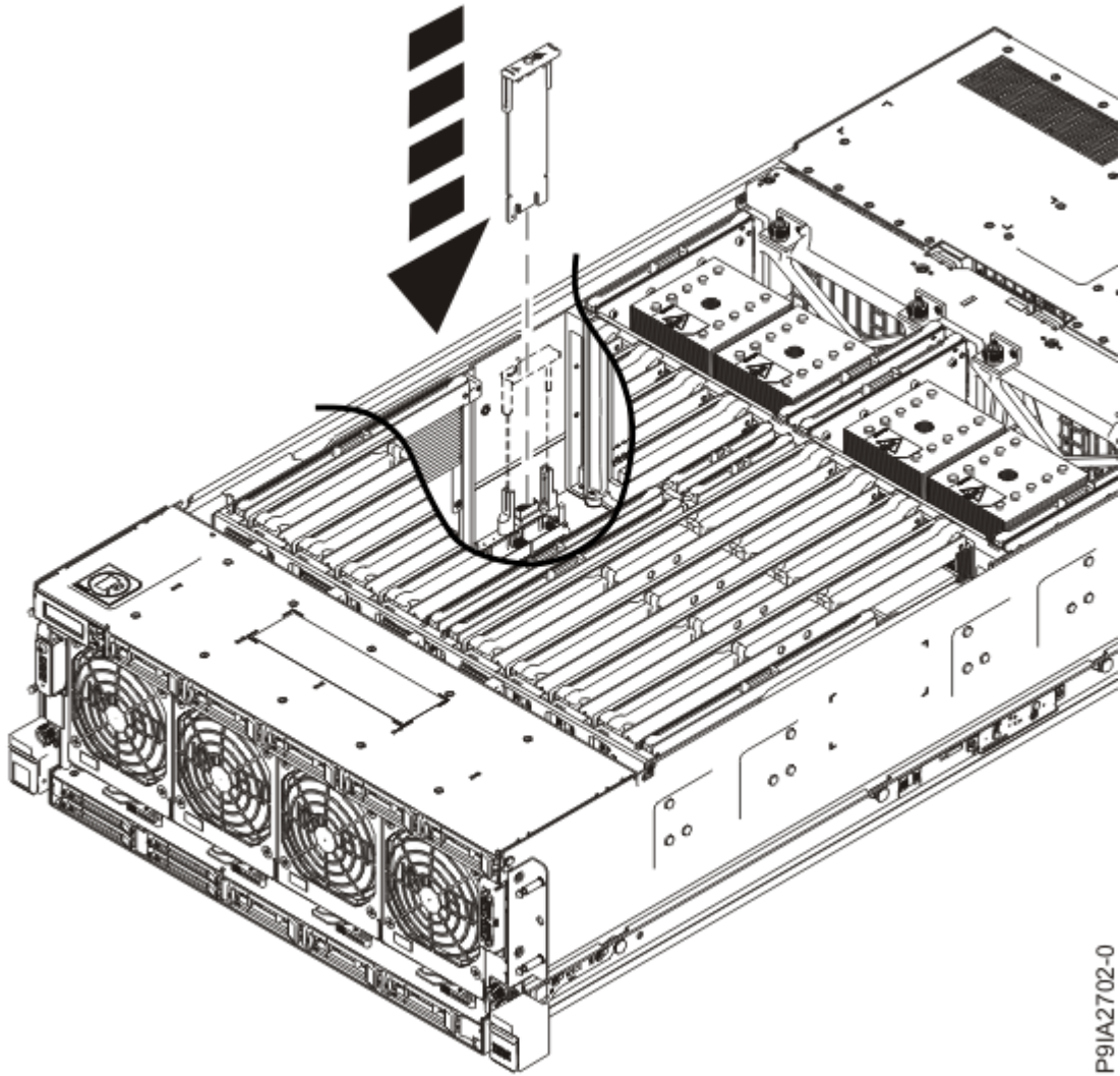
그림 8. TPM 카드 교체
