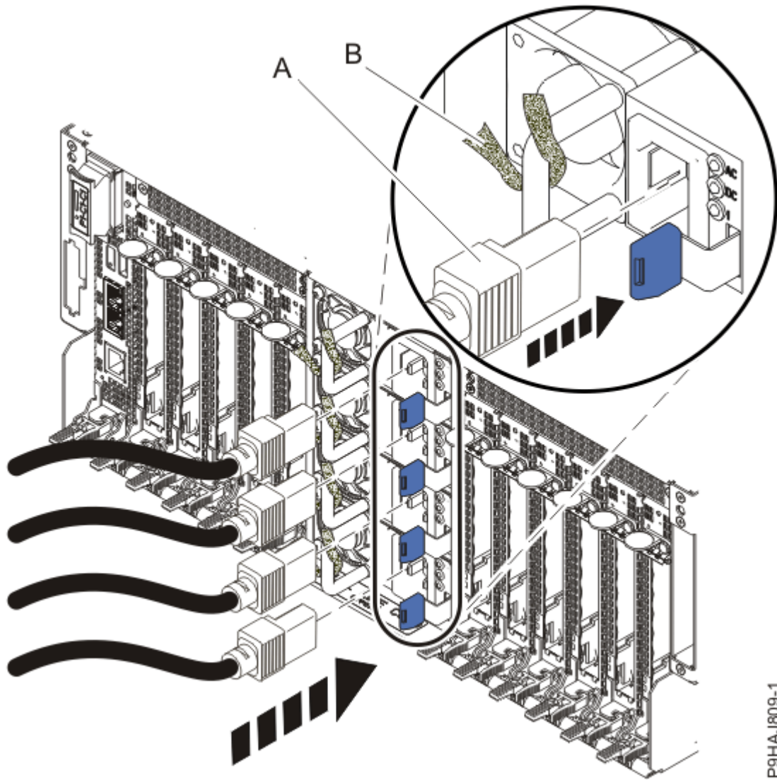
그림 12. 전원 코드 연결
