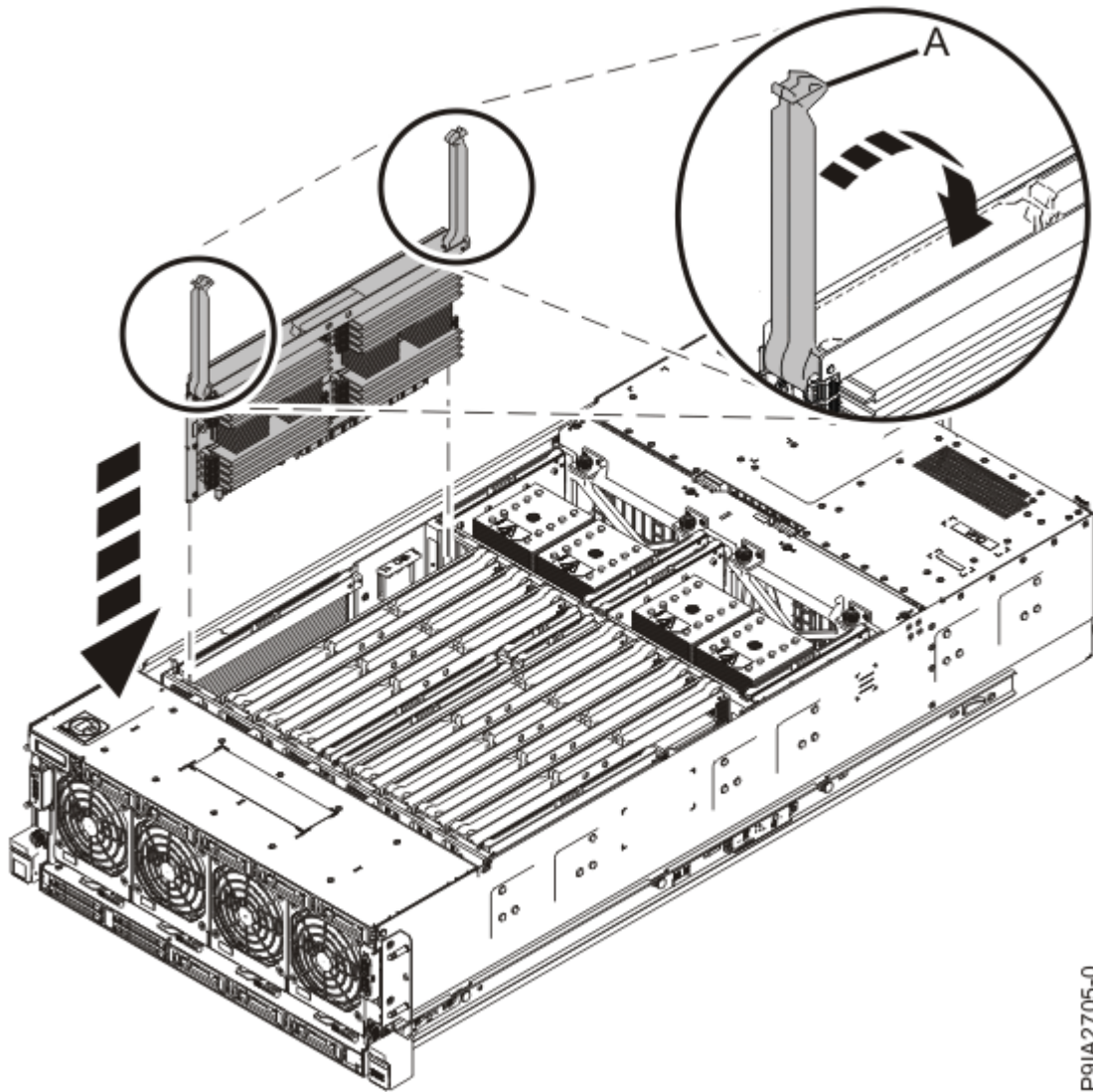
그림 9. P1-C26 위치에서 메모리 라이저 교체
