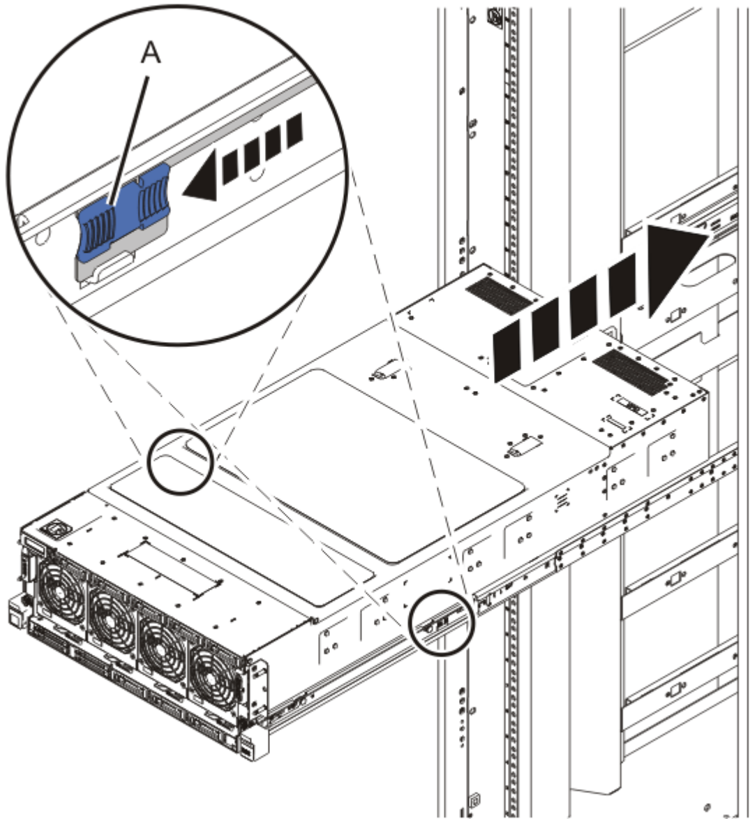
그림 11. 시스템을 작동 위치에 배치
