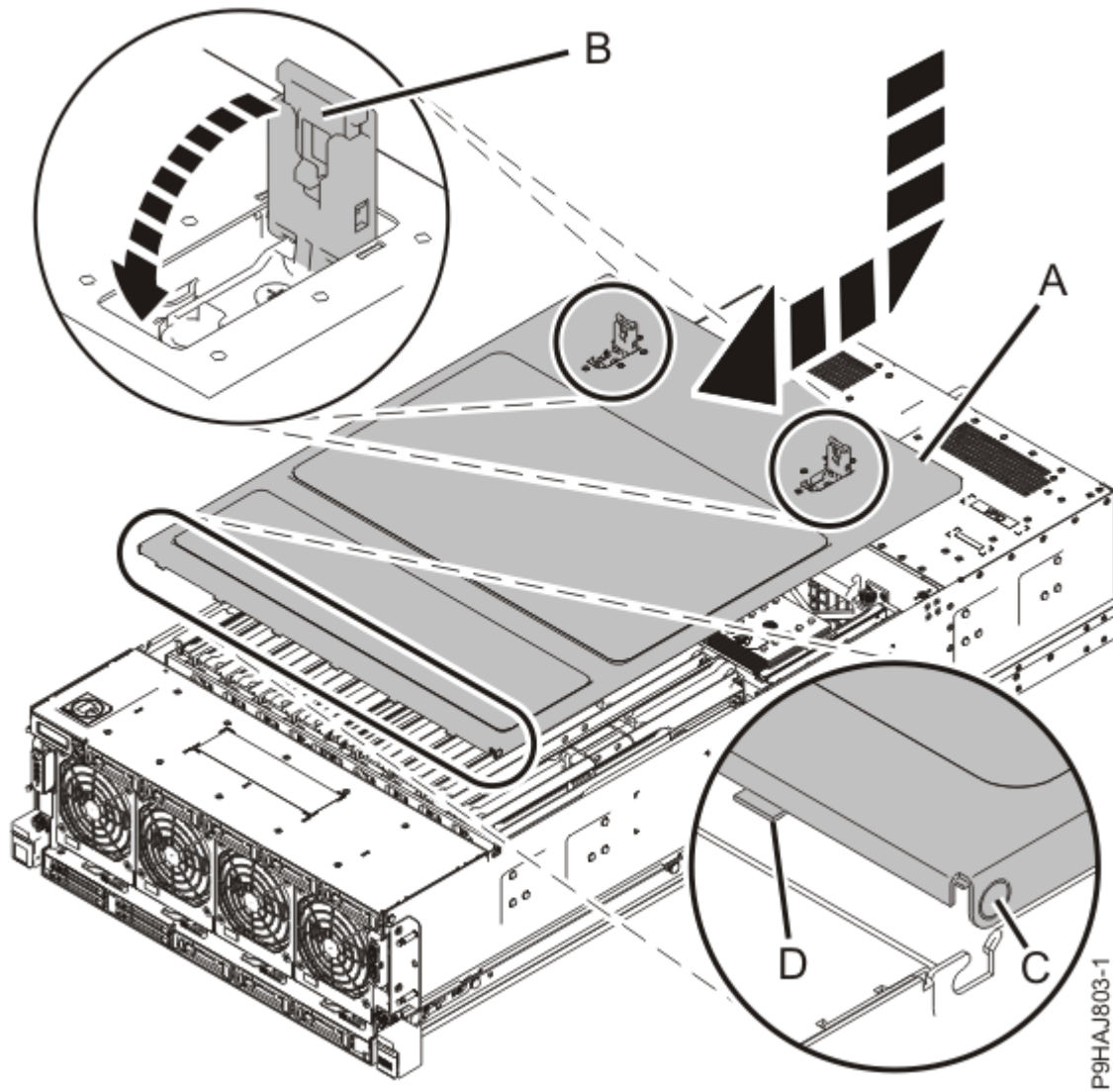
그림 10. 서비스 액세스 커버 설치
