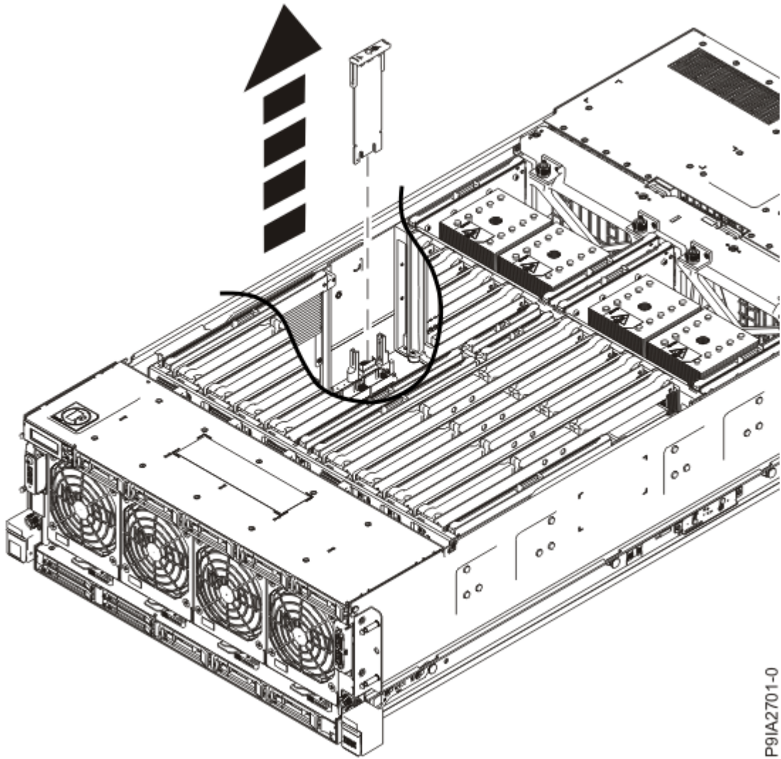
그림 7. TPM 카드 제거
