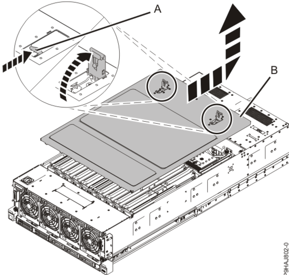
그림 3. 서비스 액세스 커버 제거
