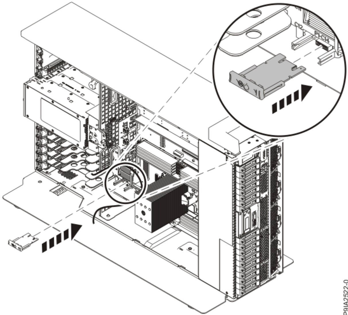
그림 13. 독립형 시스템에서 TPM 카드 교체
