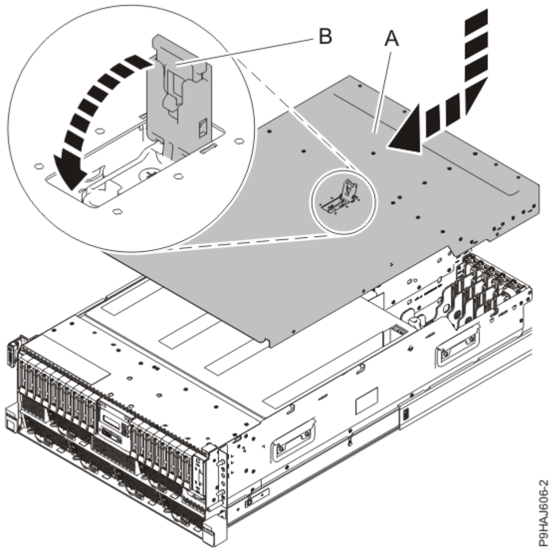
그림 14. 서비스 액세스 커버 설치
