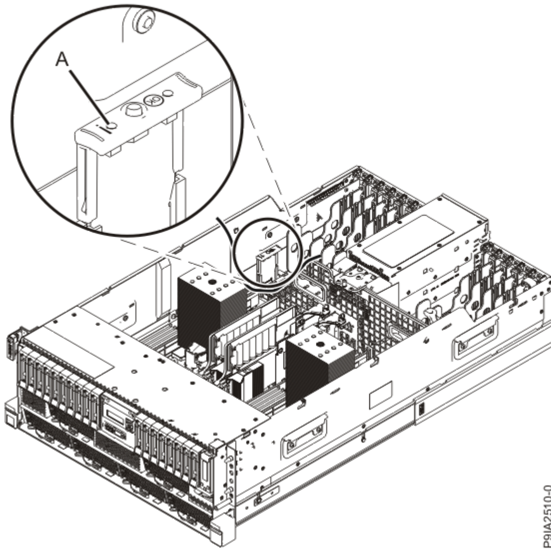
그림 8. 랙 장착 서버에서 신뢰 플랫폼 모듈 카드 서비스 표시기 LED 위치
