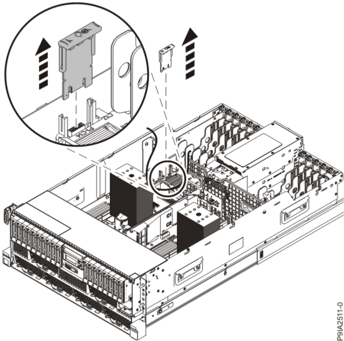
그림 10. 랙 장착형 시스템에서 TPM 카드 제거
