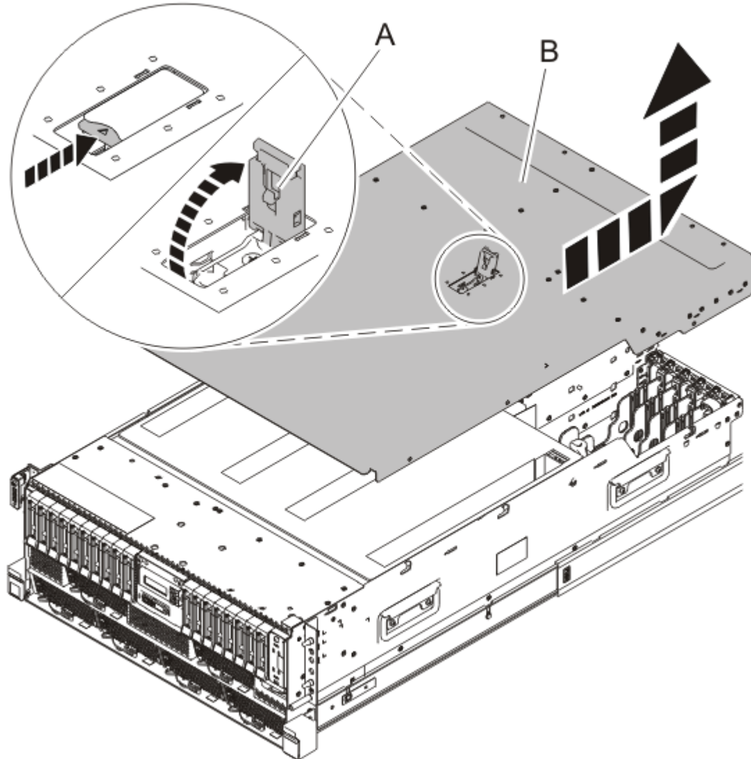
그림 4. 랙 장착형 시스템에서 서비스 액세스 커버 제거
