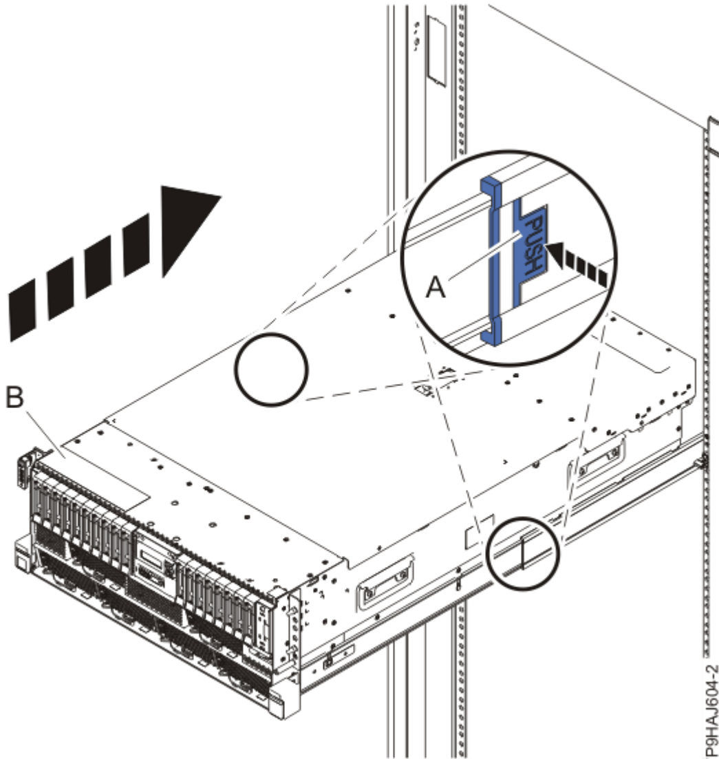
그림 16. 시스템을 작동 위치에 배치
