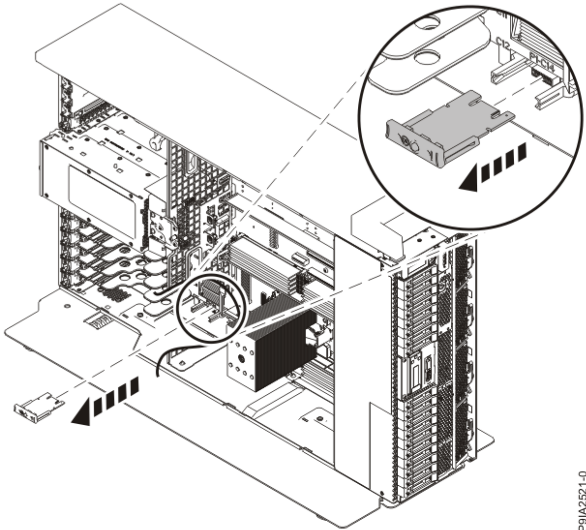
그림 11. 독립형 시스템에서 TPM 카드 제거
