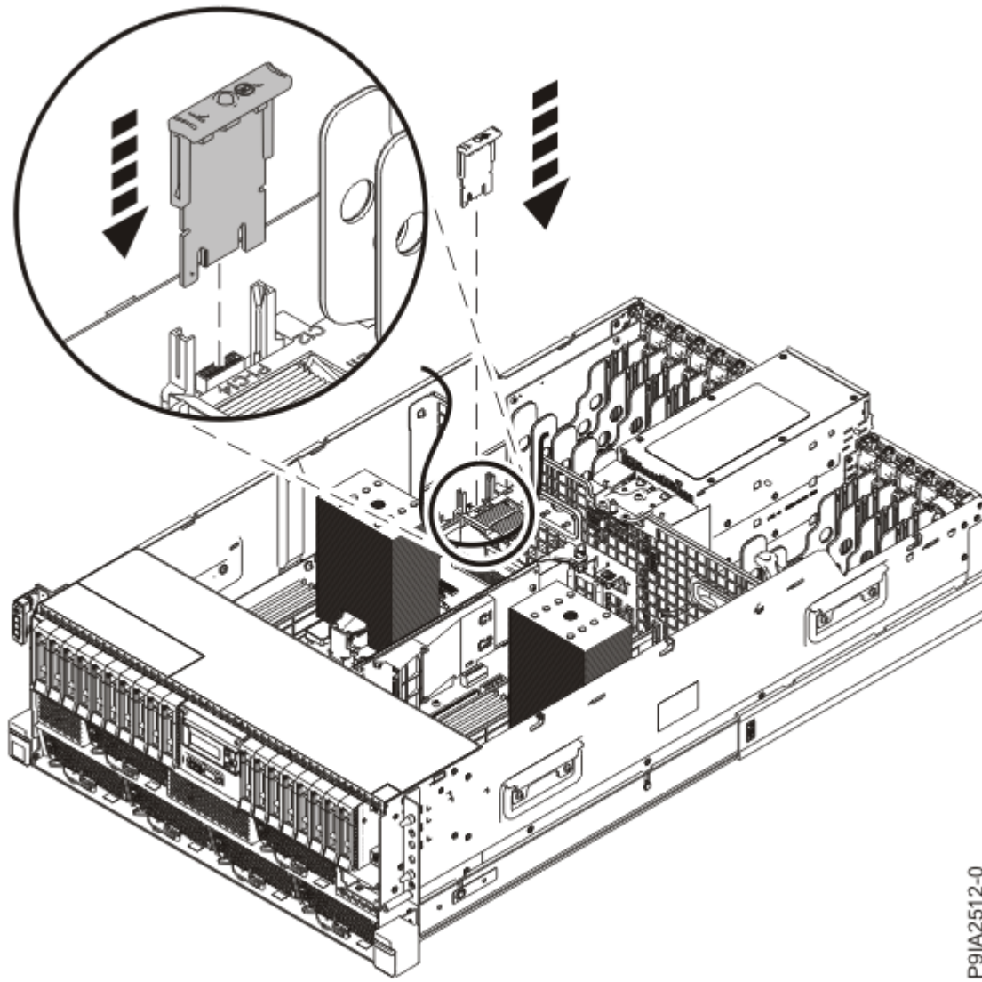
그림 12. 랙 장착형 시스템에서 TPM 카드 교체
