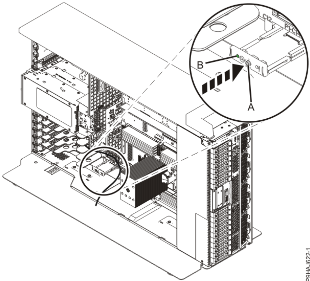
그림 7. 독립형 시스템의 식별 LED 활성화
