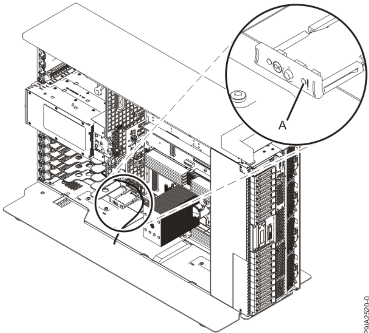
그림 9. 독립형 서버에서 신뢰 플랫폼 모듈 카드 서비스 표시기 LED 위치
