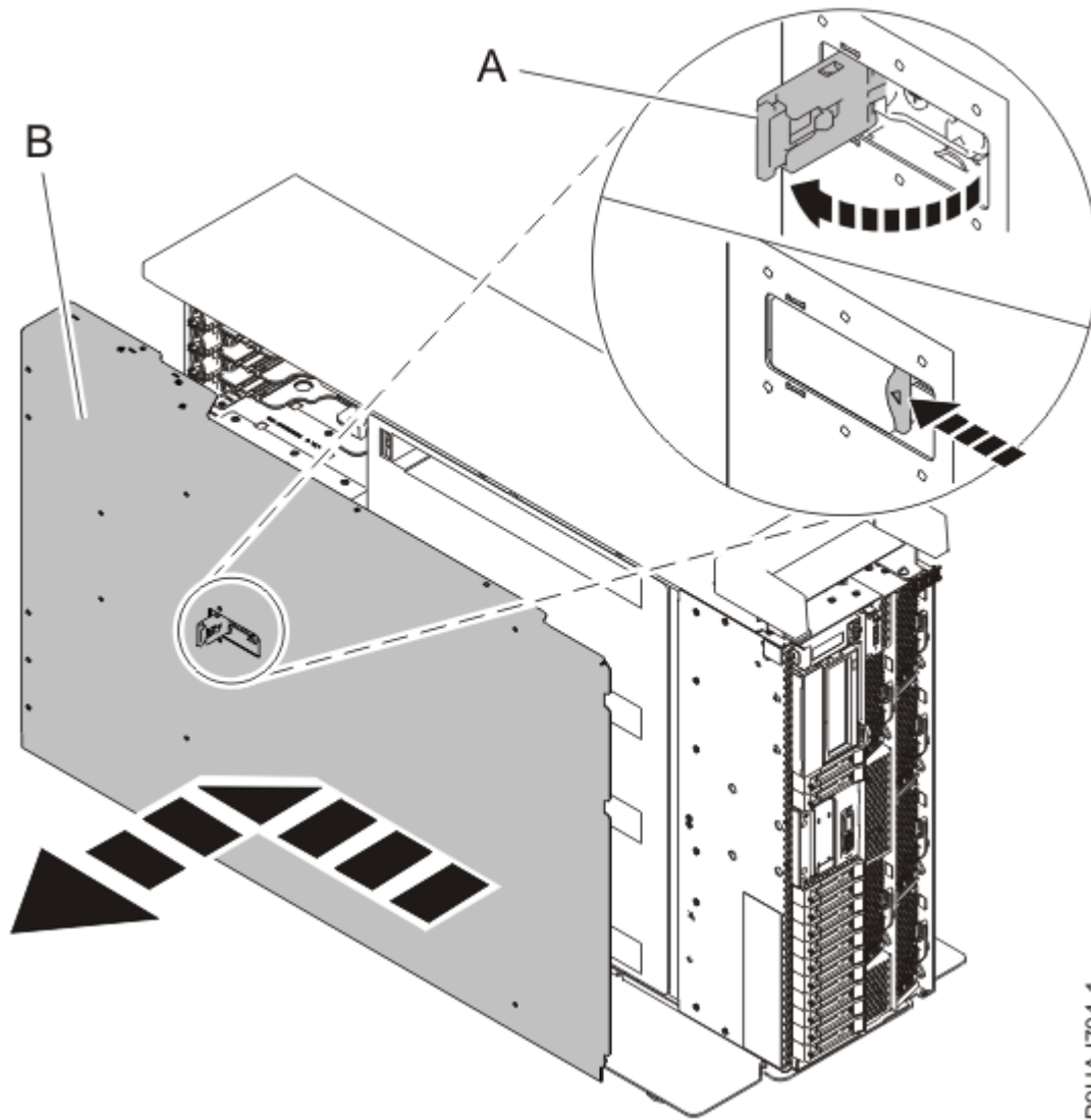
그림 5. 서비스 액세스 커버 제거
