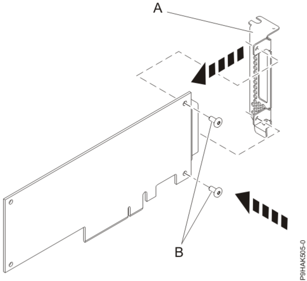
그림 21. 로우( low ) 프로파일 심압대를 어댑터에 연결
