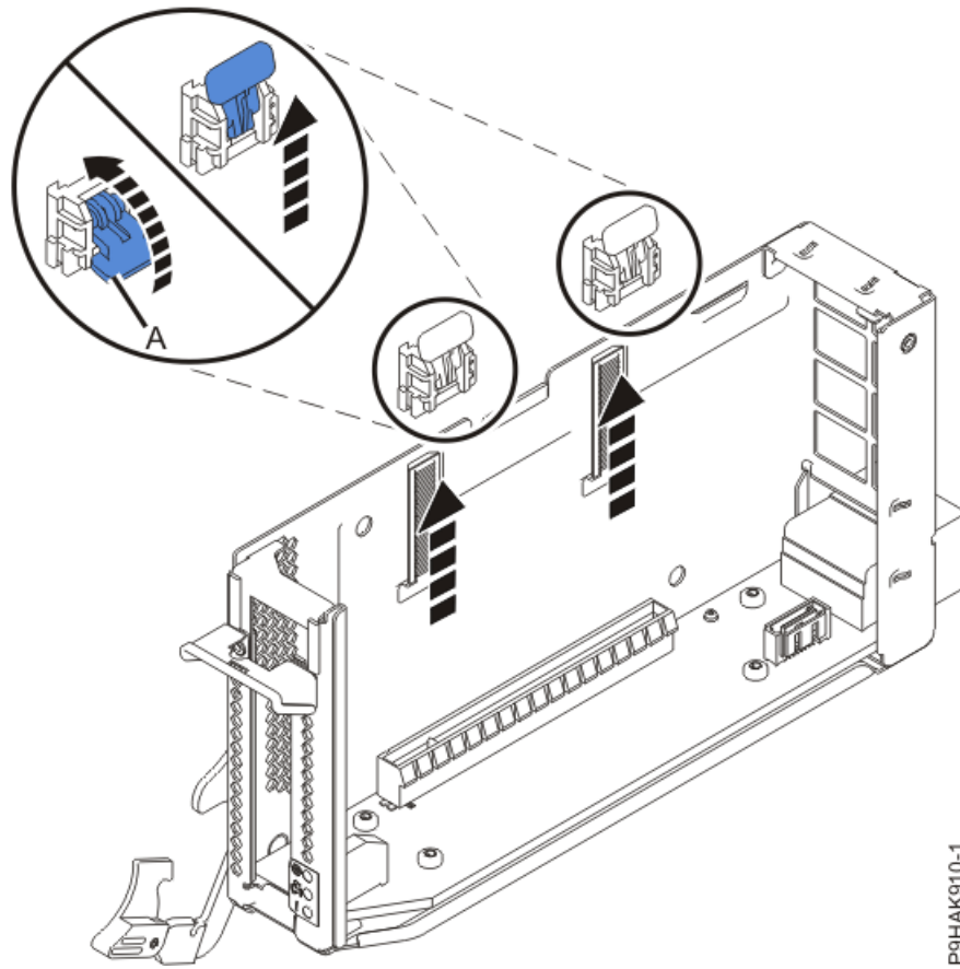
그림 10. 어댑터 고정장치를 밀어서 꺼내고 버릴 수 있도록 9080-M9S 시스템의 PCIe 어댑터 고정장치 열기
