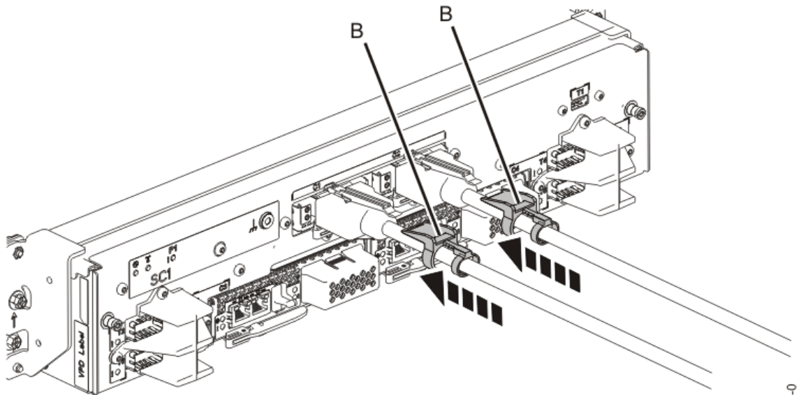
그림 16. UPIC 케이블을 시스템 제어 장치로 교체
