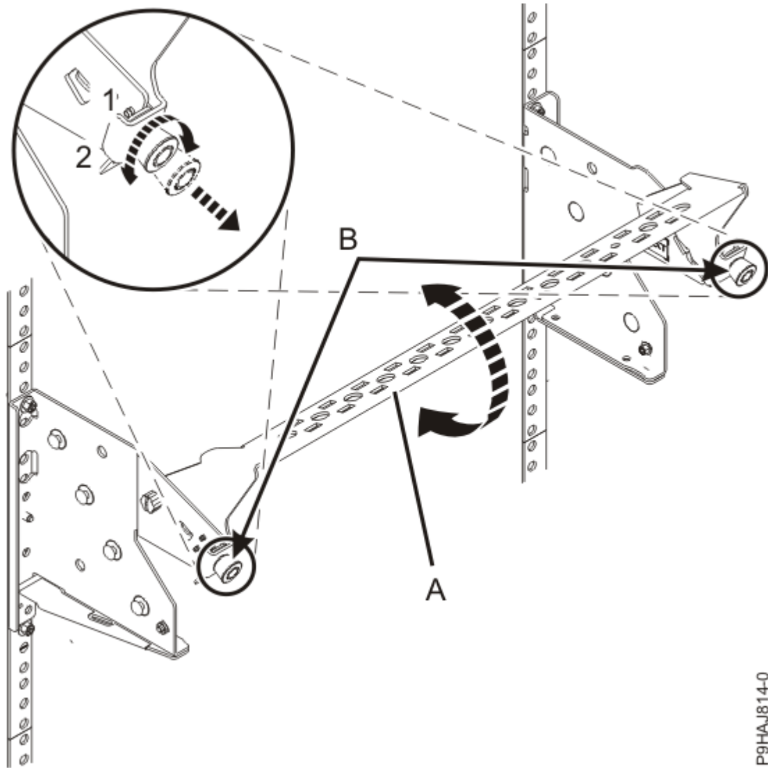
그림 5. 케이블 관리 브래킷을 서비스 위치(올린 위치)에 배치
