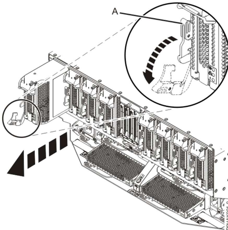
그림 6. 9080-M9S 시스템에서 어댑터 카세트 제거
