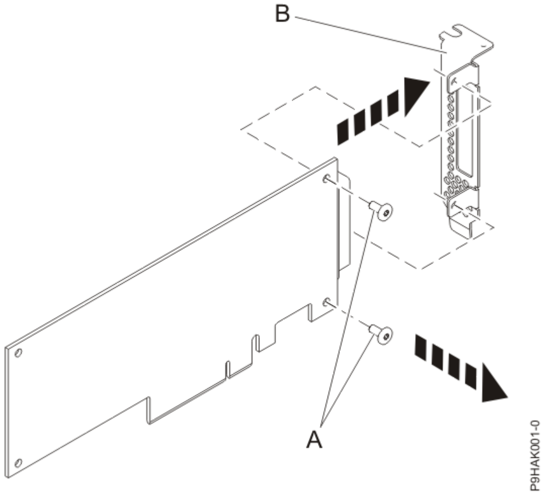
그림 18. 어댑터에서 로우(low) 프로파일 심압대 제거
