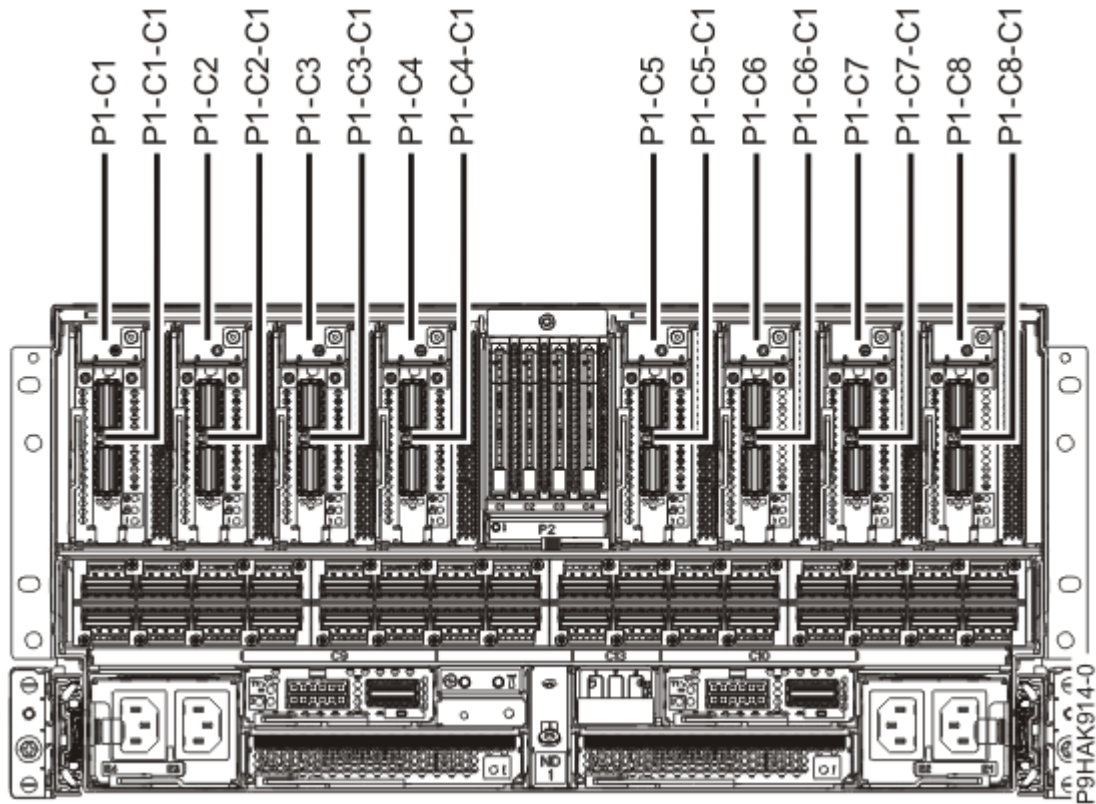
그림 1. 9080-M9S 시스템의 어댑터와 카세트 위치
