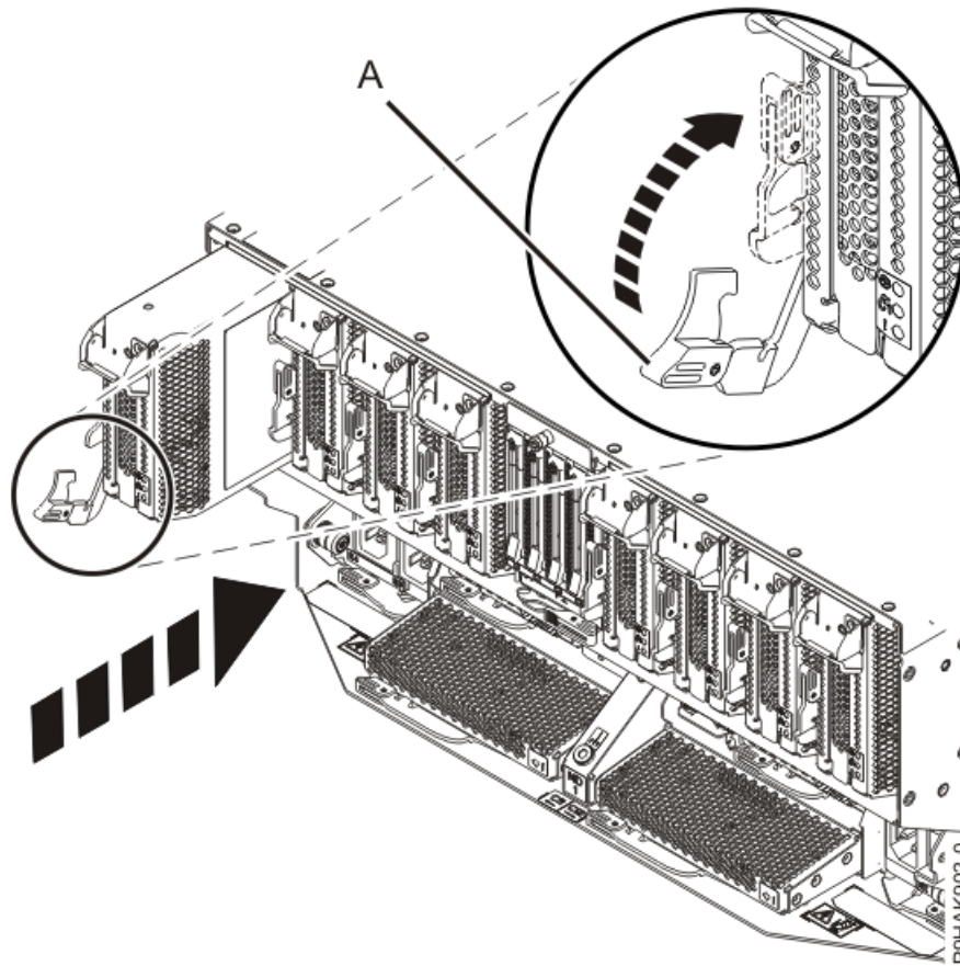
그림 14. 9080-M9S 시스템에 카세트 설치
