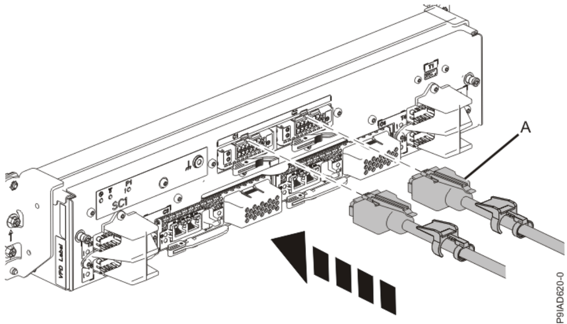
그림 16. UPIC 케이블을 시스템 제어 장치로 교체
