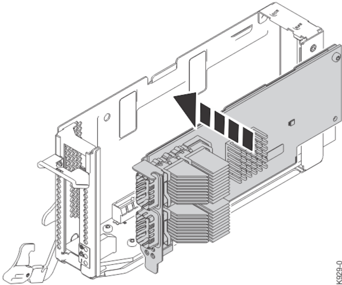
그림 11. 9080-M9S 시스템의 카세트에 어댑터 설치
