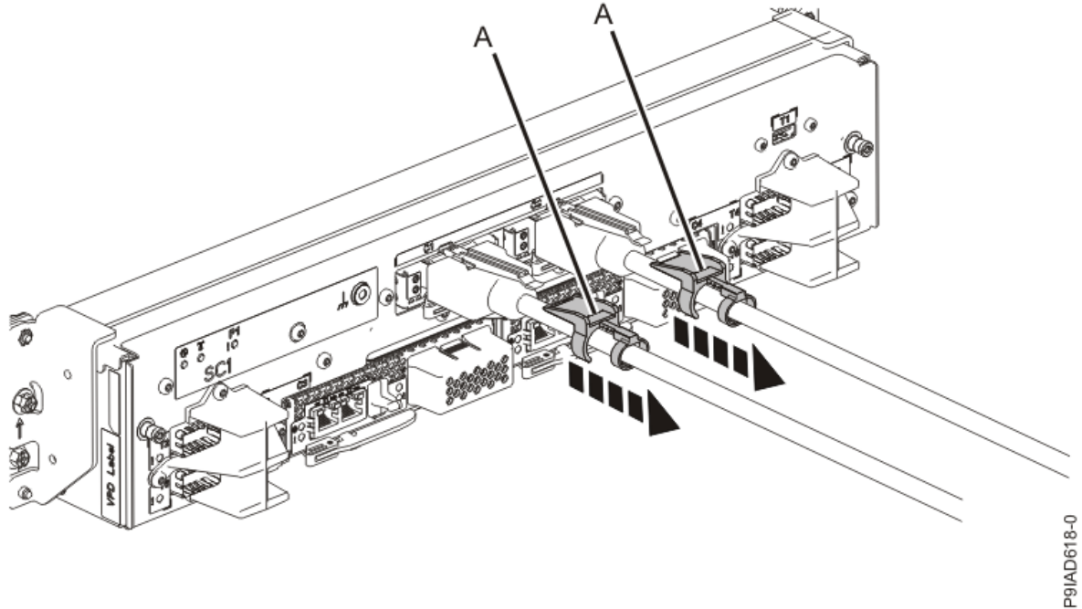
그림 3. UPIC 케이블 잠금 장치 제거
