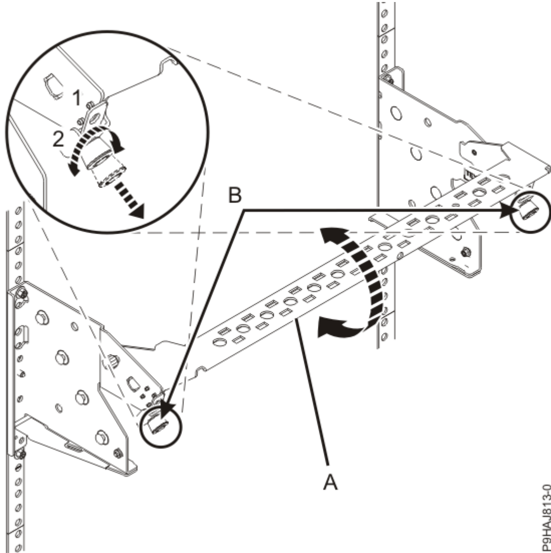
그림 15. 케이블 관리 브래킷을 하단 작동 위치에 배치
