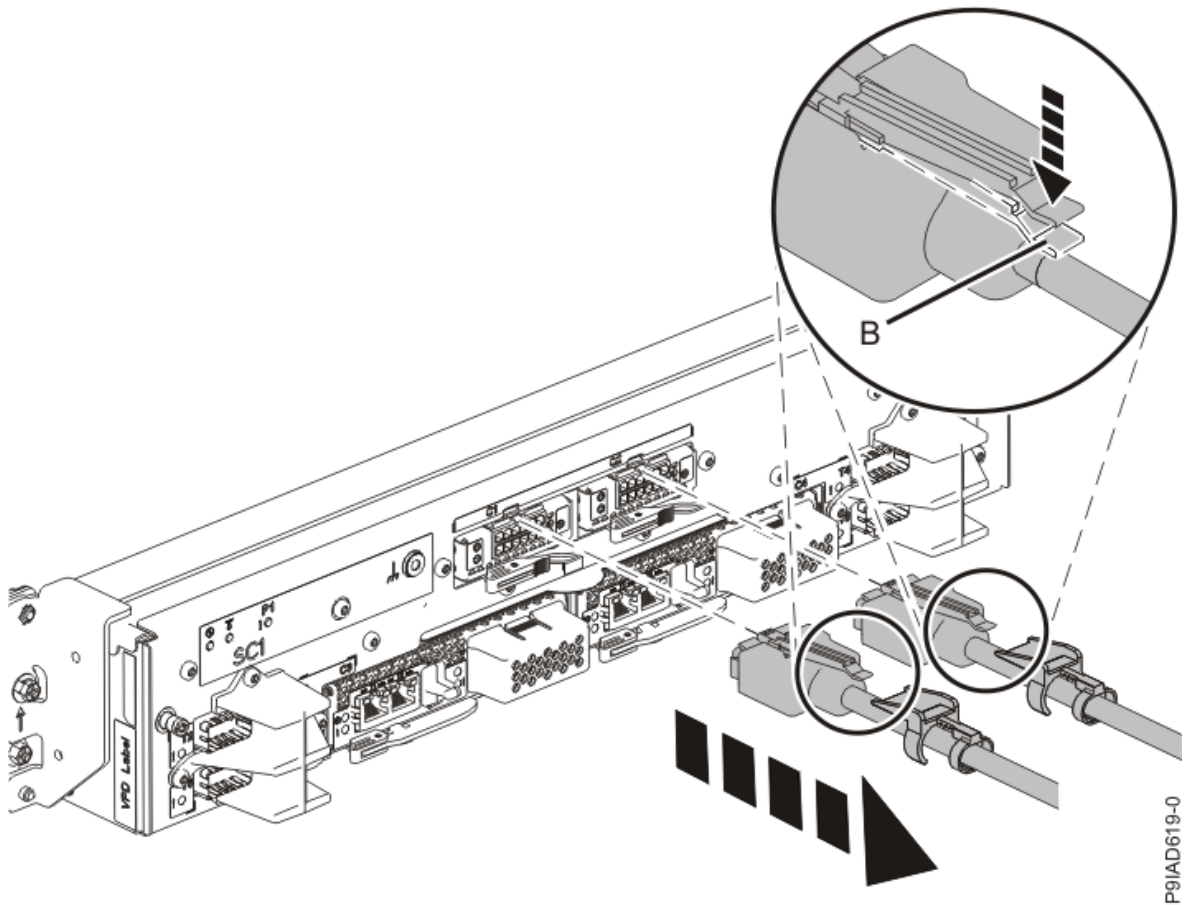
그림 4. 시스템 제어 장치에서 UPIC 케이블 제거
