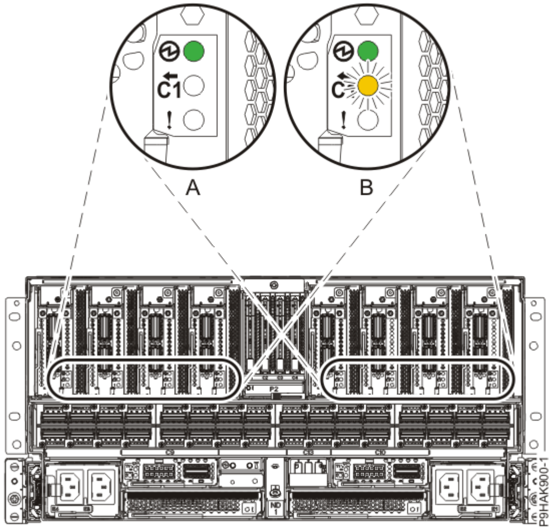
그림 2. 9080-M9S 시스템의 어댑터 LED 위치
