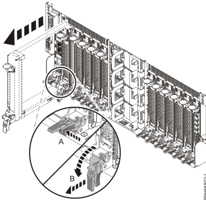
그림 29. 9040-MR9 시스템에서 어댑터 카세트 제거
