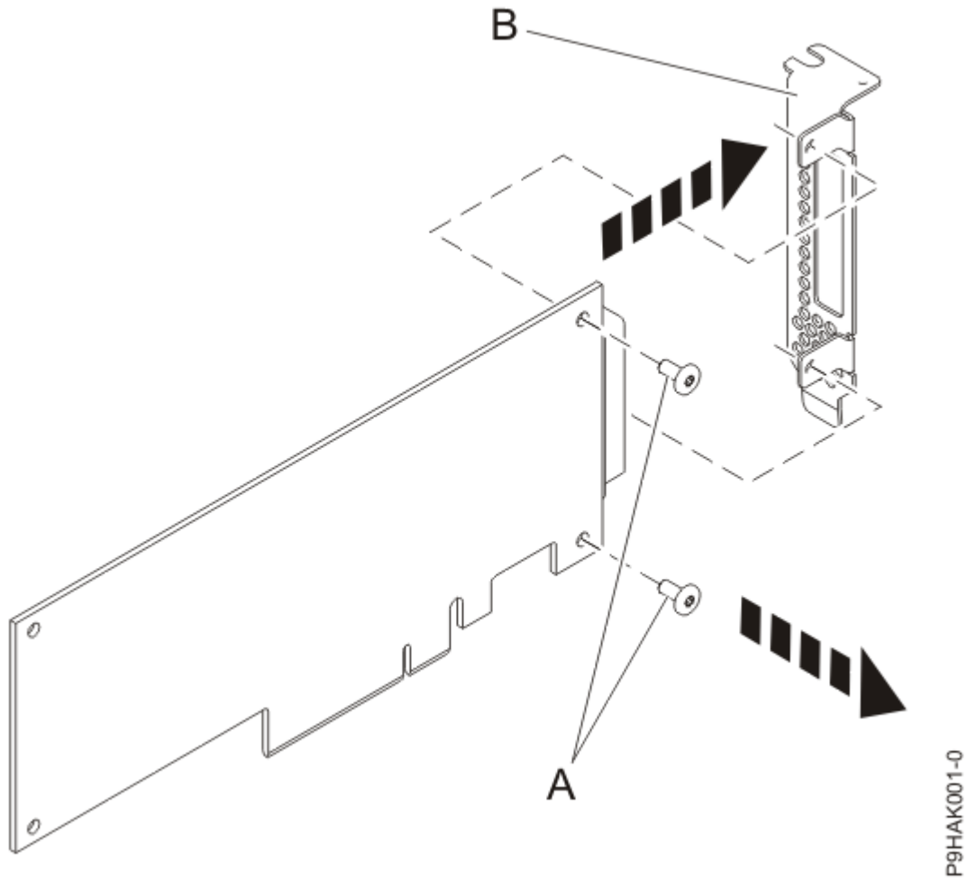
그림 36. 어댑터에서 로우(low) 프로파일 심압대 제거
