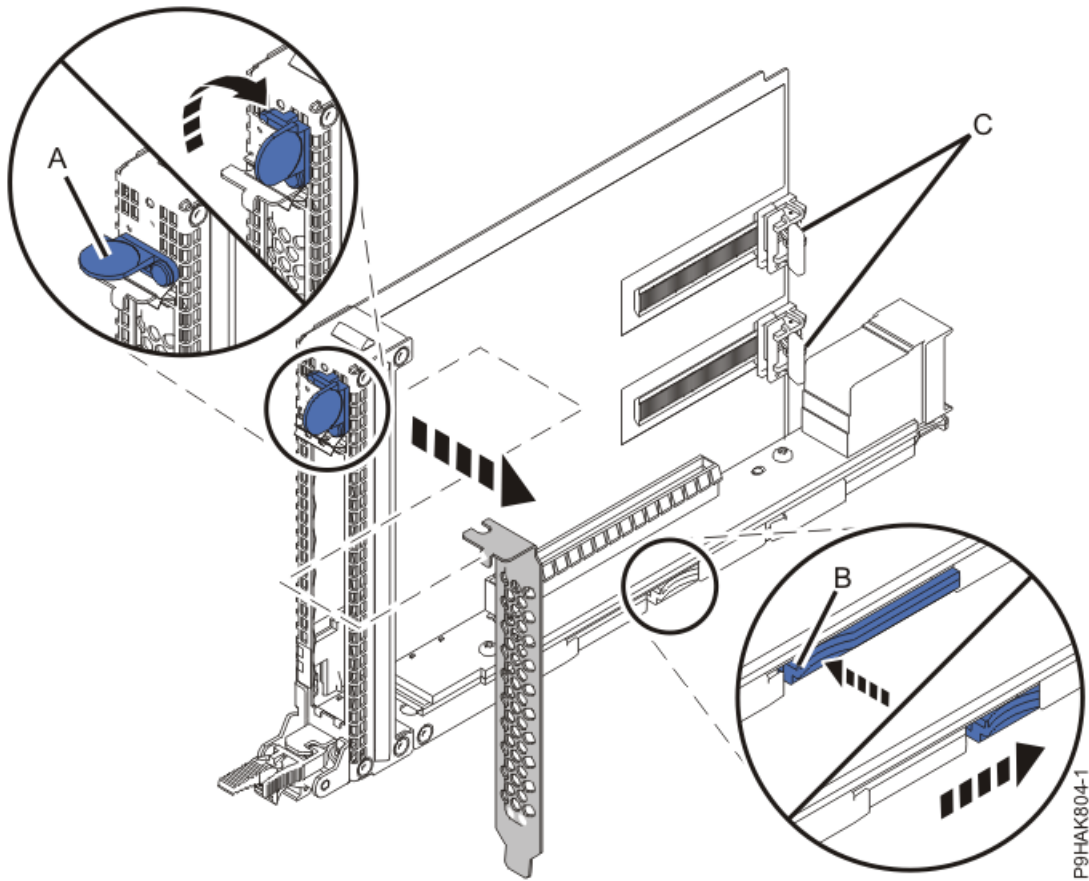
그림 5. 9040-MR9 시스템의 카세트에서 심압대 필러 제거
