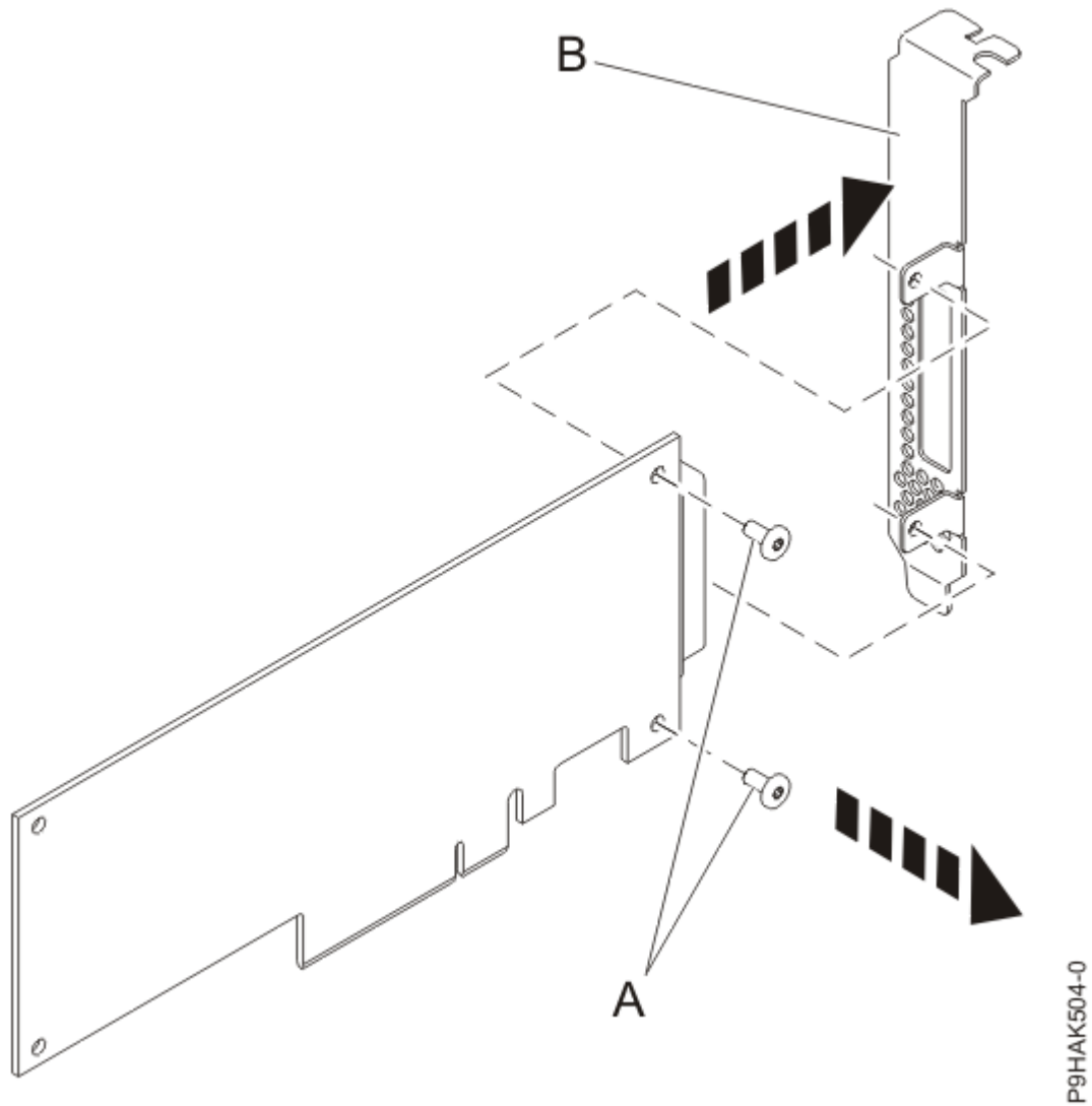
그림 38. 새 어댑터에서 하이(high) 프로파일 심압대 제거
