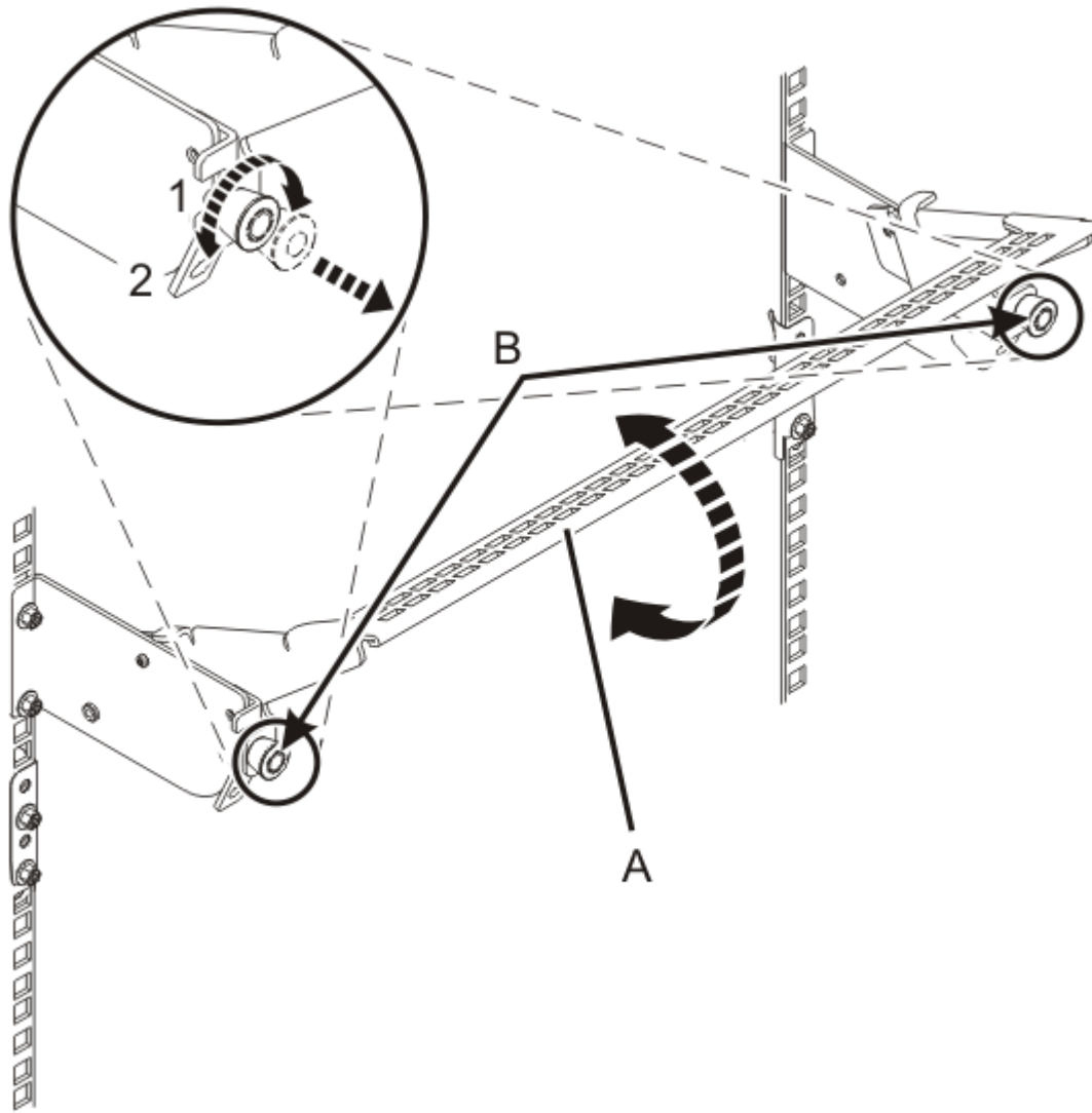
그림 12. 케이블 관리 브래킷을 하단 작동 위치에 배치
