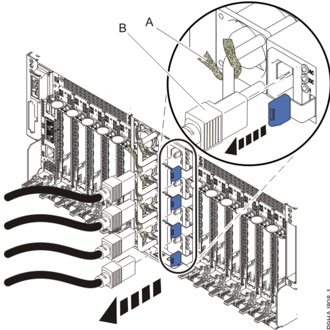
그림 2. 전원 코드 제거
