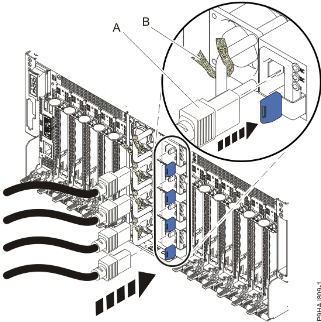
그림 34. 전원 코드 연결
