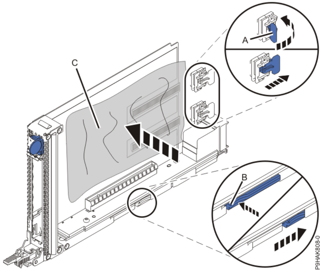
그림 20. 9040-MR9 카세트의 스트립 위에 ESD 안전 시트 두기
