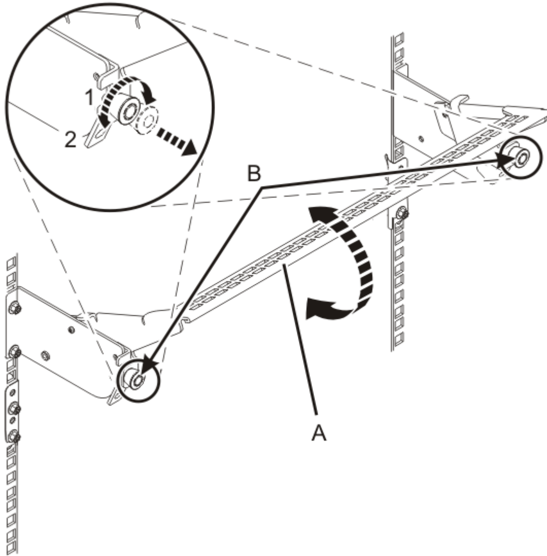
그림 28. 케이블 관리 브래킷을 서비스 위치(올린 위치)에 배치
