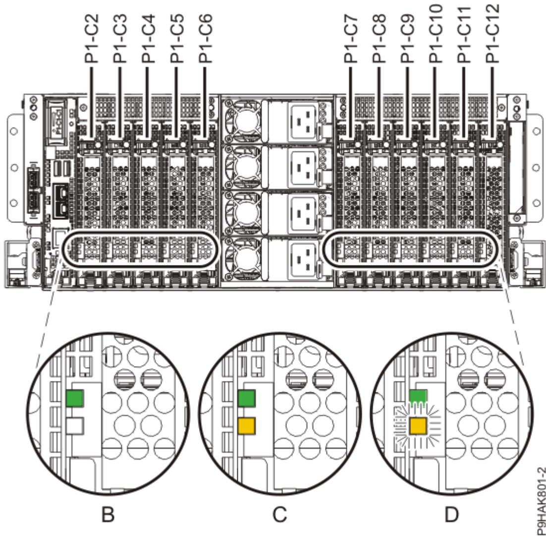
그림 26. 9040-MR9 시스템의 어댑터 슬롯 및 LED 위치
