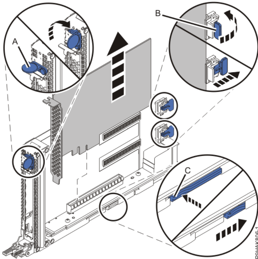
그림 18. 9040-MR9 시스템의 카세트에서 어댑터 제거
