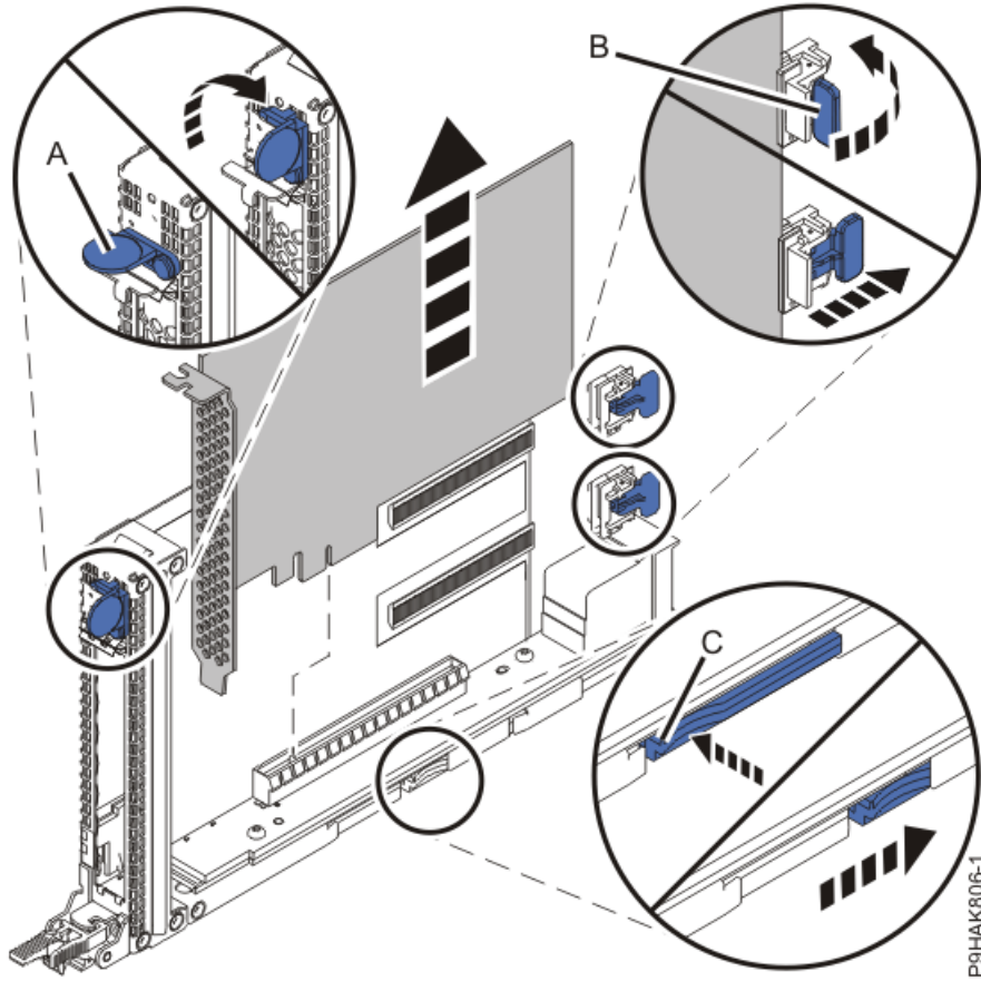
그림 30. 9040-MR9 시스템의 카세트에서 어댑터 제거
