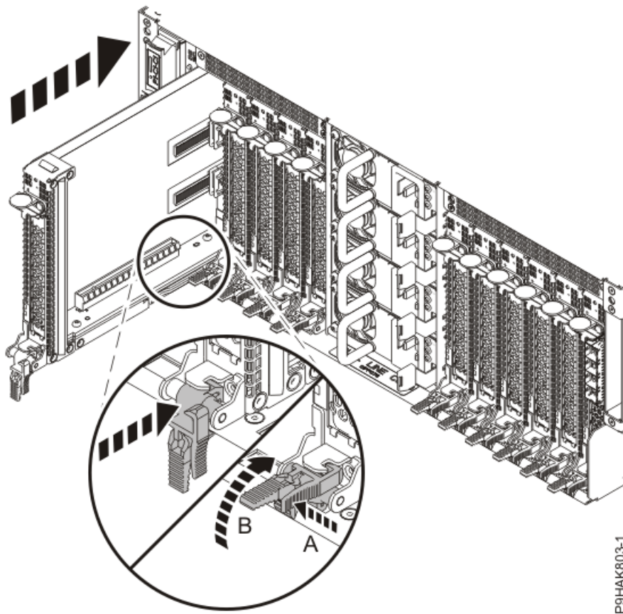
그림 33. 9040-MR9 시스템에 카세트 설치
