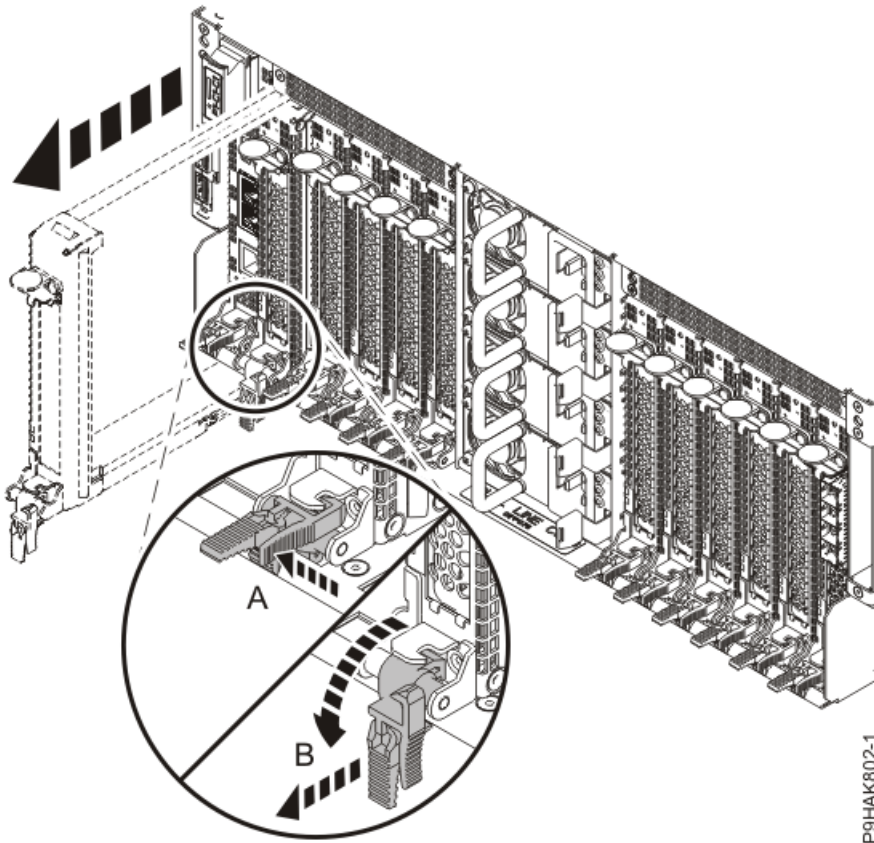
그림 17. 9040-MR9 시스템에서 어댑터 카세트 제거
