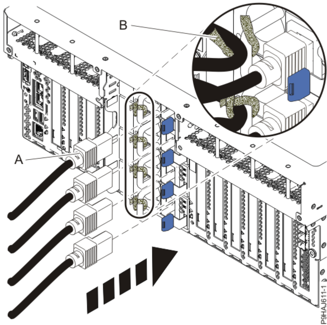
그림 11. 전원 코드 연결
