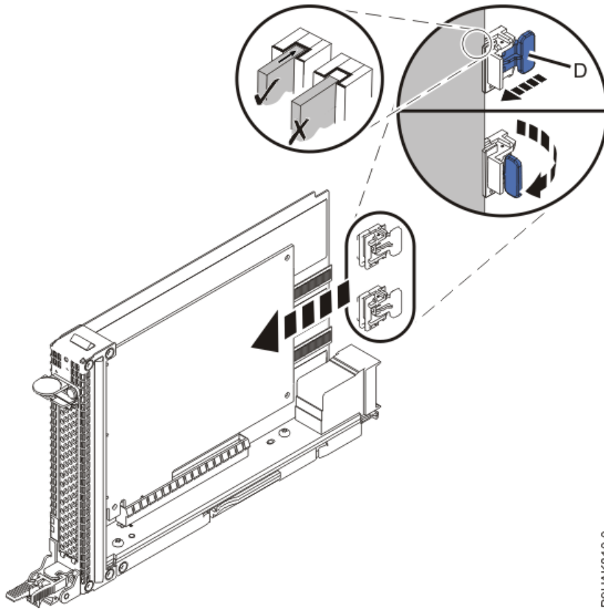
그림 22. 9040-MR9 시스템의 어댑터 고정 장치가 있는 어댑터 고정
