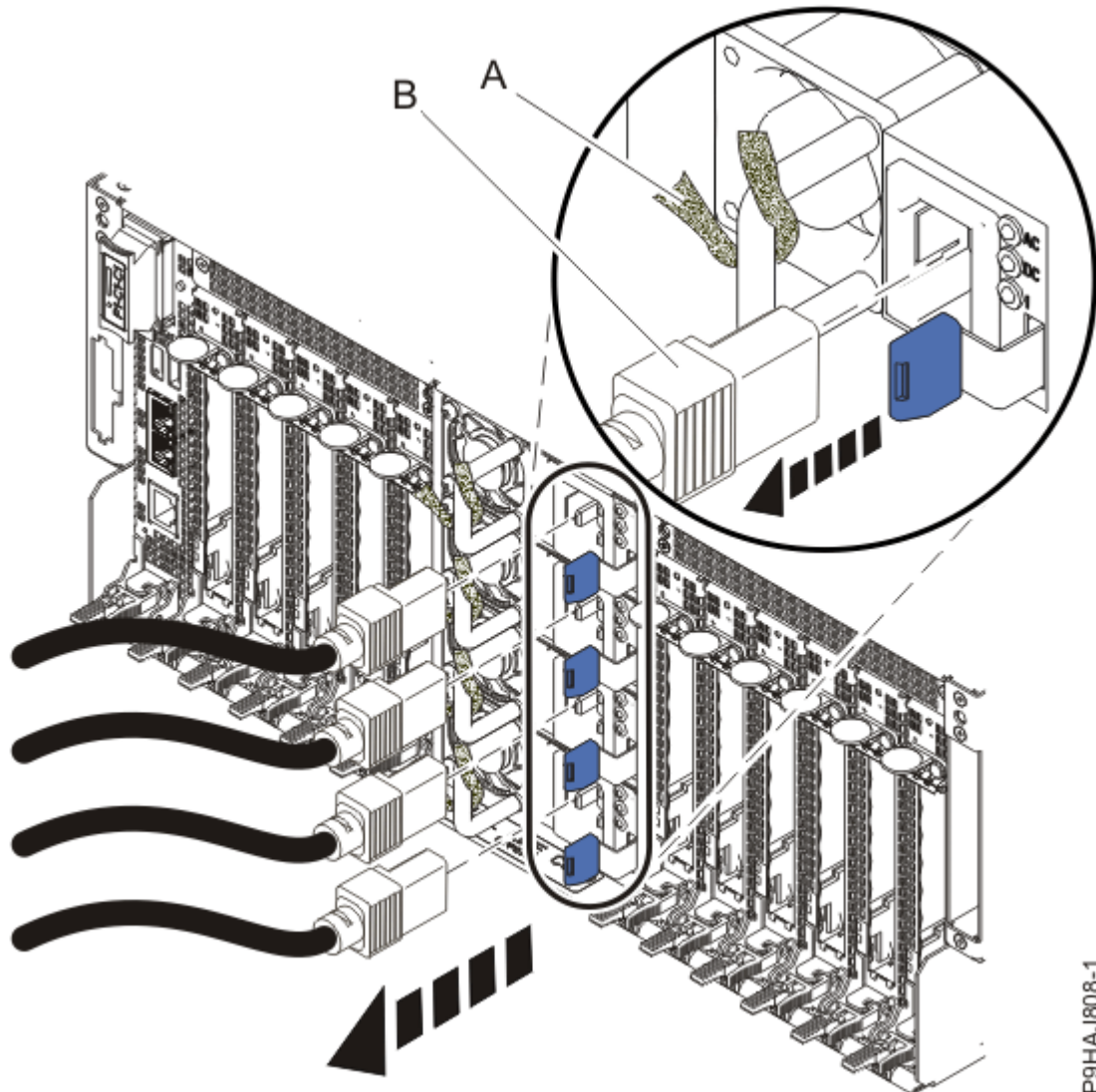
그림 14. 전원 코드 제거
