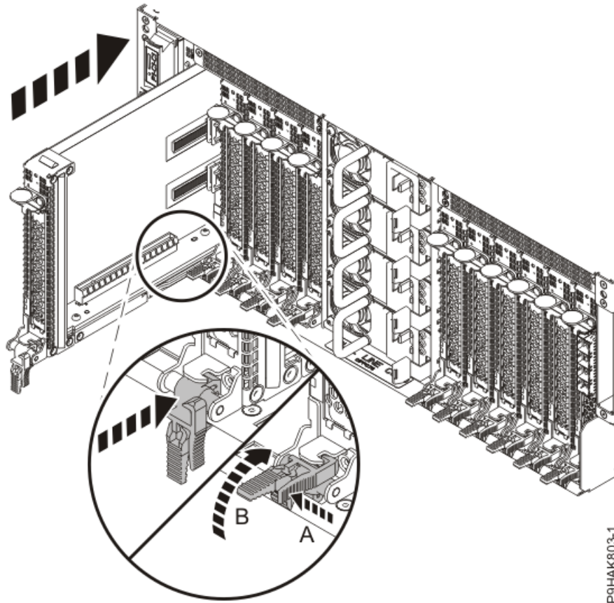
그림 24. 9040-MR9 시스템에 카세트 설치
